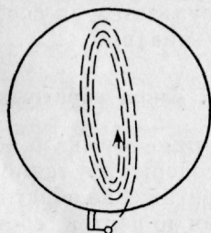
Рис. 5. Учет сопротивления воздуха по Гуку
