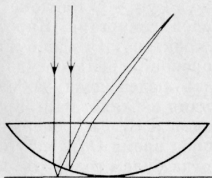
Рис. 1. Образование колец Ньютона
