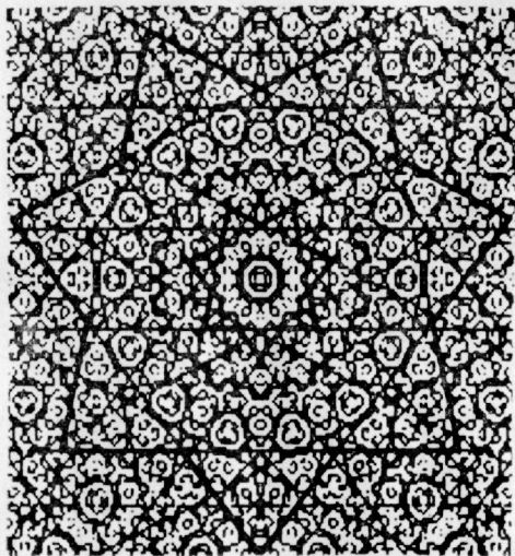
Рис. 41. Стохастическая паутина
