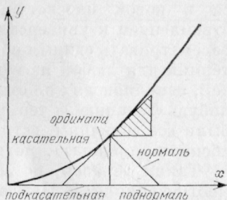
Рис. 8. Инфинитезимальный треугольник Паскаля и различные функции
