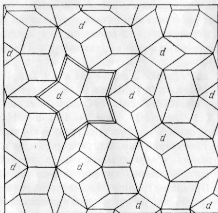
Рис. 38. Построение одномерного разбиения Пенроуза и двумерный квазикристалл
