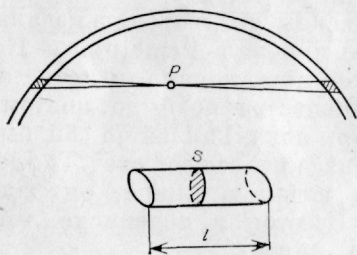
Рис. 6. Притяжение шарового слоя по Ньютону
