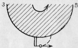
Рис. 2. Траектория в не- вращающемся простран- стве
