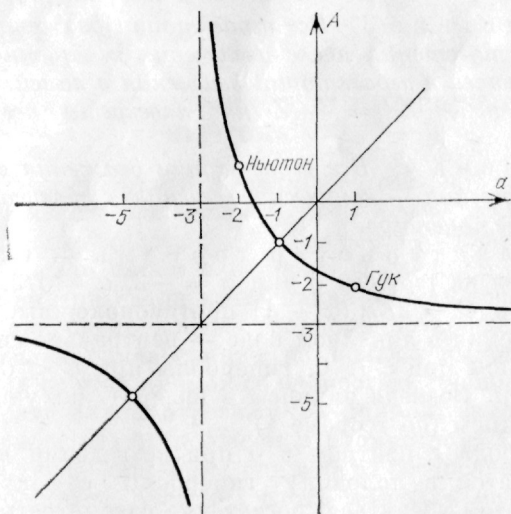
Рис. 36. Двойственные аи коны притяжения
