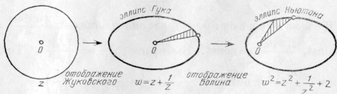
Рис. 35. Эллипсы Гука и Ньютона
