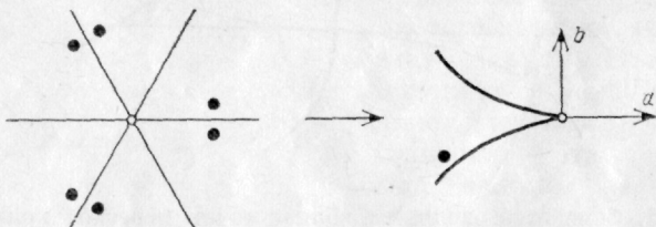
Рис. 19. Группа отражений, ее зеркала, орбита и дискриминант
