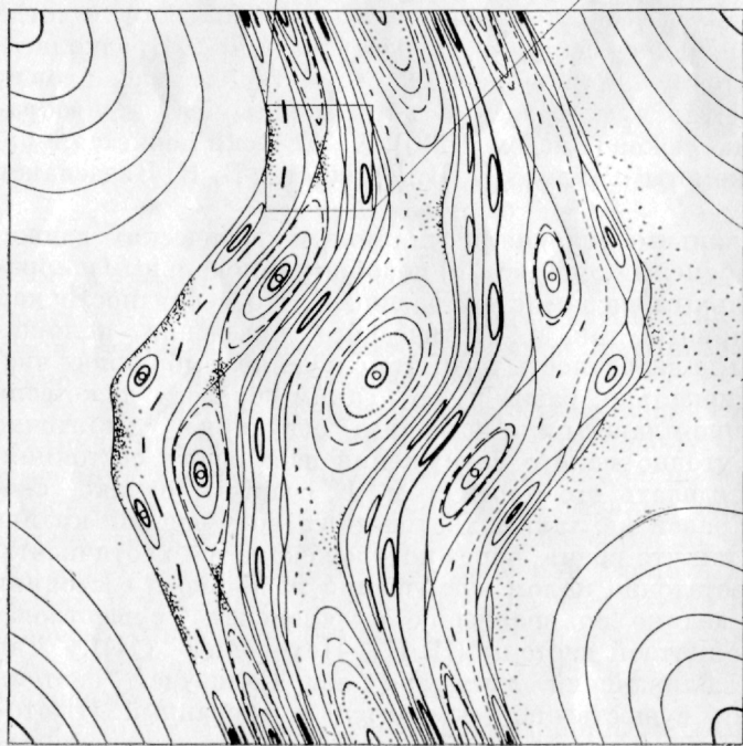
Рис. 26. Регулярные и хаотические орбиты
