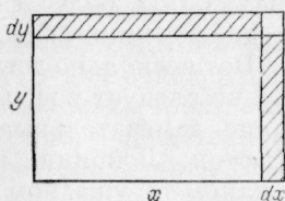
Рис. 9. Формула Лейбница
