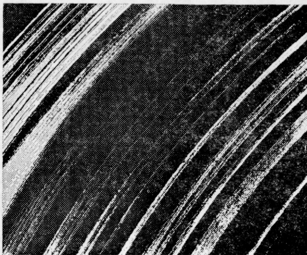
Рис. 25. Кольцо B Сатурна (участок около 6000 км, т. е. четверть ширины кольца B )
