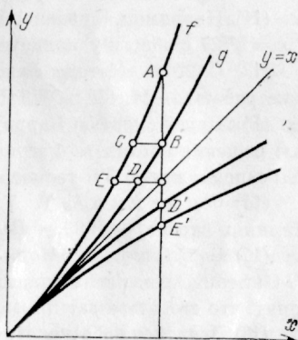
Рис. 37. Вычисление предела |AB| / |D'E|
