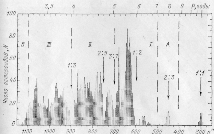
Рис. 24. Люки Кирквуда
