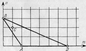
Рис. 7. Многоугольник Ньютона
