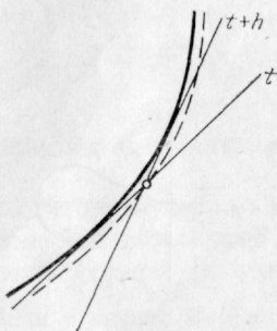
Рис. 33. Огибающая алгебраического семейства прямых алгебраична
