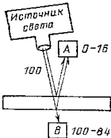
Рис. 4. Эксперимент для измерения частичного отражения света от
