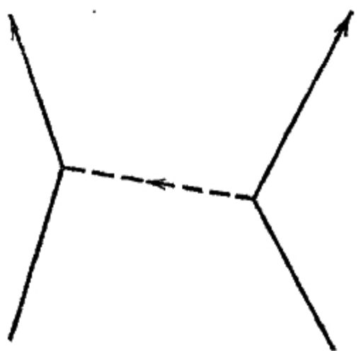
Рис. 82. Диаграмма, изображающая два кварка, которые обмениваются глюоном. Она настолько
