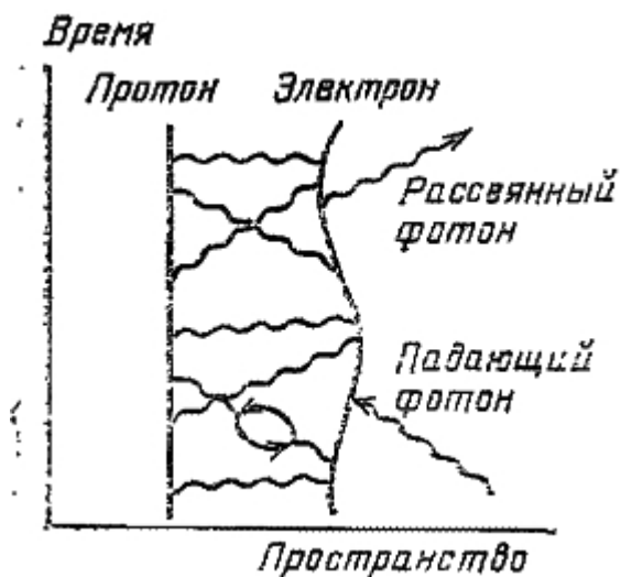
Рис. 66. Рассеяние света электроном атома — это явление, лежащее в основе частичного отражения света стеклом. Диаграмма показывает один из способов, которым такое событие может произойти в атоме водорода
