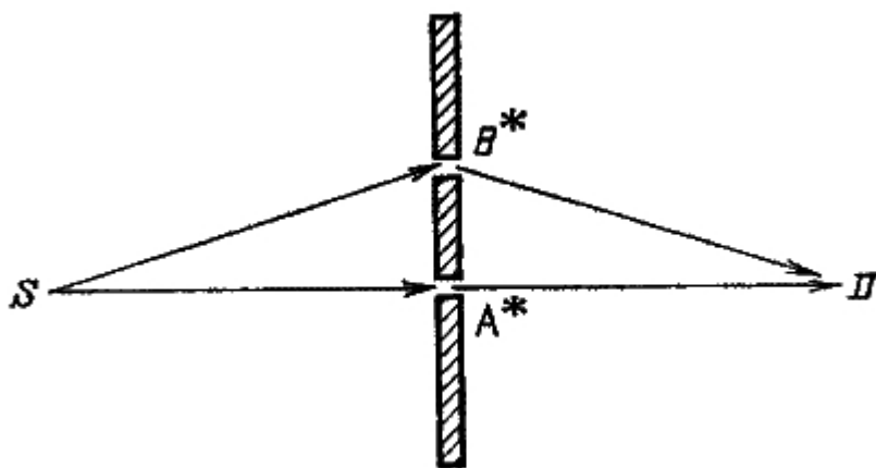
Рис. 50. Если в точках А и В расположены специальные детекторы (*), показывающие, по какому из путей распространяется свет при двух открытых отверстиях, эксперимент меняется. Поскольку фотон всегда проходит или через одно, или через другое отверстие (в случае, если вы за ними следите), имеются два конечных состояния; 1) сработали детекторы в А и D а 2) сработали детекторы в В и D. Вероятность того, что случится каждое из этих событий, равна примерно 1 %. Вероятности двух событий складываются обычным способом, и вероятность срабатывания детектора в D оказывается равной 2 % (см. рис. 51, б)
