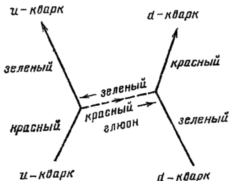
Рис. 83. Глюонная теория отличается от электродинамики тем, что глюоны взаимодействуют с «цветными» частицами (которые могут находиться в одном из трех возможных состояний — «красном», «зеленом» и «синем»). Здесь красный «кварк превращается в зеленый, испуская красно-антизеленый глюон, поглощаемый затем зеленым кварком, который превращается в красный. (Если «цвет» переносится вспять во времени, к его названию добавляется приставка «анти»)
