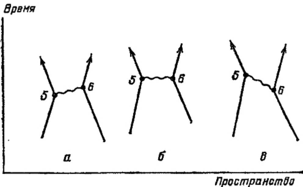
Рис. 61. Поскольку у света имеется амплитуда лететь быстрее или медленнее обычной скорости света, можно считать, что во всех трех примерах фотоны излучались в точке 5 и поглощались в точке 6. И это несмотря на то, что в примере б фотон был излучен и поглощен в одно и то же время, а в примере в был излучен позже, чем поглощен. В последней ситуации вы, может быть, предпочли бы сказать, что фотон был излучен в 6 и поглощен в 5, ведь иначе фотон должен был бы лететь вспять во времени! Поскольку поскольку это касается вычислений (и Природы), это все равно (и все возможно). Поэтому мы говорим просто, что произошел «обмен» фотоном и подставляем пространственно-временные положения в формулу для P(A - B)
