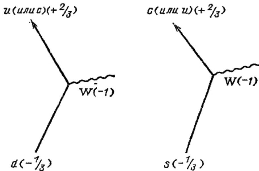
Рис 93. У d -кварка имеется небольшая амплитуда превращения вместо u -кварка в c -кварк, и у s -кварка имеется небольшая амплитуда превращения вместо c -кварка в u -кварк, причем в обоих случаях будет испускаться W -бозон. Мы видим, что W -бозон способен менять кварковый аромат из одного столбца таблицы в другой (см. рис. 92)
