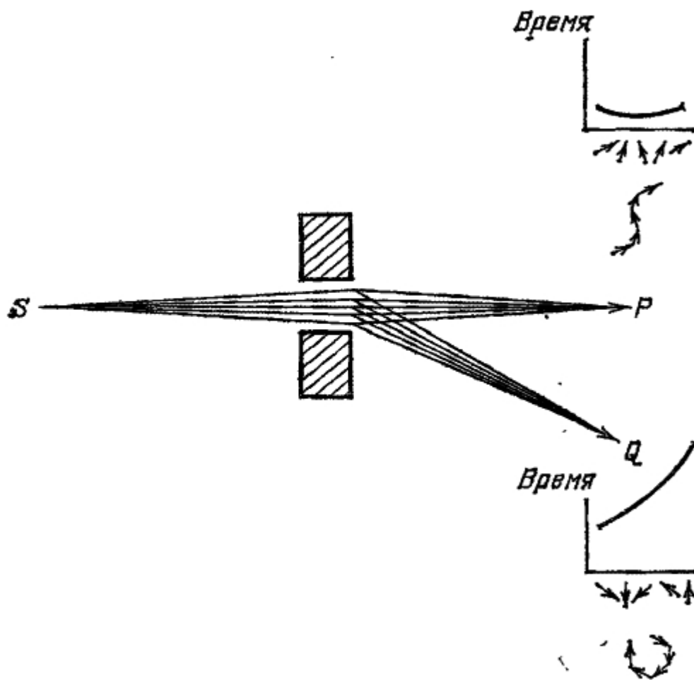
Рис. 33. Свет распространяется не только по прямой, но и по близлежащим траекториям. Когда
