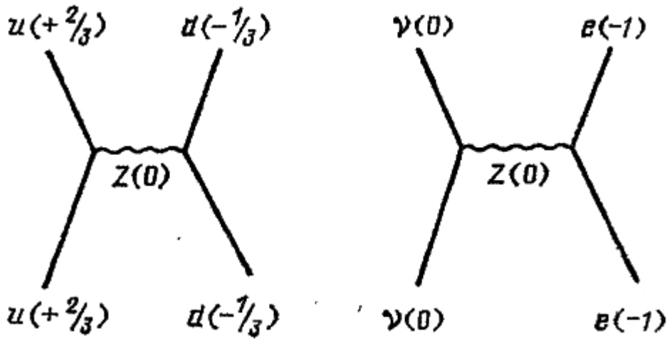
Рис. 87. Когда ни у одной из частиц заряд не меняется, W -бозон тоже не заряжен (он в этом случае называется Z^0 -бозоном). Такие взаимодействия называются «нейтральными токами». Здесь показаны две возможности
