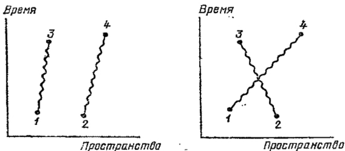
Рис. 70. Амплитуда попадания фотонов из точек 1 и 2 пространства-времени в точки 3 и 4 может быть приближенно найдена, если рассмотреть два изображенных на рисунке основных способа осуществления этого события: P(1-3)P(2-4) и P(1-4) \cdot P(2-3) . При изменении относительного положения точек 1, 2, 3 и 4 в различной степени проявляется интерференция
