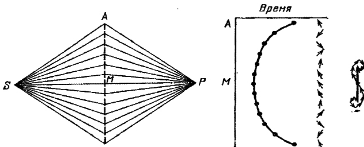
Рис. 35. Анализ всех возможных траекторий из S в P упрощается, если учитывать только ломаные линии с одним изломом (лежащие в одной плоскости). Результат такой же, как и в более сложном, реальном случае: получается кривая времени с минимумом в том месте, где набегаёт наибольший вклад в результирующую стрелку
