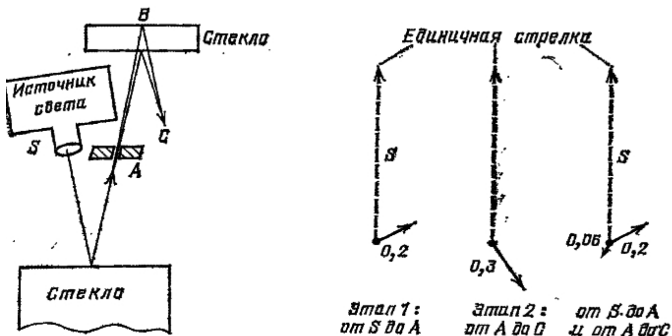
Рис. 37. Анализируя составное событие, можно разделить его на последовательные этапы. В этом примере траекторию фотона S — C можно разделить на два этапа.: 1) фотон летит из S в A и 2) фотон летит из A в C. Можно анализировать каждый этап по отдельности и каждую стрелку рассматривать по-новому; как единичную стрелку (стрелку длиной 1, указывающую на 12 часов), подвергнутую сжатию и повороту. В этом примере сжатие и поворот для 1-го этапа составляют 0,2 и 2 часа; сжатие и поворот для 2-го этапа составляют 0,3 и 5 часов- Чтобы получить амплитуду двух последовательных этапов, мы последовательно сжимаем и поворачиваем. Сначала сжимаем единичную стрелку до 0,2 и поворачиваем на 2 часа затем сжимаем полученную стрелку до 0,3 и поворачиваем на 5
