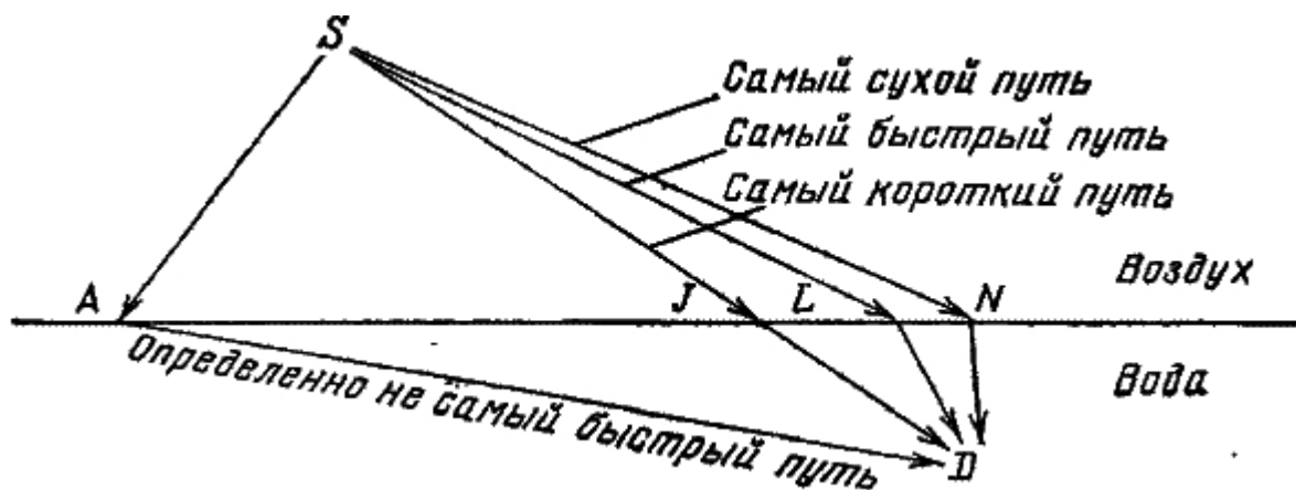
Рис. 30. Выбрать самый быстрый путь для света — все равно, что выбрать самый быстрый путь для спасателя, который сначала бежит, а затем плывет, чтобы спасти утопающего. На самом коротком пути надо слишком долго плыть; на пути, где меньше всего плыть, надо слишком долго бежать; самый быстрый путь компромиссный между ними
