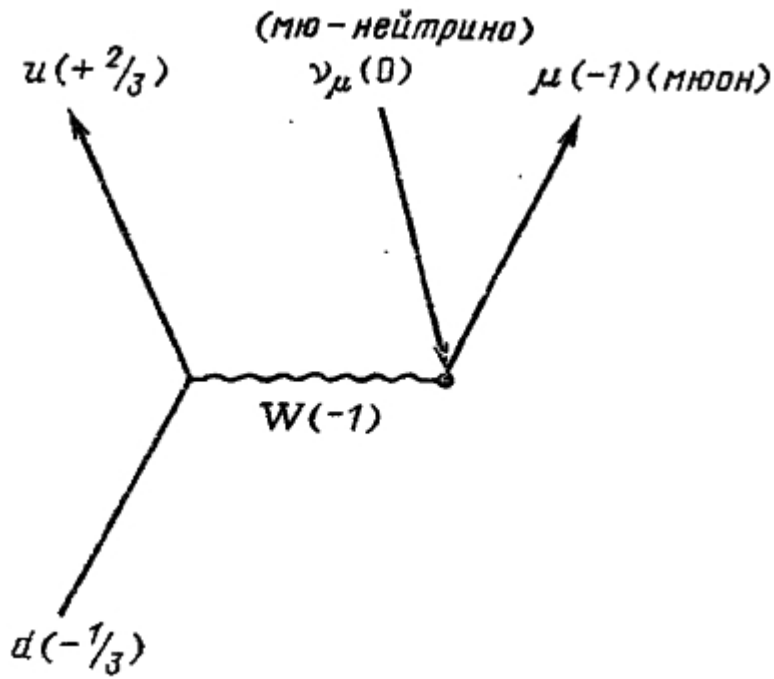
Рис. 90. W — бозона имеется амплитуда излучения мюона вместо электрона. В этом случае место электронного нейтрино занимает мюонное нейтрино
