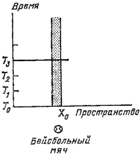
Рис. 52. Сцена, на которой разыгрываются все действия во Вселенной — это пространство-время. Обычно имеющее четыре измерения (три пространственных и одно временное), пространство-время здесь будет представляться двумерным — с одним пространственным (горизонтальная ось) и одним временным (вертикальная ось) измерениями. Когда бы мы ни посмотрели на бейсбольный мяч (например в момент T_3 ), он занимает одно и то же место. Так образуется «полоса бейсбольного мяча», растущая со временем вверх
