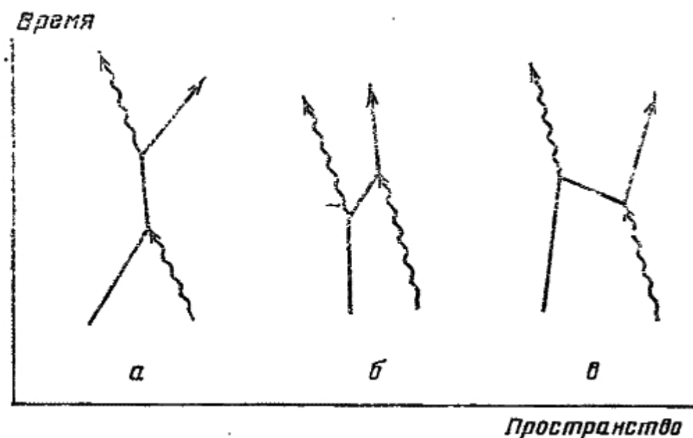
Рис. 63. При рассеянии света фотон может сначала поглощаться электроном, а потом излучаться (а). Такая последовательность событий необязательна, как видно из примера б. Пример — иллюстрирует странную, но реальную возможность: электрон излучает фотон, мчится вспять во времени, чтобы поглотить фотон, а затем снова летит вперед во времени
