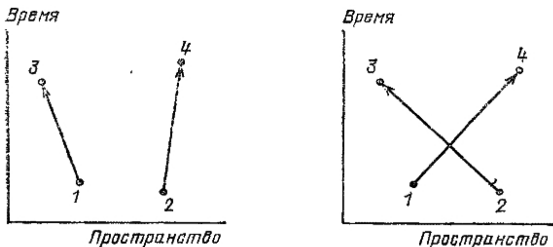
Рис. 59. Чтобы вычислить вероятность того, что электроны попадут из точек 1 и 2 пространства-времени в точки 3 и 4, вычисляем стрелку «первого пути» (из точки 1 в 3 и из 2 в 4), используя формулу для E(A - B) . Затем вычисляем стрелку «второго пути» — «перекрестного» (из точки 1 в 4 и из 2 в 3). Складываем стрелки «первого пути» и «второго пути» и получаем хорошее приближение для результирующей стрелки. (Это справедливо для фальшивого, упрощенного электрона «со спином нуль». Если учитывать поляризацию электрона, то надо не складывать, а вычитать стрелки друг из друга)
