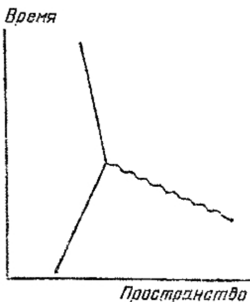
Рис. 58. У электрона, изображаемого прямой линией, есть некоторая амплитуда излучить или поглотить фотон, изображаемый волнистой линией. Поскольку амплитуды поглощения или излучения одинаковы, я буду называть и то и другое «взаимодействием» или «связью». Амплитуда взаимодействия есть число, которое я назову j , оно примерно равно -0,1 (это число иногда называют «зарядом»)
