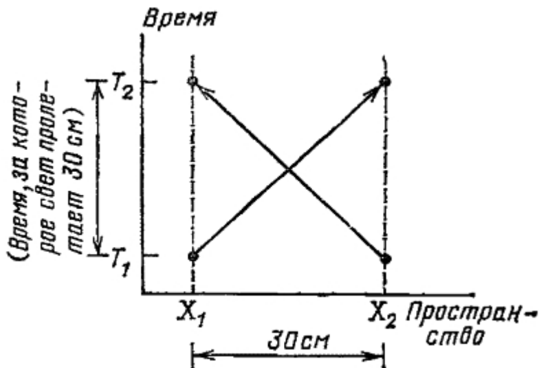
Рис. 54. В этих графиках я буду использовать такую шкалу времени, что частицы, летящие со скоростью света, будут распространяться под углом в 45^\circ в пространстве-времени. Время, которое нужно свету, чтобы пролететь 30 см — из X_1 в X_2 или из X_2 в X_1 — порядка одной миллиардной доли секунды
