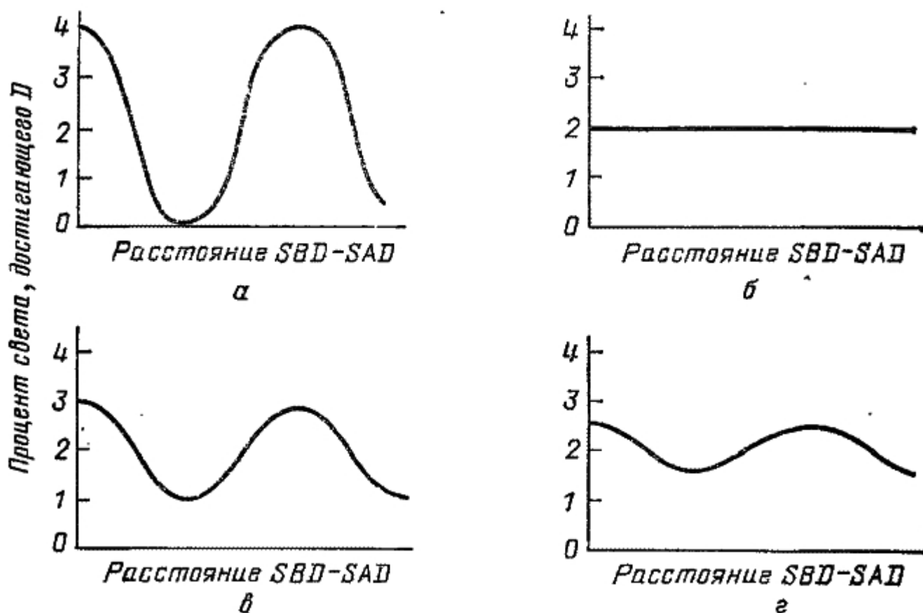
Рис. 51. Если в A и B нет детекторов, возникает интерференция: доля прошедшего света колеблется от 0 до 4 % (а). Если в A и B имеются детекторы, надежные на 100 %, интерференция не возникает — доля попавшего в D света постоянна, 2 % (б). Если детекторы в A и B не надежны на все 100 % (т. е. если иногда в A и B не остается ничего, что можно было бы зарегистрировать), имеются три возможных конечных условия: A и D сработала, B и D сработала, только D сработал. Окончательная кривая на рисунках обусловлена, следовательно, смесью вкладов всех возможных конечных условий. При уменьшении надежности детекторов в A и B интерференция усиливается. Так в случае (в) детекторы менее надежны, чем в случае (г). Принцип, которым надо руководствоваться, встретившись с интерференцией, таков: необходимо независимо вычислить вероятность каждого из различных конечных условий путем сложения стрелок и возведена я в квадрат длины результирующей стрелки; после этого вероятности складываются обычным образом
