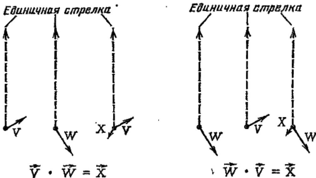
Рис. 39. Математики установили, что умножение стрелок может быть также выражено при помощи последовательных преобразований (в нашем случае — сжатия и поворота) единичной стрелки. Как и при обычном умножении от перемены мест сомножителей произведение не меняется. Чтобы получить ответ — стрелку X, вы можете умножать стрелку V на стрелку W или стрелку W на стрелку V
