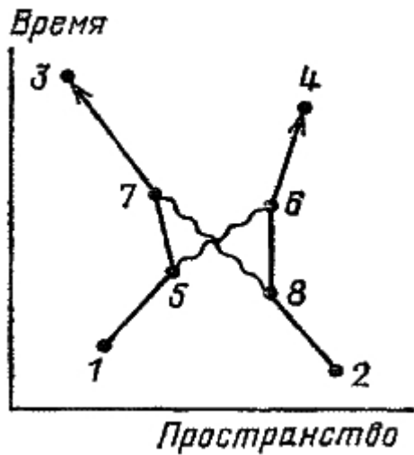
Рис. 62. Событие на рис. 59 может произойти еще одним способом (третьим): путем обмена двумя фотонами. Для этого способа (как мы увидим подробнее ниже) имеется множество диаграмм, одна из которых здесь показана. Стрелка для этого способа учитывает все возможные положения промежуточных точек 5, 6, 7 и 8, и поэтому вычислять ее очень трудно. Поскольку j меньше, чем 0,1, длина этой стрелки, вообще говоря, меньше, чем одна десятитысячная (так как в процессе происходят четыре взаимодействия) — по сравнению с не содержащими j стрелками «первого способа» и «второго способа» на рис. 59
