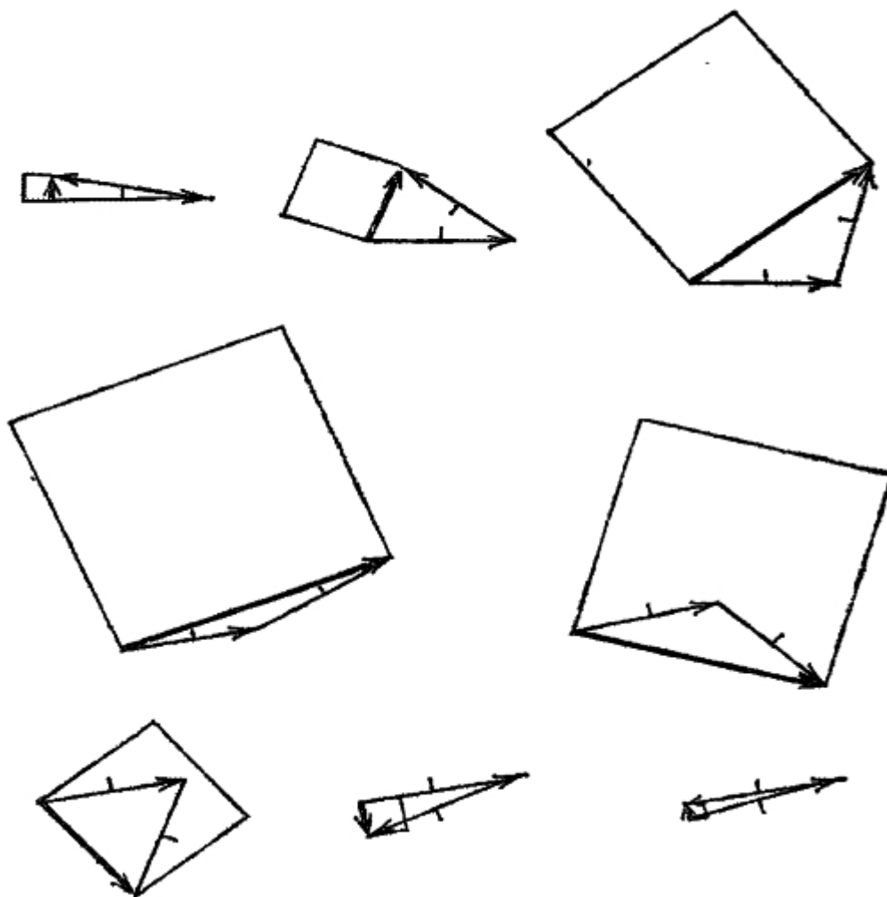
Рис. 17. Когда тонкое стекло заменяют более толстым, стрелка часов, отмеряющая время движения фотона, отраженного от задней поверхности, поворачивается чуть больше, и относительный угол между стрелками переднего и заднего отражения меняется. Это приводит к тому, что результирующая стрелка снова и снова изменяет длину, а ее квадрат колеблется от 0 до 16% и опять до 0
