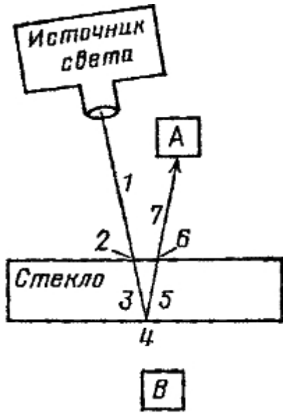
Рис. 42. Отражение от задней поверхности стеклянной пластинки можно разделить на семь этапов. На этапах 1, 3, 5 и 7 происходит только поворот; на этапах 2 и 6 происходит сжатие до 0,98, а на этапе 4 — сжатие до 0,2. В итоге получается стрелка длиной 0,192, которую мы округляем до 0,2 (см. первую лекцию), повернутая на угол, равный полному повороту воображаемой часовой стрелки
