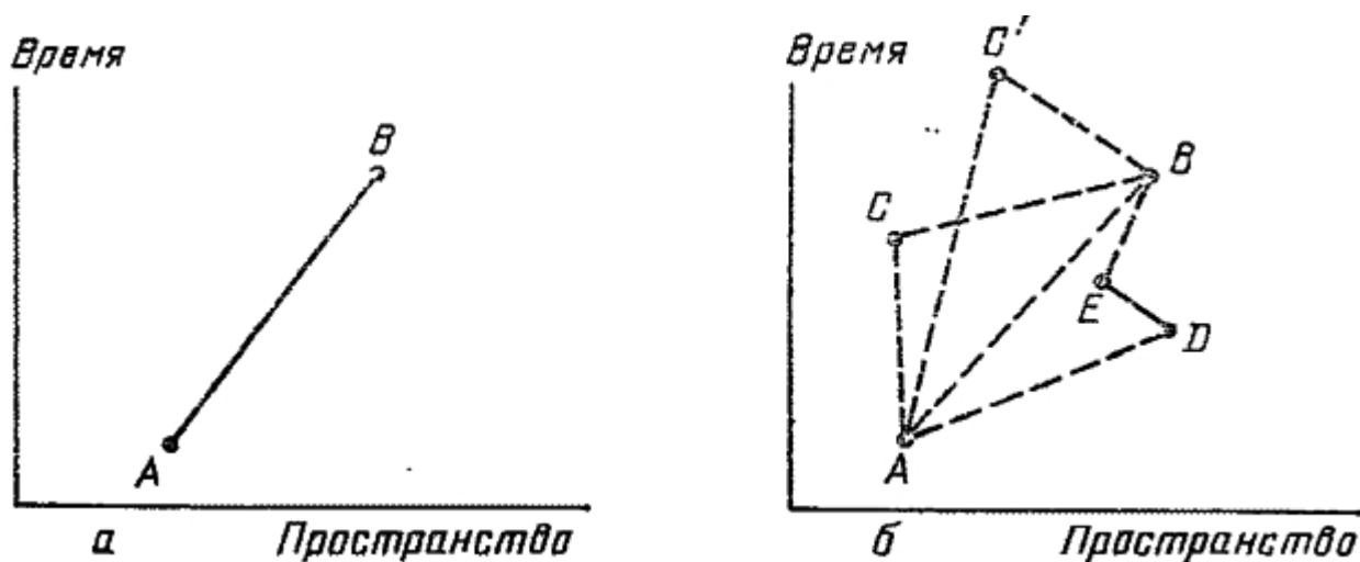
Рис. 57. У электрона имеется амплитуда попасть из одной точки пространства-времени в другую — я буду называть ее E(A - B) . Хотя я и буду изображать E(A - B) прямой линией, соединяющей две точки
