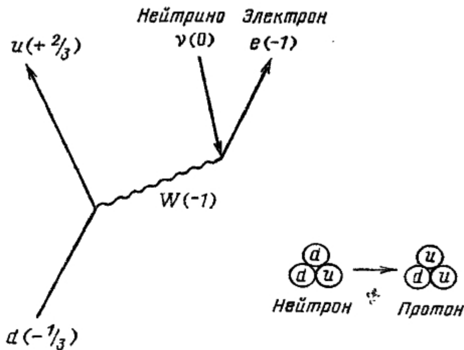
Рис. 85. Когда нейтрон превращается в протон (этот процесс называется бета- распадом), единственное, что изменяется — это «аромат» одного из кварков, d -кварк превращается в u -кварк, что сопровождается вылетом электрона и антинейтрино. Такой процесс происходит довольно медленно, поэтому предположили, что существует промежуточная частица (названная промежуточным W -бозоном) и очень большой массой (порядка 80 000 МэВ) и зарядом -1
