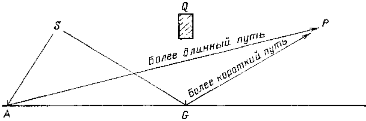
Рис. 23. В то время как длина стрелок существенно не меняется, направление будет различным, потому что фотону требуется разное время для движения по разным траекториям. Ясно, что время прохождения пути S — A—P больше, чем время прохождении пути S — G—P
