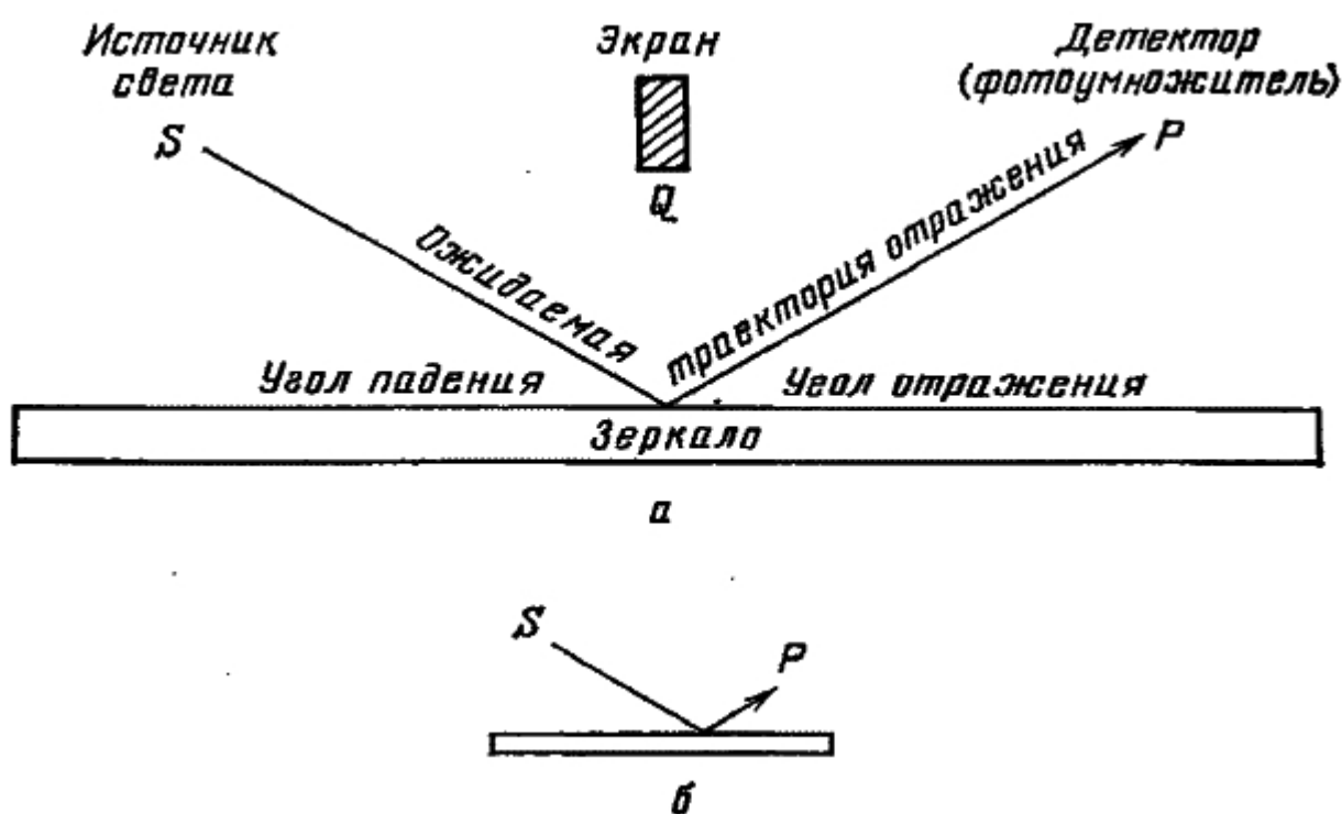
Рис. 19. Согласно классической картине мира зеркало будет отражать свет там, где угол падения равен углу отражения, даже если источник и детектор находятся на разных уровнях, как показано в случае б. [В дальнейшем на рисунках источник изображается буквой S (от source), фотоумножитель — P (от photomultiplier). — Примеч. пер.]
