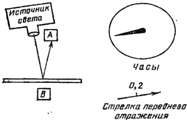
Рис. 10. В эксперименте с отражением от двух поверхностей мы можем сказать, что один фотон может попасть в А двумя способами; отразившись от передней или задней поверхности. Для каждого способа рисуется стрелка длиной 0,2, причем ее направление определяется стрелкой «часов», которая вращается, пока фотон движется. Стрелка «переднего отражения» рисуется в направлении, обратном, остановившейся стрелке часов
