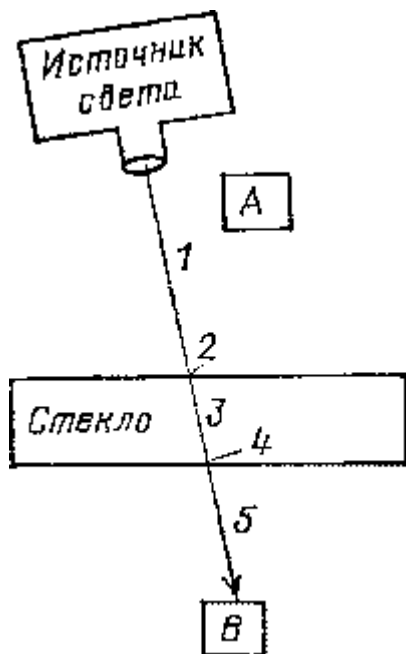
Рис. 43. Прохождение через две поверхности можно разделить на пять этапов. На этапе 2 единичная стрелка сжимается до 0,98, на этапе 4 стрелка длиной 0,98 сжимается еще раз до 0,98 (что дает примерно 0,96). На этапах 1, 3 и 5 происходит только поворот. В итоге квадрат стрелки длиной 0,96 будет равен примерно 0,92, что дает вероятность прохождения через две поверхности, равную 92 %. (Это соответствует 8 %-ному отражению, правильному лишь «дважды в сутки».) Когда толщина пластинки такова, что вероятность отражения равна 16 %, то в сумме с 92 % вероятности прохождения получается 108 %, т. е. мы учли 108 % света. В нашем анализе что-то неправильно!
