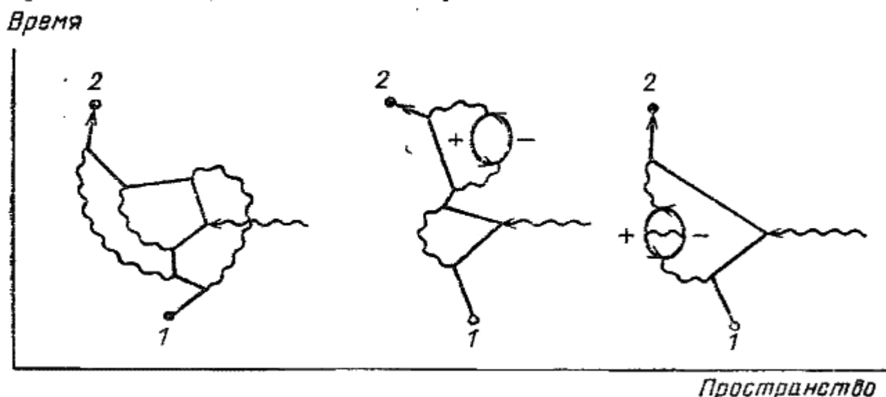
Рис. 76. И сейчас продолжают вычисления, еще более повышающие точность теоретического значения. Следующий вклад в амплитуду, учитывающий все возможности с шестью взаимодействиями, состоит примерно из 70 диаграмм. Три из них показаны на рисунке. В 1983 г. теоретическое значение равнялось 1,00115965246 (с погрешностью около 20 в последних двух цифрах), экспериментальное — 1,00115965221 (с неопределенностью порядка 4 в последней цифре). Такая точность эквивалентна измерению расстояния от Лос-Анджелеса до Нью-Йорка (примерно 3 000 миль) с точностью до толщины человеческого волоса
