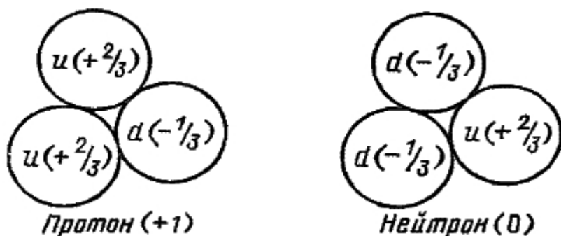
Рис. 80. Все частицы, состоящие из кварков, принадлежат к одному из двух классов. Одни состоят из кварка и антикварка, а другие из трех кварков. Самые известные из этих последних — протон и нейтрон. Заряды u-кварка и d-кварка комбинируются в +1 для протона и в 0 для нейтрона. Тот факт, что протон и нейтрон состоит из движущихся внутри них заряженных частиц, дает ключ к пониманию того, почему у протона магнитный момент превышает 1 , а у, казалось бы, нейтрального нейтрона не равен нулю
