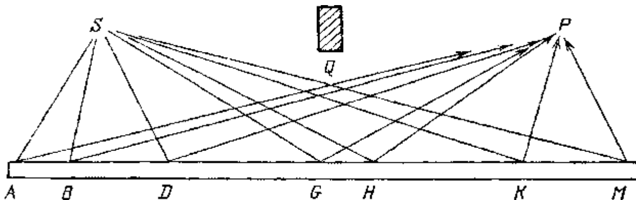
Рис. 20. Согласно квантовой картине мира свет имеет одинаковую амплитуду отразиться от любой части зеркала, от А до М
