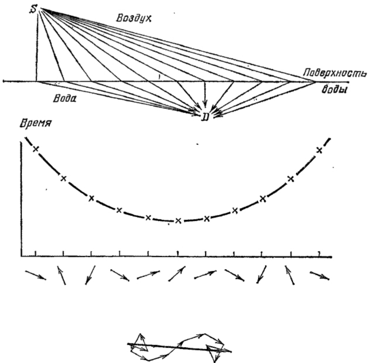
Рис. 29. Согласно квантовой теории свет может попасть из источника, находящегося в воздухе, в детектор, находящийся под водой, разными путями. Если упростить задачу, как в случае с зеркалом, можно нарисовать график, показывающий время каждой траектории, а под ним — направление каждой стрелки. И снова основной вклад в длину результирующей стрелки вносят те траектории, чьи стрелки указывают почти в одном направлении, так как у них почти одинаковое время; и снова для этих траекторий время будет наименьшим
