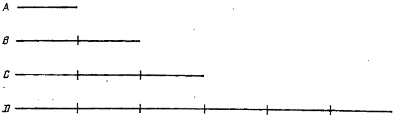
Рис. 38. Любое число может быть выражено в виде преобразования единичного отрезка посредством растяжения или сжатия. Если А — это 1, то В представляет собой 2 (растяжение), а С — 3 (растяжение). Умножение отрезков выполняется путем последовательных преобразований. Например, что значит умножить 3 на 2? Единичный отрезок растягивается в 3 раза, а затем еще в 2 раза, результат — растяжение в 6 раз (отрезок D). Если D — единичный отрезок, то отрезок С представляет собой 1/2 (сжатие), а отрезок В — 1/3 (сжатие), и умножение 1/2 на 1/3 означает, что единичный отрезок D сжат до 1/2, а затем до 1/3 от этого, давая ответ — сжатие до 1/6
