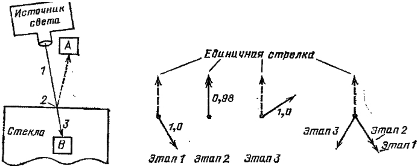
Рис. 41. Прохождение сквозь единственную поверхность также можно разделить на три этапа, со сжатием и/или поворотом на каждом этапе. Квадрат стрелки длиной 0,98 равен примерно 0,96, что дает 96 % вероятности прохождения (в сумме о 4 % вероятности отражения это дает все 100 % света)
