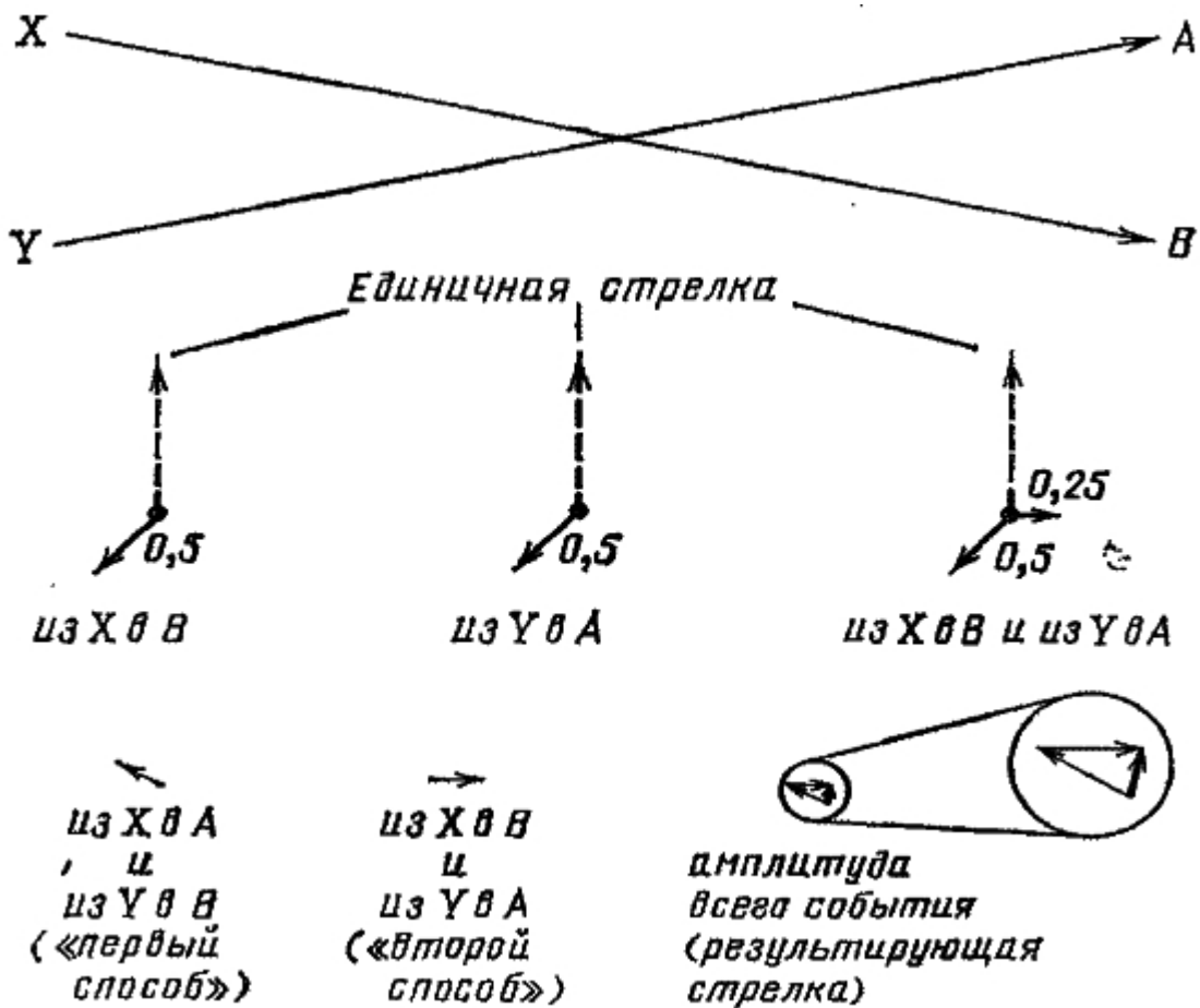
Рис. 48. Событие, обсуждаемое в подписи к рис. 47, могло бы происходить другим способом фотоны летят из X в B и из Y в A. В этом случае все событие (также зависело бы от двух независимых процессов, так что амплитуда этого «второго способа» вычисляется также путем умножения стрелок для независимых событий. Стрелки для «первого» и «второго» способов в конце концов складываются, давая результирующую стрелку всего события. Вероятность события всегда представляется единственной результирующей стрелкой — независимо от того, сколько стрелок было нарисовано, сложено и умножено, чтобы ее получить
