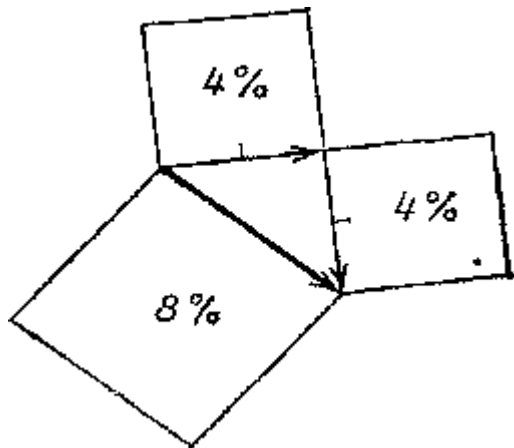
рис. 16. Когда стрелки переднего и заднего отражения составляют прямой угол, результирующая стрелка представляет собой гипотенузу прямоугольного треугольника. Таким образом, ее квадрат равен сумме двух других квадратов 8 %
