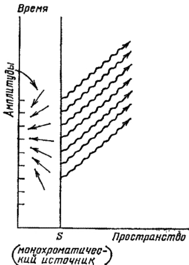
Рис. 67. Монохроматический источник света —
