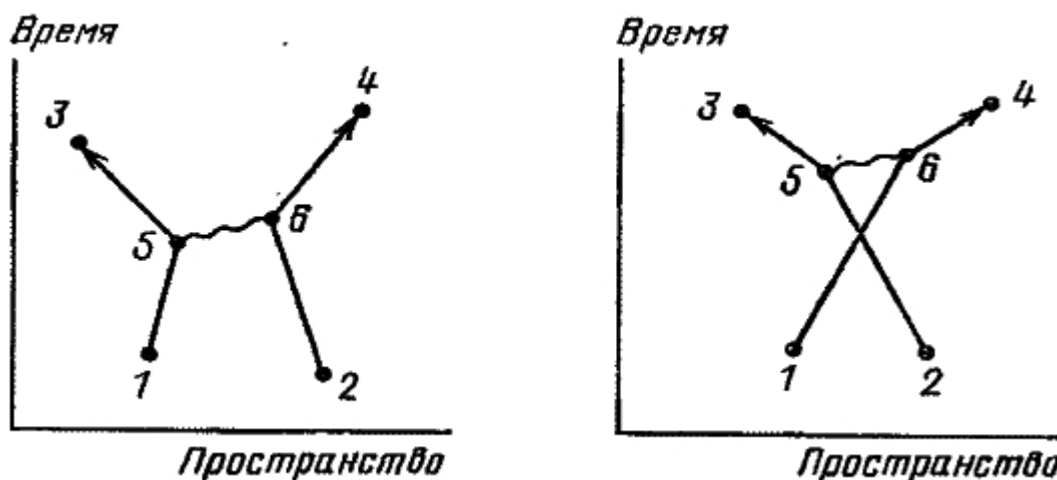
Рис. 60. Вот два других способа, которыми может произойти событие на рис. 59; на каждом
