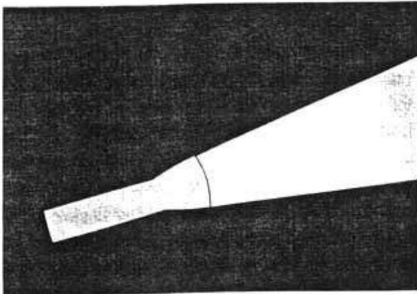
Рис. 2.1. Свет от электрического фонарика
