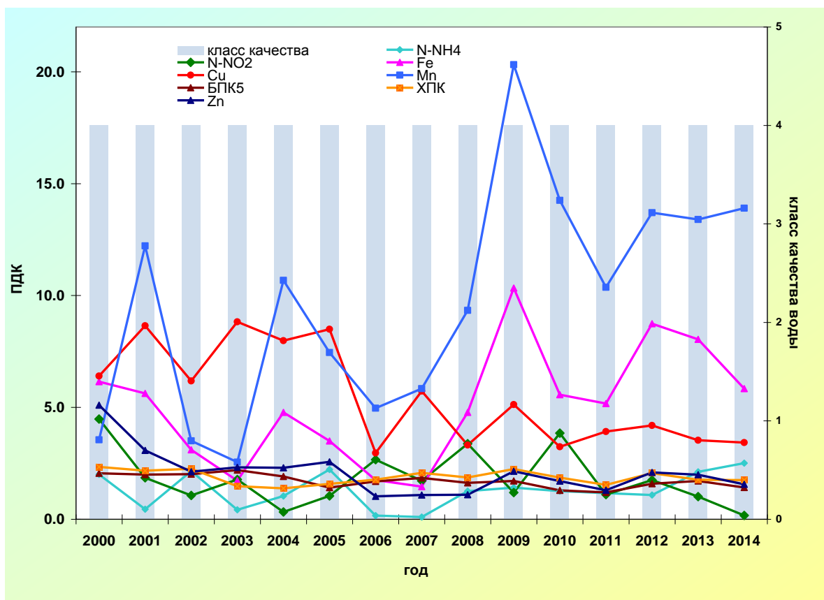
Рис. 3.27. Изменение среднегодовых концентраций отдельных ингредиентов и качества воды р. Охта, в черте г. Санкт-Петербург
