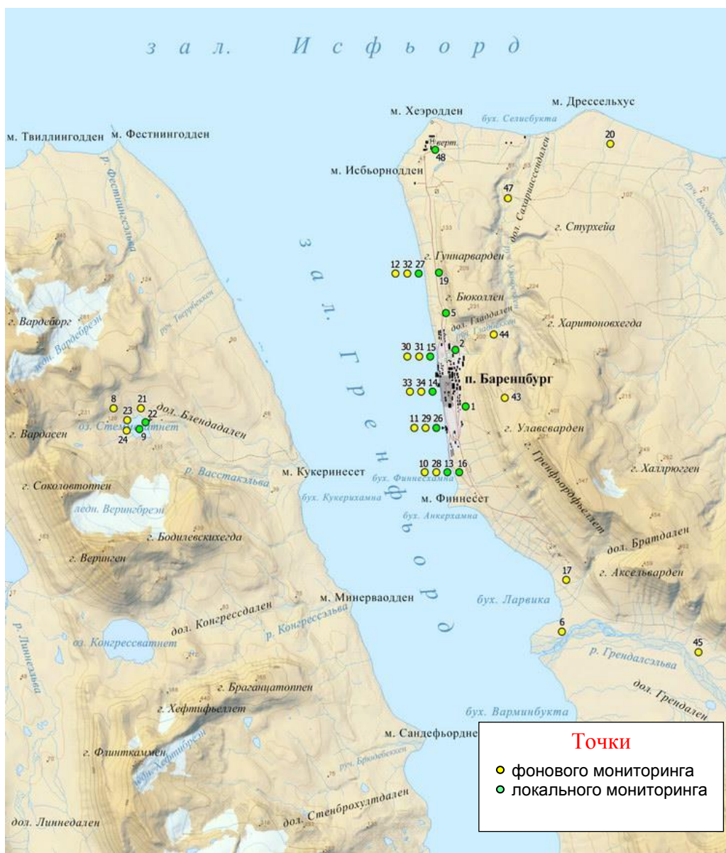
Рис. 4.25. Схема точек выполнения наблюдений и отбора проб при проведении фонового и локального экологического мониторинга в районе пос. Баренцбург
