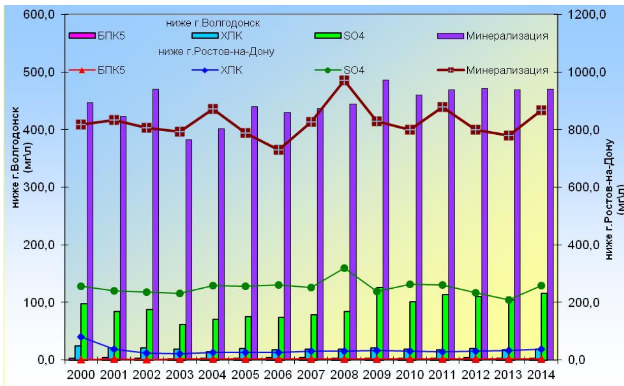
Рис. 3.29. Динамика концентраций отдельных характерных загрязняющих веществ в воде р. Дон ниже г. Волгодонск и ниже г. Ростов-на-Дону
