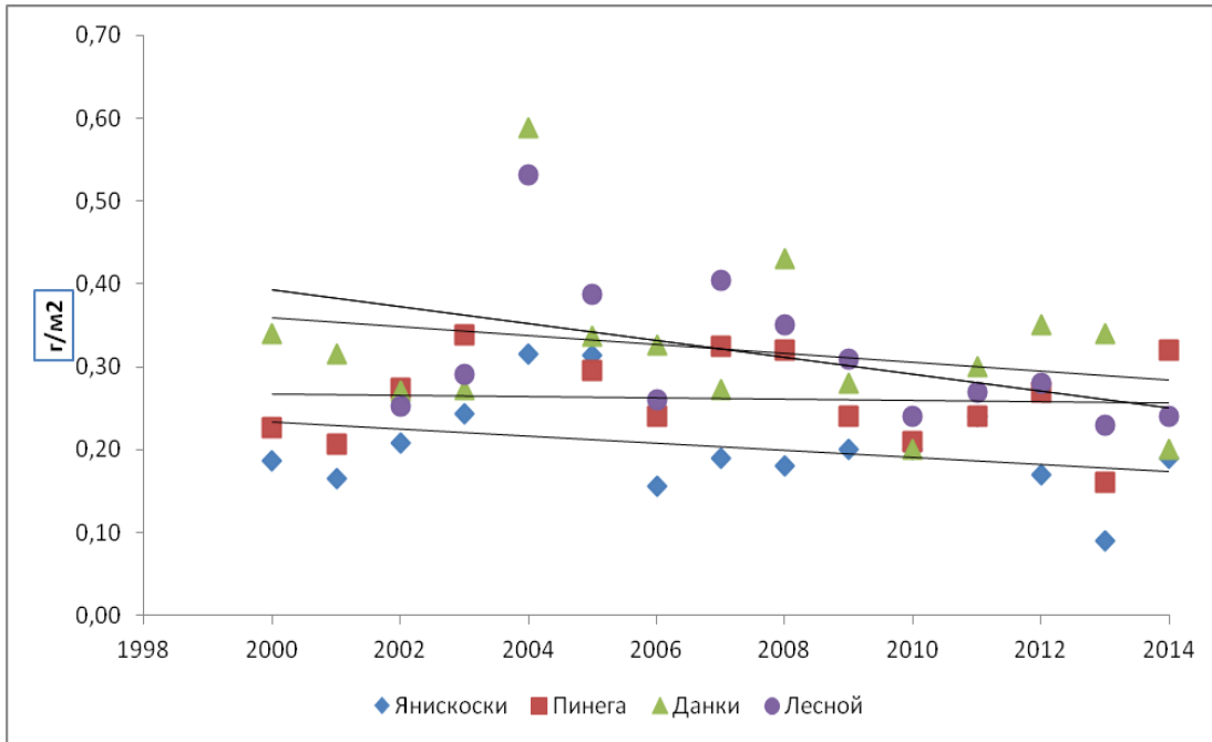
Рис. 2.38. Среднегодовые выпадения сульфатной серы из атмосферы с осадками, г S/м 2 /год
