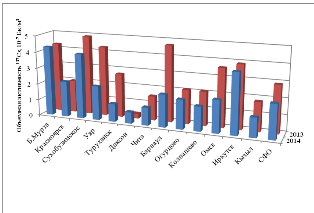
Рис. 2.60. Среднегодовая объемная активность 137 Cs в населенных пунктах СФО, 10 -7 Бк/м 3
