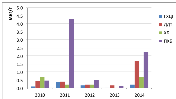
Рис. 4.26. Изменения средних концентраций ХОС в атмосферном воздухе за период 2010-2014 года
