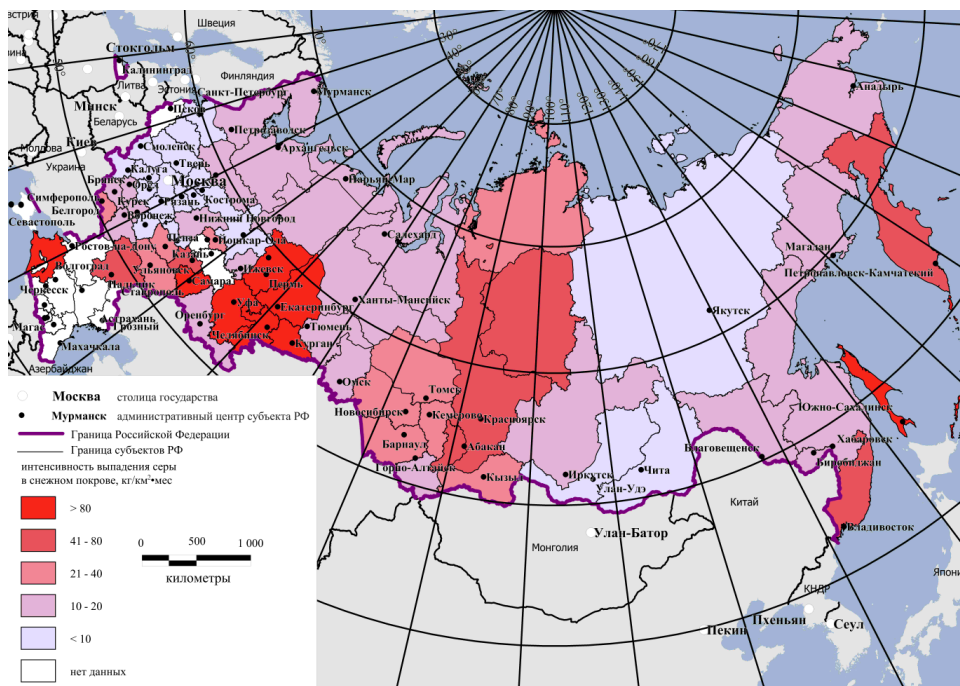
Рис. 2.33. Средняя интенсивность выпадений серы P_s на территории РФ в зимний период 2013-2014 гг., по данным мониторинга содержания сульфатов в снежном покрове
