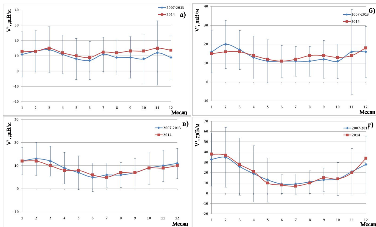
Рис. 2.15. Годовой ход V' по станциям: (а) Воейково, (б) Верхнее Дуброво, (в) Иркутск, (г) Южно-Сахалинск в 2014 г. на фоне осредненного годового хода V' за предшествующий период измерений. Вертикальными отрезками показаны стандартные отклонения для средних месячных значений V' за период с 2007 по 2013 гг.
