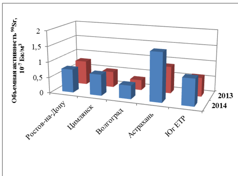
Рис. 2.61. Среднегодовая объемная активность ^{90}\text{Sr} в населенных пунктах ЮФО в 2013-2014 годах, 10^{-7} Бк/м 3
