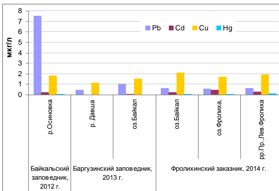
Рис. 4.23. Средние значения концентраций тяжелых металлов в водах рек заповедников: Байкальский, Баргузинский, Фролихинский заказник и оз. Байкал
