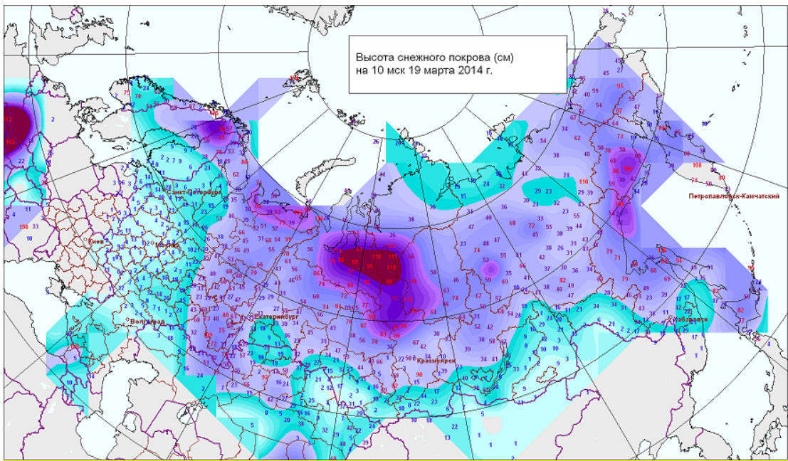
Рис. 1.14. Высота снежного покрова (см) по данным на 19.03.2014 г.
