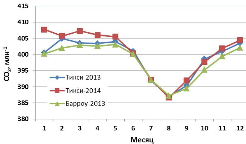
Рис. 2.7. Сезонный ход концентрации CO 2 для станции Тикси и Барроу
