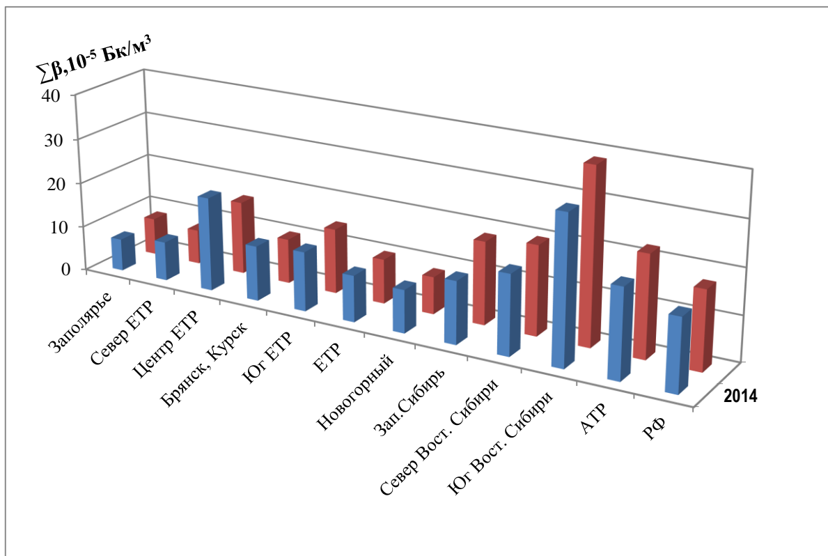
Рис. 2.58. Средние значения объемной \Sigma В в приземном слое атмосферы на территории РФ в 2013-2014 годах, 10^{-5} Бк/м 3
