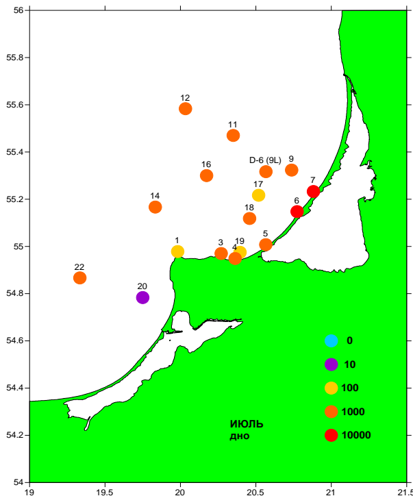
Рис. 3.65. Средние значения НВЧ НМ, кл/мл, на придонных горизонтах в юго-восточной части Балтийского моря в июле 2003-2014 гг.
