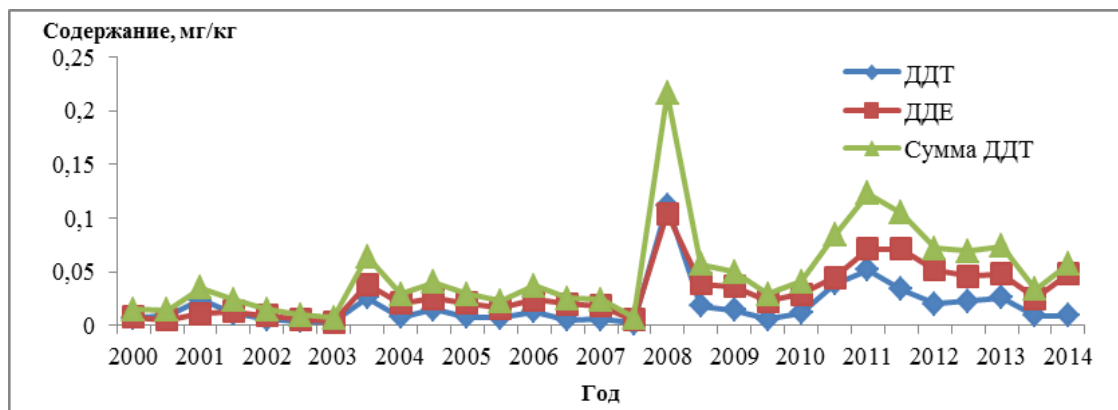
Рис. 3.26. Среднее содержание ДДТ и ДДЭ в почве хозяйств «Путиенко» с. Халкидон Черниговского района Приморского края
