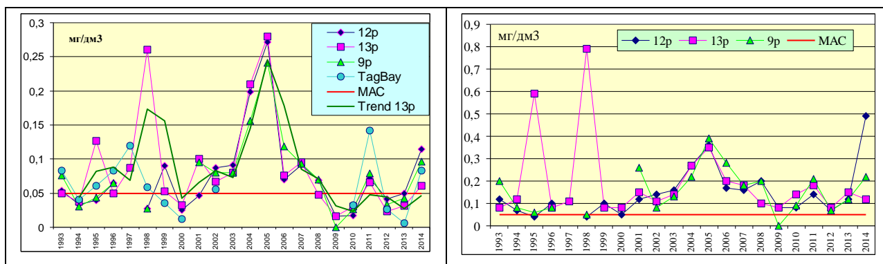
Рис. 3.56. Динамика средней и максимальной концентрации нефтяных углеводородов в водах устьевых протоков реки Дон и в восточной части Таганрогского залива в 1993-2014 гг.
