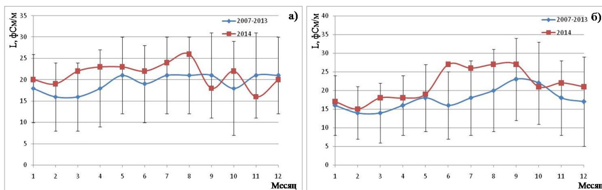
Рис. 2.16 Годовой ход L_5 по станциям (а) Воейково, (б) Иркутск в 2014 г. на фоне осредненного годового хода годового L_5 за предшествующий период измерений. Вертикальными отрезками обозначены стандартные отклонения для средних месячных значений L_5 за 2007 - 2013 гг.
