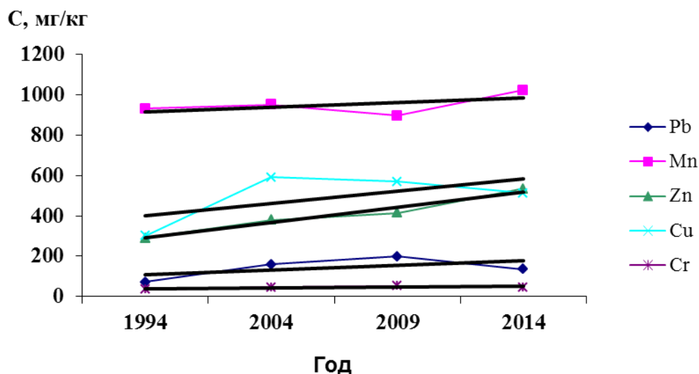
Рис. 3.22. Динамика средних значений (С) массовых долей кислоторастворимых форм свинца, марганца, цинка, меди и хрома в почвах пятикилометровой зоны вокруг ОАО «Среднеуральский медеплавильный завод» в г. Ревда
