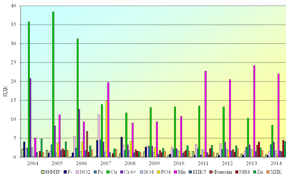
Рис. 3.45. Динамика среднегодового содержания основных загрязняющих веществ в воде р. Чусовая в створе 1,7 км ниже г. Первоуральск
