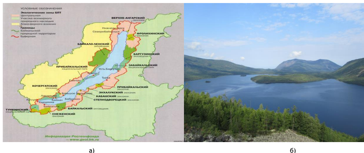
Рис 4.16. а) - Заповедники Прибайкалья; б) Фролихинский заказник Баргузинского заповедника, оз. Фролиха
