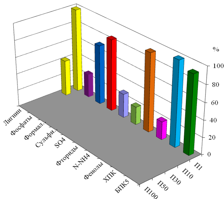
Рис. 3.36. Повторяемость числа случаев превышения ПДК загрязняющими веществами в воде р. Вихорева, 7 км ниже с. Кобляково в 2014 г.
