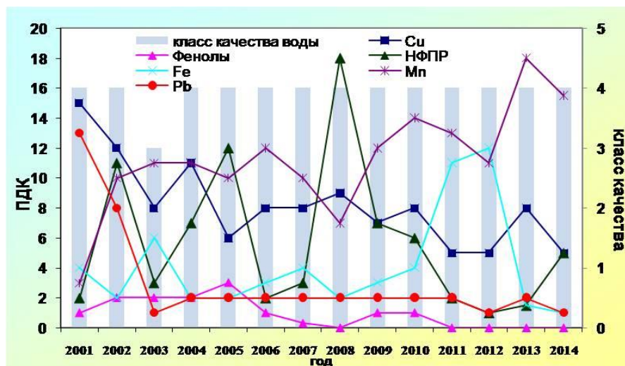
Рис. 3.38. Изменение среднегодовых концентраций отдельных ингредиентов и качества воды р. Колыма, п. Усть-Среднекан
