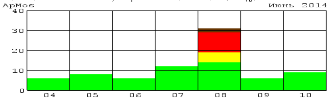
Рис. 1.4. Суточные значения ApMos
