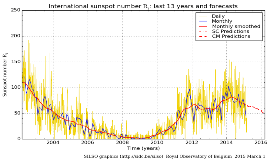
Рис. 1.2. График изменения среднемесячных значений чисел Вольфа
