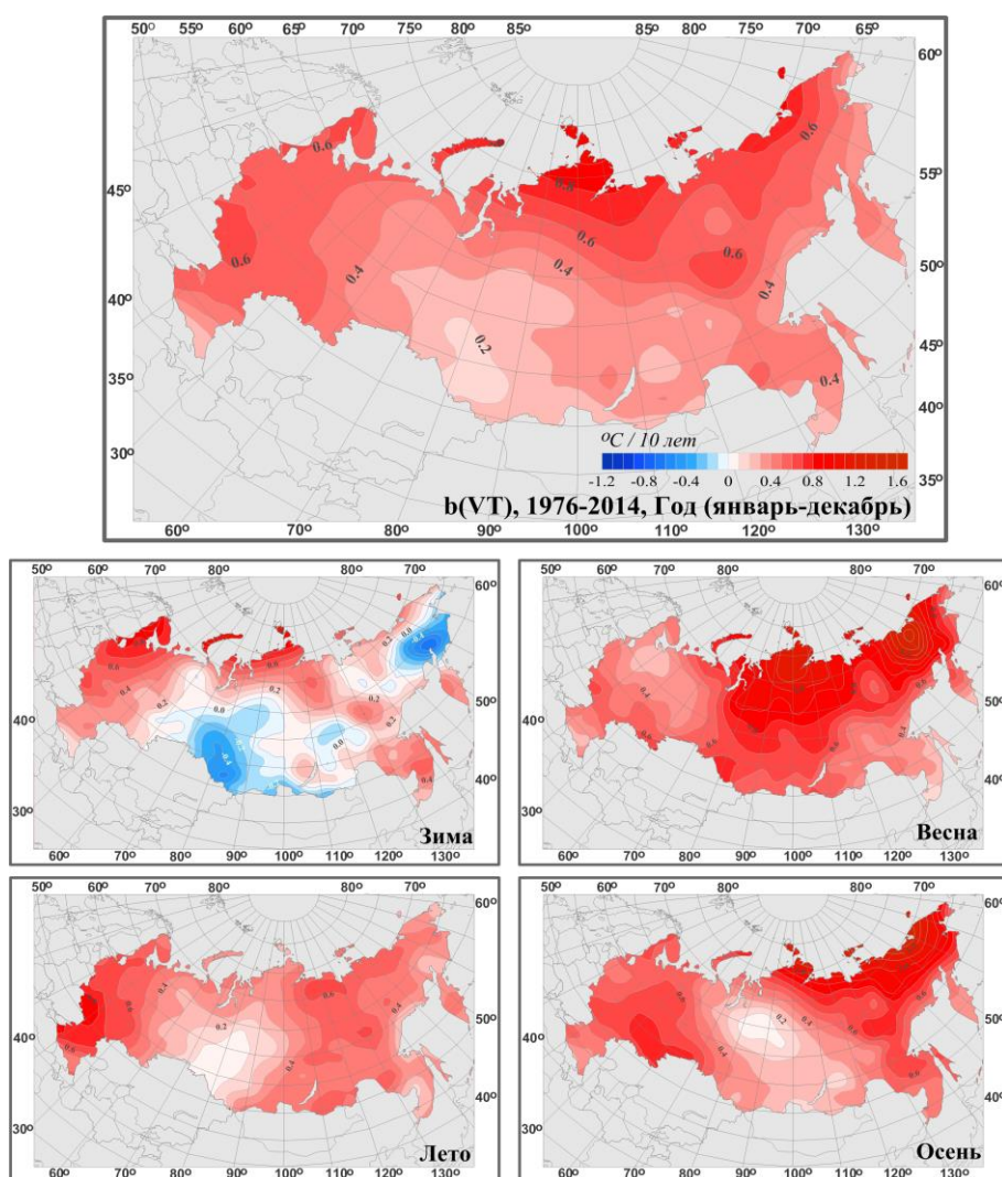
Рис. 1.10. Распределение коэффициентов линейного тренда среднегодовой и средних сезонных значений температуры приземного воздуха на территории РФ за период 1976-2014 гг. (в °С/10 лет)
