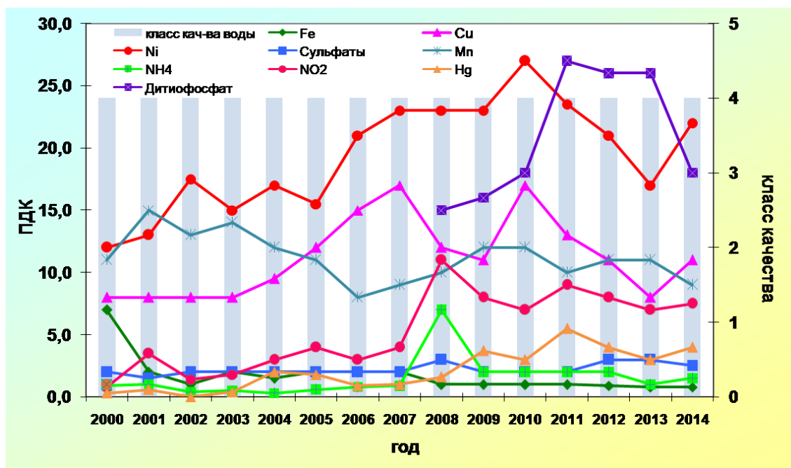
Рис. 3.28. Изменение среднегодовых концентраций отдельных ингредиентов и показателей качества воды р. Хауки-лампи-йоки, г. Заполярный
