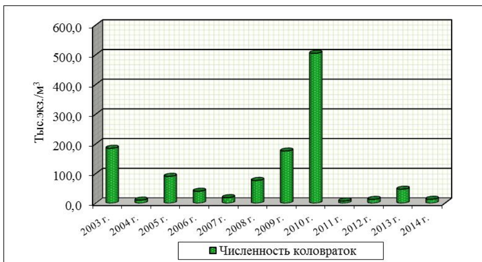
Рис. 3.68. Средняя численность коловраток в юго-восточной части Балтийского моря в июле 2003-2014 гг.
