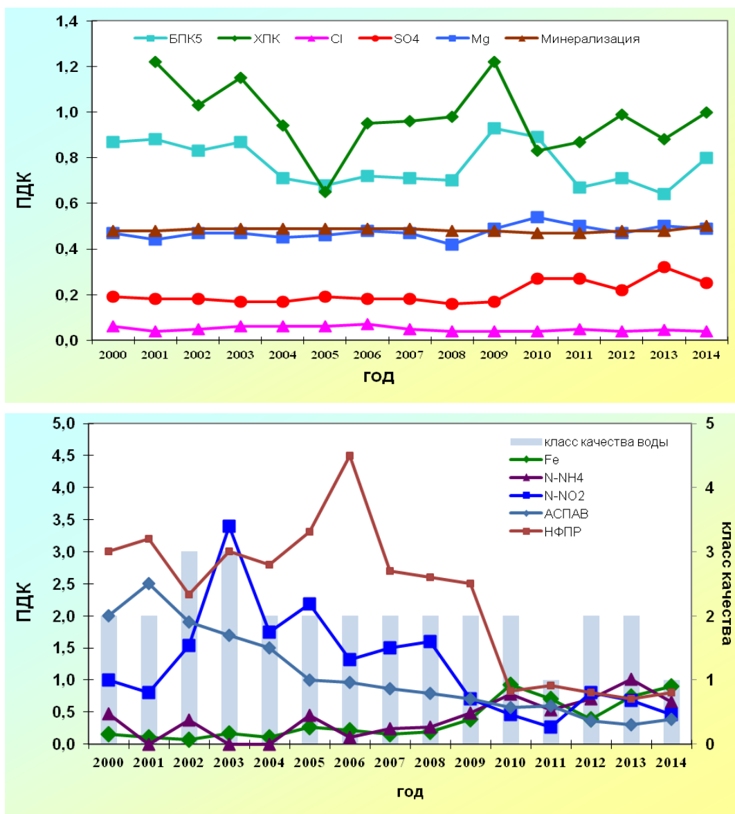
Рис. 2.50. Изменение среднегодовых концентраций основных ингредиентов и качества воды р. Ворона в черте г. Уварово
