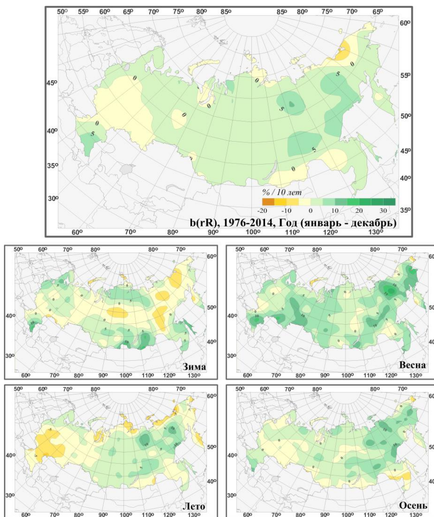
Рис. 1.13. Пространственные распределения локальных коэффициентов линейного тренда годовых и сезонных сумм атмосферных осадков за 1976-2014 гг. на территории РФ (% от нормы за 10 лет)
