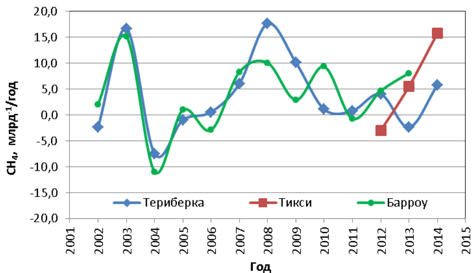
Рис. 2.6. Межгодовые изменения концентрации CH 4
