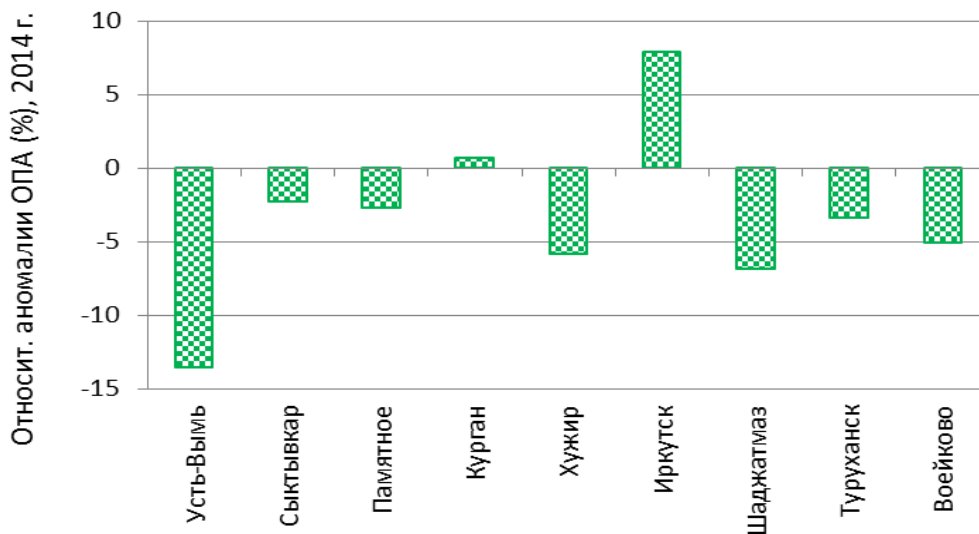
Рис. 2.11. Относительные аномалии ОПА (%) на станциях фоновое мониторинга в 2014 г.
