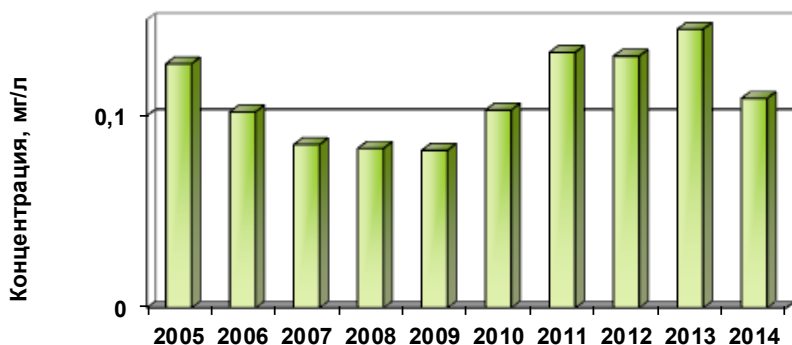
Рис. 4.9. Изменение среднегодовых концентраций нитритного азота в целом по водным объектам Московского региона
