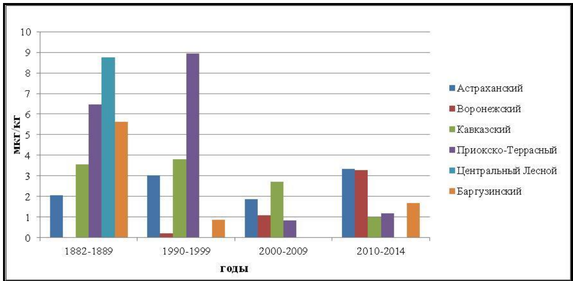
Рис. 2.47. Динамика средних значений \gamma - ГХЦГ в почвах биосферных заповедников по 10-ти летним периодам
