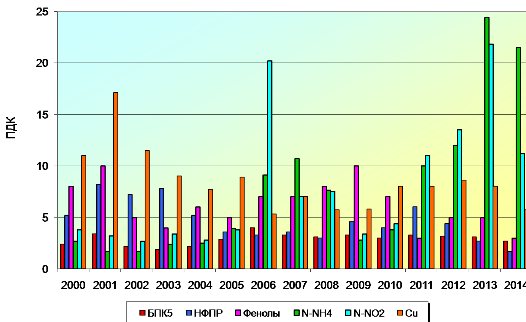
Рис. 3.43. Динамика загрязняющих веществ в воде р. Москва, г. Москва выше Бесединского моста
