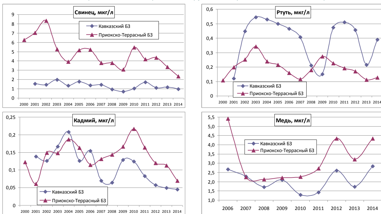
Рис. 2.37. Изменение содержания тяжелых металлов в атмосферных осадках фоновых районов в 2000-2014 гг.
