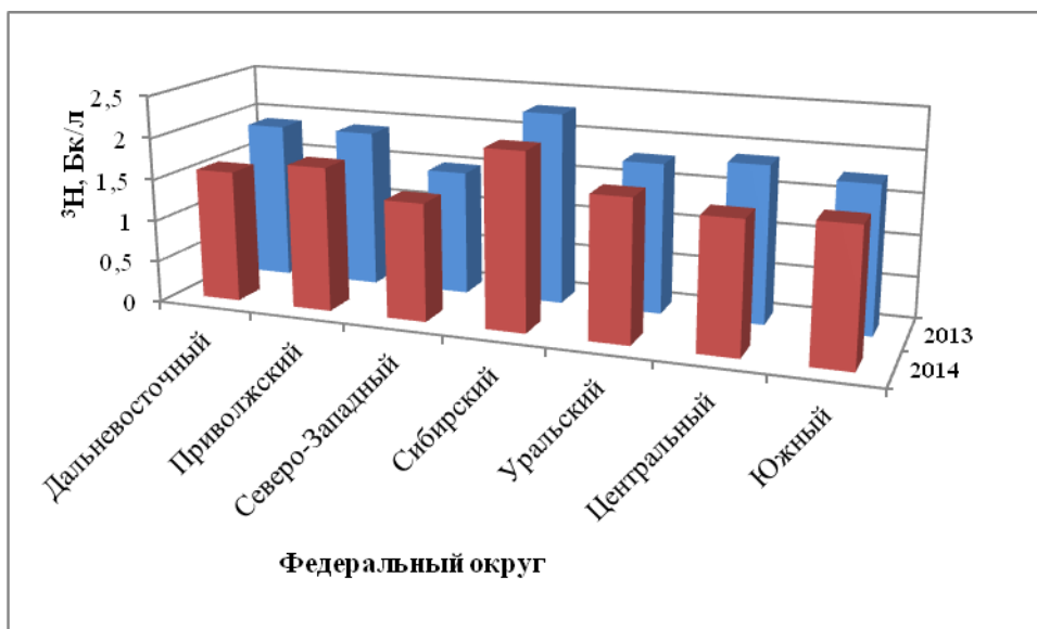
Рис. 2.62. Среднегодовая объемная активность 3 H в атмосферных осадках на территории федеральных округов РФ в 2013-2014 годах, Бк/л
