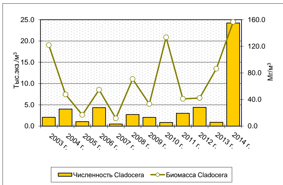
Рис. 3.69. Средние значения численности и биомассы Cladocera в юго-восточной части Балтийского моря в июле 2003-2014 гг.
