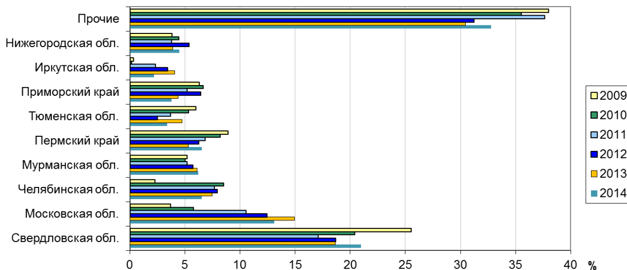
Рис. 3.52. Распределение случаев ВЗ и ЭВЗ по субъектам Российской Федерации
