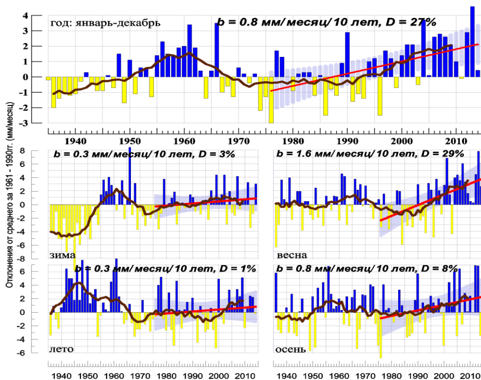
Рис. 1.11. Средние годовые и сезонные аномалии осадков (мм/месяц), осредненные по территории РФ, 1936-2014 гг. Аномалии рассчитаны как отклонения от среднего за 1961-1990 гг. Сглаженная кривая получена 11-летним скользящим осреднением. Линейный тренд проведен по данным за 1976-2013 гг.; b - коэффициент тренда (мм/мес/10 лет), D - вклад в суммарную дисперсию (%)
