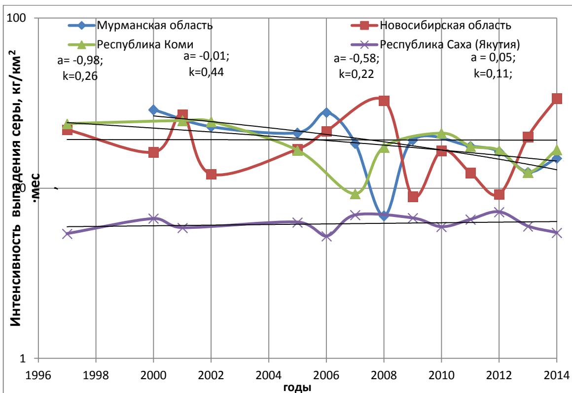
Рис. 2.34. Интенсивность выпадений серы P_s в промышленных и фоновых регионах на ЕТС и АТС по данным мониторинга химического состава снежного покрова в 1997-2014 гг.
