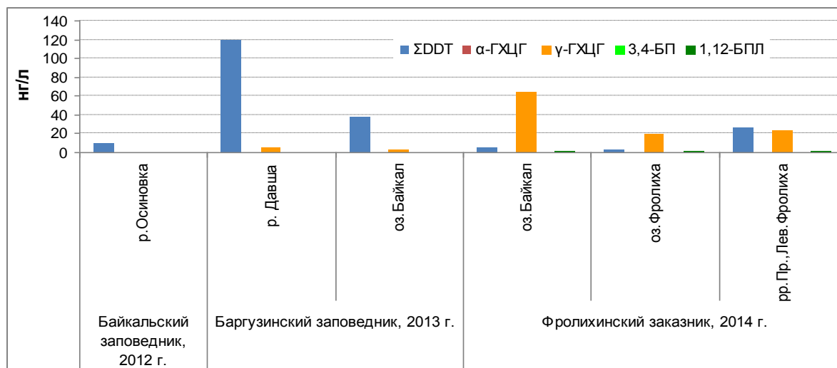
Рис. 4.24. Средние значения концентраций пестицидов и полиароматических углеводов в водах рек заповедников: Байкальский, Баргузинский, Фролихинский заказник и оз. Байкал
