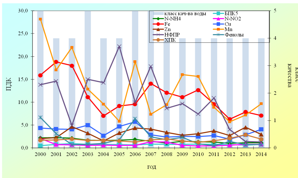
Рис. 3.33. Изменение среднегодовых концентраций отдельных ингредиентов и класса качества воды р. Обь ниже г. Салехард
