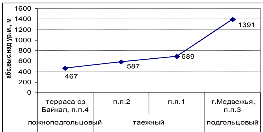
Рис. 4.17. Вертикальный профиль отбора проб растений и почвы на пробных площадках (п.п.) биосферного заказника Фролихинский Баргузинского заповедника
