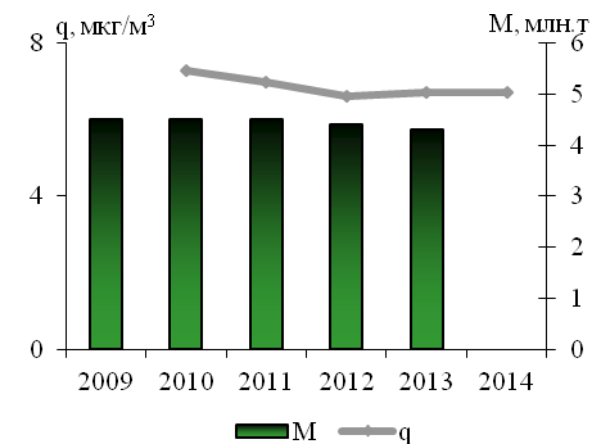
Рис. 3.10. Среднегодовые концентрации (q) и суммарные выбросы (M) диоксида серы
