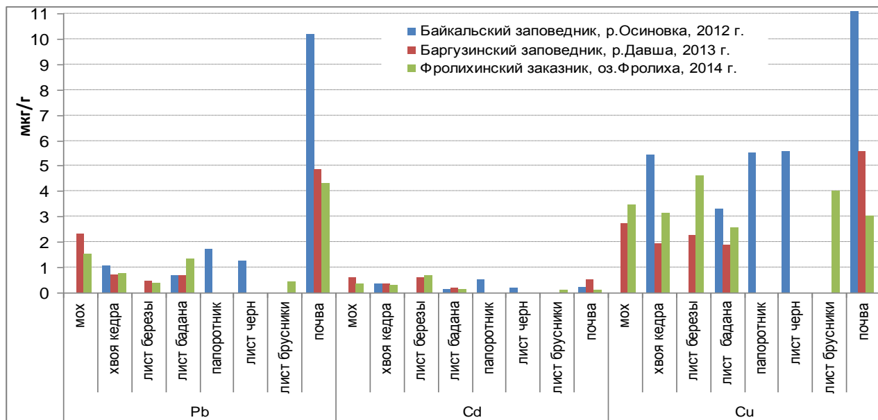
Рис. 4.19. Среднее содержание тяжелых металлов в образцах растений и почвы в заповедниках: Байкальском (р. Осиновка-Танхойская, 2012 г.), Баргузинском (р. Давша, 2013 г.), и Фролихинском заказнике (оз. Фролиха, 2014 г.)
