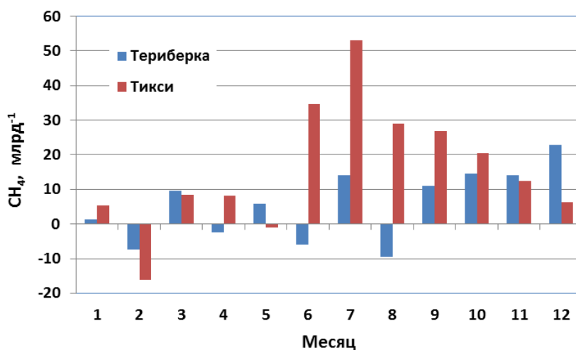
Рис. 2.9. Изменение среднемесячных значений концентрации метана 2013-2014 гг. для станций Тикси и Териберка
