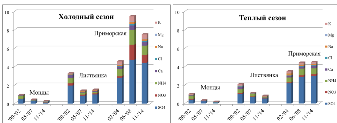
Рис. 2.41. Изменение среднего химического состава аэрозолей (мкг/м³) на станциях ЕАНЕТ в холодный (слева) и теплый (справа) периоды по наблюдениям в 2000-2014 г.
