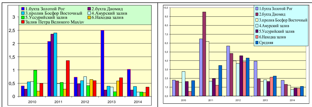
Рис. 3.62. Максимальная концентрация нефтяных углеводородов ( \text{мг}/\text{дм}^3 ) и средняя концентрация (в ПДК) в различных частях акватории залива Петра Великого Японского моря
