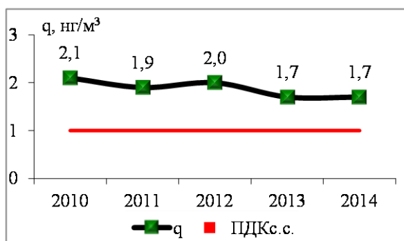
Рис. 3.13. Среднегодовые концентрации бенз(а)пирена
