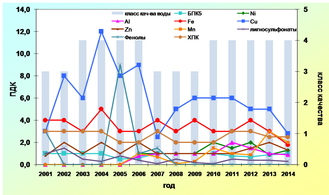
Рис. 3.31. Изменение среднегодовых концентраций отдельных ингредиентов и показателей качества воды р. Северная Двина, г. Красавино, 3,5 км ниже города за многолетний период
