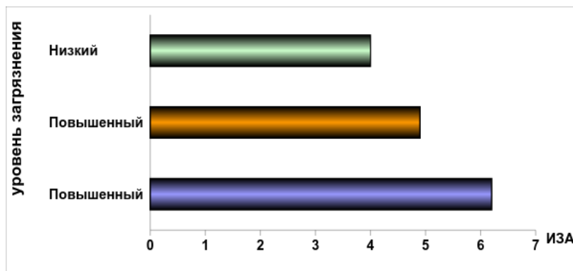
Рис. 4.3. Уровень загрязнения атмосферного воздуха в различных зонах Москвы в 2014 году
