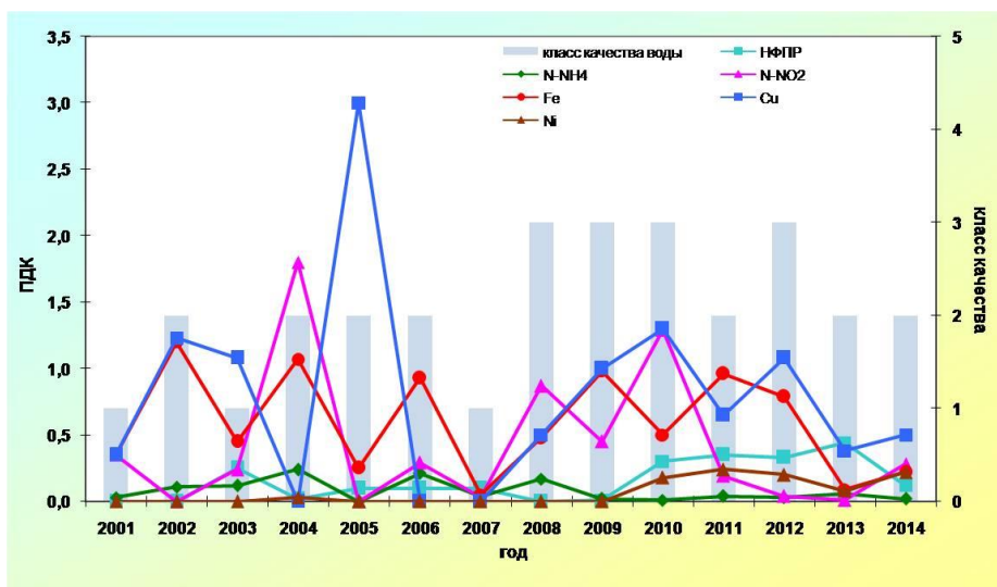
Рис. 2.55. Изменение среднегодовых концентраций отдельных ингредиентов и качества воды р. Лена, г. Усть-Кут
