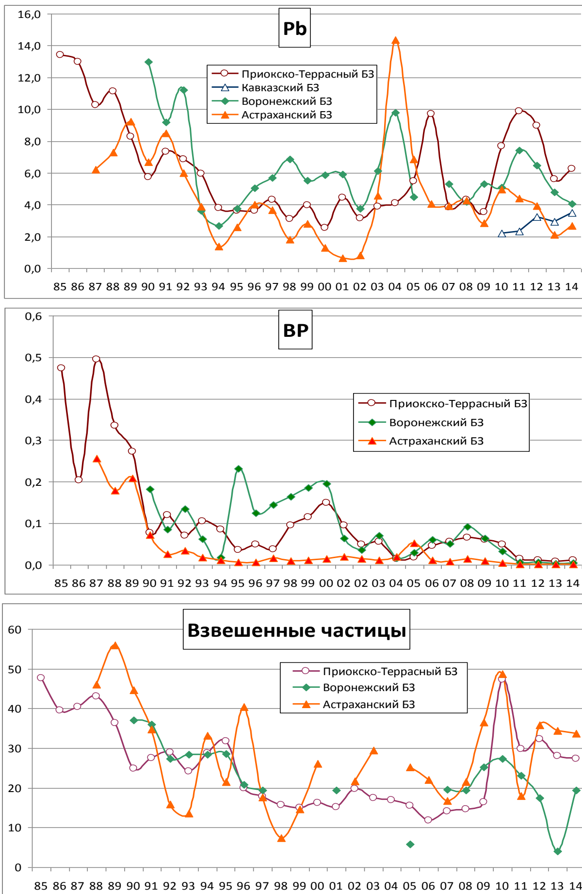
Рис. 2.22. Изменение фонового содержания свинца, 3,4-бензпирена ( \text{нг}/\text{м}^3 ) и взвешенных частиц ( \text{мкг}/\text{м}^3 ) в атмосферном воздухе фоновых районов
