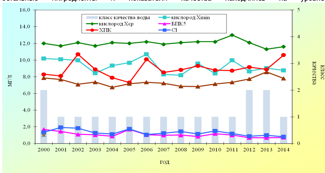
Рис. 2.53. Изменение класса качества и среднегодовых концентраций отдельных ингредиентов и показателей качества воды Иркутского водохранилища, ОПП-1 Исток Ангары за многолетний период
