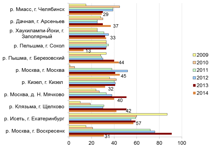
Рис. 3.55. Пункты наблюдения, в которых регистрировалось максимальное число повторений случаев ВЗ и ЭВЗ в течение года
