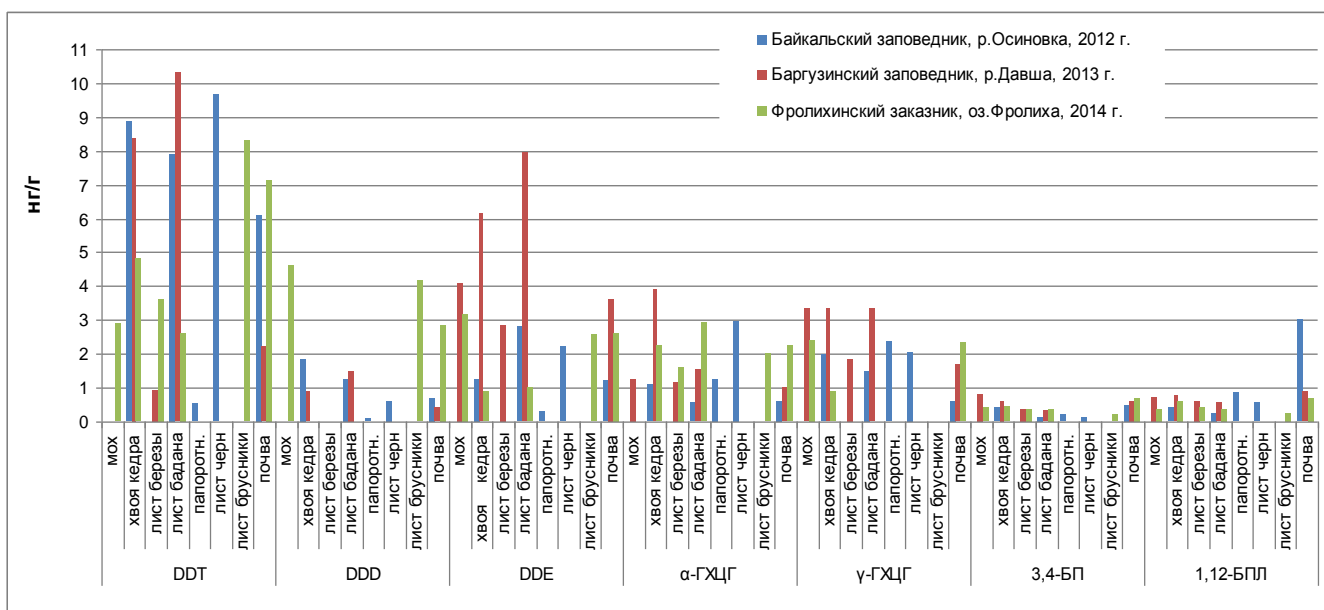
Рис. 4.22. Среднее содержание пестицидов и полиароматических углеводородов в образцах растений и почвы в заповедниках Байкальском (р. Осиновка-Танхойская, 2012 г.), Баргузинском (р. Давша, 2013 г.) и Фролихинском заказнике (оз. Фролиха, 2014 г.)
