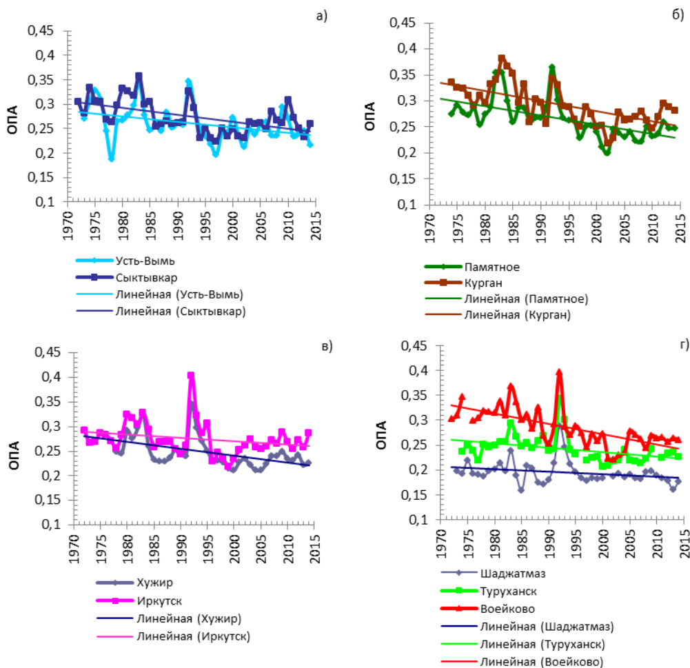
Рис. 2.13. Межгодовая изменчивость ОПА на парных (а, б, в) и непарных (г) станциях фоновый мониторинга атмосферы
