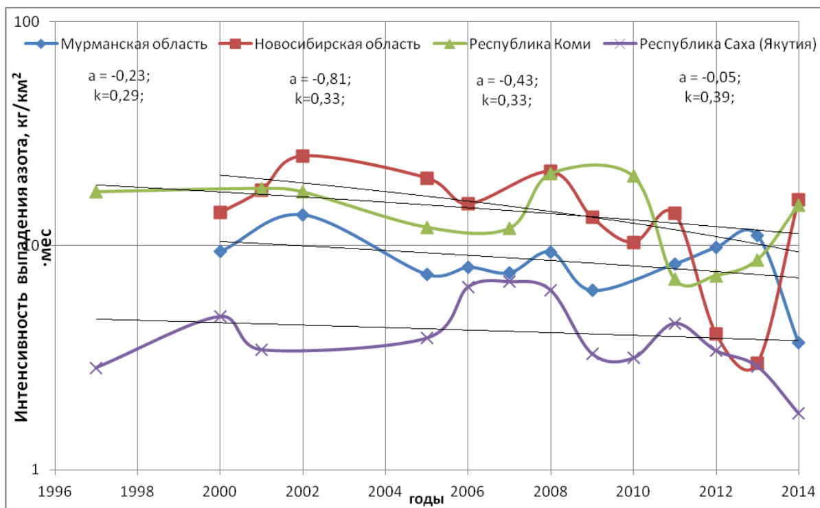
Рис. 2.36. Интенсивность выпадений азота P_N в промышленных и фоновых регионах на ЕТС и АТС по данным мониторинга химического состава снежного покрова в 1997-2014 гг.
