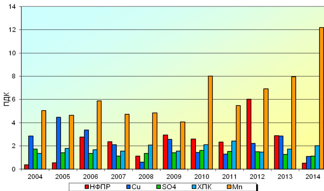
Рис. 3.44. Динамика среднегодового содержания основных загрязняющих веществ в воде Нижнекамского водохранилища в районе д. Андреевка
