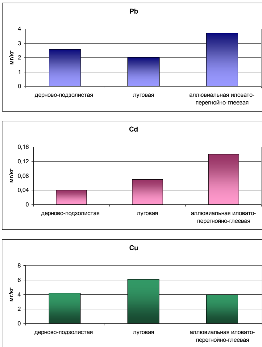
Рис. 2.44. Распределение содержания соединений тяжелых металлов в геохимически сопряженных почвах ландшафта Воронежского БЗ по данным 2013 г.
