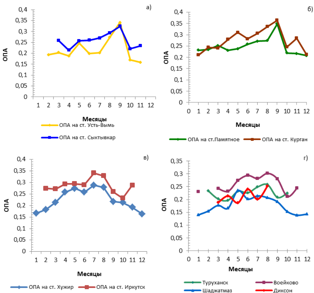
Рис. 2.12. Изменение ОПА в течение года на парных (фоновая - городская) станциях: а) Усть-Вымь-Сыктывкар, б) Памятная-Курган, в) Хужир-Иркутск, г) на непарных станциях - арктическая станция о-в Диксон
