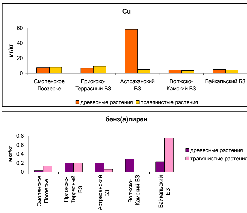
Рис. 2.49. Сравнительное содержание загрязняющих веществ в растительности древесного и травянистого ярусов в биосферных заповедниках
