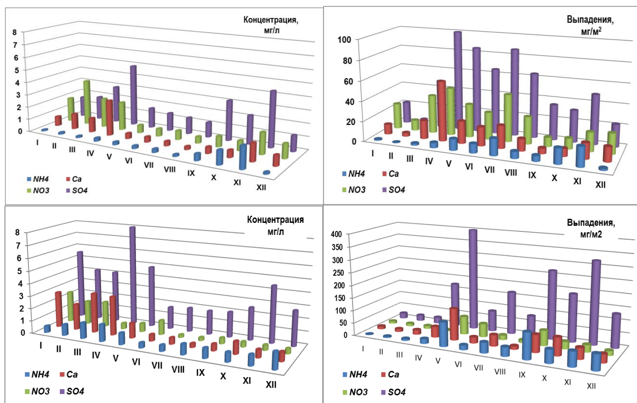
Рис. 2.43. Годовой ход концентраций (слева) и выпадений (справа) основных кислотообразующих ионов с осадками в регионе оз. Байкал (ст. Листвянка, верхний) и на Дальнем Востоке (ст. Приморская, нижний) в 2014 году
