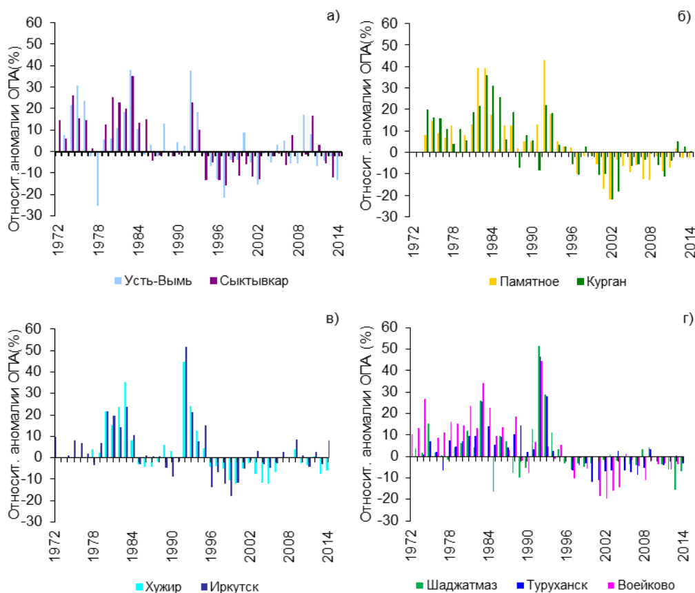
Рис. 2.14. Межгодовая изменчивость относительных аномалий ОПА (%) на парных (а, б, в) и непарных (г) станциях фоновый мониторинга атмосферы
