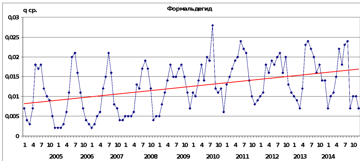
Рис. 4.7. Тенденция изменения концентраций формальдегида (мг/м³) за период 2005-2014 годы в Москве
