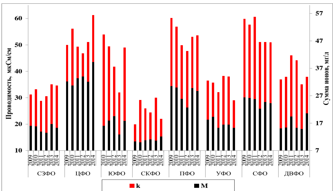
Рис. 2.30. Ход изменений со временем минерализации (тёмные гистограммы) и удельной электропроводности (проводимости) осадков по ФО за период 2009-2014 гг.
