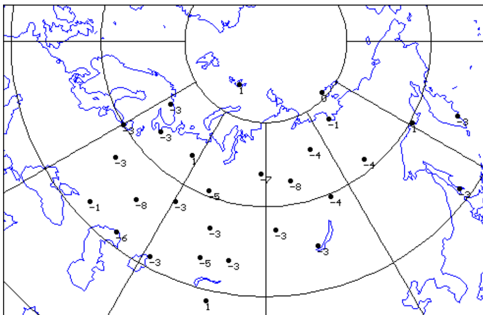
Рис. 2.17. Поле отклонений (%) общего содержания озона в целом за 2014 г. от нормы по данным озонометрической сети стран СНГ
