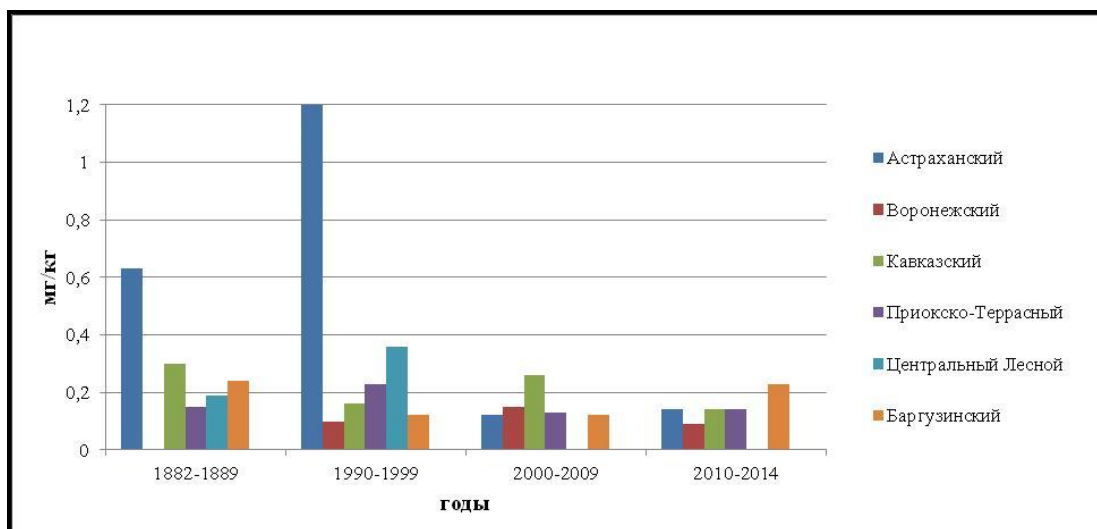
Рис. 2.46. Динамика средних значений валовой концентрации кадмия в почвах биосферных заповедников по 10-ти летним периодам
