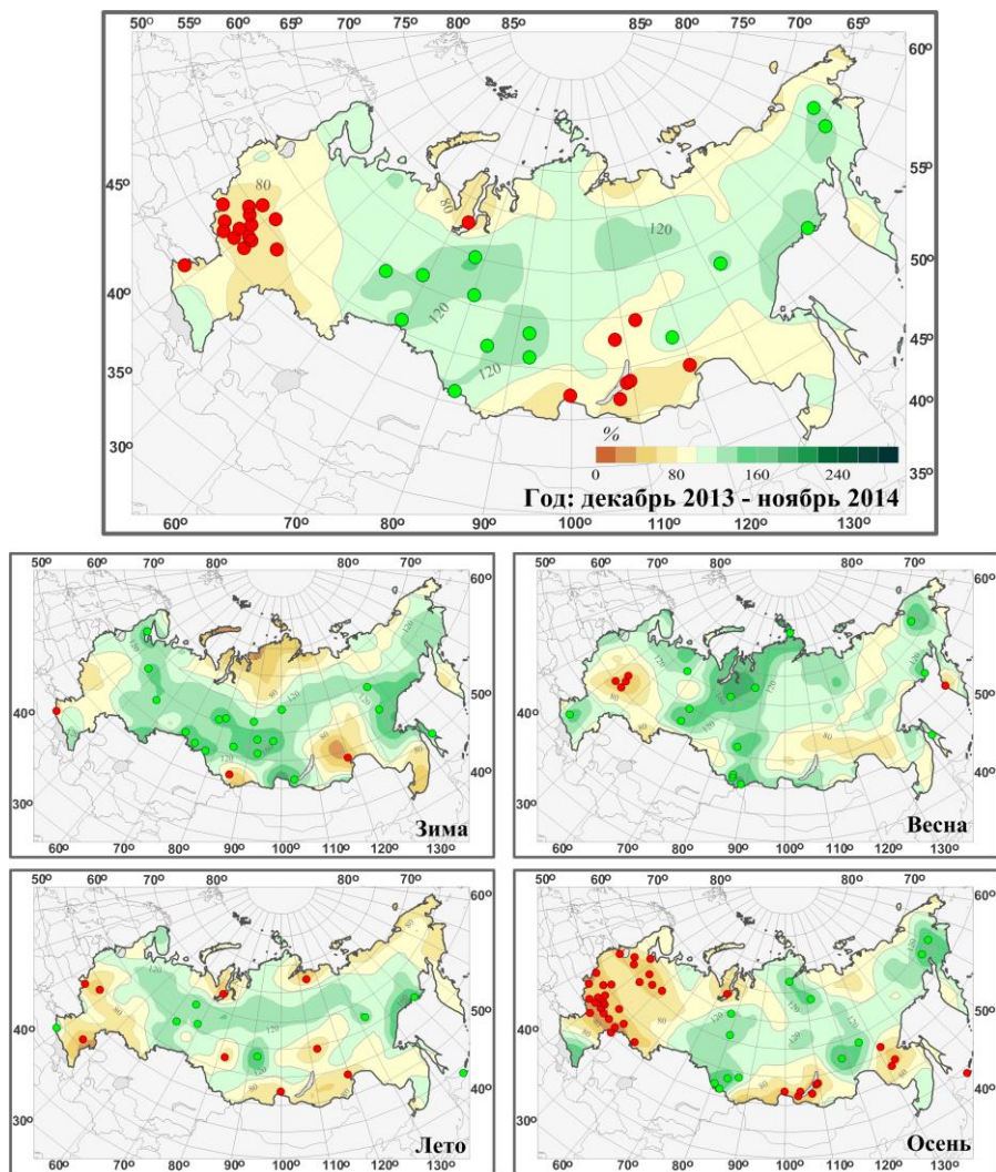
Рис. 1.12. Аномалии годовых и сезонных сумм осадков на территории РФ в 2014 г. (% от нормы 1961-1990 гг.). Кружками красного и зеленого цвета показаны станции, на которых осадки оказались соответственно ниже 5-го или выше 95-го перцентиля
