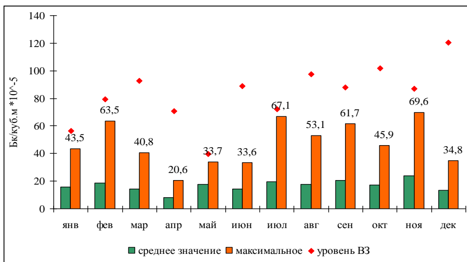
Рис. 4.13. Изменение среднесуточной радиоактивности аэрозолей воздуха в 2014 году
