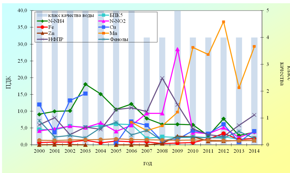
Рис. 3.34. Изменение среднегодовых концентраций отдельных ингредиентов и класса качества воды р. Каменка в 2014 г.
