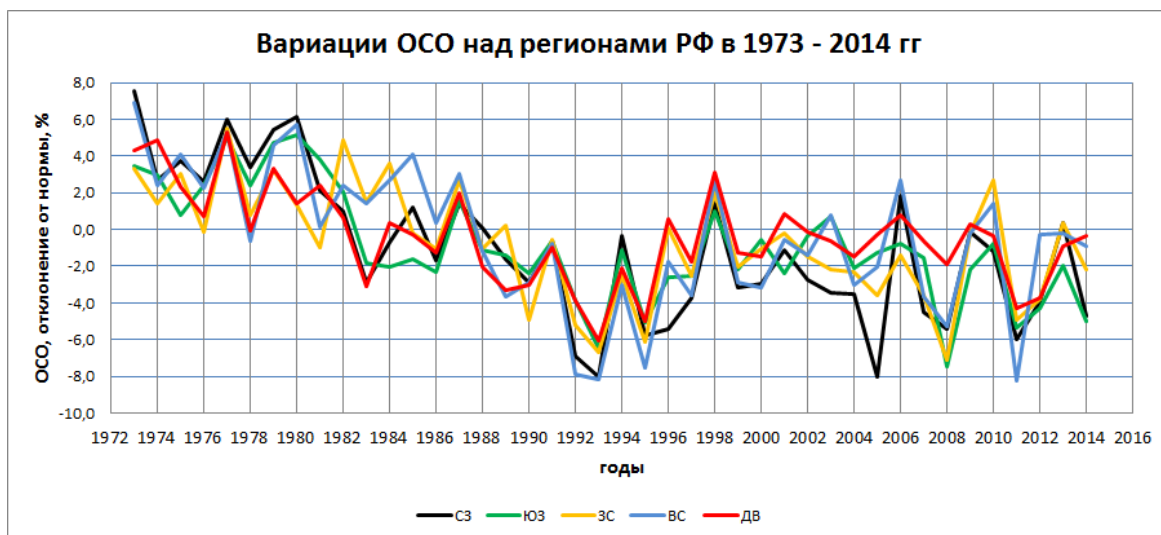
Рис. 2.20. Отклонения среднегодовых значений ОСО от нормы в регионах РФ в период 1973-2014 гг. на Севере Европейской территории России (СЗ), Юге Европейской территории России (ЮЗ), в Западной Сибири (ЗС), в Восточной Сибири (ВС), на Дальнем Востоке (ДВ)
