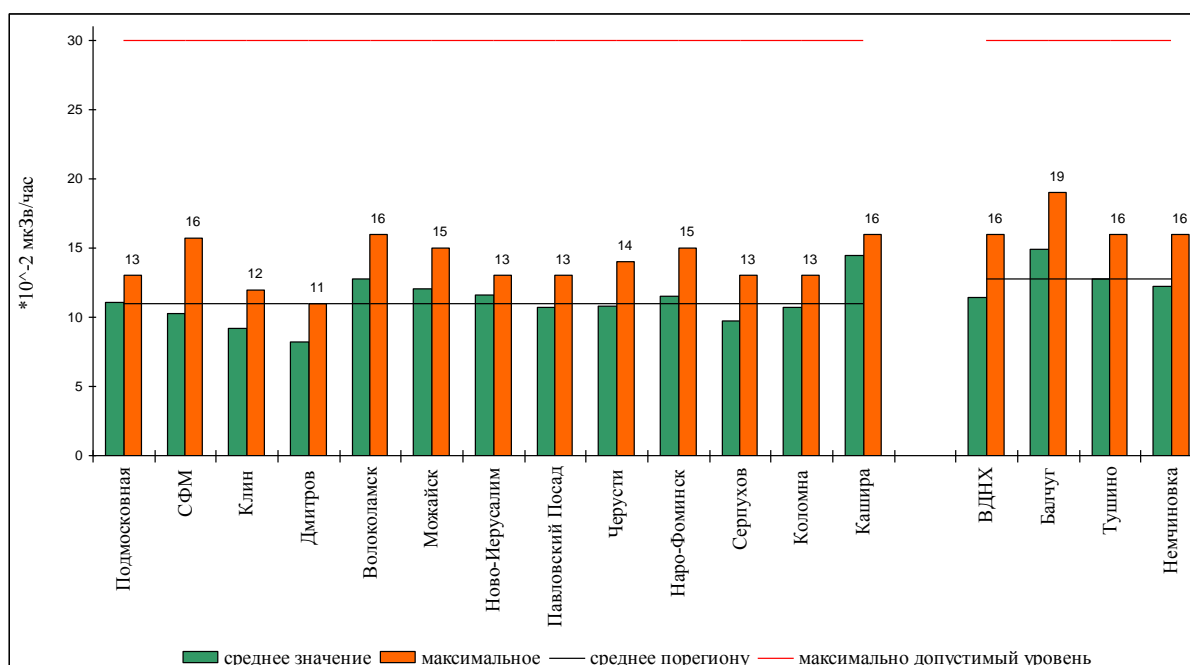
Рис. 4.15. Мощность экспозиционной дозы (МЭД) на станциях московского региона в 2014 году
