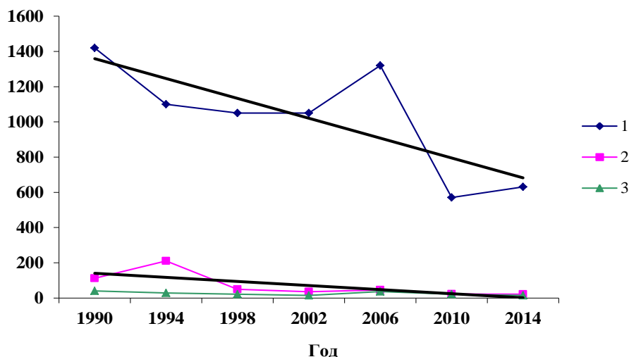
Рис. 3.23. Динамика плотности атмосферных выпадений фтористых соединений (Р) в районах: а) ОАО «РУСАЛ-БрАЗ» (1 - п. Чекановский, 2 км на С от БрАЗ; 2 - п/х «Пурсей», 8 км на СВ; 3 - г. Братск, 12 км на СВ; 4 - п. Падун, 30 км на СВ), б) ОАО «ИрКАЗ-СУАЛ» (1 - г. Шелехов; 2 - г. Иркутск; 3 - п. Листвянка, фон)
