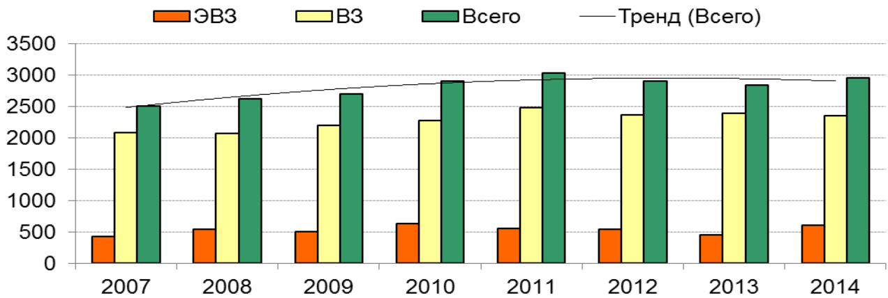
Рис. 3.49. Динамика количества случаев ВЗ и ЭВЗ поверхностных вод суши на территории Российской Федерации
