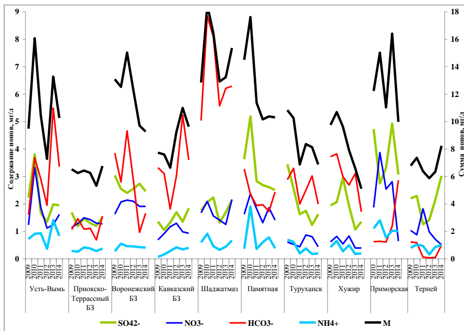
Рис. 2.26. Временной ход концентрации ионов в осадках за период 2009-2014 гг.
