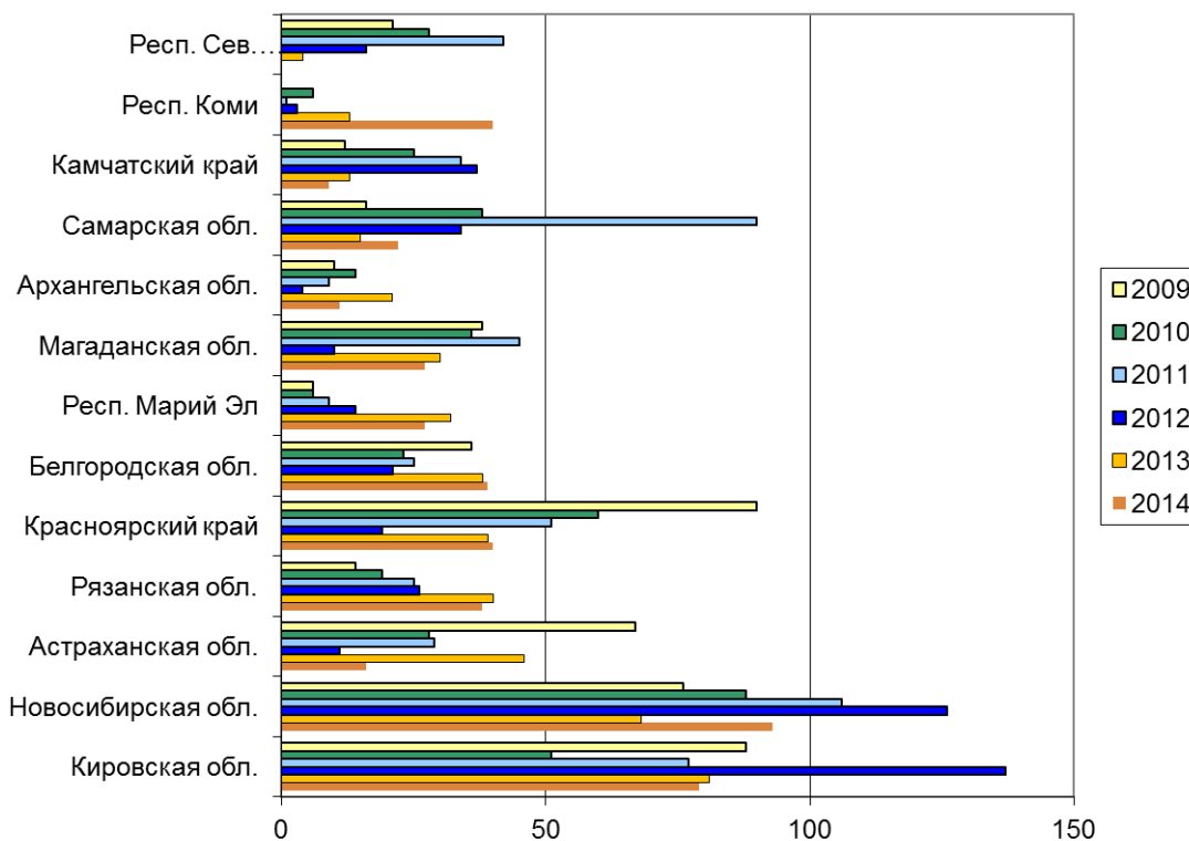
Рис. 3.53. Динамика количества случаев ВЗ и ЭВЗ в отдельных субъектах Российской Федерации
