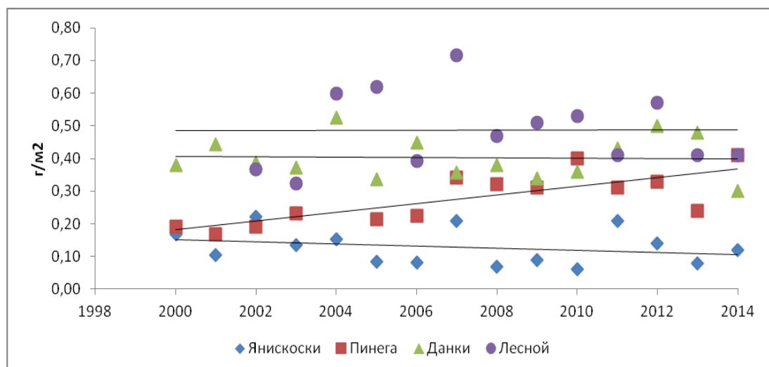
Рис. 2.39. Среднегодовые выпадения суммы нитратного и аммонийного азота из атмосферы с осадками, г N/м 2 /год
