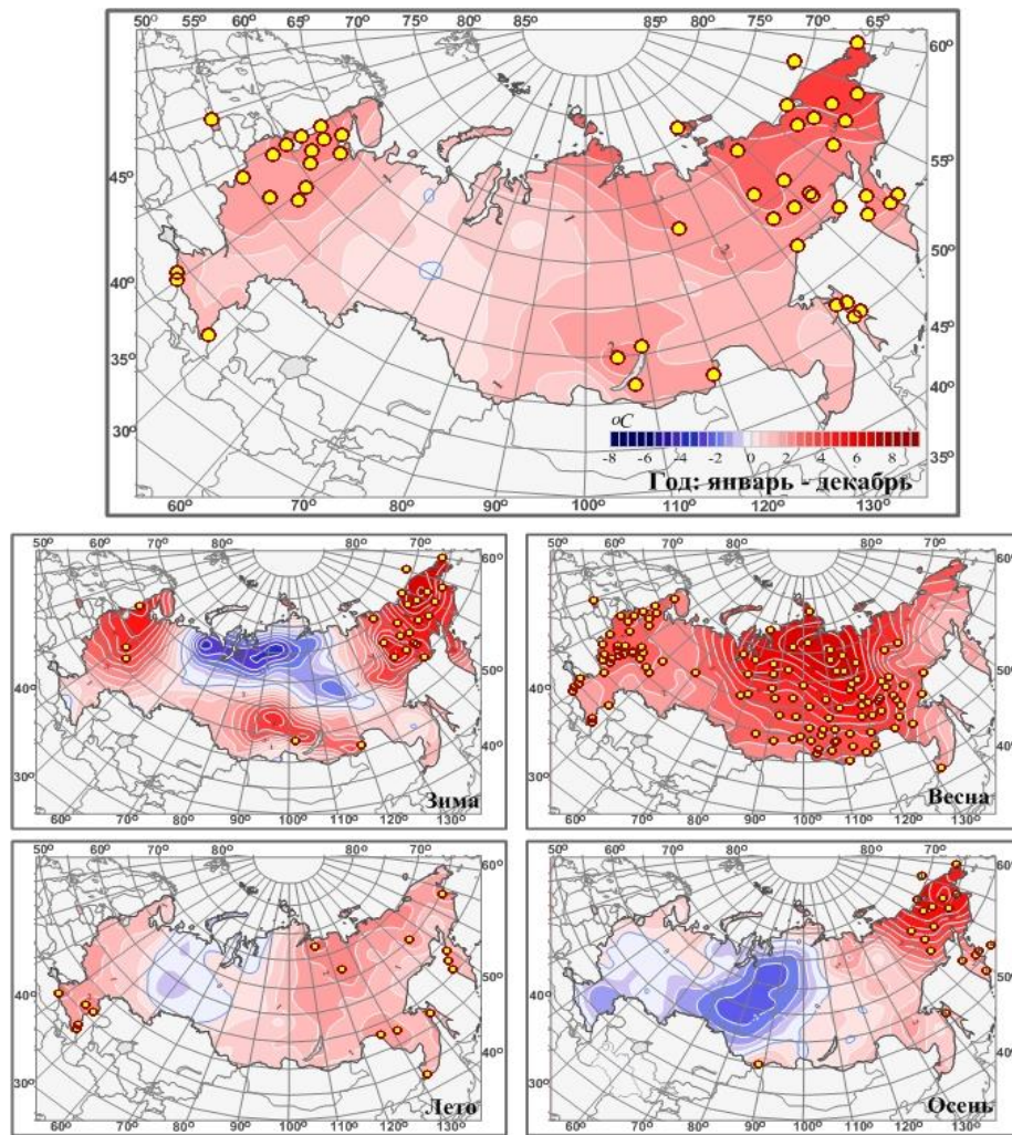
Рис. 1.9. Аномалии средней годовой и сезонных температур приземного воздуха на территории РФ в 2014 г. (отклонения от средних за 1961-1990 гг.) с указанием локализации 5%-х (белые кружки) и 95%-х (желтые кружки) экстремумов
