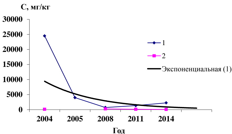
Рис. 3.24. Динамика изменения массовых долей НП (С) в почвах зоны нефтяного пятна (1) размером 2,5 га и за его пределами (2) вблизи пос. Еловка Ангарского района Иркутской области
