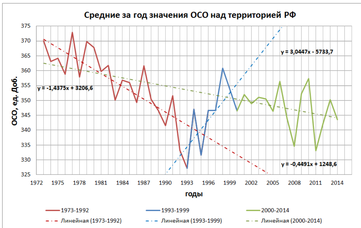
Рис. 2.21. Ход среднегодовых значений ОСО над территорией РФ в период 1973-2014 гг.
