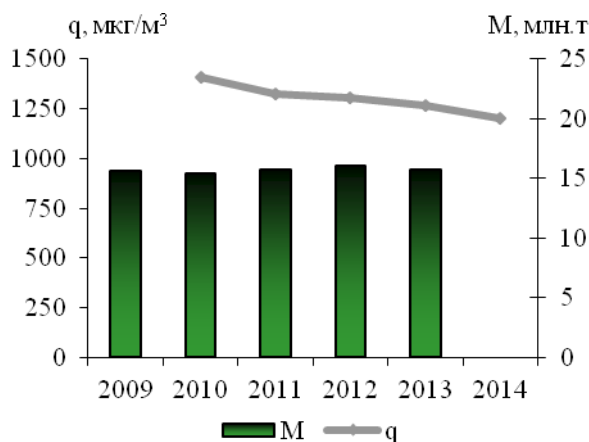
Рис. 3.9. Среднегодовые концентрации (q) взвешенных веществ и суммарные выбросы (M) твердых веществ
