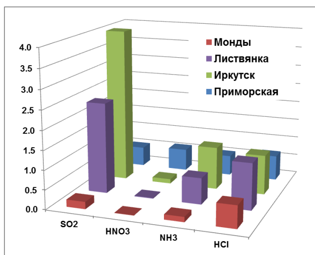
Рис. 2.40. Среднегодовое содержание газовых примесей в воздухе по данным измерений на станциях ЕАНЕТ в 2014 г. (мкг/м³).
