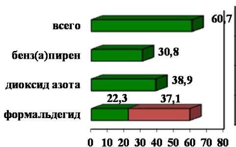
Рис. 3.19. Число жителей в городах (млн.), находящихся под воздействием средних концентраций примесей в воздухе выше 1 ПДК, для формальдегида дано с учетом прежней и новой ПДК
