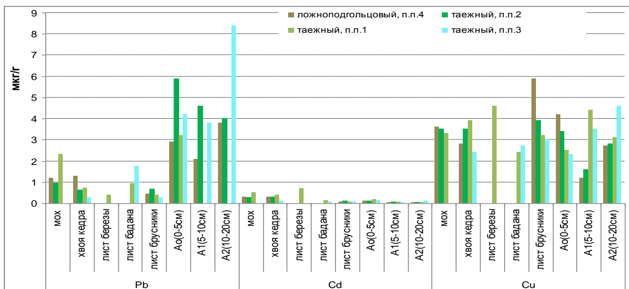
Рис. 4.18. Распределение тяжелых металлов в образцах растений и почвы по высотным поясам биосферного Фролихинского заказника
