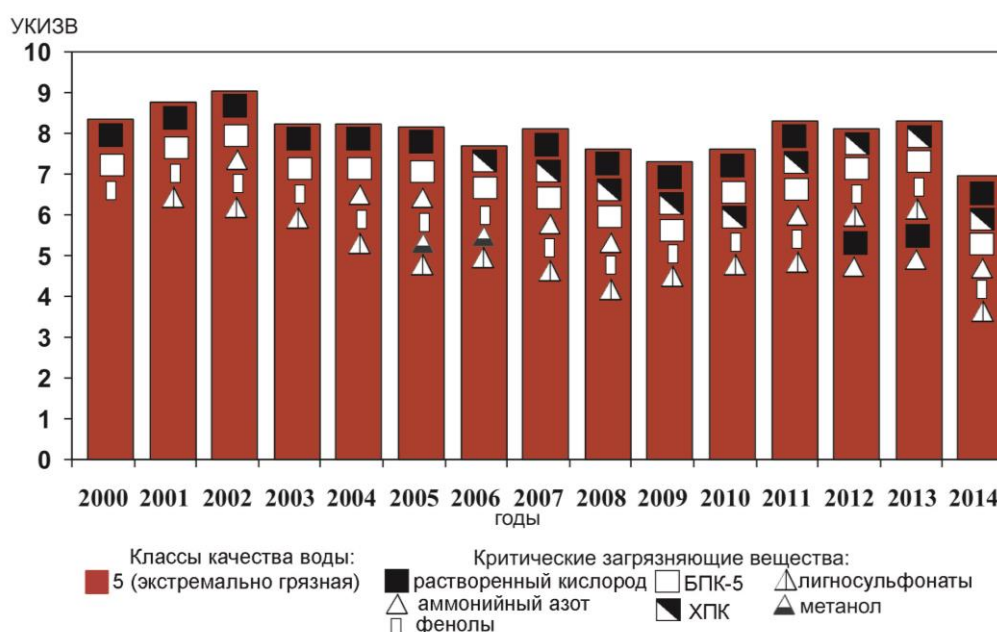
Рис. 3.32. Динамика качества воды р. Пельшма, г. Сокол в многолетнем плане
