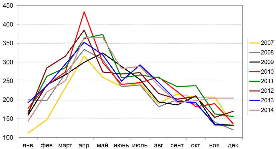
Рис. 3.50. Динамика внутригодичного распределения количества случаев ВЗ и ЭВЗ поверхностных вод суши на территории Российской Федерации за период 2007-2014 гг.
