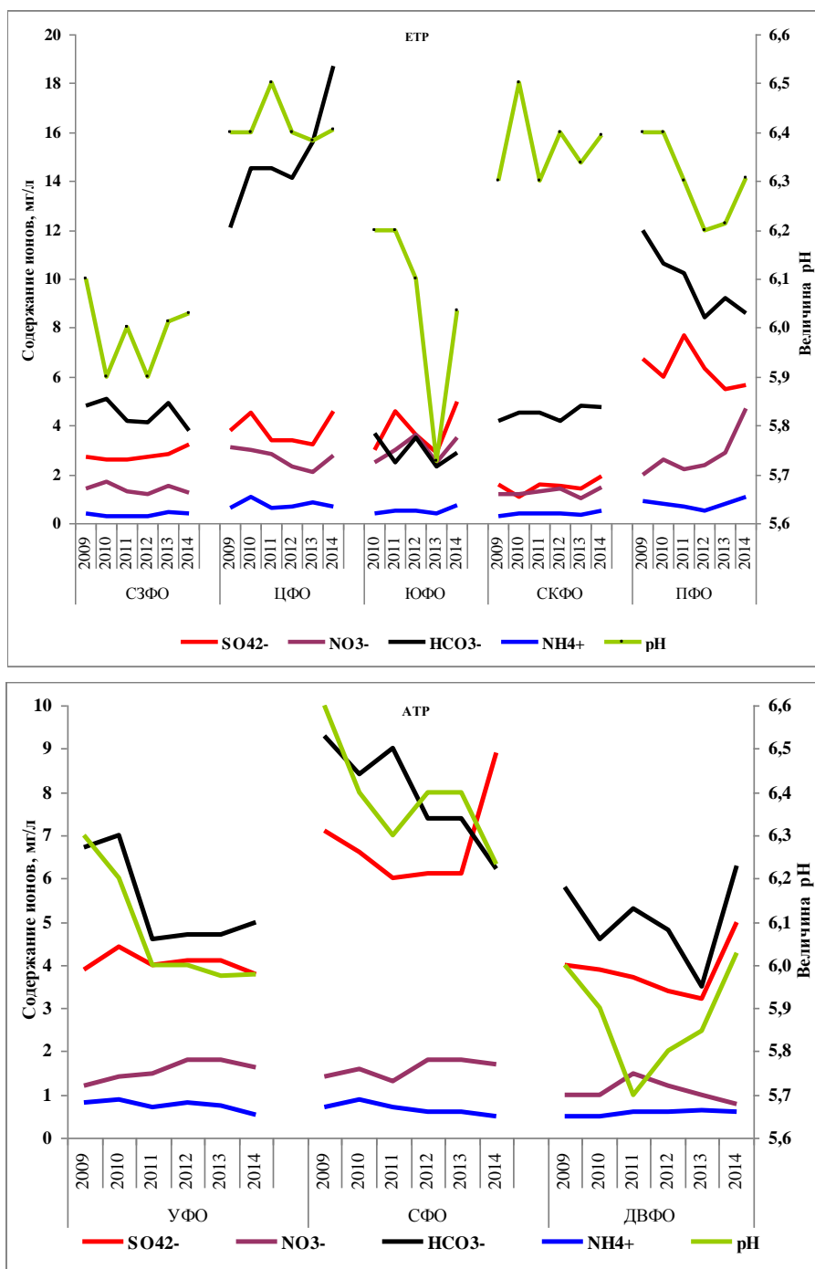
Рис. 2.31. Временной ход концентрации ионов в осадках по Федеральным округам
