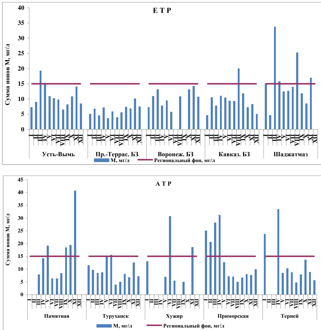
Рис. 2.25. Изменения суммы ионов в осадках по месяцам на ЕТР и АТР в 2014 году
