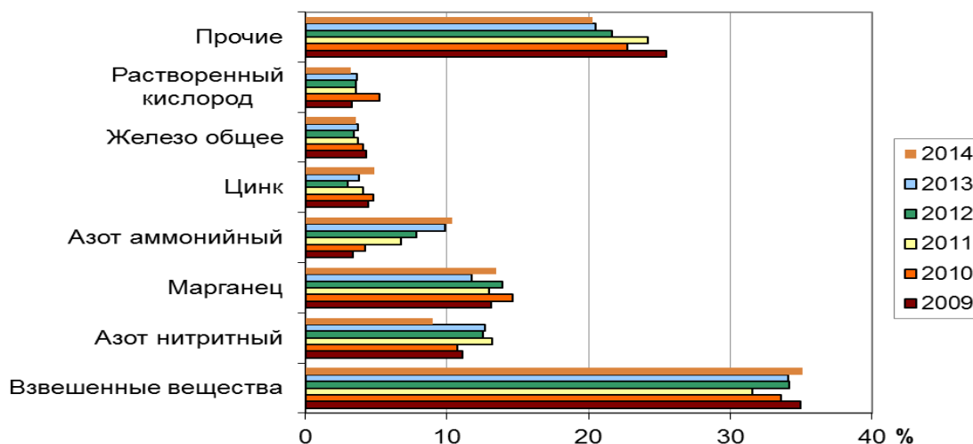
Рис. 3.54. Распределение случаев ВЗ и ЭВЗ по ингредиентам (в % от общего количества случаев ВЗ и ЭВЗ)
