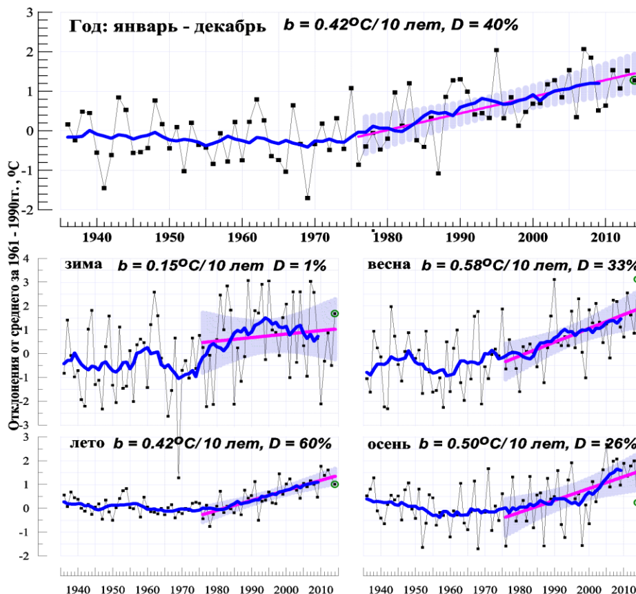
Рис. 1.8. Средние годовые (вверху) и сезонные аномалии температуры приземного воздуха ( ^{\circ}\text{C} ), осредненные по территории РФ, 1936-2014 гг. Аномалии рассчитаны как отклонения от среднего за 1961-1990 гг. Показаны также 11 - летнее скользящее среднее, линейный тренд за 1976-2014 гг. с 95%-й доверительной полосой; b - коэффициент тренда ( ^{\circ}\text{C}/10 лет), D - вклад в суммарную дисперсию (%)
