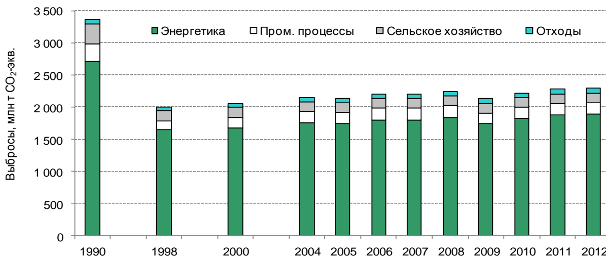
Рис. 2.1. Динамика выбросов парниковых газов в атмосферу, без учета сектора землепользования, изменения землепользования и лесного хозяйства
