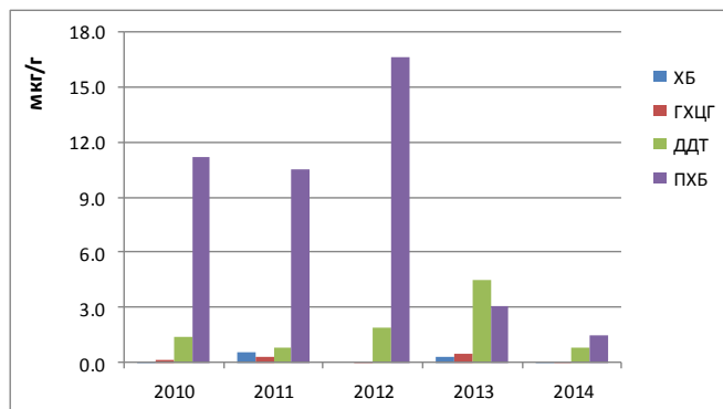
Рис. 4.27. Изменения средних концентраций ХОС в снежном покрове за период 2010-2014 года
