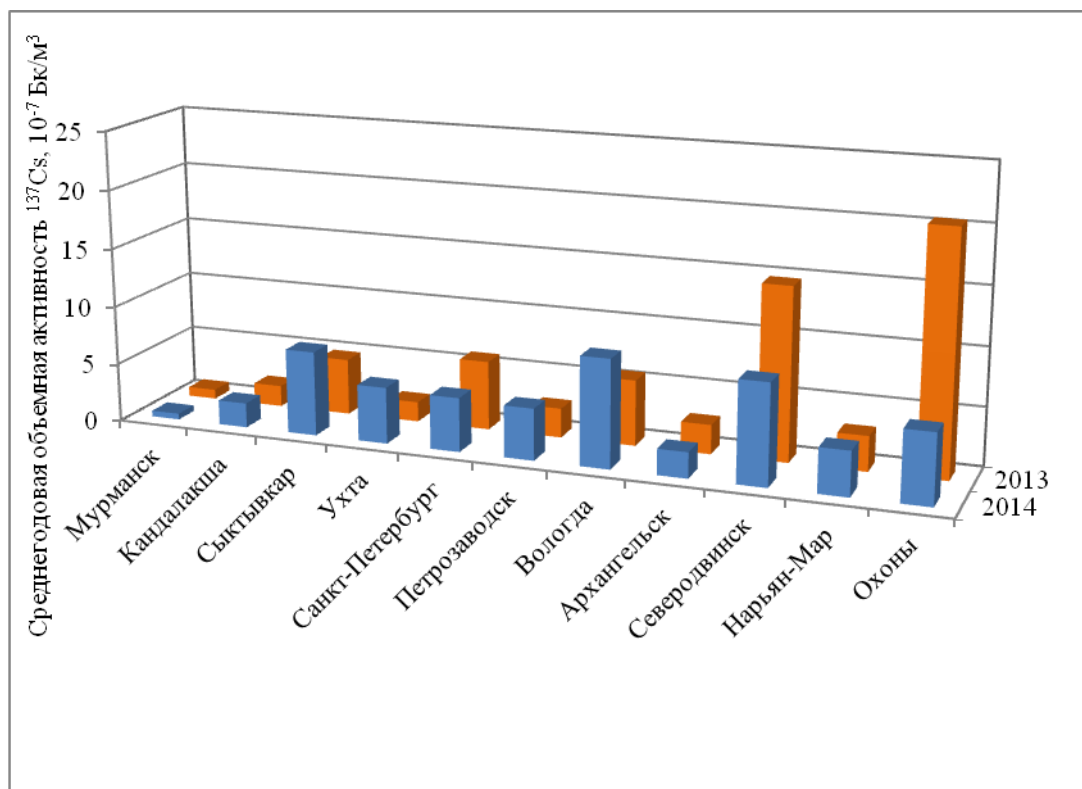
Рис. 2.59. Среднегодовая объемная активность 137 Cs в населенных пунктах СЗО в 2013-2014 годах, 10 -7 Бк/м 3
