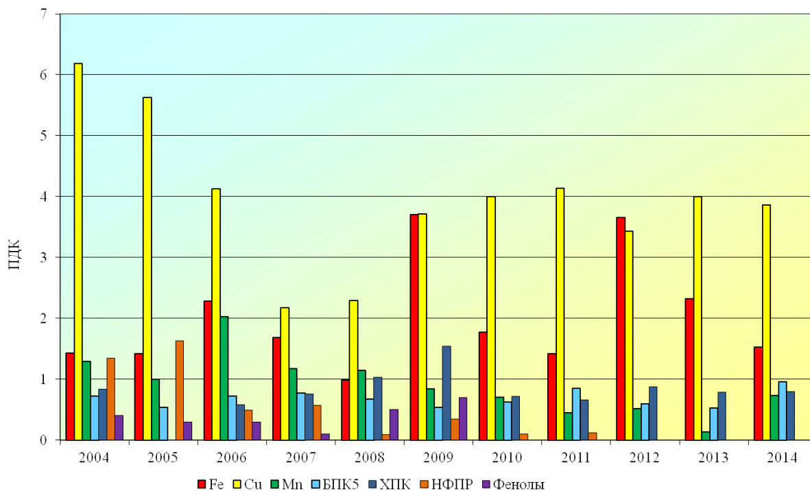
Рис. 2.56. Динамика среднегодового содержания основных загрязняющих веществ в воде р. Правда выше п. Правда
