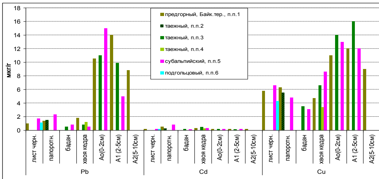
Рис. 4.21. Содержание тяжелых металлов в образцах растений и почвы по высотным поясам в Байкальском заповеднике (р. Осиновка-Танхойская, 2012 г.)
