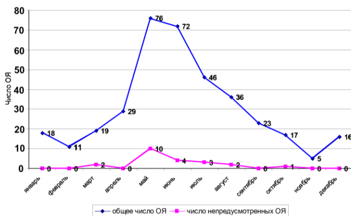
Рис. 1.7. Распределение гидрометеорологических ОЯ, нанесших ущерб, по месяцам в 2014 году
