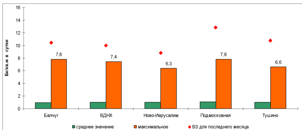
Рис. 4.14. Радиоактивные выпадения (планшет) на станциях московского региона в 2014 году
