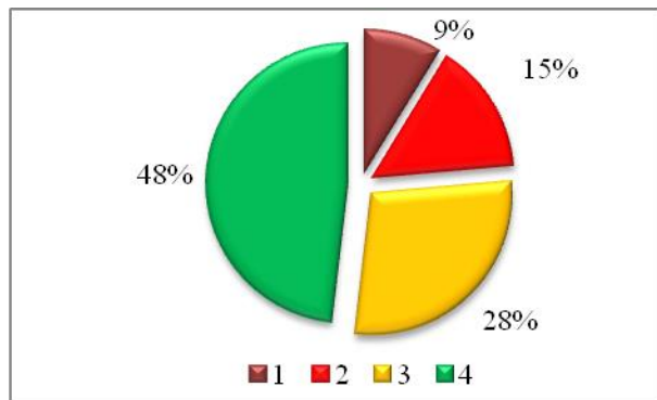
Рис. 3.15. Количество городов (%), где ИЗА ≥ 14 (1), 7-13 (2), 5-6 (3), ≤5 (4)
