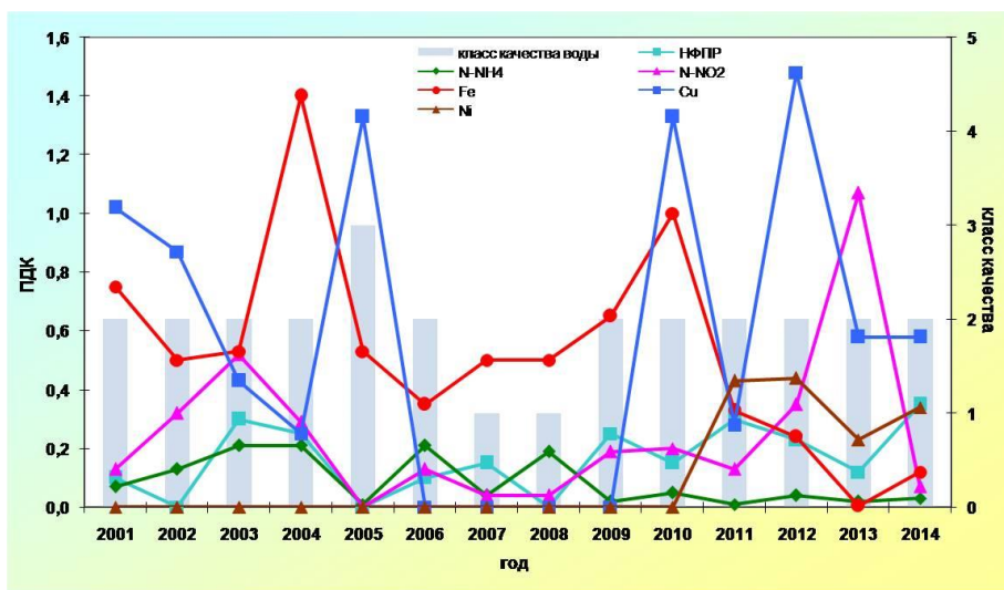
Рис. 2.54. Изменение среднегодовых концентраций отдельных ингредиентов и качества воды р. Лена, р.п. Качуг
