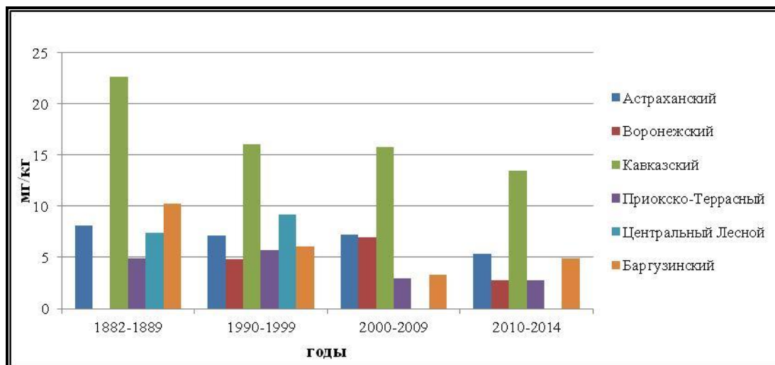
Рис. 2.45. Динамика средних значений валовой концентрации свинца в почвах биосферных заповедников по 10-ти летним периодам
