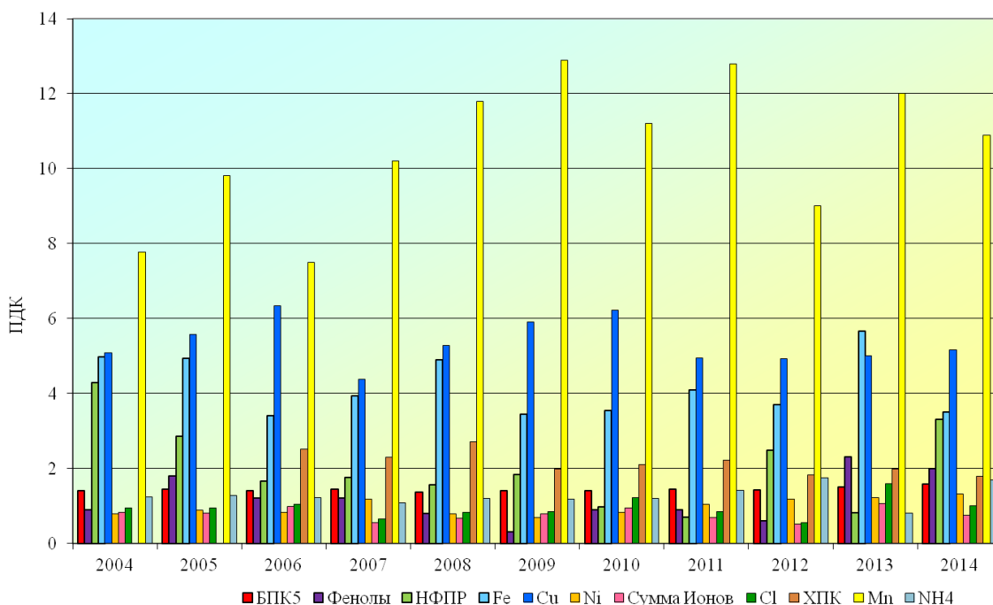
Рис. 3.46. Динамика среднегодового содержания основных загрязняющих веществ в воде р. Белая в створе 10,5 км ниже г. Стерлитамак
