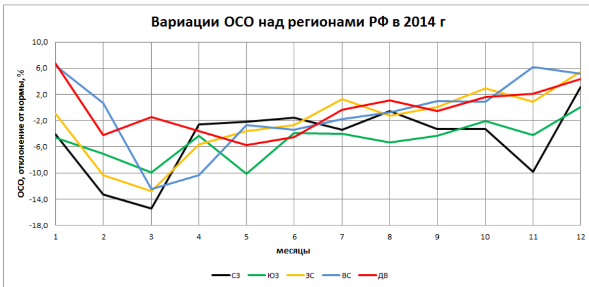
Рис. 2.19. Отклонения среднемесячных значений ОСО от нормы в регионах РФ в 2014 году на Севере Европейской территории России (СЗ), Юге Европейской территории России (ЮЗ), в Западной Сибири (ЗС), в Восточной Сибири (ВС), на Дальнем Востоке (ДВ)
