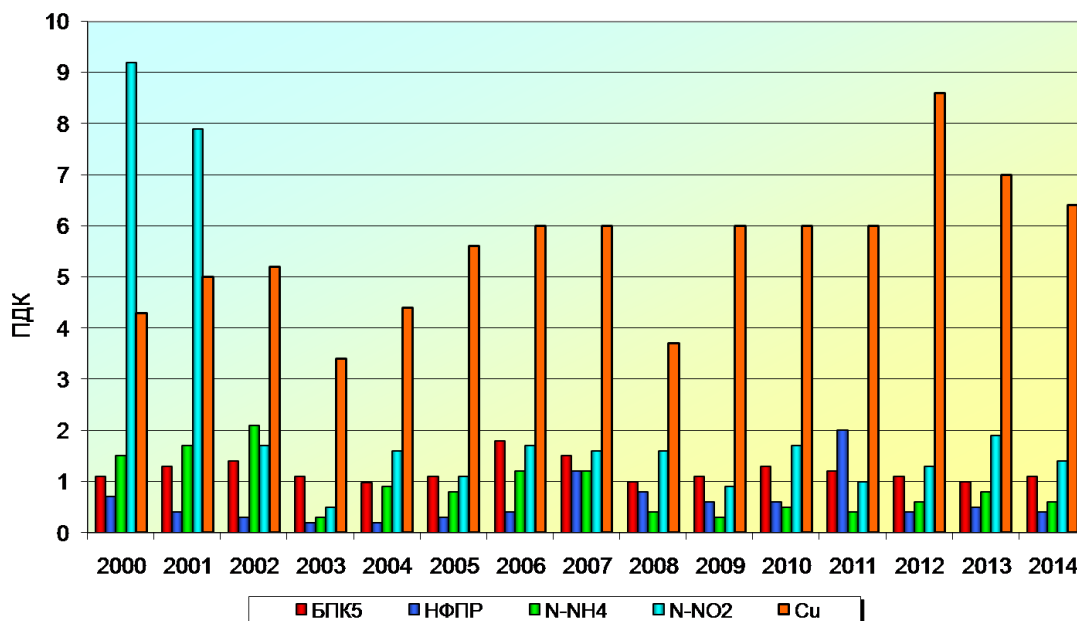
Рис. 3.40. Динамика содержания загрязняющих веществ в воде Чебоксарского водохранилища, 4,2 км ниже г. Нижний Новгород
