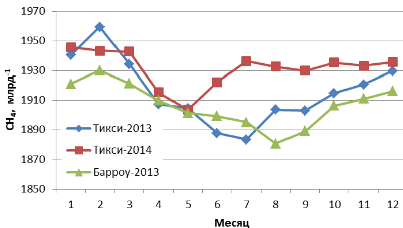
Рис. 2.8. Сезонный ход концентрации CH 4 для станции Тикси и Барроу
