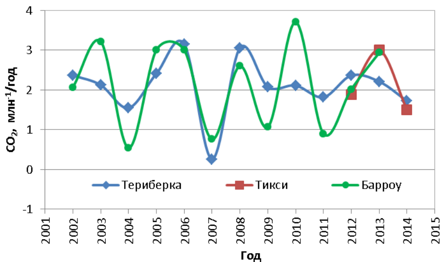
Рис. 2.5. Межгодовые изменения концентрации CO 2
