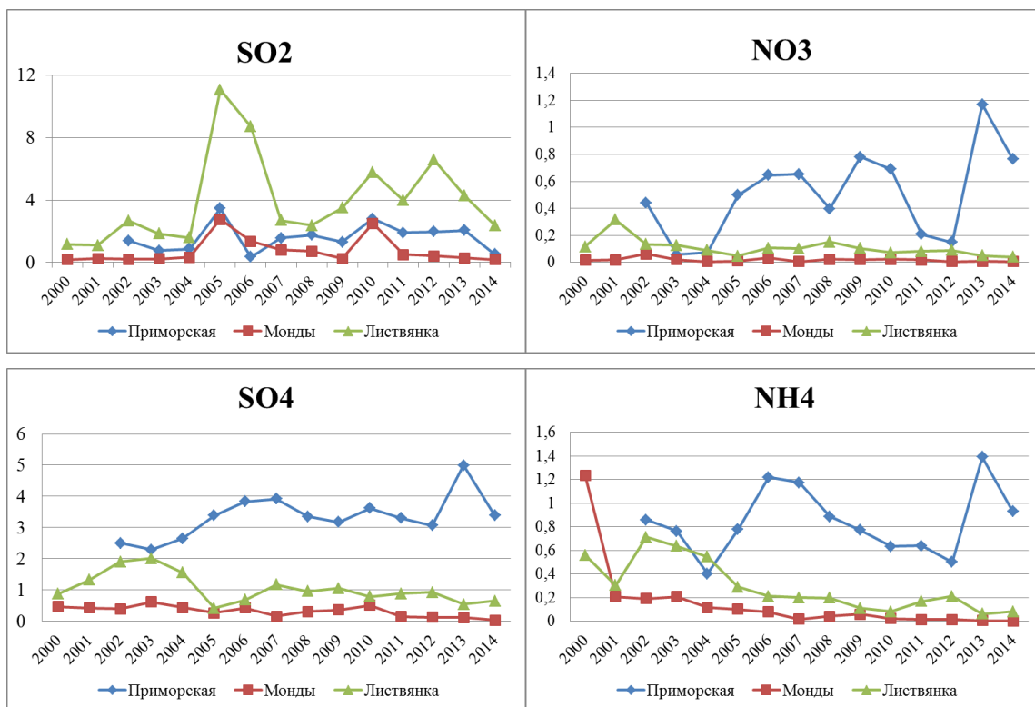
Рис. 2.42. Изменения средних годовых концентрации соединений серы (слева) и азота (справа) в воздухе на станциях ЕАНЕТ (мкг/м 3 )
