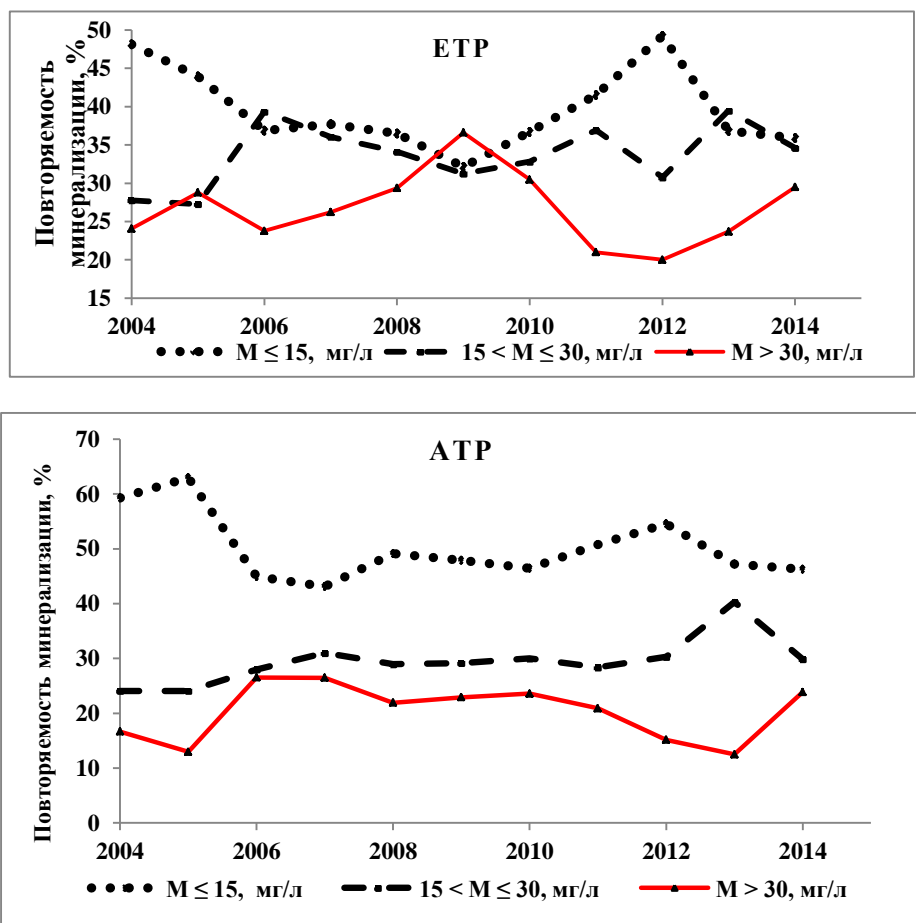
Рис. 2.29. Ход изменений минерализации осадков по ЕТР и АТР за период 2004-2014 гг.
