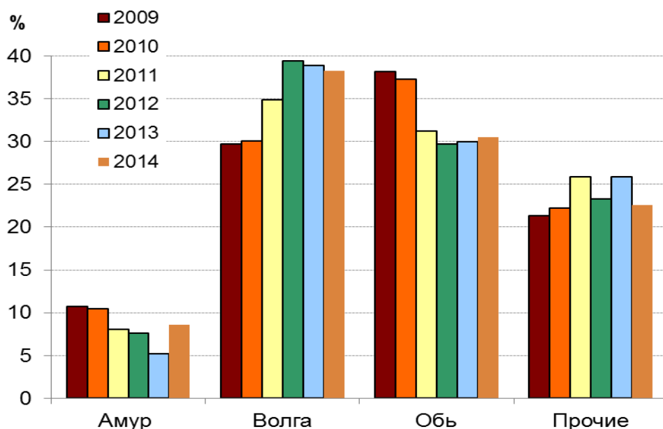
Рис. 3.51. Распределение случаев ВЗ и ЭВЗ по бассейнам рек (в % от общего числа случаев на территории Российской Федерации) за период 2009-2014 гг.
