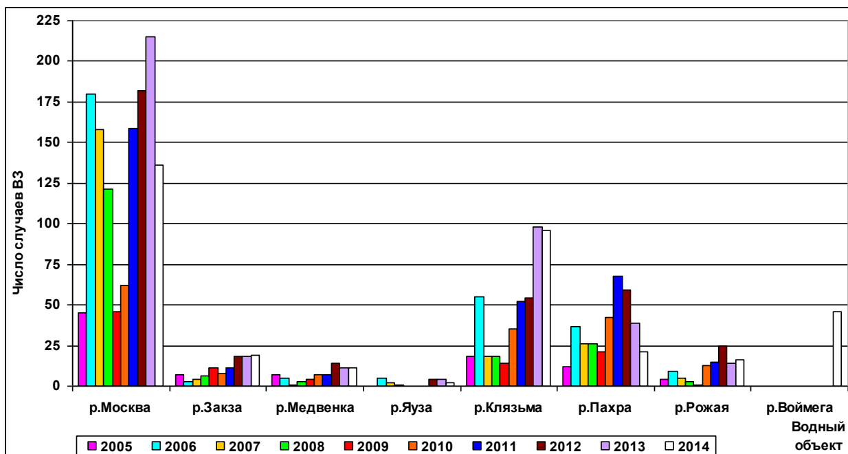
Рис. 4.11. Распределение случаев высокого загрязнения по водотокам Московского региона в 2005-2014 гг.
