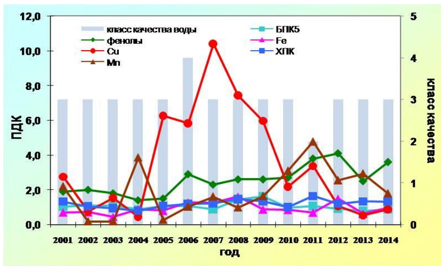
Рис. 3.37. Изменение среднегодовых концентраций отдельных ингредиентов и качества воды р. Лена, г. Якутск в многолетнем плане
