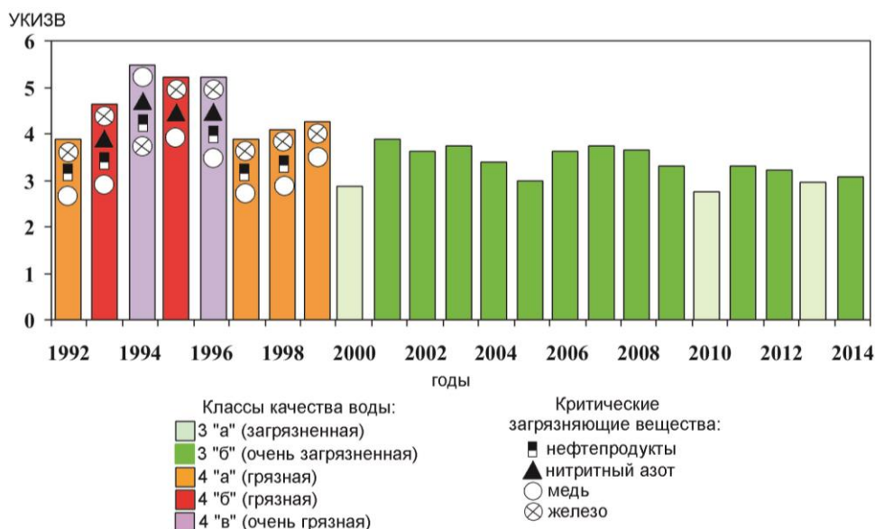
Рис. 3.30. Динамика качества воды р. Кубань, г. Краснодар в многолетнем плане
