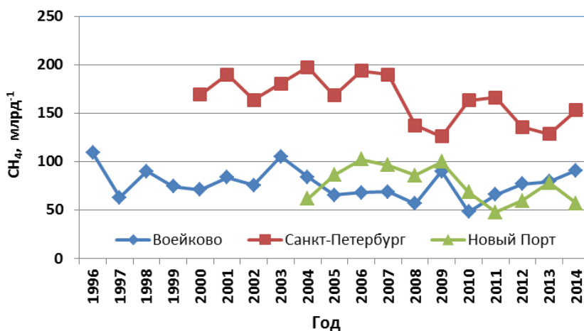
Рис. 2.10. Среднегодовое превышение концентрации CH 4 над фоновым уровнем
