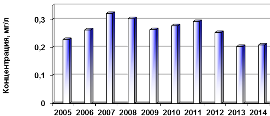
Рис. 4.10. Изменение среднегодовых концентраций фосфатов в целом по водным объектам Московского региона
