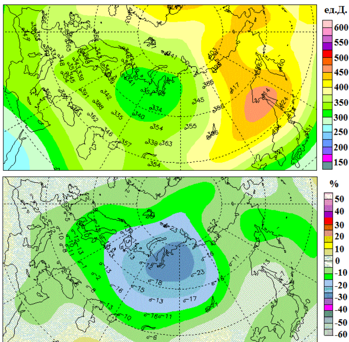
Рис. 2.18. Поле общего содержания озона (ед. Д.;верху) в марте 2014 г. и его отклонения (%; внизу) от средних многолетних (1978-1988 гг.) значений по данным WOUDC, Канада
