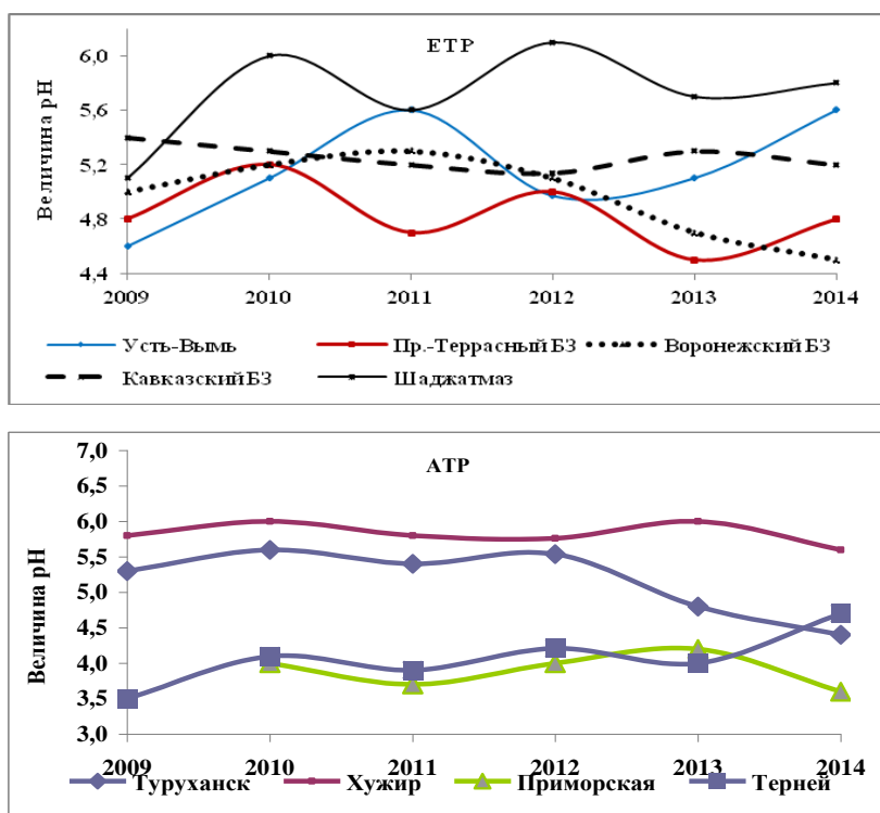
Рис. 2.28. Ход изменений со временем абсолютно минимальной величины pH осадков на станциях ЕТР и АТР
