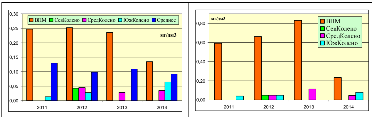
Рис. 3.59. Динамика средней и максимальной концентрации нефтяных углеводородов (мг/дм³) в водах порта г. Мурманск и Северном, Среднем и Южном коленах Кольского залива
