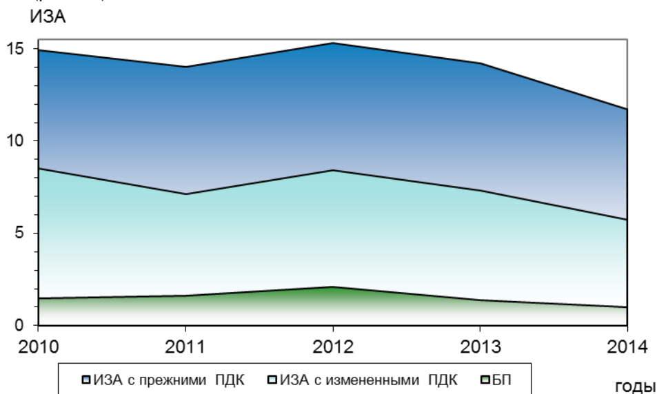
Рис. 4.5. Изменение комплексного ИЗА, рассчитанного с прежними и измененными величинами ПДК с.с. формальдегида, и тенденция загрязнения воздуха бенз(а)пиреном в г. Москве за 2010-2014 гг.
