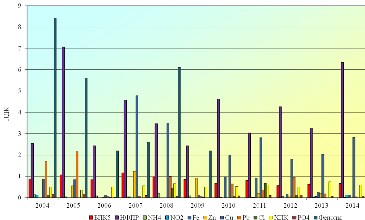
Рис. 2.57. Динамика среднегодового содержания основных загрязняющих веществ в воде р. Берш 2,5 км к западу от с. Пушино
