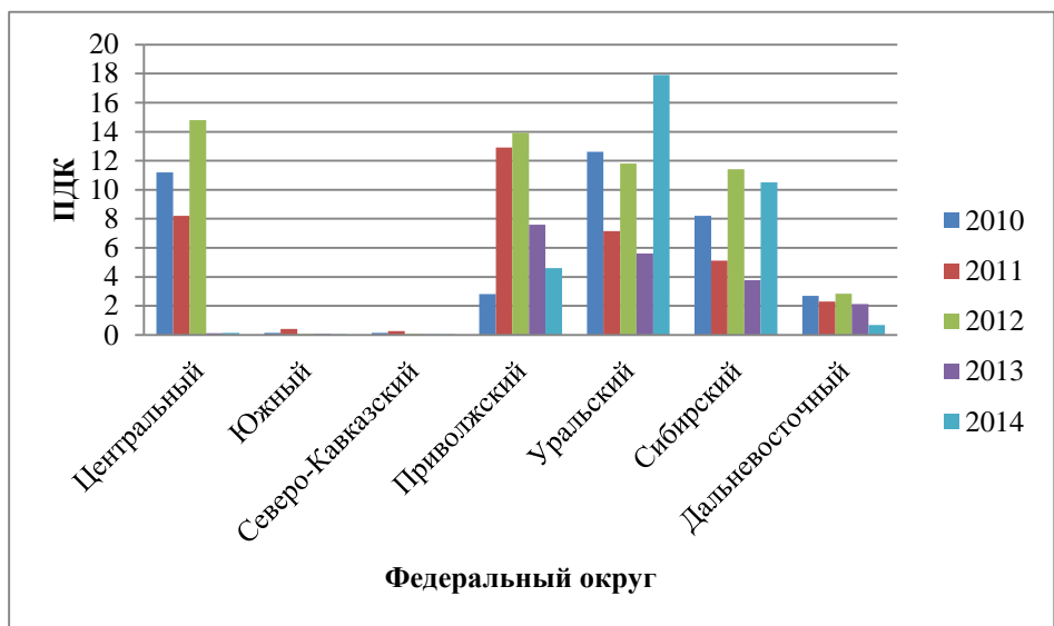
Рис. 3.25. Максимальное содержание ДДТ в почвах (в долях ПДК)
