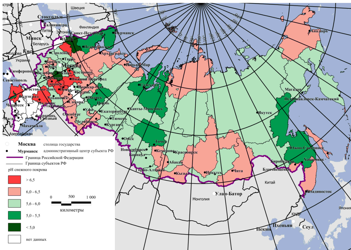
Рис.2.32. Средние показатели кислотности (рН) к снежного покрова в регионах РФ в зимний период 2013-2014 гг.
