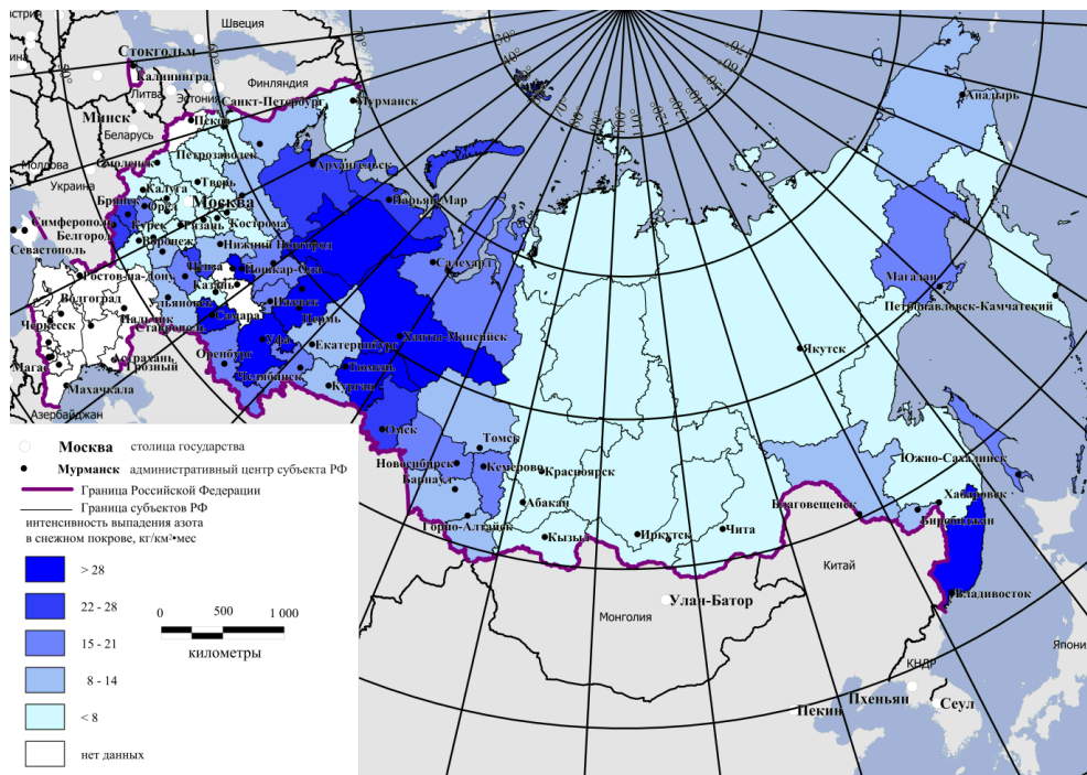
Рис. 2.35. Средняя интенсивность выпадений азота P_N в регионах РФ в зимний период 2013-2014 гг. по данным мониторинга содержания нитратов и ионов аммония в снежном покрове
