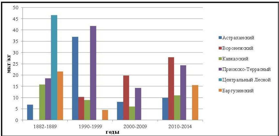
Рис. 2.48. Динамика средних значений концентрации ДДТ (с метаболитами) в почвах биосферных заповедников по 10-ти летним периодам
