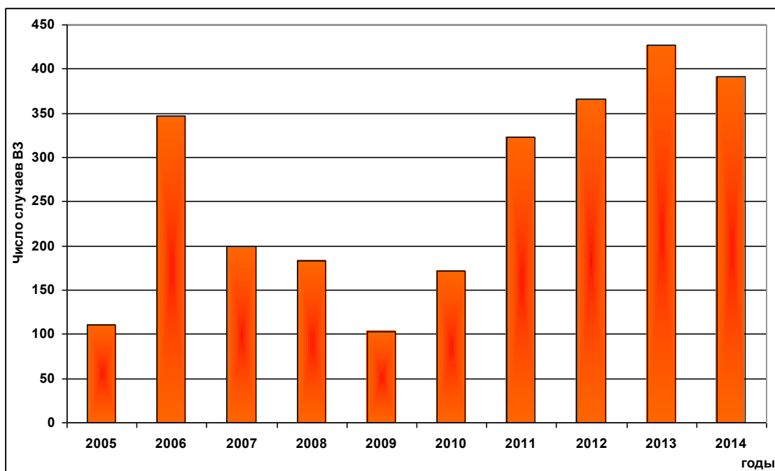
Рис. 4.12. Изменение количества случаев высокого загрязнения водотоков Московского региона в 2005-2014 гг.
