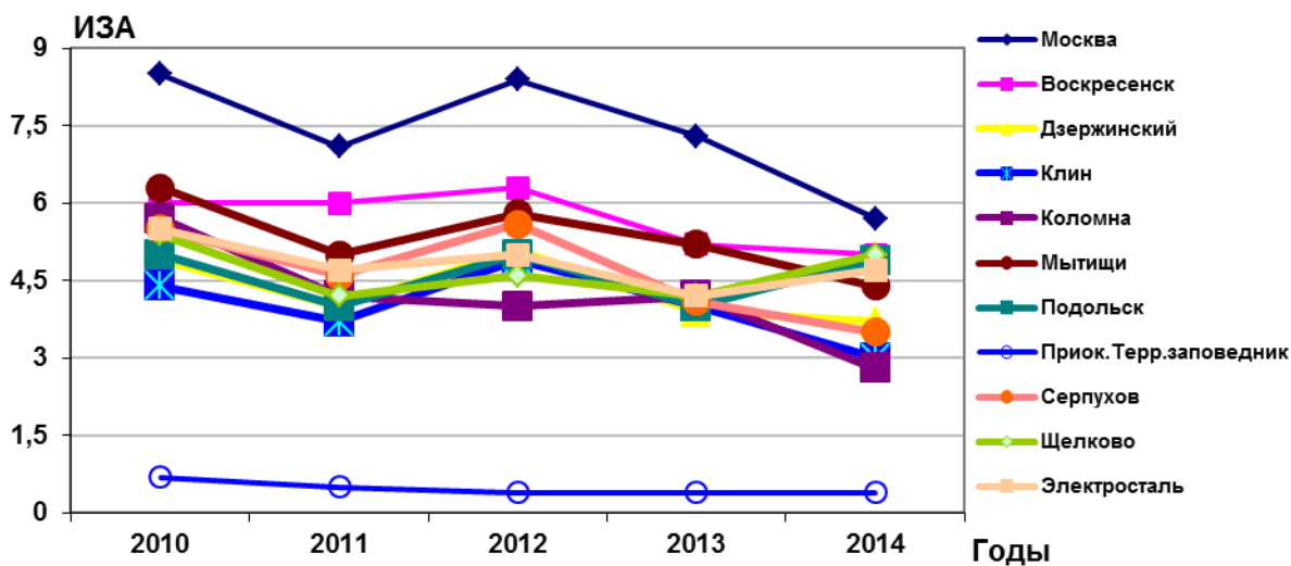
Рис. 4.2. Степень загрязнения атмосферного воздуха в Московском регионе
