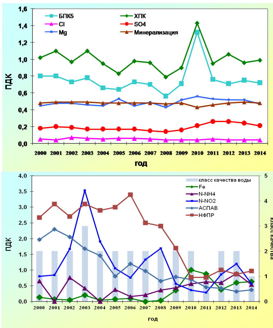
Рис. 2.51. Изменение среднегодовых концентраций основных ингредиентов и качества воды р. Лесной Воронеж, выше г. Мичуринск
