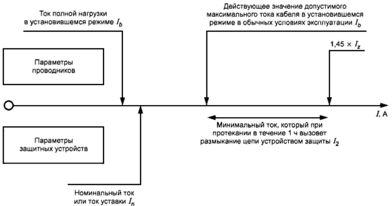
Рисунок D.2 - Параметры проводников и защитных устройств
