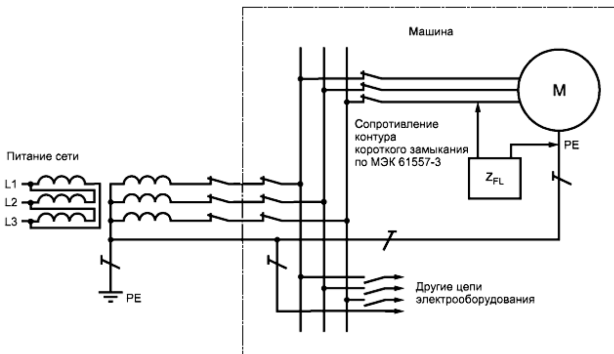
Рисунок А.1 - Типовая схема измерения полного сопротивления контура короткого
