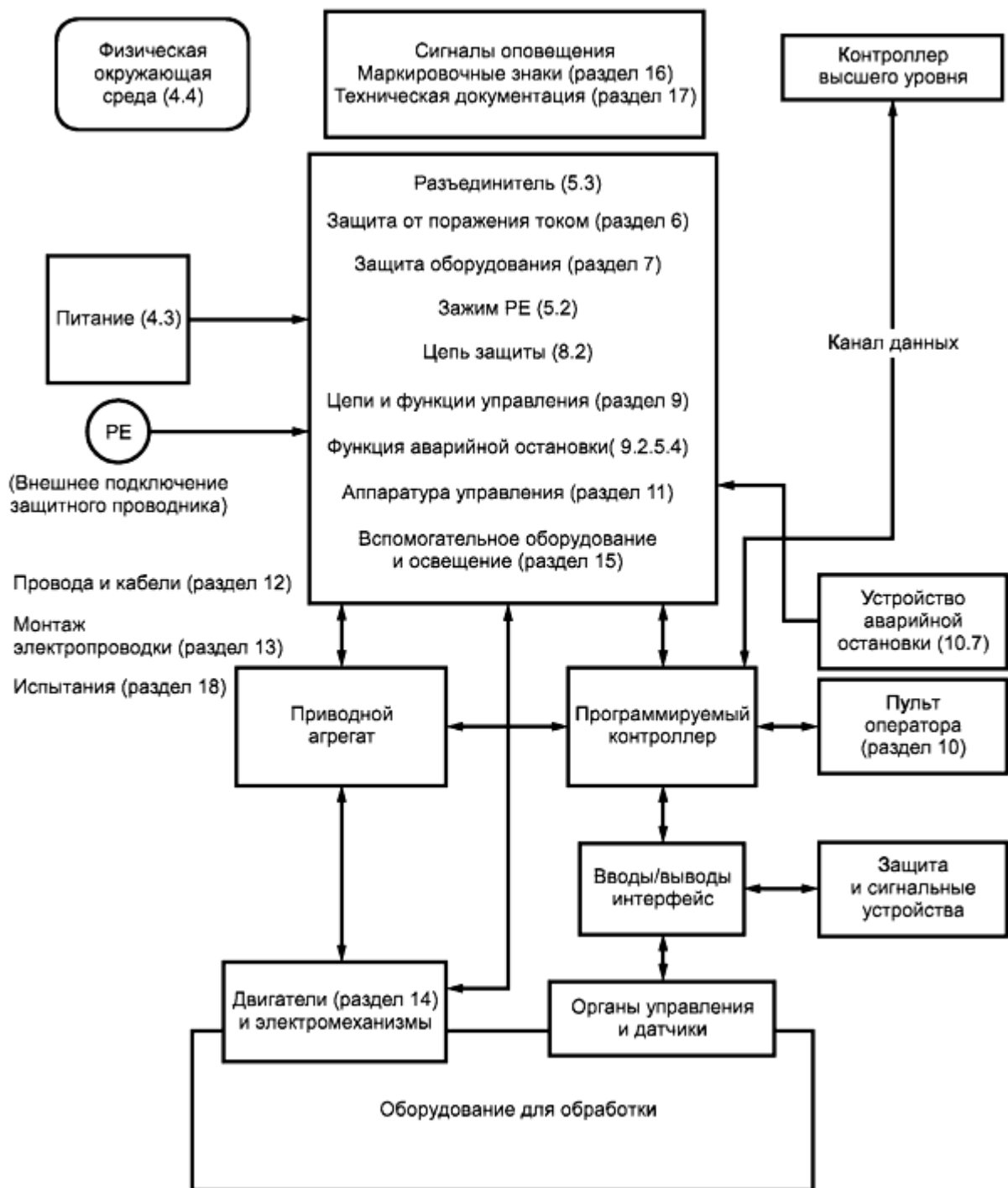
Рисунок 1 - Функциональная схема типовой машины
