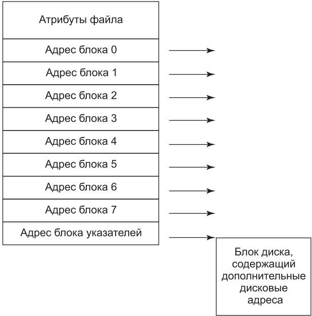
Рис. 4.10. Пример i-узла
