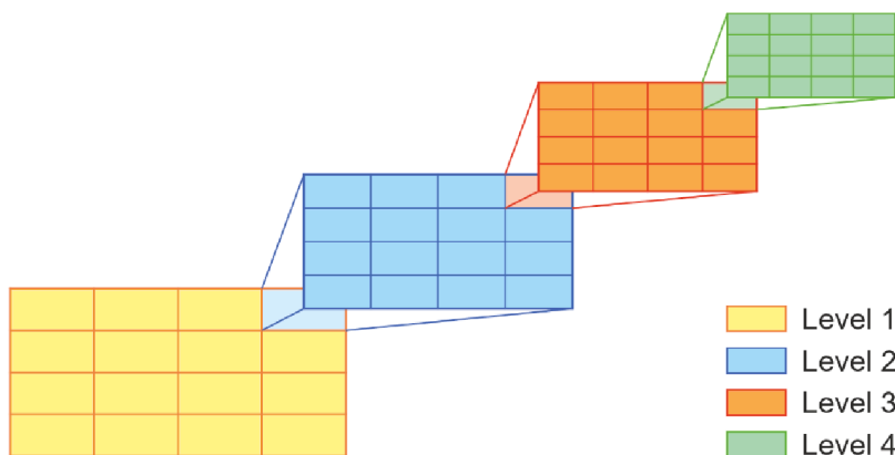
Рисунок 43 – Пространственная сетка
