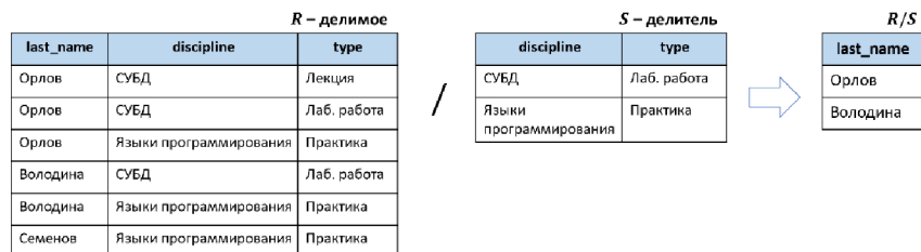
Рисунок 25 – Операция «Деление»
