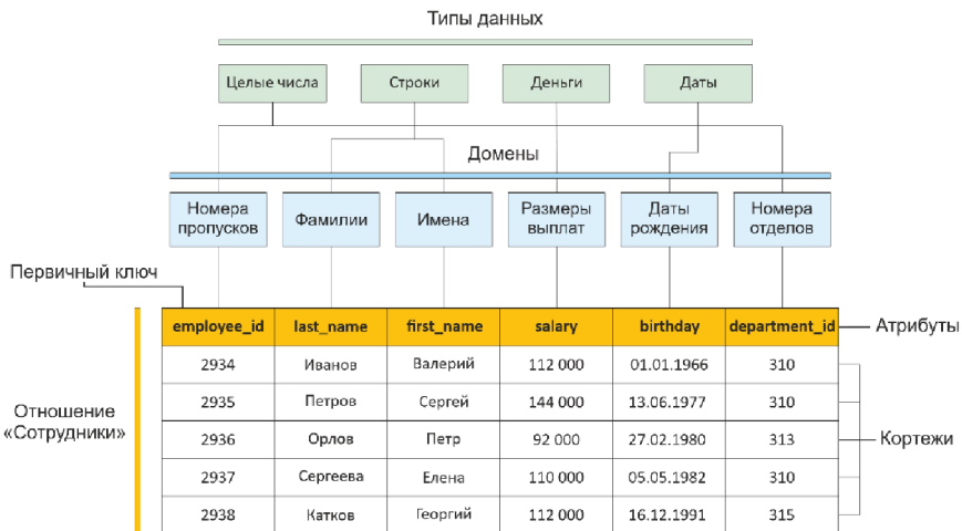
Рисунок 12 – Отношение «Сотрудники»
