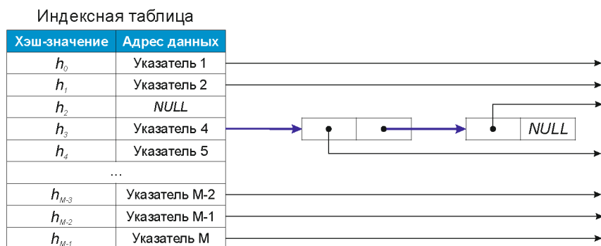
Рисунок 41 – Разрешение коллизий
