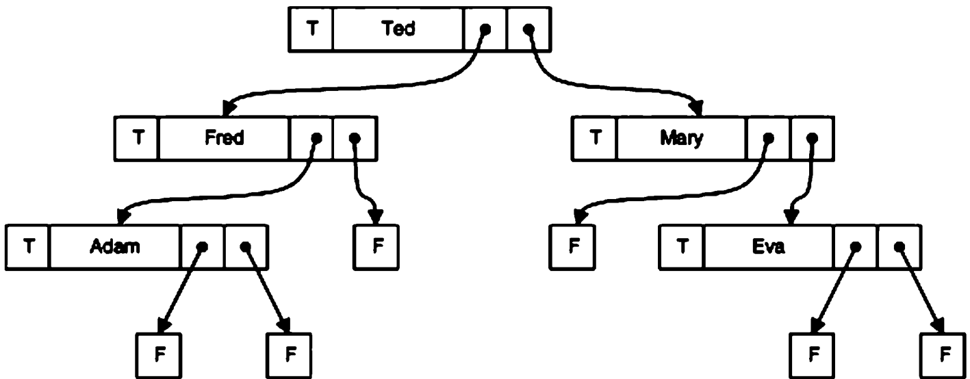
Рис. 4.3. Структура данных, связанная указателями
