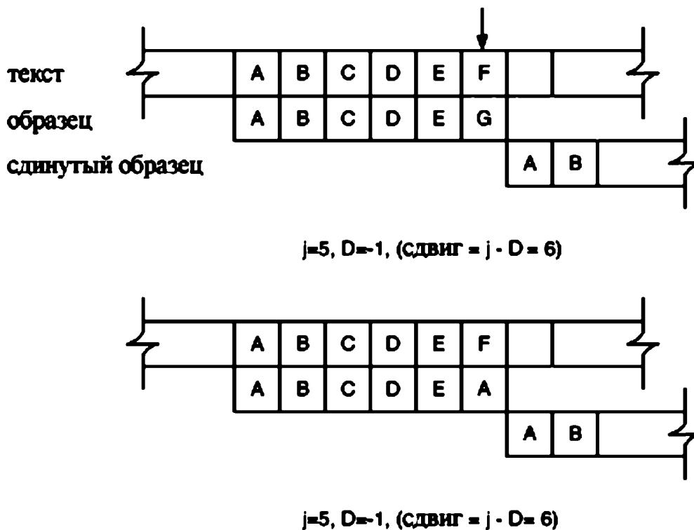
Рис. 1.13. Сдвиг образца за позицию последней литеры
