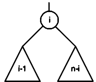
Рис. 4.29. Распределение весов по ветвям
