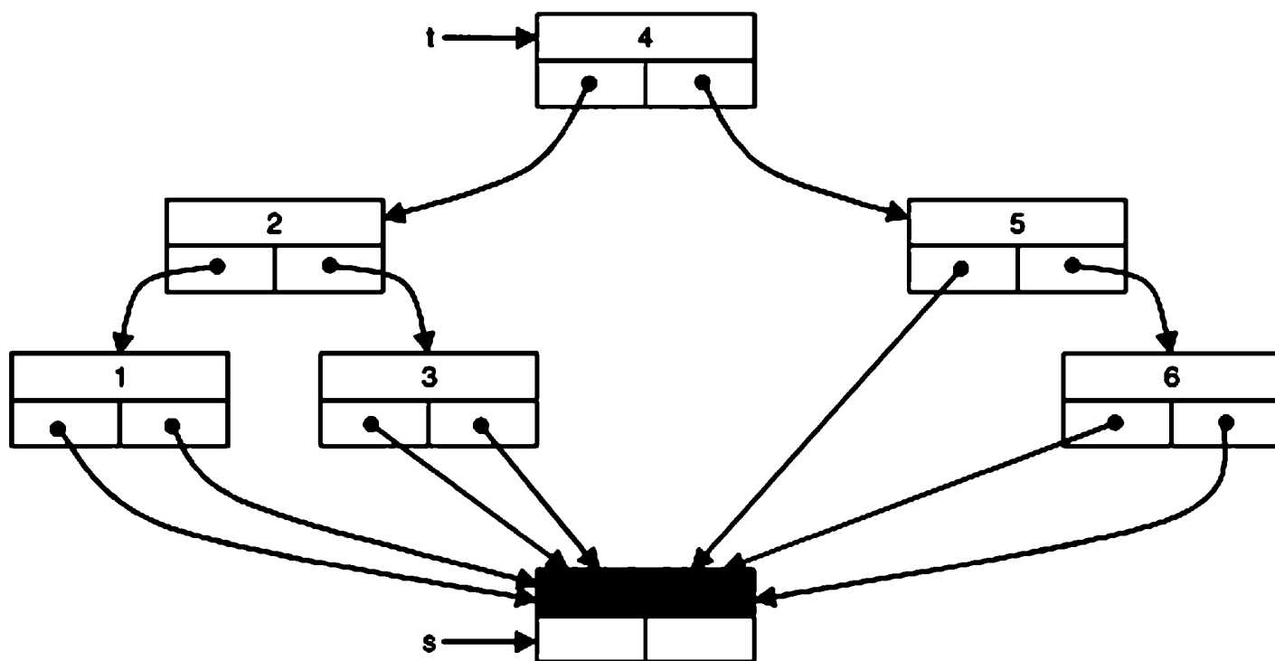
Рис. 4.25. Дерево поиска с барьером (узел s)
