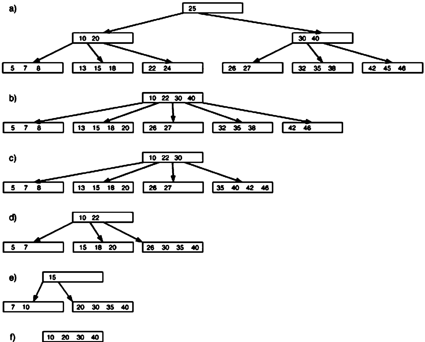
Рис. 4.46. Удаление элементов из Б-дерева порядка 2
