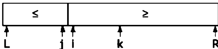
Рис. 2.9. Значение x слишком мало
