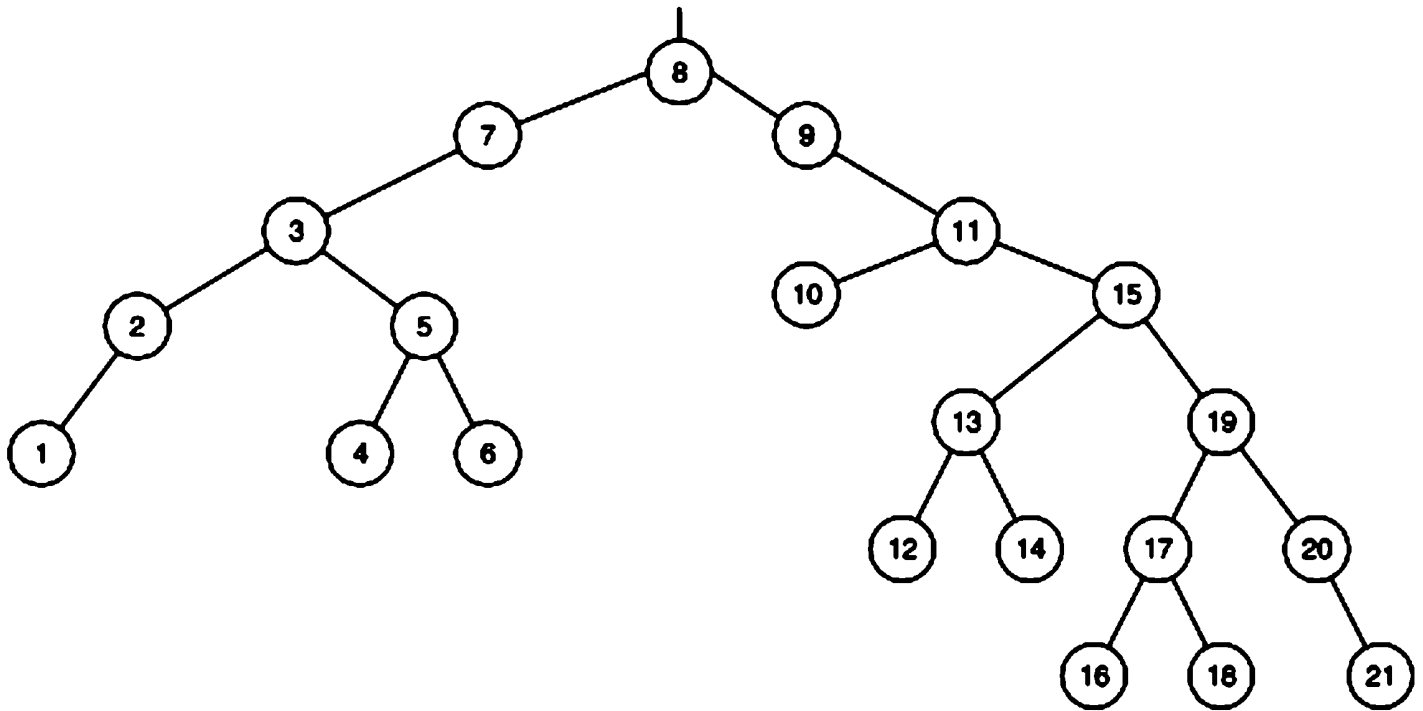
Рис. 4.27. Дерево поиска, порожденное процедурой поиска и вставки
