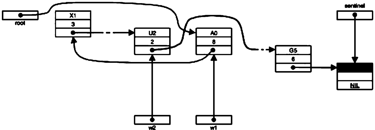
Рис. 4.12. Список после переупорядочения
