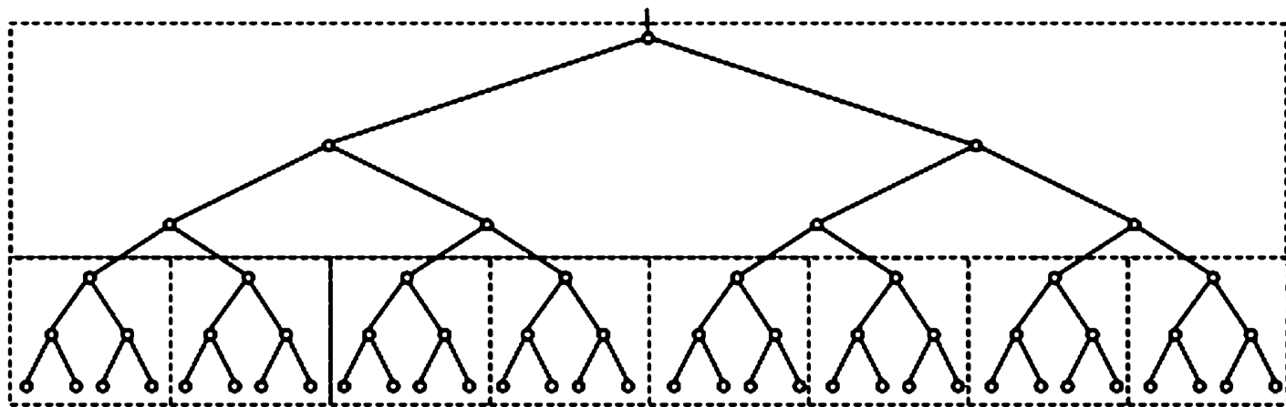
Рис. 4.41. Двоичное дерево, разделенное на страницы
