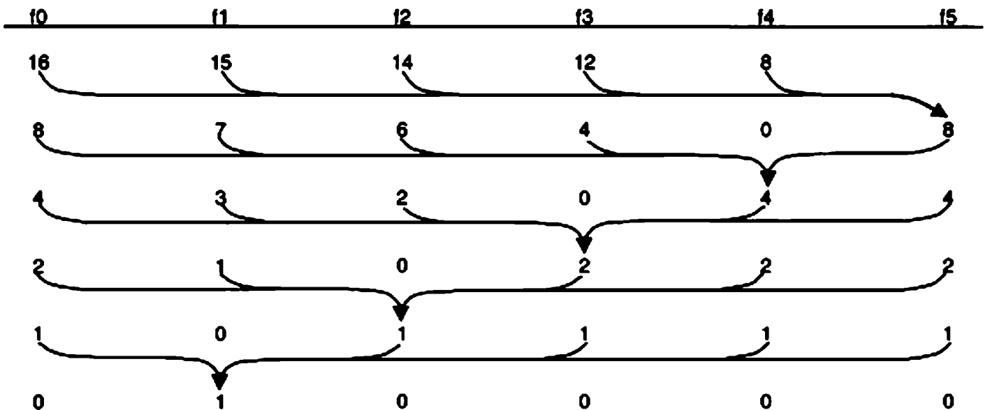
Рис. 2.15. Многофазная сортировка слиянием 65 серий с использованием 6 последовательностей
