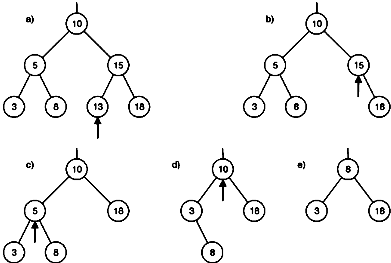
Рис. 4.28. Удаление из дерева
