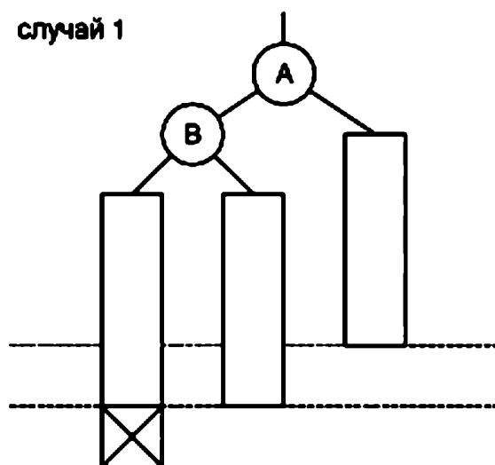
Рис. 4.32. Нарушение баланса в результате вставки
