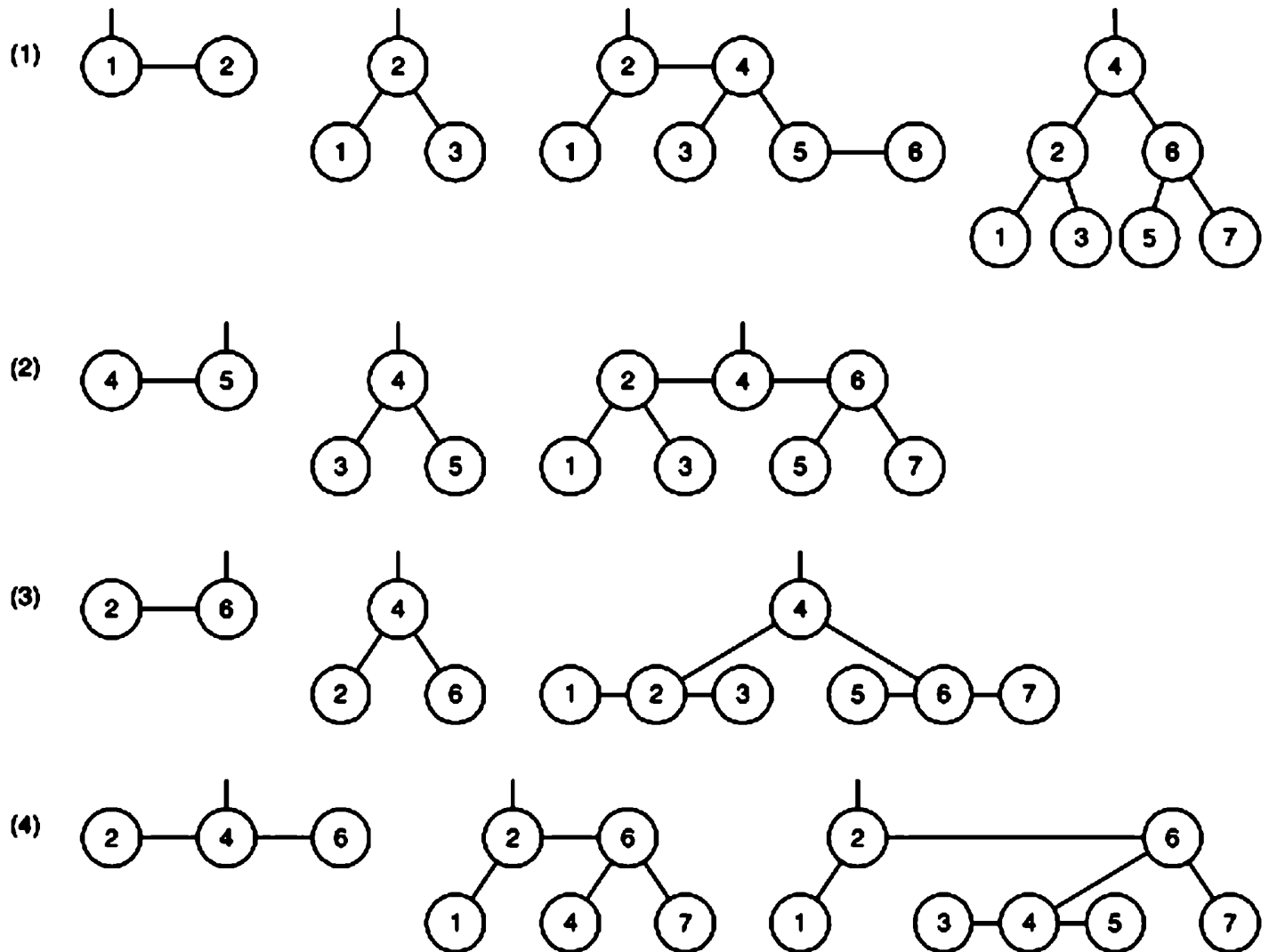
Рис. 4.50. Вставки ключей с 1 по 7
