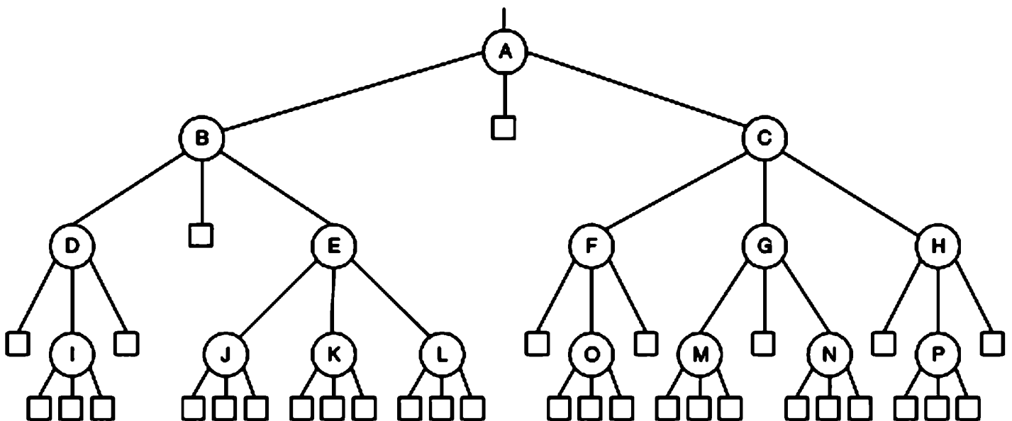
Рис. 4.19. Троичное дерево, расширенное дополнительными узлами
