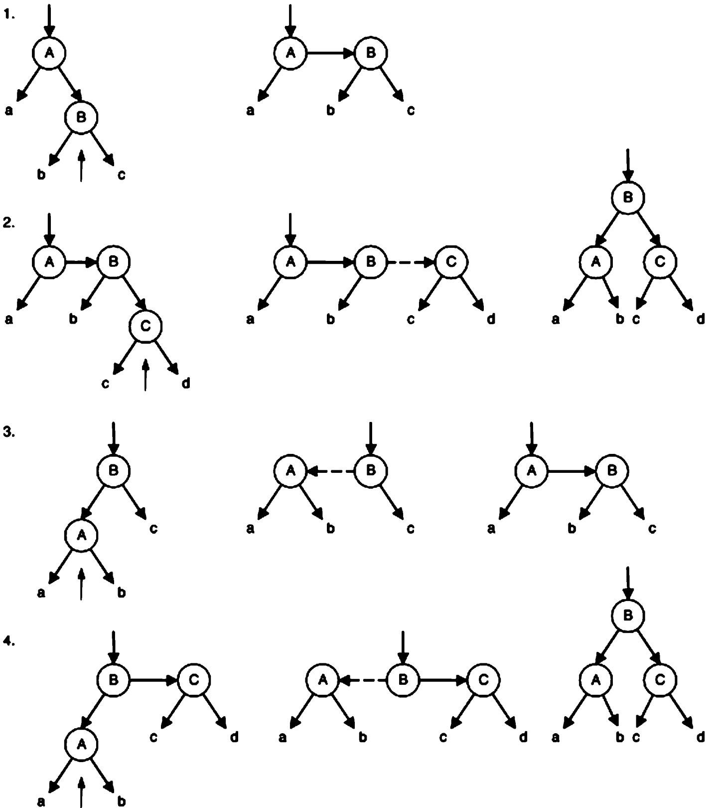
Рис. 4.48. Вставка узлов в ДБ-дереве
