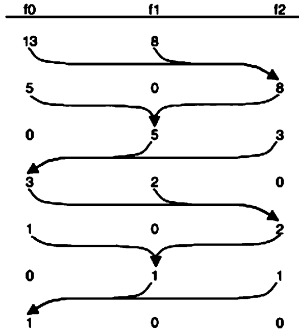
Рис. 2.14. Многофазная сортировка с тремя последовательностями, содержащими 21 серию
