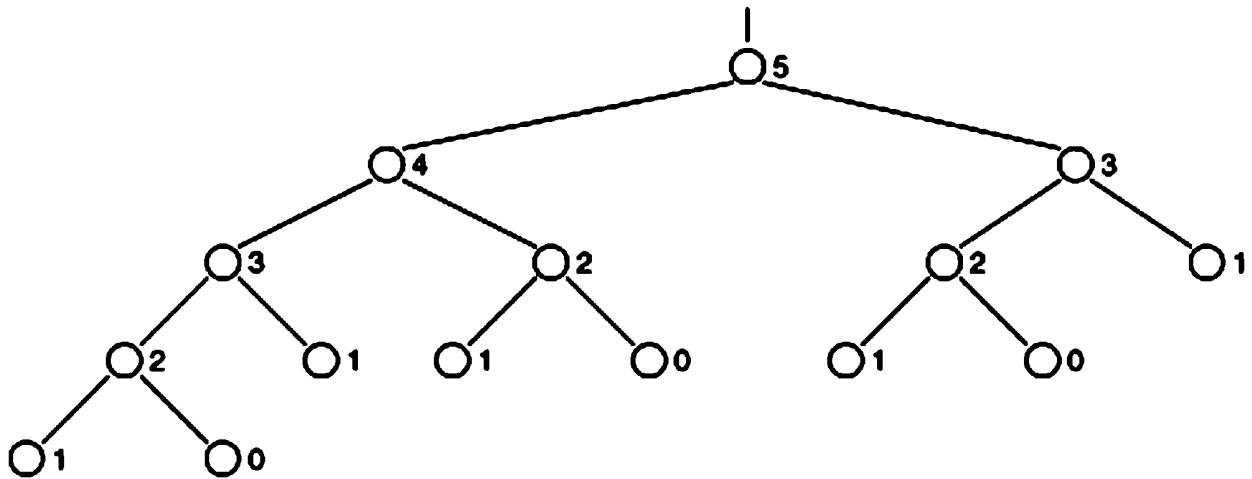
Рис. 3.2. Пятнадцать активаций при вызове \text{Fib}(5)
