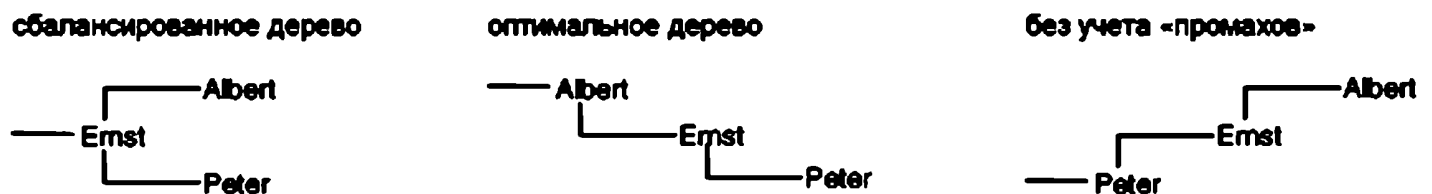
Рис. 4.39. Три дерева, построенные процедурой ComputeOptTree
