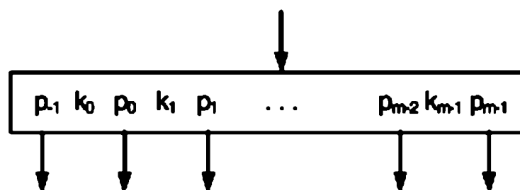
Рис. 4.43. Б-дерево с m ключами
