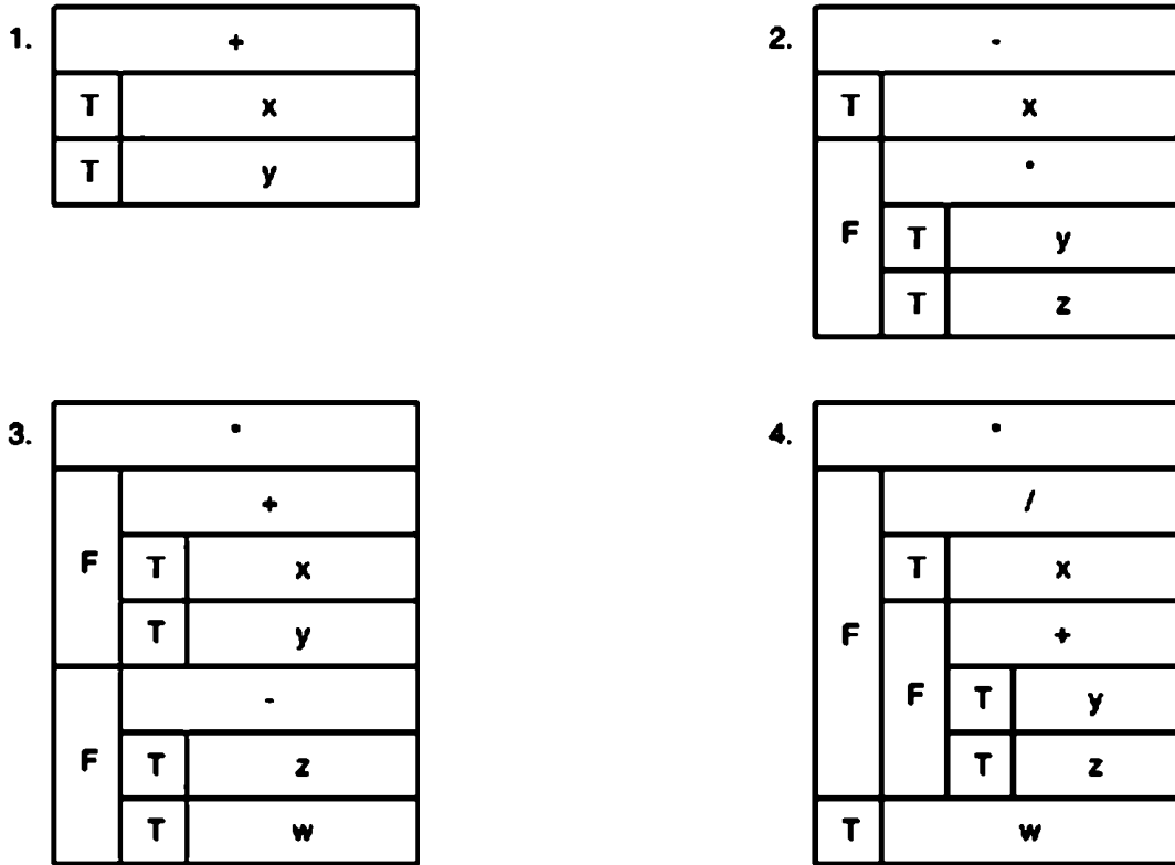
Рис. 4.1. Схемы расположения в памяти рекурсивных записевых структур
