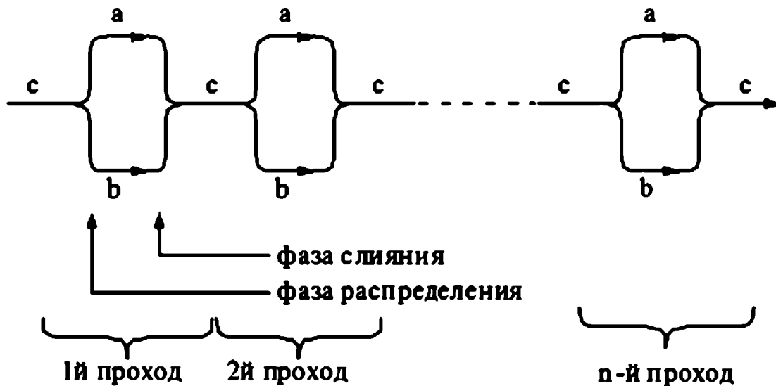
Рис. 2.13. Фазы сортировки и проходы
