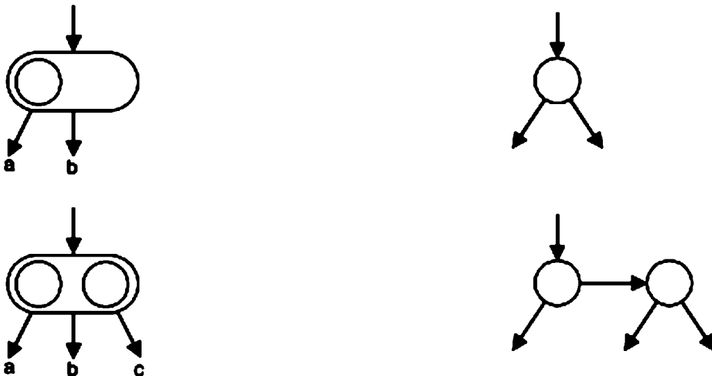
Рис. 4.47. Представление узлов ДБ-деревьев
