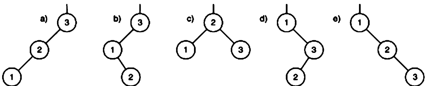
Рис. 4.36. Деревья поиска с 3 узлами
