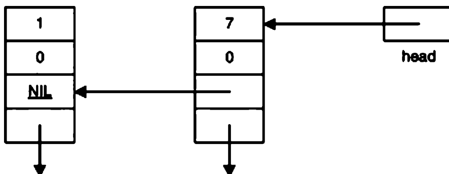
Рис. 4.16. Список ведущих с нулевым числом предшественников
