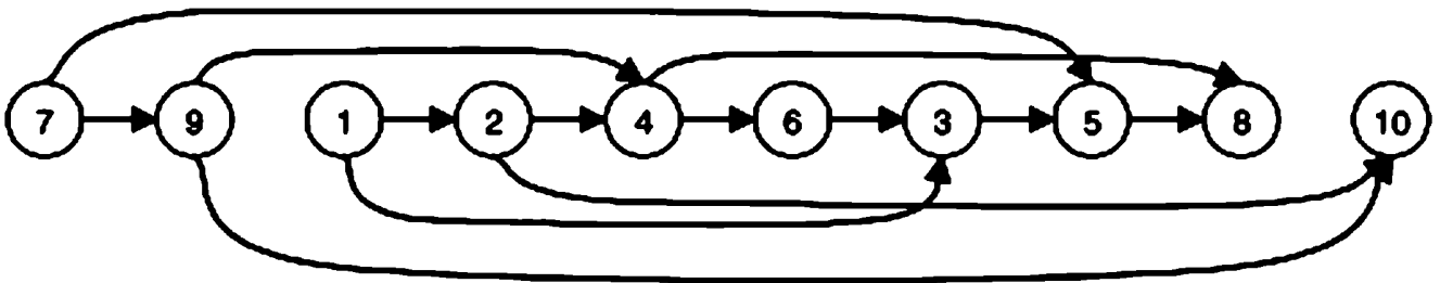
Рис. 4.14. Расположение в линию частично упорядоченного множества из рис. 4.13
