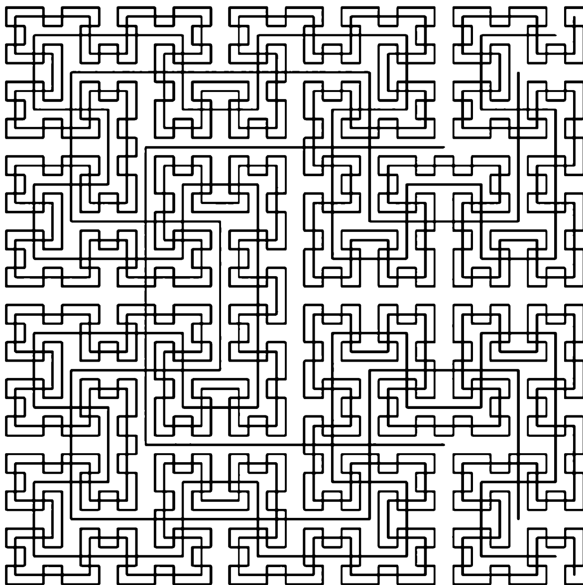
Рис. 3.4. Гильбертовы кривые H_1 \dots H_5
