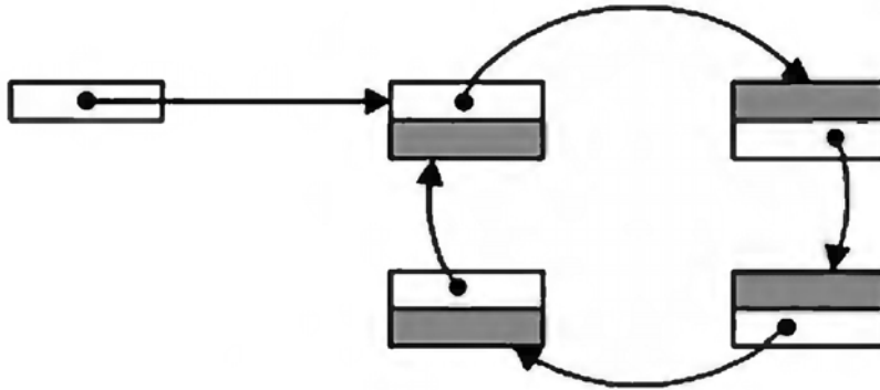
Рис. 4.52. Циклический список
