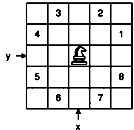
Рис. 3.7. Восемь возможных ходов коня
