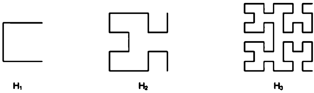
Рис. 3.3. Гильбертовы кривые порядков 1, 2 и 3
