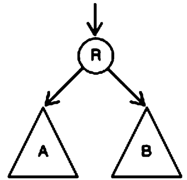
Рис. 4.24. Двоичное дерево
