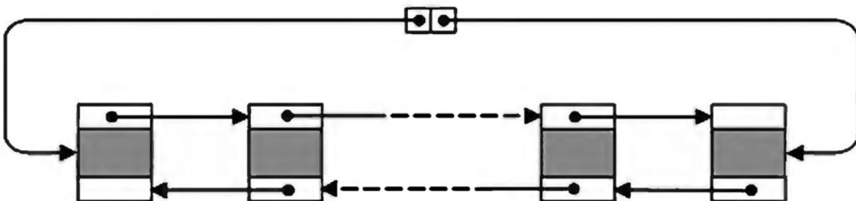
Рис. 4.53. Двухнаправленный список
