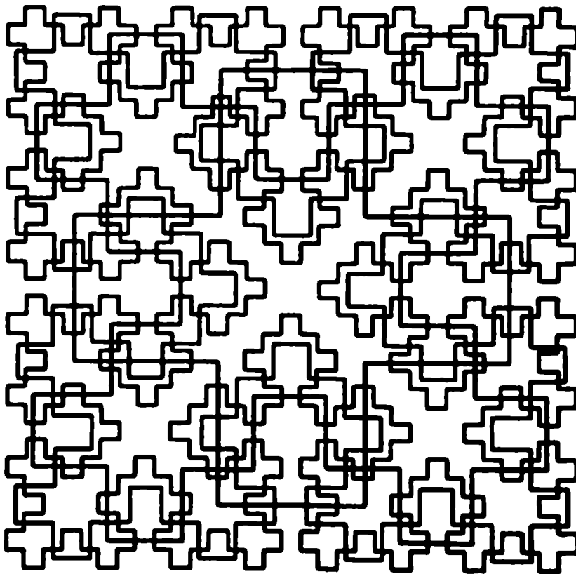
Рис. 3.10. Кривые W_1 - W_4
