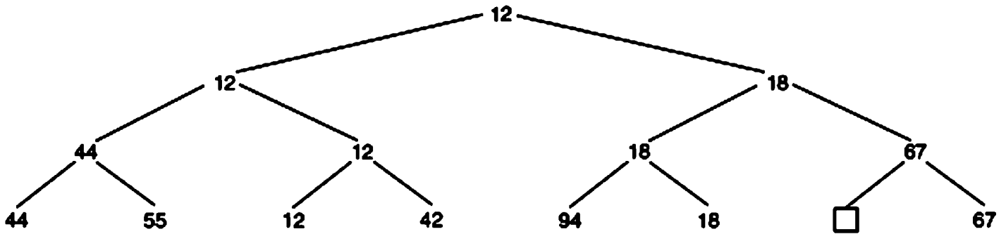
Рис. 2.5. Заполнение дырок
