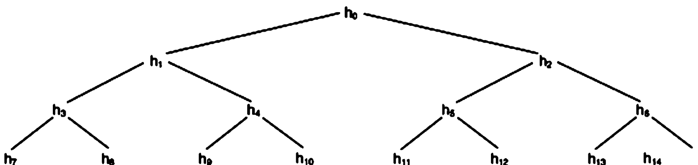
Рис. 2.6. Массив, представленный в виде двоичного дерева
