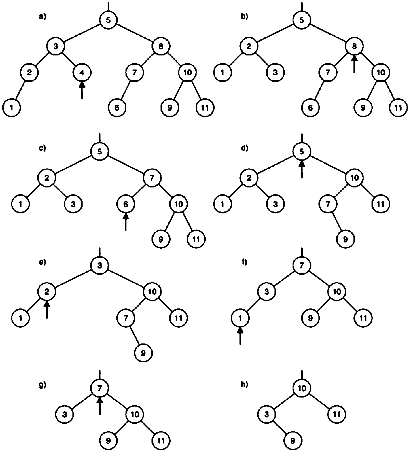
Рис. 4.35. Удаления из сбалансированного дерева
