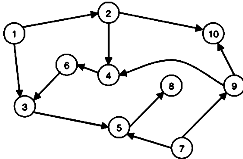
Рис. 4.13. Частично упорядоченное множество
