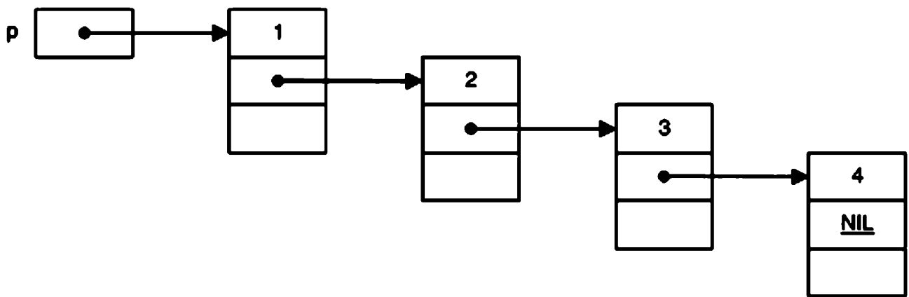
Рис. 4.6. Пример связанного списка
