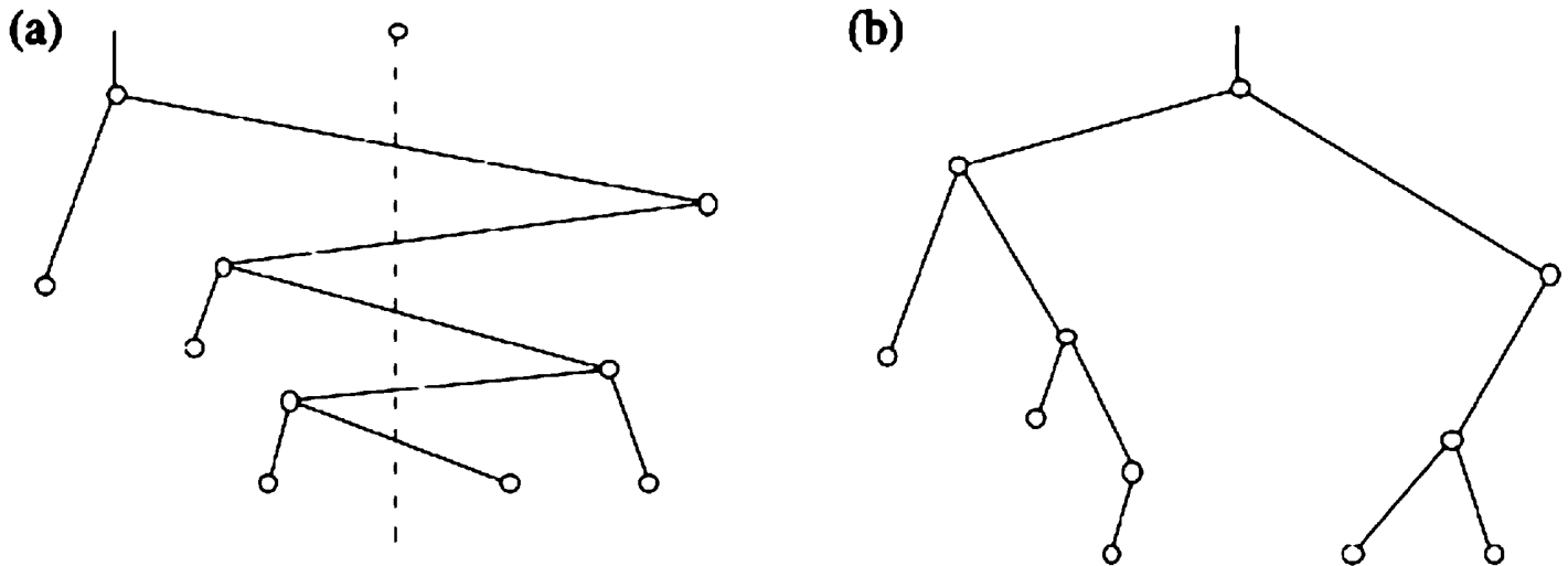
Рис. 4.51. Вставка в приоритетное дерево поиска
