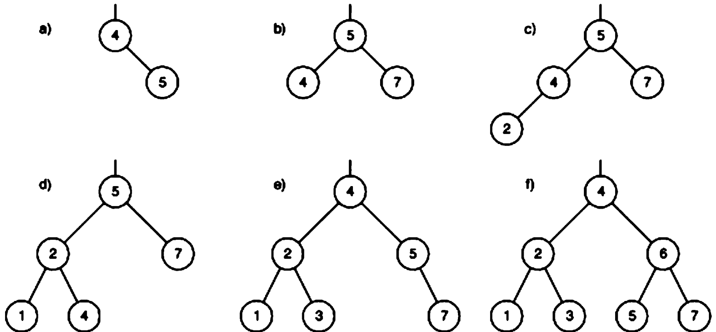
Рис. 4.34. Вставки в сбалансированное дерево
