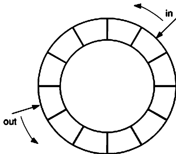
Рис. 1.8. Кольцевой буфер с индексами in и out
