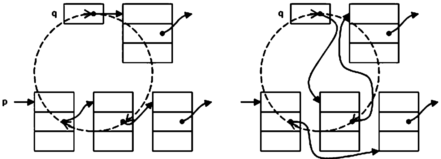
Рис. 4.9. Удаление и повторная вставка
