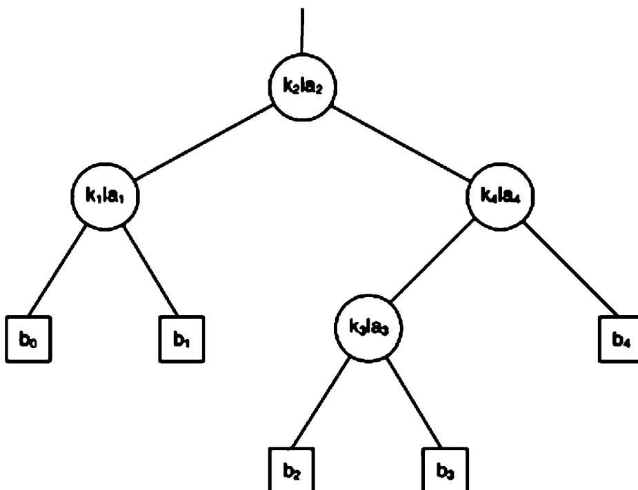
Рис. 4.37. Дерево поиска с частотами обращений
