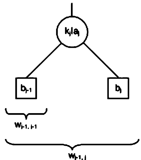
Рис. 4.38. Оптимальное дерево поиска с единственным узлом
