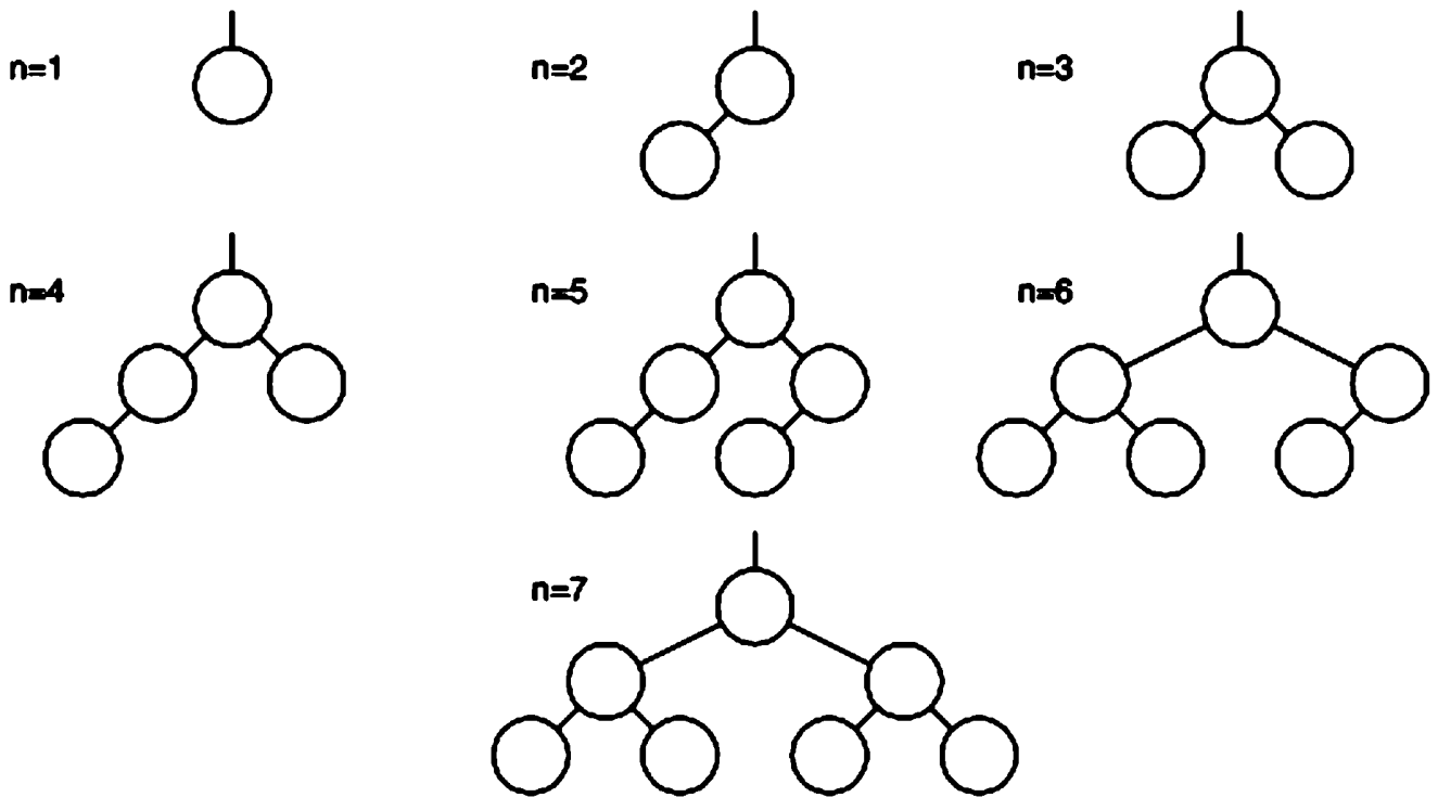
Рис. 4.22. Идеально сбалансированные деревья
