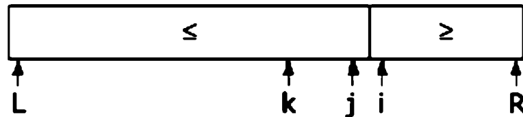
Рис. 2.10. Значение x слишком велико
