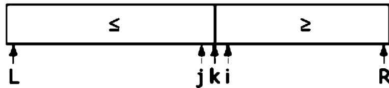
Рис. 2.11. Значение x оказалось правильным
