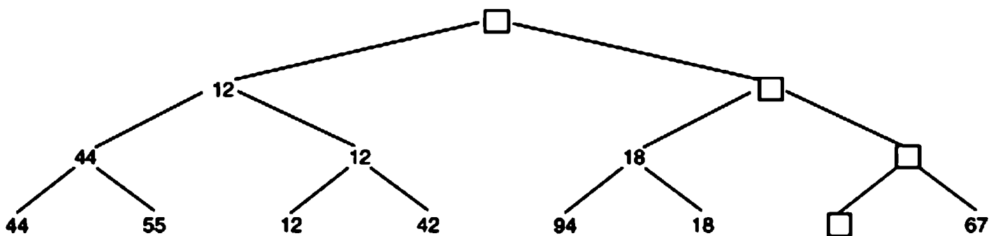
Рис. 2.4. Выбор наименьшего ключа
