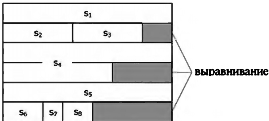
Рис. 1.7. Представление упакованной записи
