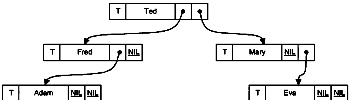
Рис. 4.5. Структура данных с указателями, имеющими значение NIL
