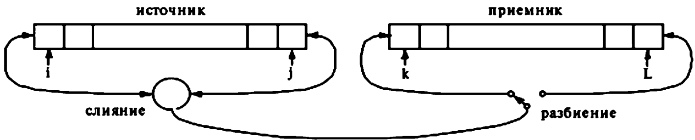
Рис. 2.12. Простая сортировка слияниями с двумя массивами
