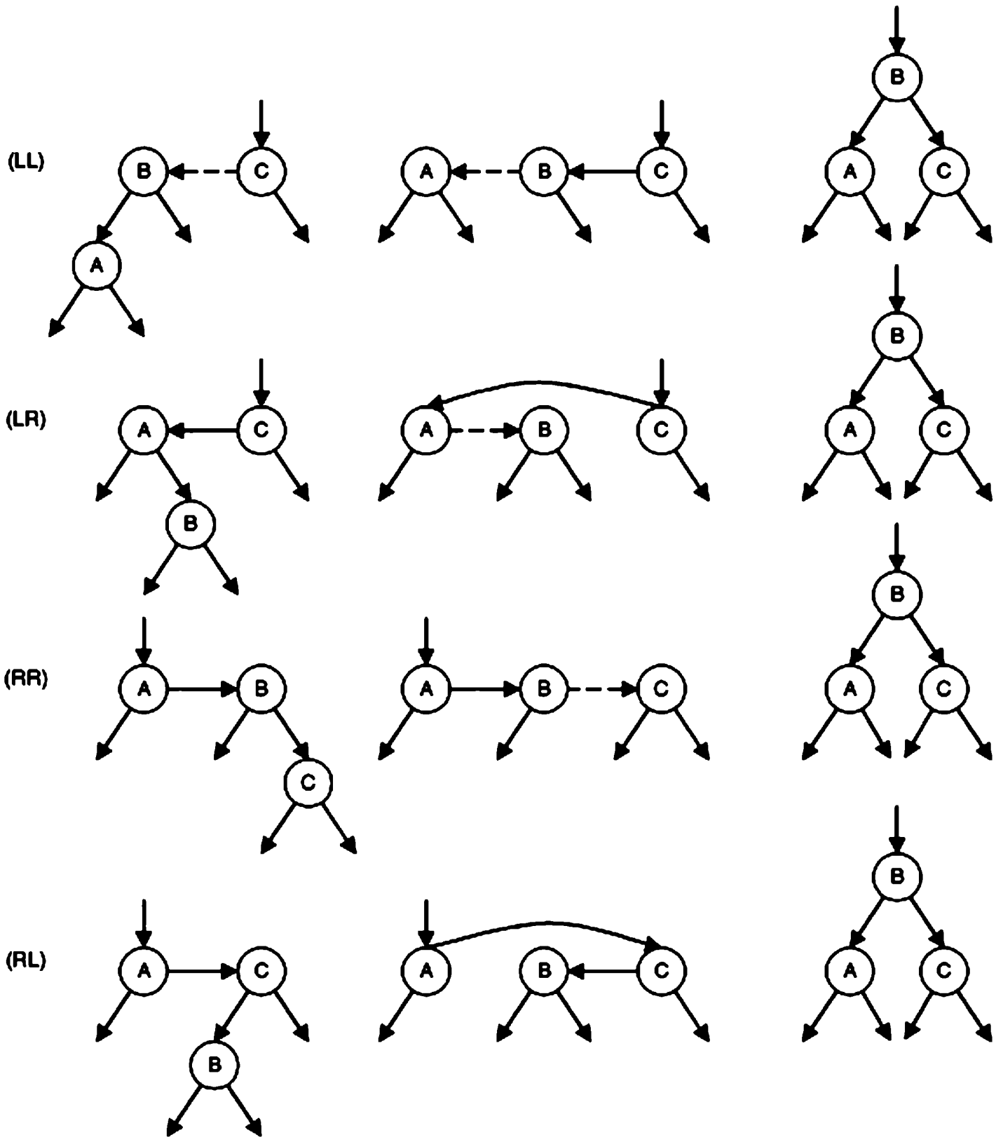
Рис. 4.49. Вставка в СДБ-деревьях
