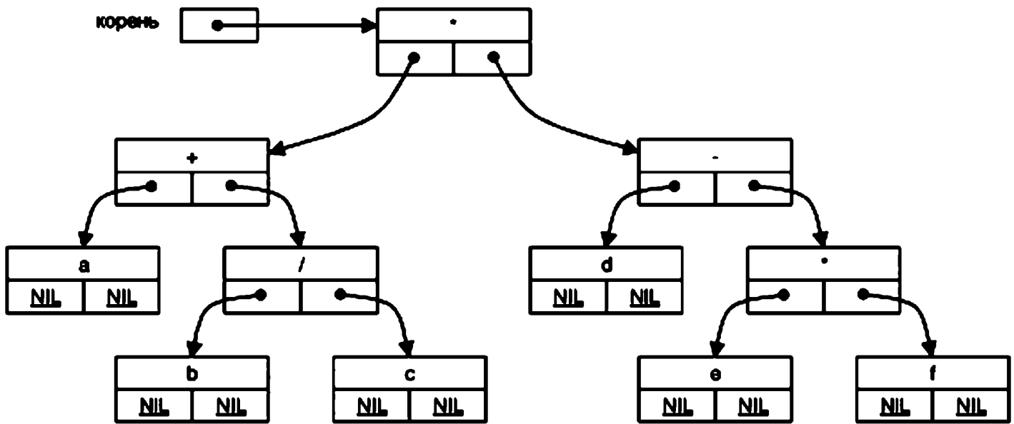
Рис. 4.21. Дерево рис. 4.20, представленное как связанная структура данных
