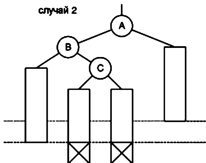
Рис. 4.32. Нарушение баланса в результате вставки
