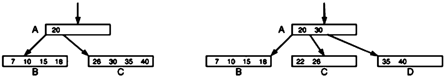
Рис. 4.44. Вставка ключа 22 в Б-дерево
