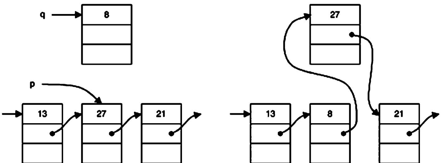
Рис. 4.8. Вставка перед p^{\wedge}
