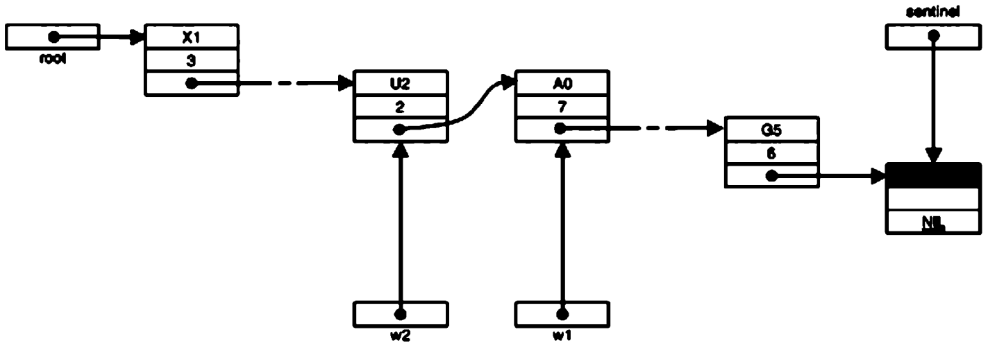
Рис. 4.11. Список до переупорядочения
