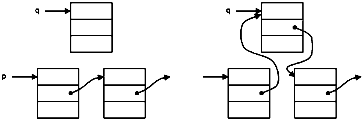
Рис. 4.7. Вставка после p^{\wedge}
