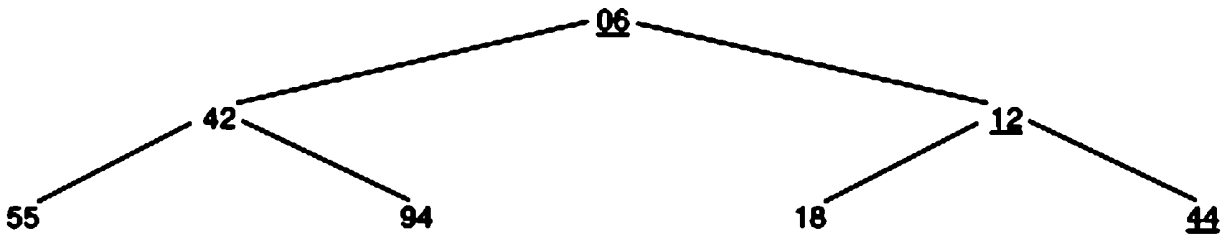
Рис. 2.8. Просеивание ключа 44 сквозь пирамиду
