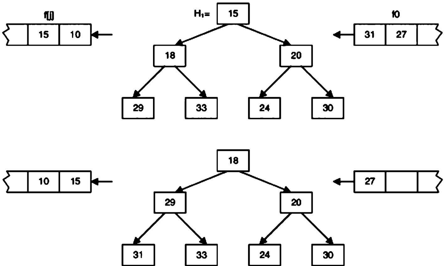
Рис. 2.17. Просеивание ключа сквозь пирамиду
