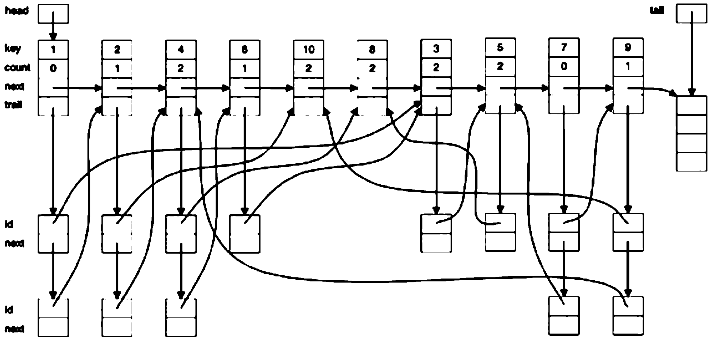
Рис. 4.15. Списковая структура, порожденная программой TopSort
