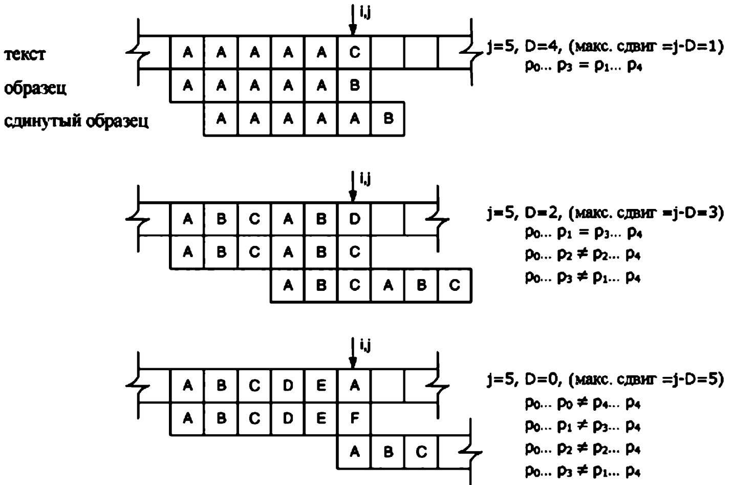
Рис. 1.12. Частичные совпадения образца и вычисление D
