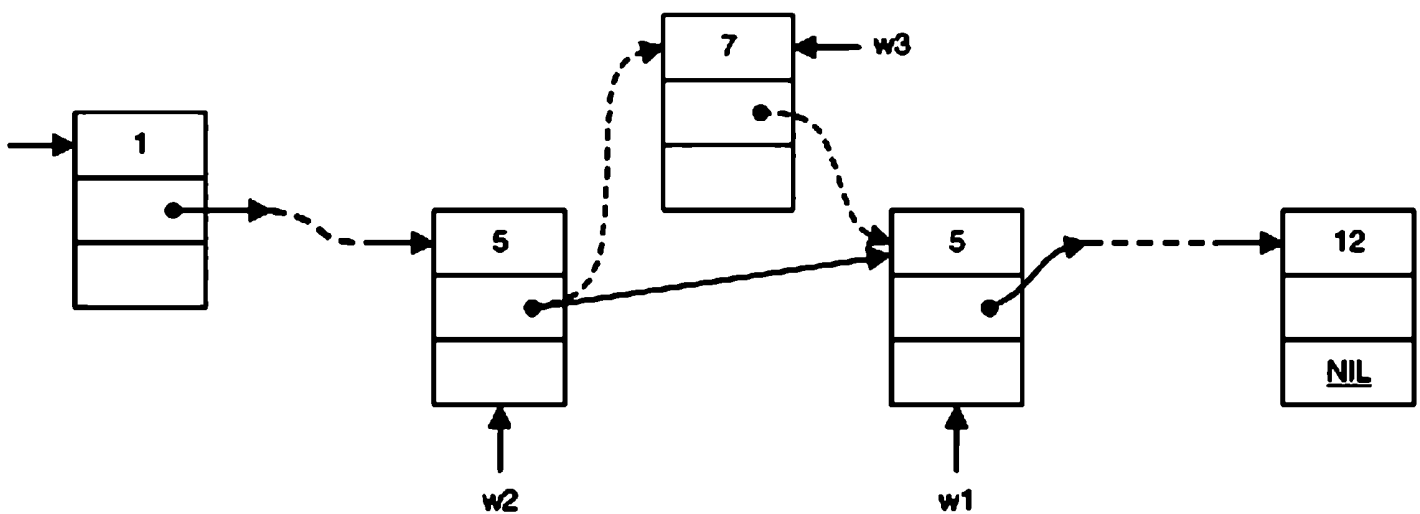
Рис. 4.10. Вставка в упорядоченный список
