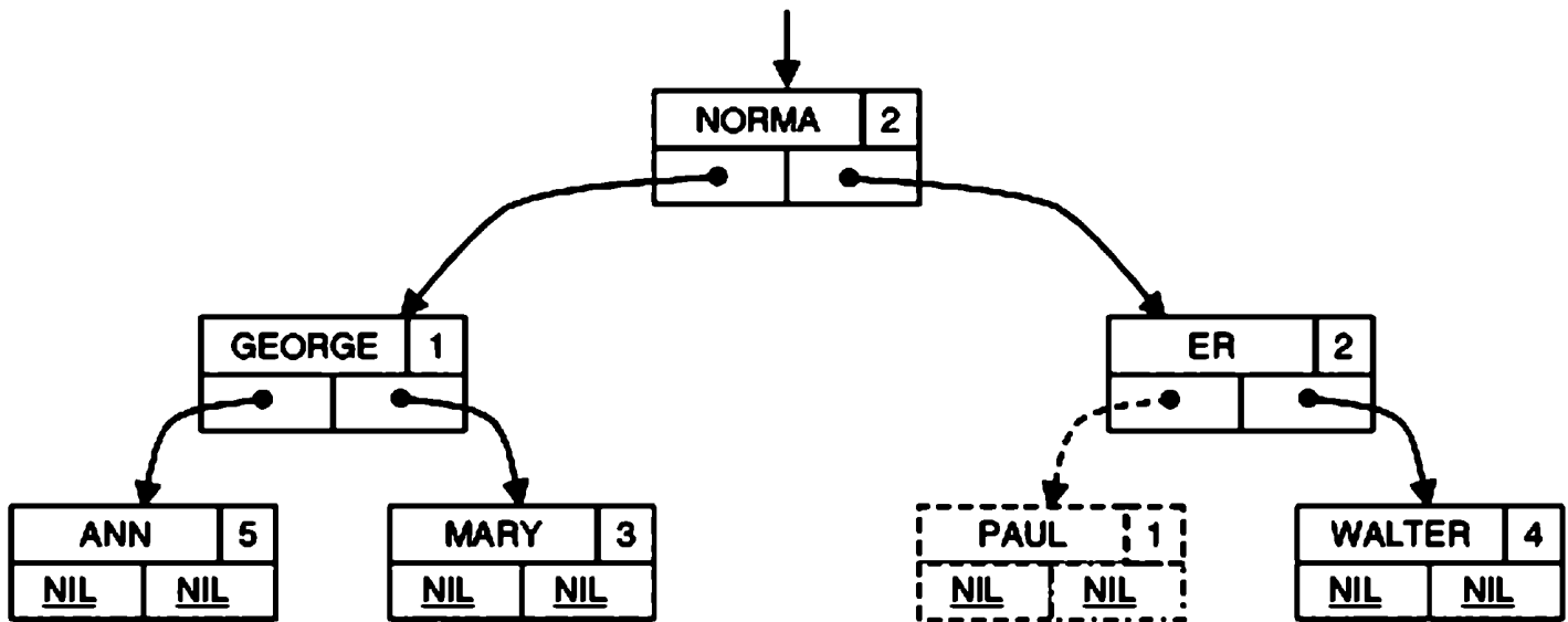
Рис. 4.26. Вставка в упорядоченное двоичное дерево
