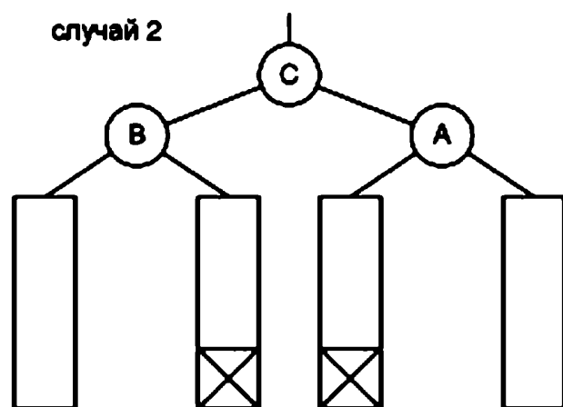
Рис. 4.33. Восстановление баланса
