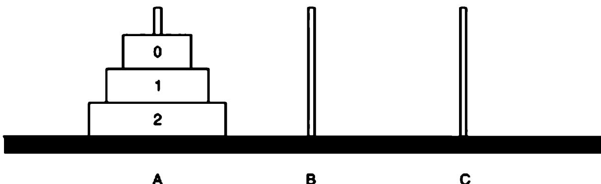
Рис. 3.9. Ханойские башни
