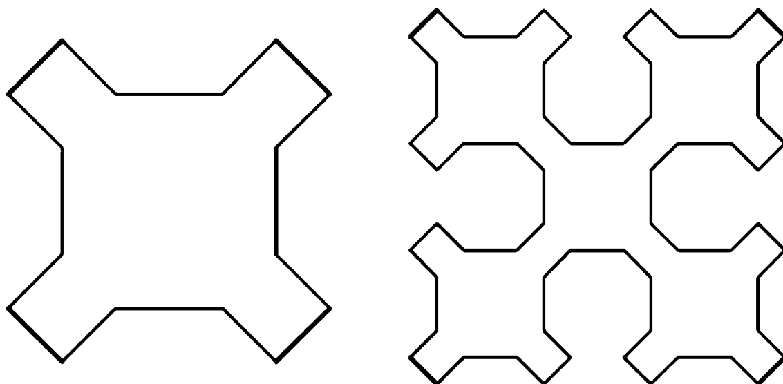
Рис. 3.5. Кривые Серпиньского S_1 и S_2
