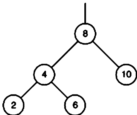
Рис. 4.31. Сбалансированное дерево
