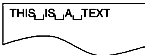
Рис. 1.1. Представление текста
