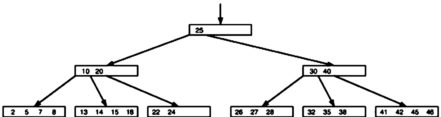
Рис. 4.42. Б-дерево порядка 2
