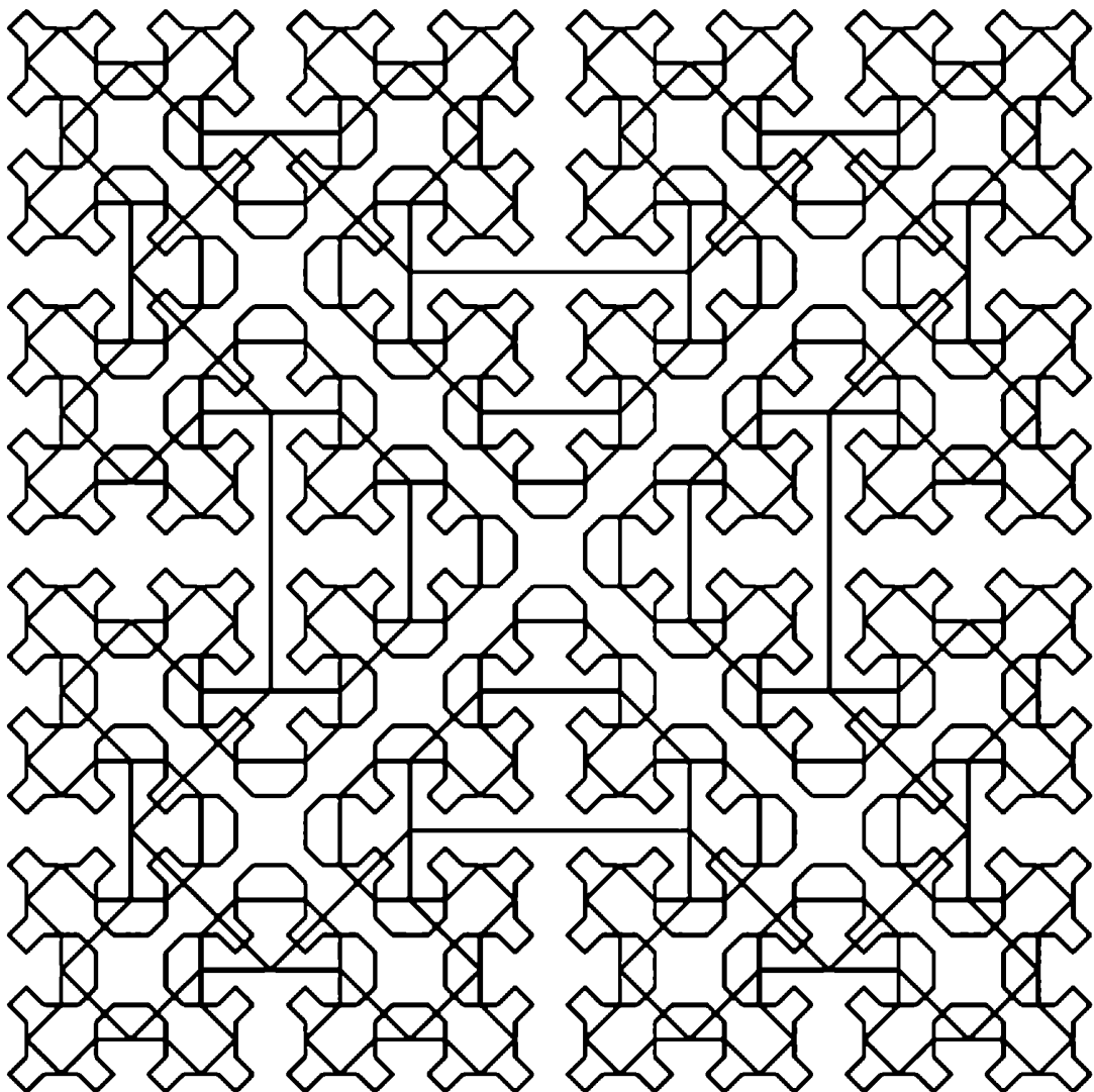
Рис. 3.6. Кривые Серпиньского S_1, \dots, S_4
