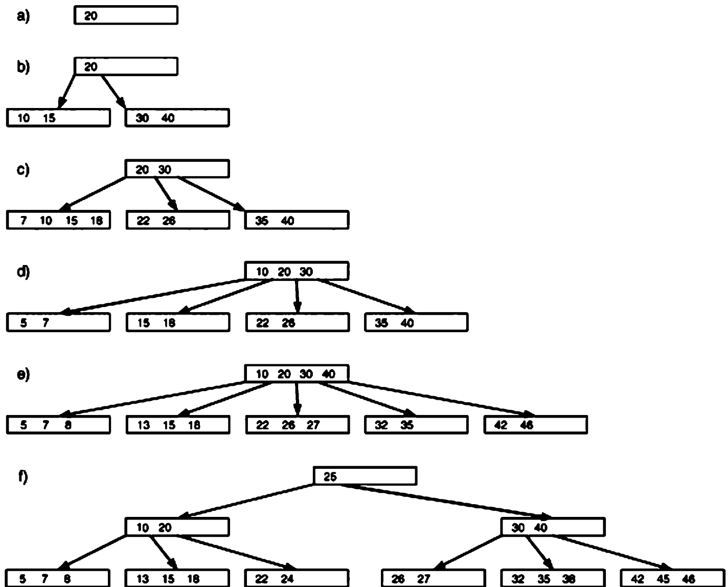
Рис. 4.45. Рост Б-дерева порядка 2
