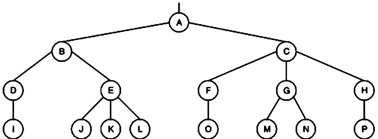
Рис. 4.17. Представление дерева посредством (a) вложенных подмножеств, (b) скобочного выражения, (c) текста с отступами, (d) графа
