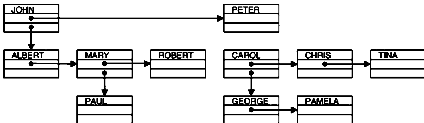
Рис. 4.40. Сильно ветвящееся дерево, представленное как двоичное дерево
