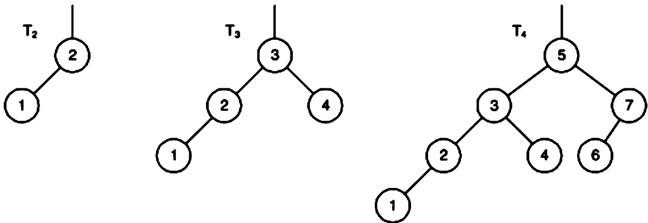
Рис. 4.30. Деревья Фибоначчи высоты 2, 3 и 4
