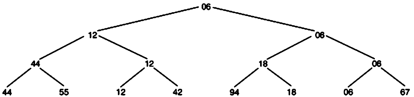
Рис. 2.3. Повторные выборы среди двух ключей («турнир ключей»)
