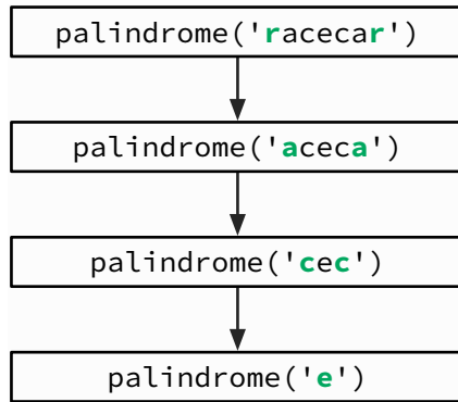
Рис. 3.4. Рекурсивная проверка, является ли слово гасекар палиндромом
