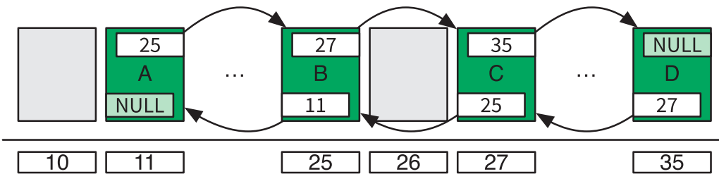
Рис. 4.4. Двусвязный список в памяти компьютера
