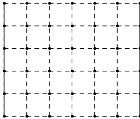
Рис. 11.2. Игра Гейла.
