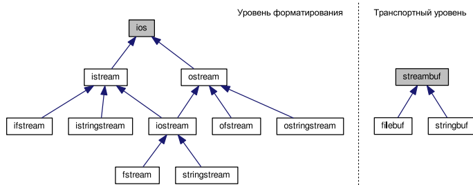
Рис. 10.4: Иерархия классов потокового ввода-вывода
