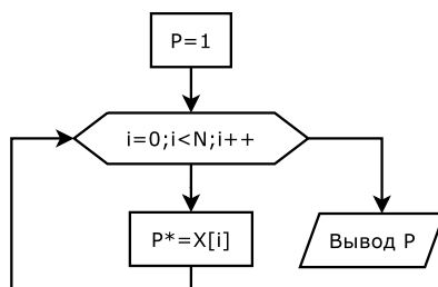
Рис. 5.5: Вычисление произведения элементов массива
