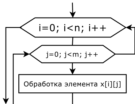
Рис. 6.1: Блок-схема построчной обработки матрицы
