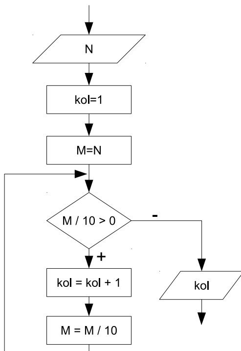
Рис. 3.30: Алгоритм определения количества цифр в числе.
