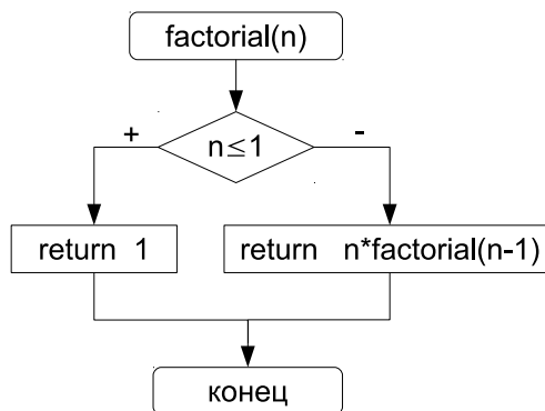
Рис. 4.10: Рекурсивный алгоритм вычисления факториала
