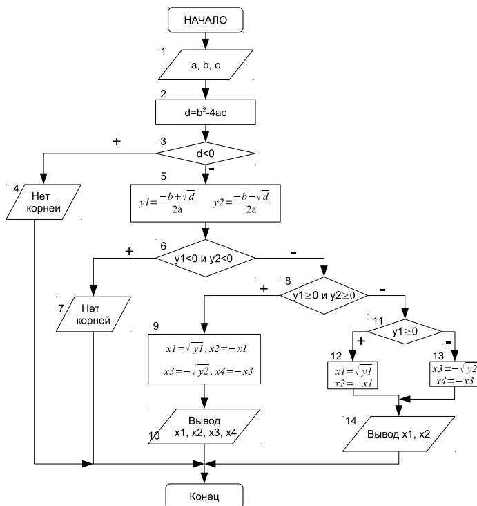
Рис. 3.18: Алгоритм решения биквадратного уравнения
