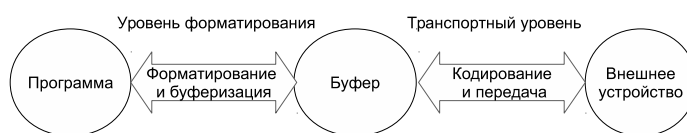
Рис. 10.3: Модель потокового ввода-вывода в C++
