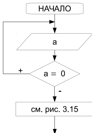
Рис. 3.24: Блок-схема проверки ввода данных
