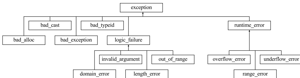
Рис. 10.5: Предопределённые индикаторы исключений
