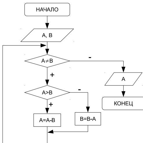
Рис. 3.25: Поиск наибольшего общего делителя двух чисел.
