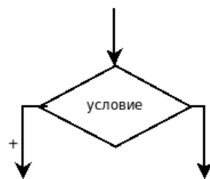
Рис. 3.4: Условный блок
