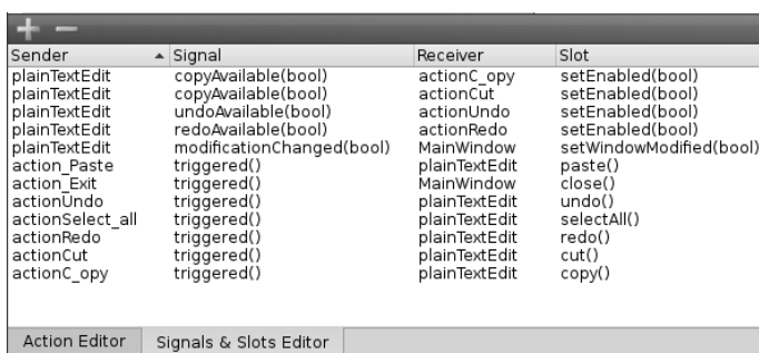
Рис. 15.7: Вид редактора сигналов и слотов (Signals & Slots Editor) после редактирования
