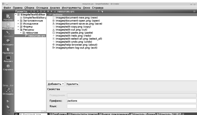
Рис. 15.8: Редактирование файла ресурсов
