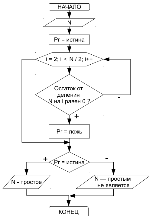
Рис. 3.29: Алгоритм определения простого числа.
