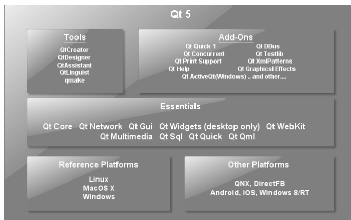
Рис. 11.1: Состав Qt5
