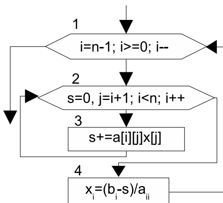
Рис. 6.13: Блок-схема алгоритма обратного хода метода Гаусса
