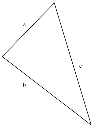
Рис. 1.7: Треугольник
