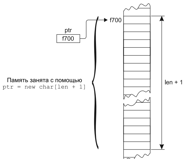
Рис. 10.14. Память, выделенная с помощью операции new
