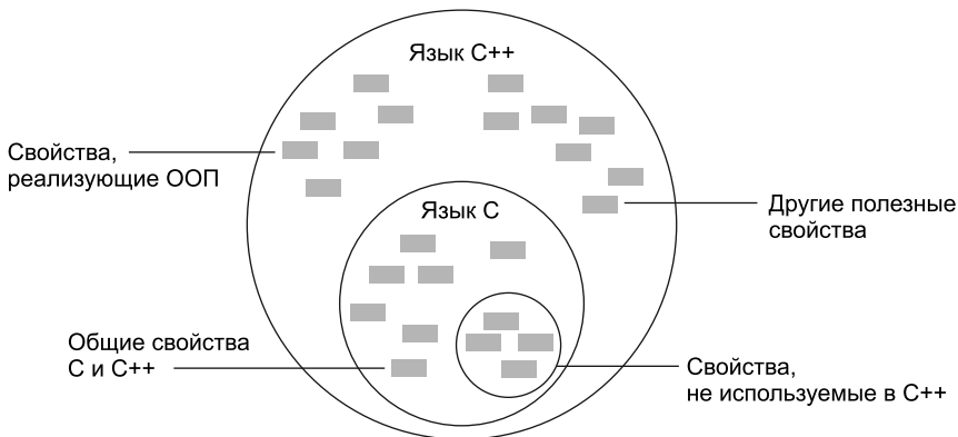
Рис. 1.7. Отношения между C и C++
