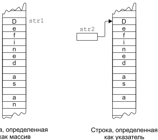
Рис. 10.10. Строки как массив и как указатель
