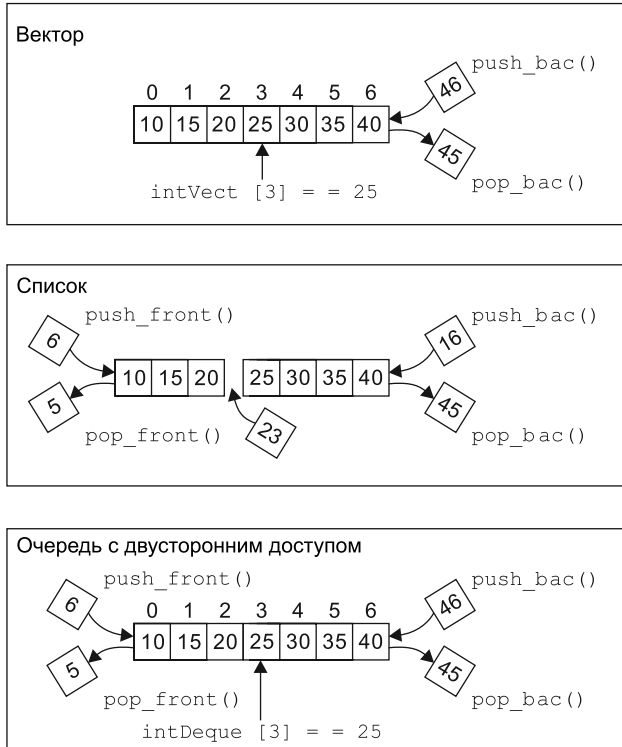
Рис. 15.2. Последовательные контейнеры
