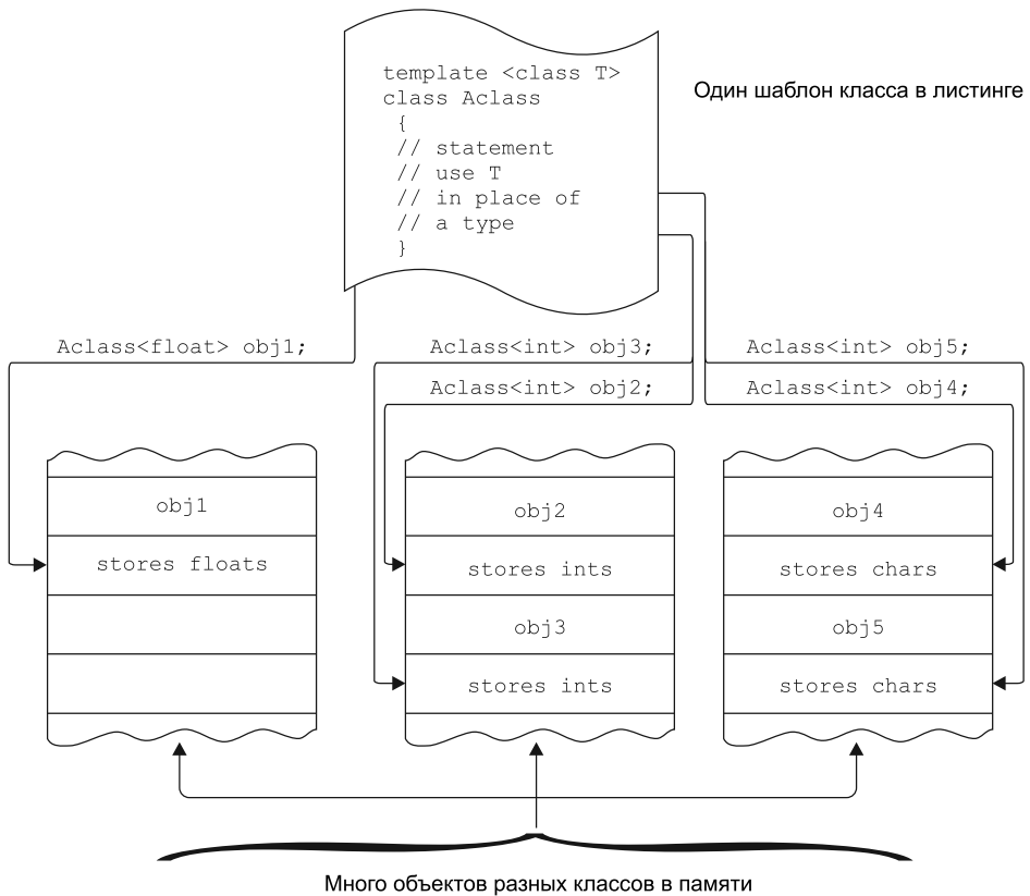
Рис. 14.2. Шаблон класса
