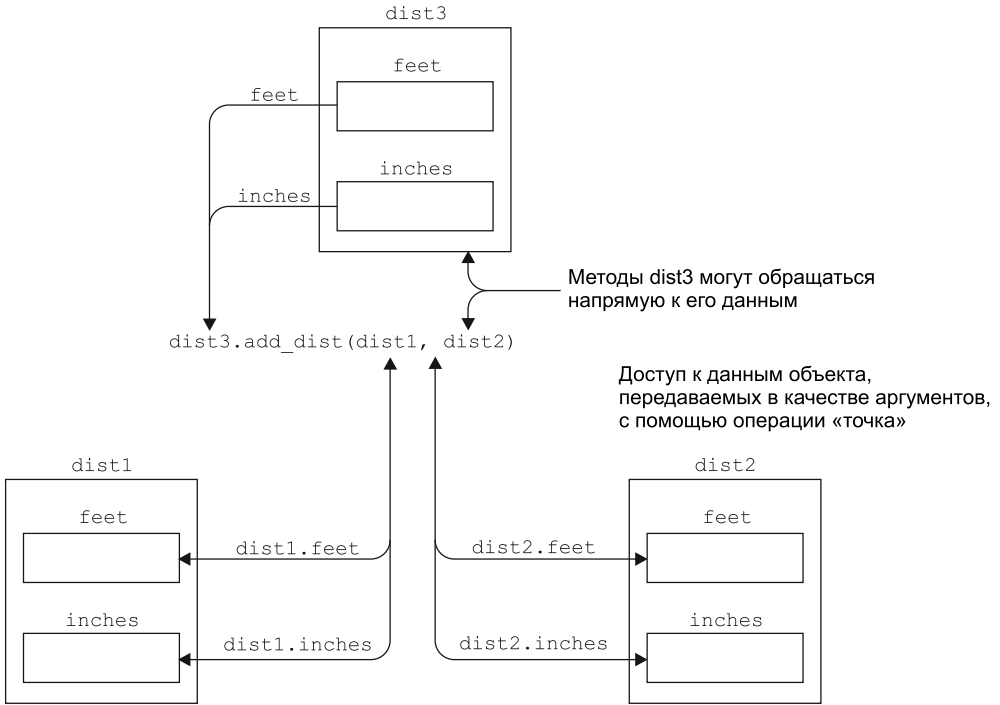
Рис. 6.6. Результат
