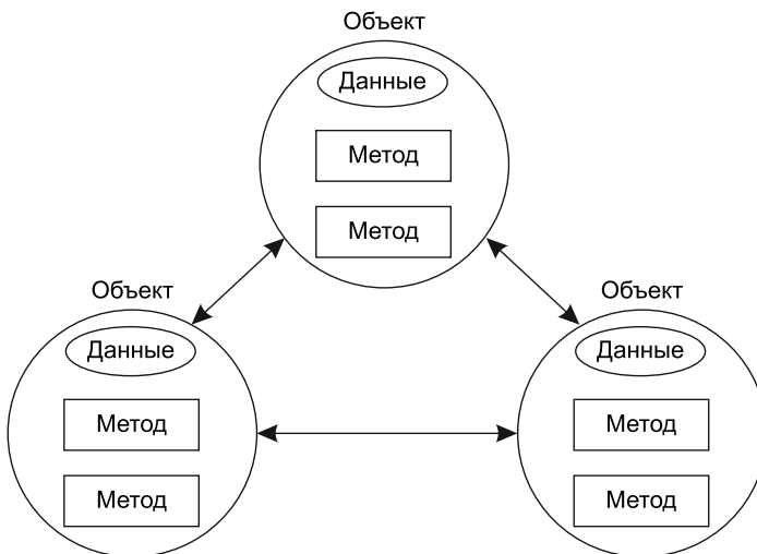
Рис. 1.3. Объектно-ориентированный подход
