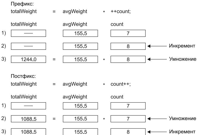
Рис. 2.11. Операция инкремента
