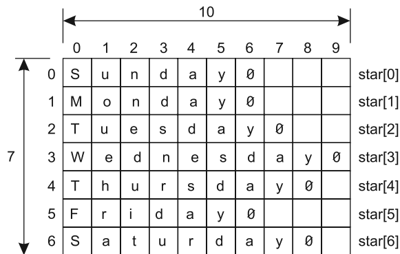
Рис. 7.10. Массив строк
