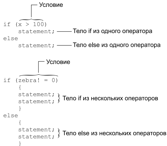
Рис. 3.9. Синтаксис if...else
