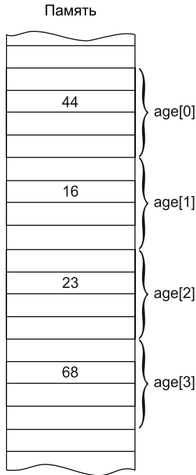
Рис. 7.2. Элементы массива
