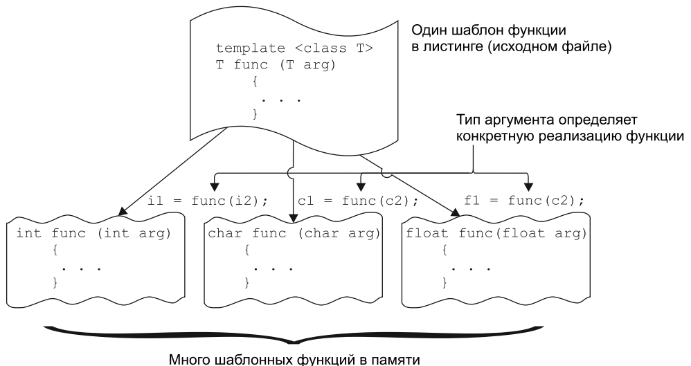
Рис. 14.1. Шаблон функции
