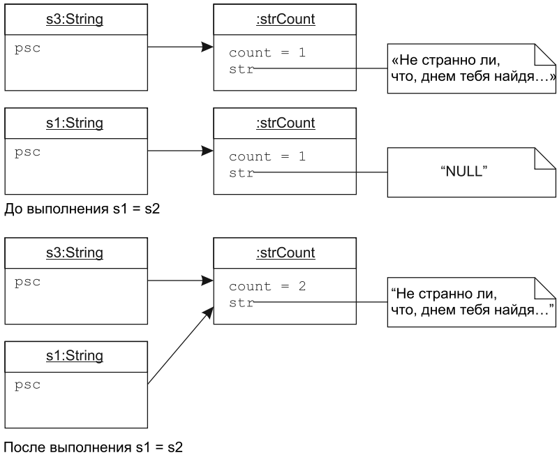
Рис. 11.7. Оператор присваивания в STRIMEM
