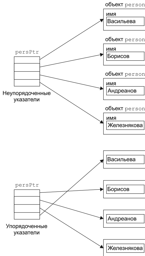
Рис. 10.17. Сортировка массива указателей
