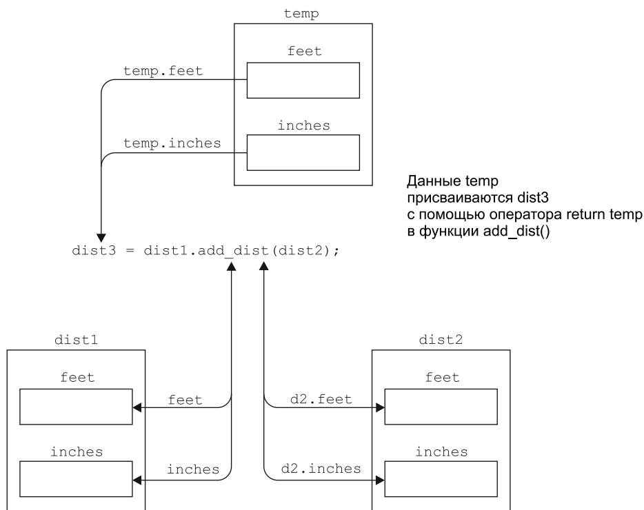
Рис. 6.7. Результат, возвращаемый из временного объекта
