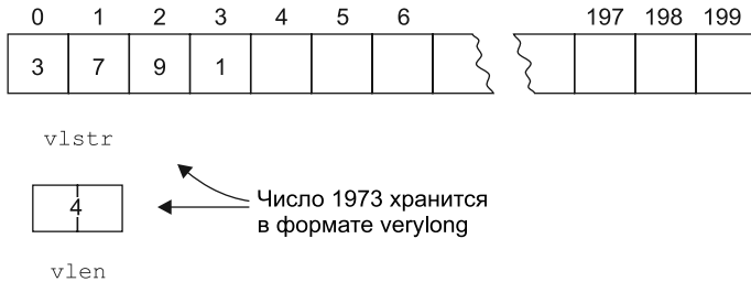
Рис. 13.2. Число типа verylong
