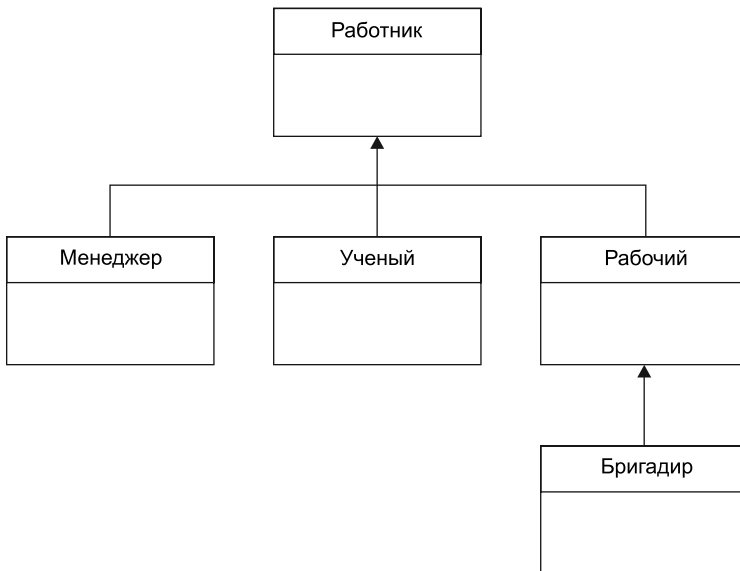
Рис. 9.8. UML диаграмма классов программы EMPLOY2
