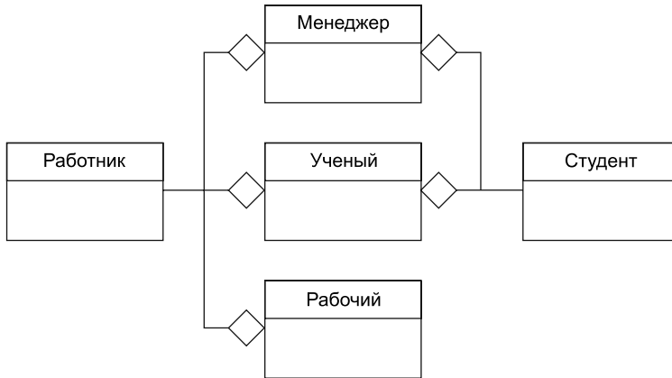
Рис. 9.12. Диаграмма классов UML для программы EMPCONT
