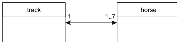
Рис. 10.20. UML-диаграмма классов программы HORSE
