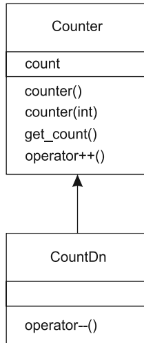
Рис. 9.2. Диаграмма классов UML для примера COUNTEN
