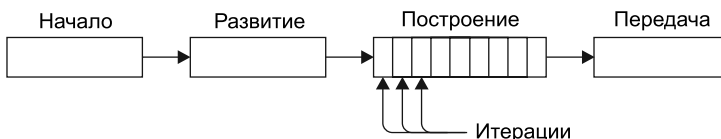
Рис. 16.2. Унифицированный процесс
