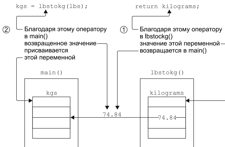
Рис. 5.6. Возврат значения
