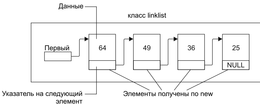
Рис. 10.15. Связный список
