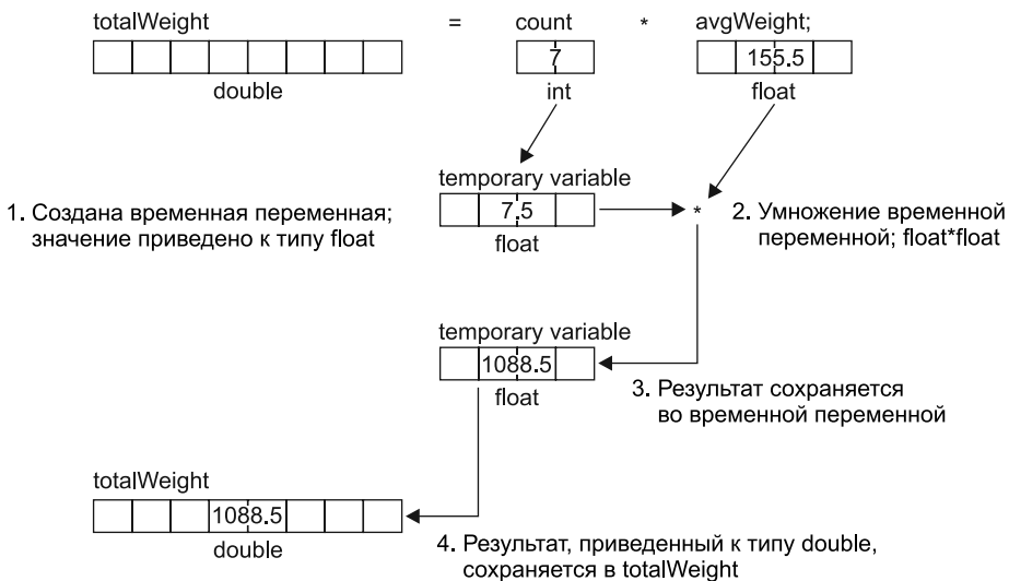
Рис. 2.9. Преобразования типов
