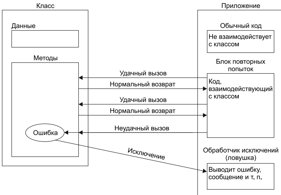
Рис. 14.4. Механизм исключений
