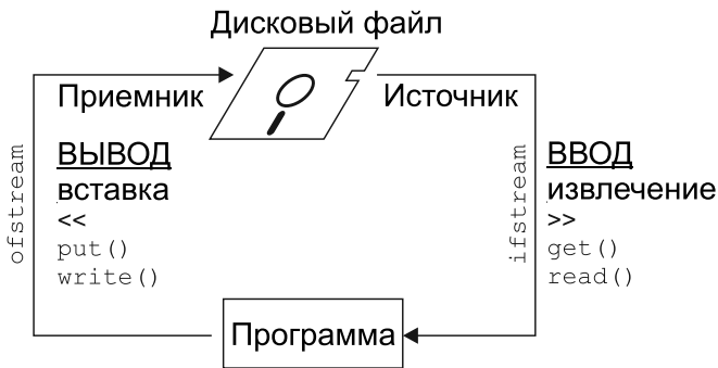
Рис. 12.2. Файловый ввод/вывод
