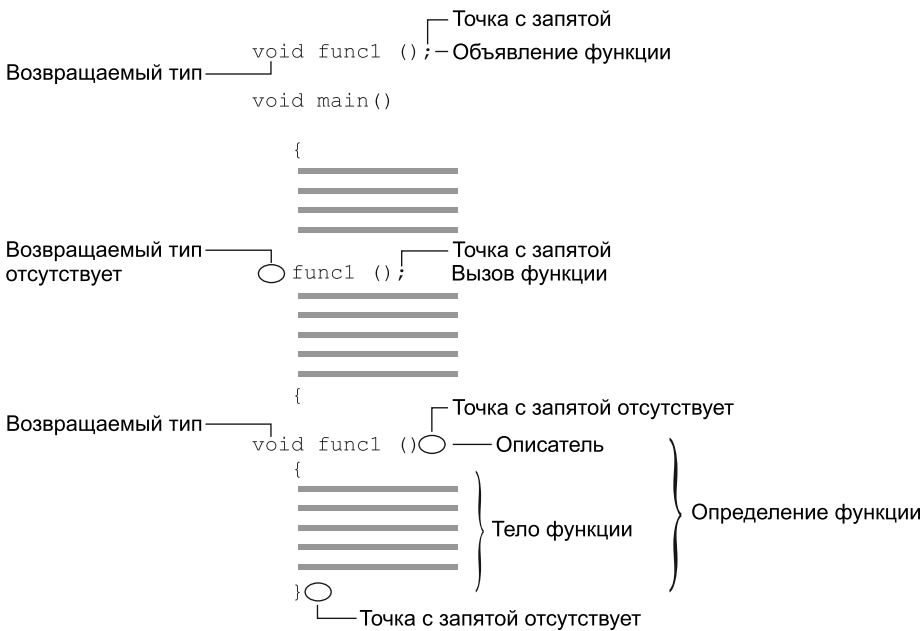
Рис. 5.2. Синтаксис функции
