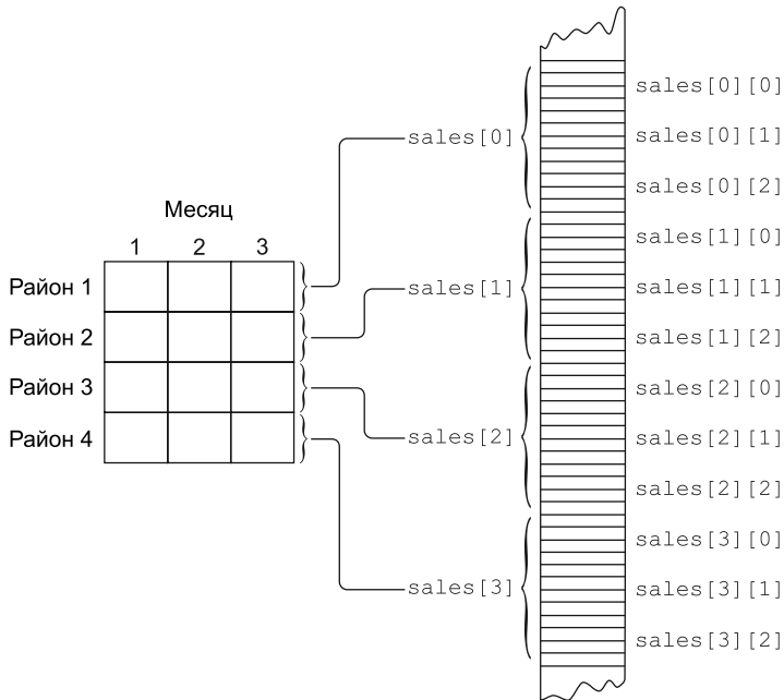
Рис. 7.4. Двумерный массив
