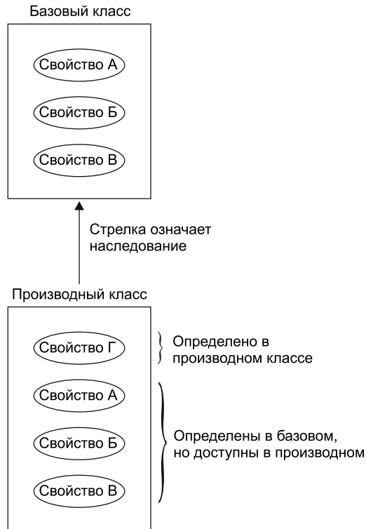
Рис. 9.1. Наследование
