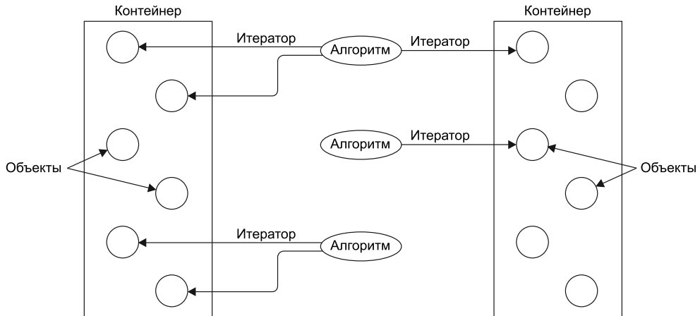
Алгоритмы используют итераторы для работы с объектами контейнеров.
