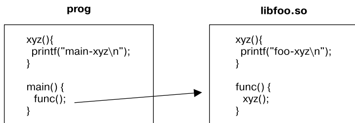
Рис. 41.5. Разрешение ссылки на глобальный символ
