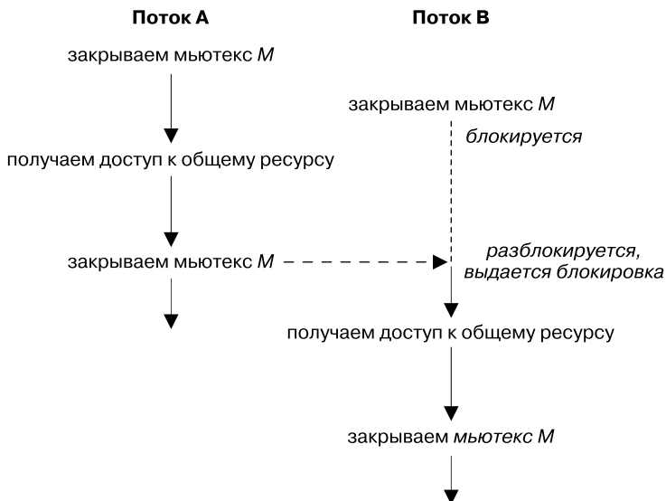
Рис. 30.2. Использование мьютекса для защиты критического участка
