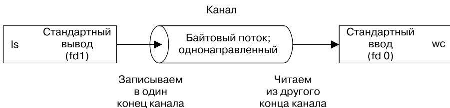
Рис. 44.1. Использование канала для соединения двух процессов
