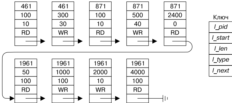
Рис. 51.6. Пример списка блокировок записей для одного файла
