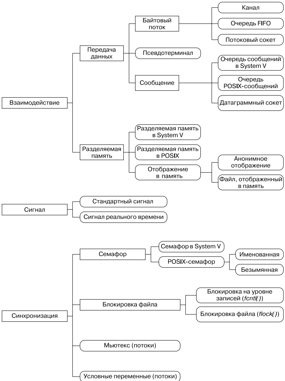
Рис. 43.1. Классификация IPC-механизмов в UNIX
