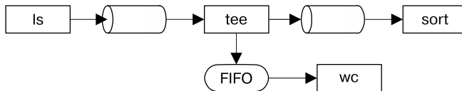
Рис. 44.5. Использование очереди FIFO и команды tee(1) для дублирования конвейера
