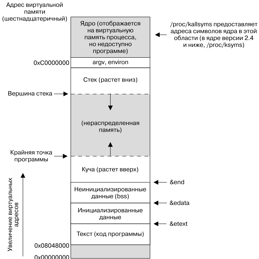
Рис. 6.1. Типичная структура памяти процесса в Linux/x86-32
