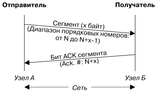
Рис. 57.3. Подтверждения в протоколе TCP
