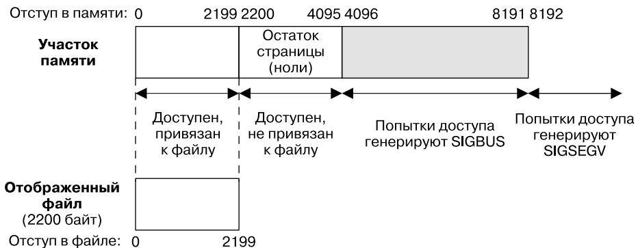
Рис. 45.4. Отображение в память выходит за пределы отображаемого файла
