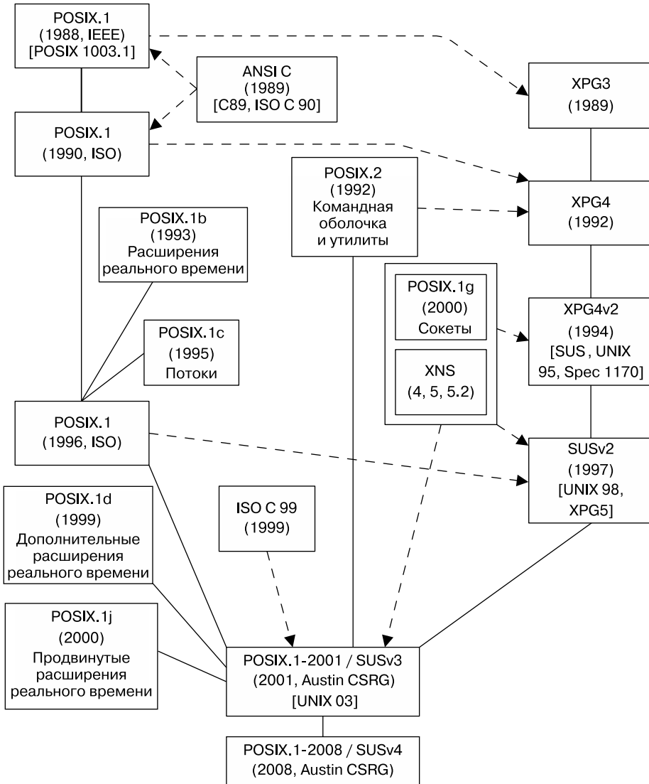
Рис. 1.1. Взаимоотношения между различными стандартами UNIX и C
