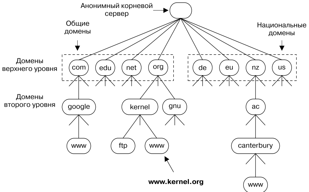
Рис. 55.2. Часть иерархии DNS
