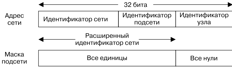
Рис. 54.6. Разделение на подсети в IPv4
