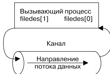
Рис. 44.2. Файловые дескрипторы процесса после создания канала
