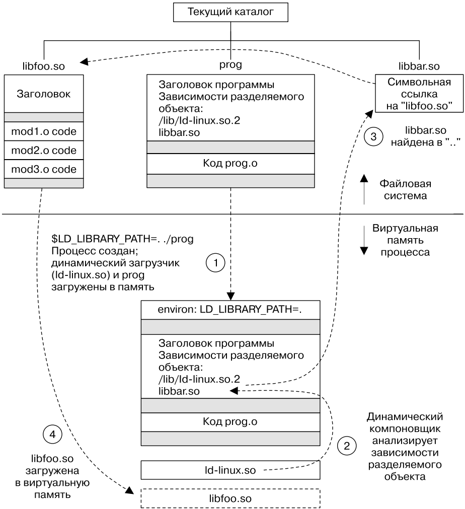
Рис. 41.2. Выполнение программы, загружающей разделяемую библиотеку
