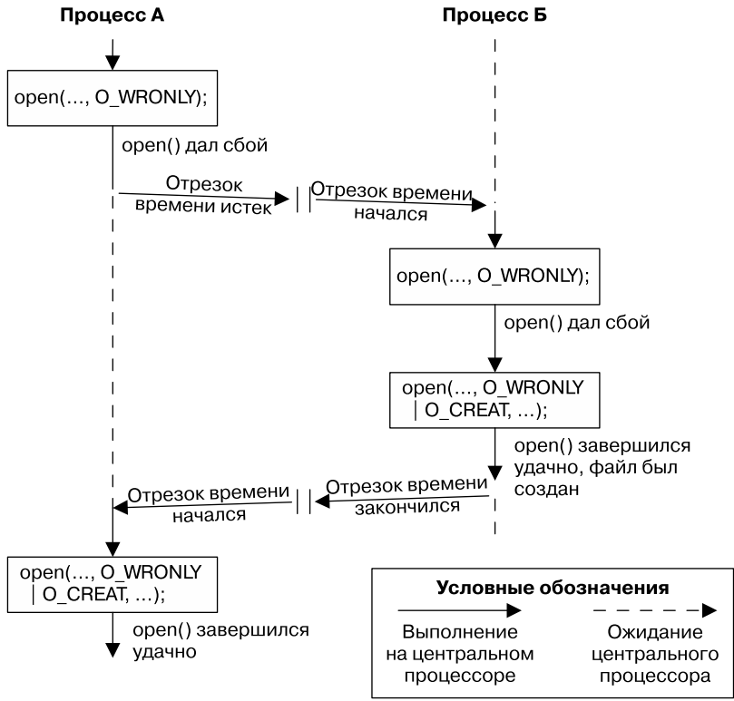
Рис. 5.1. Неудачная попытка эксклюзивного создания файла
