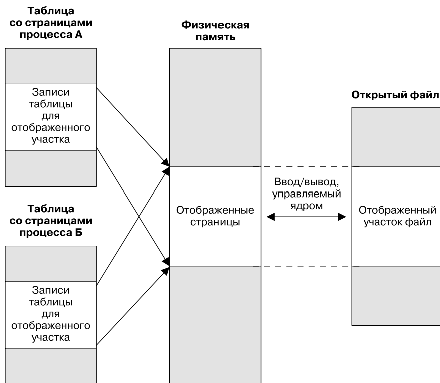
Рис. 45.2. Два процесса, совместно отображающие один и тот же участок файла
