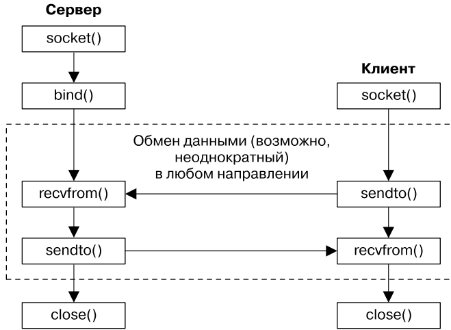
Рис. 52.4. Список системных вызовов, которые используются для работы с датаграммными сокетами
