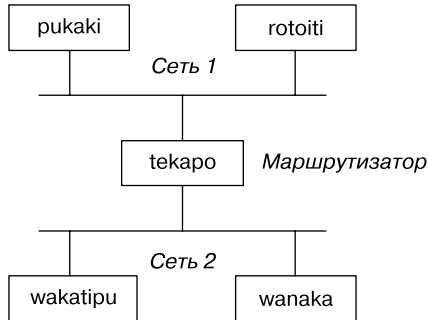
Рис. 54.1. Интернет использует маршрутизатор для соединения двух подсетей
