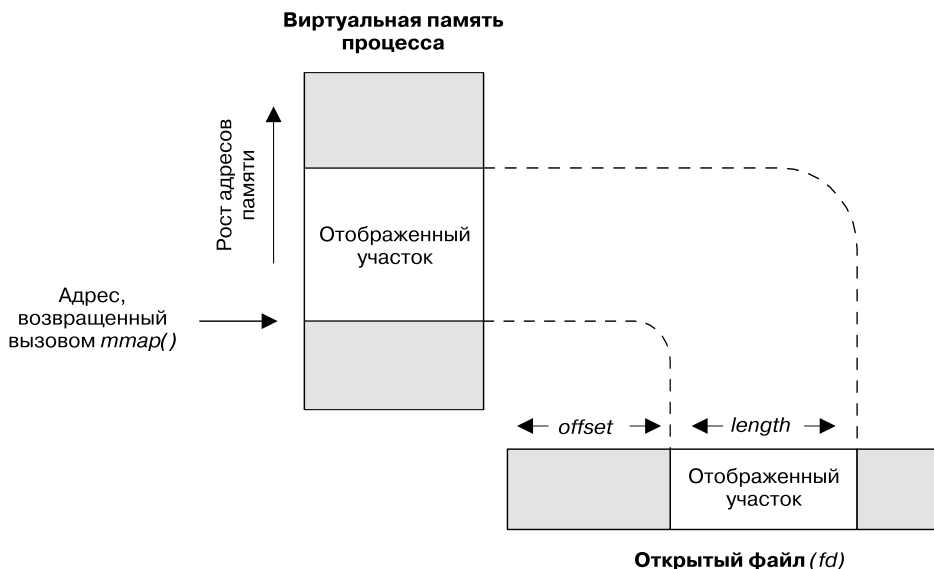
Рис. 45.1. Структура файла, отображенного в память
