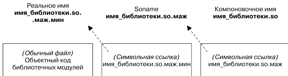
Рис. 41.3. Традиционная структура имен разделяемой библиотеки
