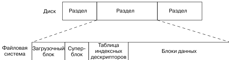
Рис. 14.1. Структура разделов диска и файловой системы
