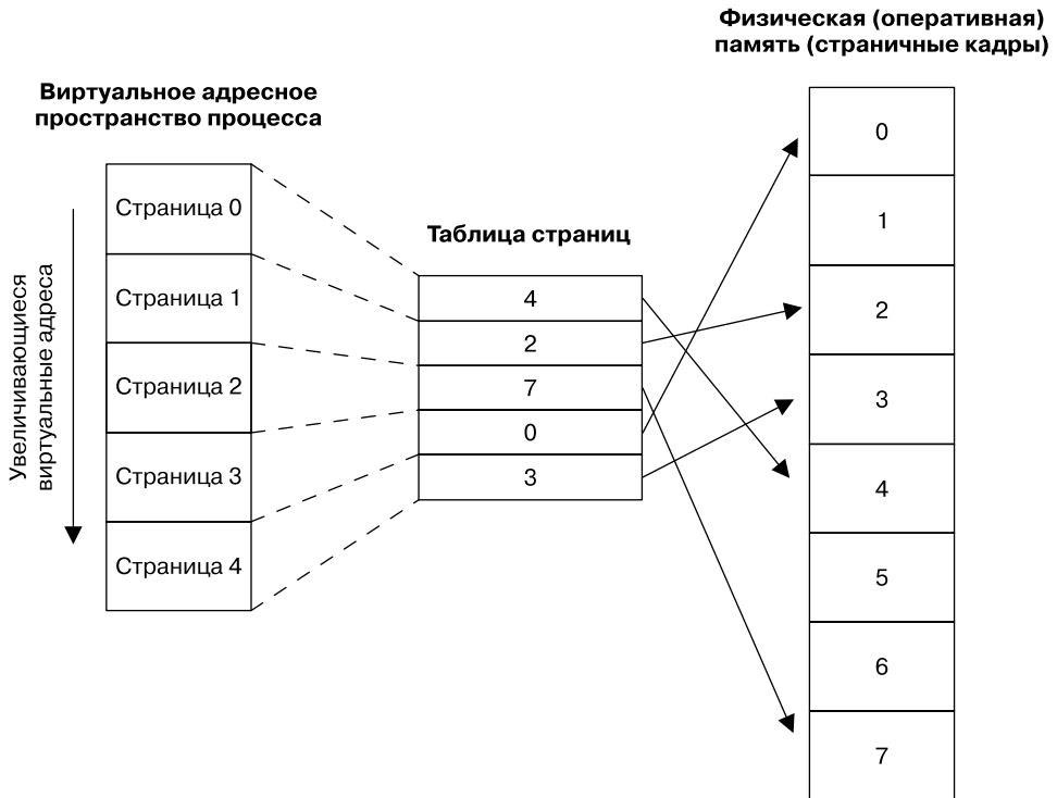
Рис. 6.2. Общий вид виртуальной памяти
