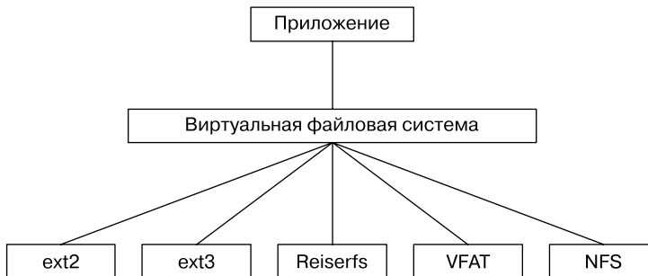
Рис. 14.3. Виртуальная файловая система
