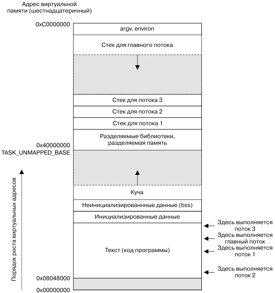
Рис. 29.1. Четыре потока, выполняющиеся внутри процесса (Linux/x86-32)
