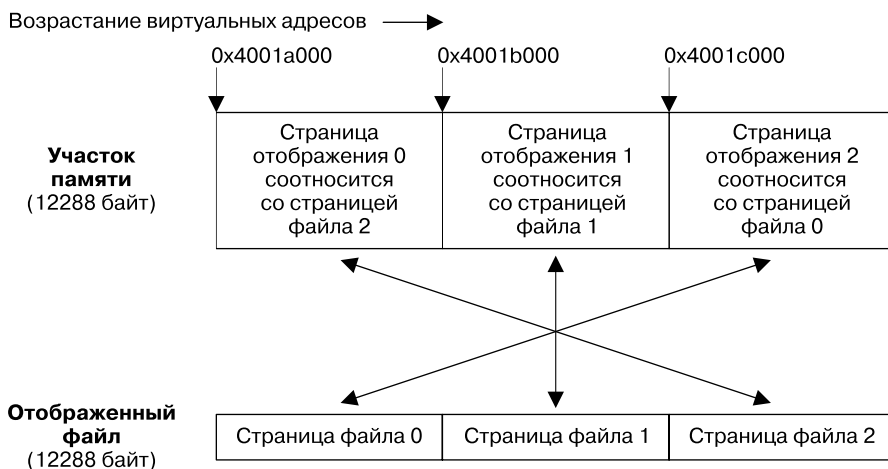
Рис. 45.5. Нелинейное отображение файла
