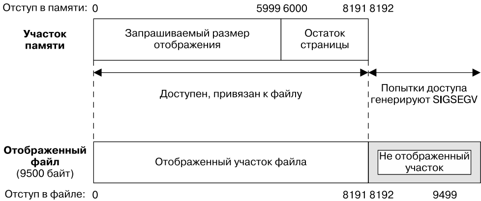
Рис. 45.3. Отображение, чья длина не кратна размеру страницы памяти в системе
