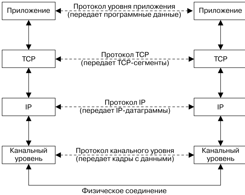
Рис. 54.3. Многоуровневое взаимодействие на основе протоколов TCP/IP
