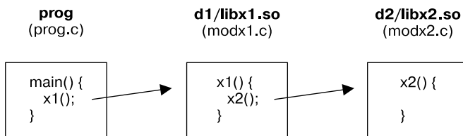
Рис. 41.4. Разделяемая библиотека, зависящая от другой разделяемой библиотеки
