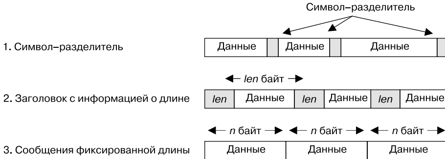
Рис. 44.7. Разделение сообщений в байтовом потоке
