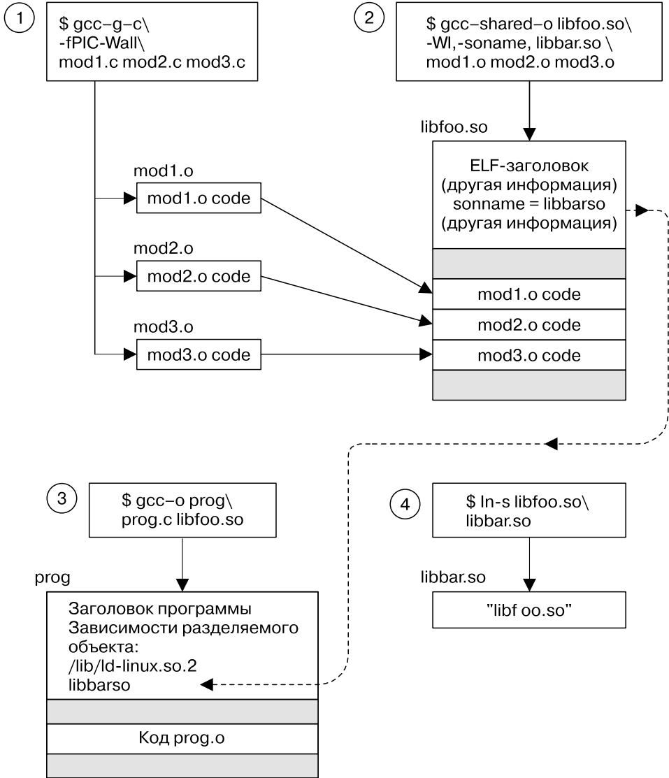
Рис. 41.1. Создание разделяемой библиотеки и компоновка с ней программы
