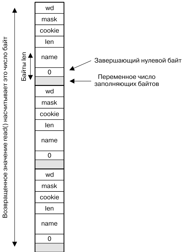
Рис. 19.2. Входящий буфер, содержащий три структуры inotify_event
