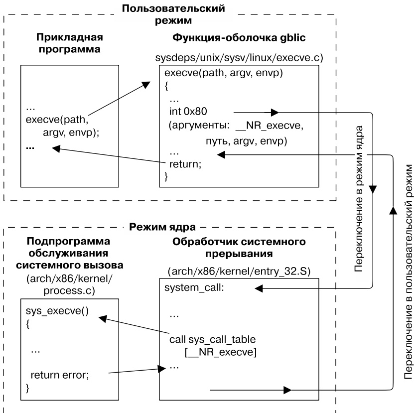
Рис. 3.1. Этапы выполнения системного вызова
