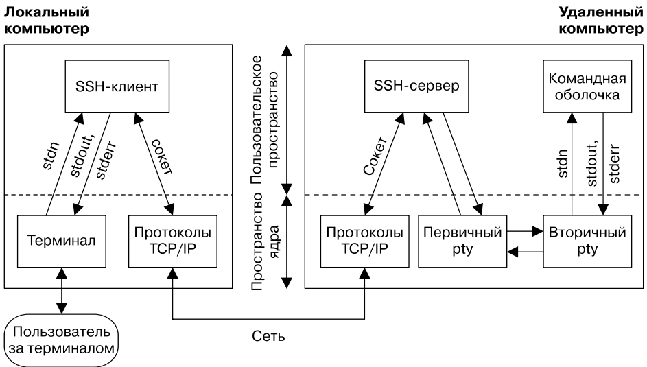
Рис. 60.3. Как ssh использует псевдотерминал
