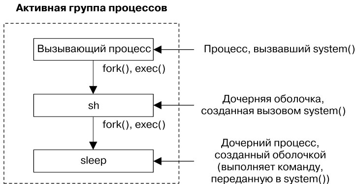
Рис. 27.2. Организация процессов во время выполнения system("sleep 20")
