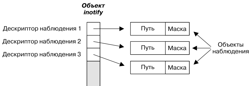
Рис. 19.1. Объект inotify и связанные структуры данных ядра
