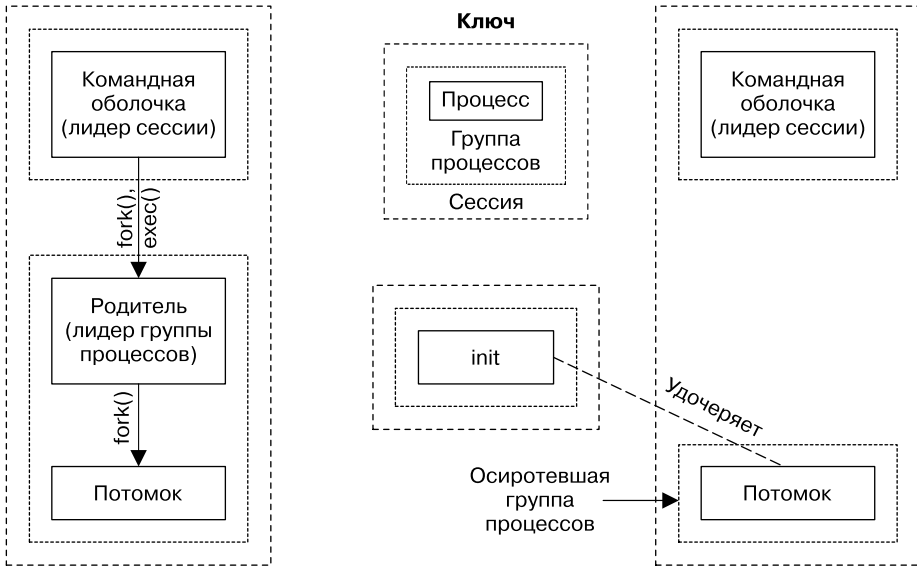
Рис. 34.3. Этапы создания «осиротевшей» группы процессов
