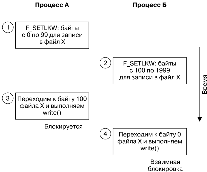
Рис. 51.7. Взаимная блокировка в случае поддержки строгих блокировок
