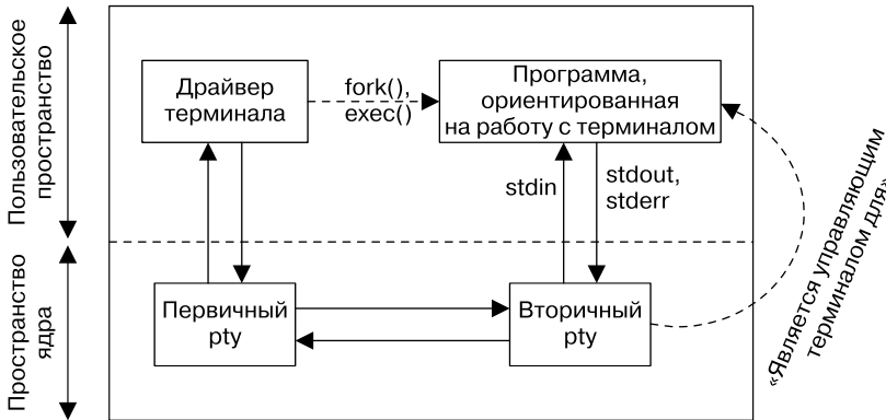
Рис. 60.2. Две программы, общающиеся через псевдотерминал
