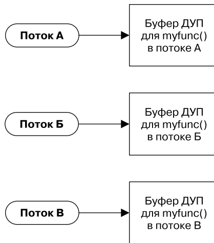
Рис. 31.1. Данные уровня потока (ДУП) предоставляют функции хранилище, относящееся к отдельному потоку
