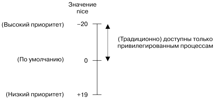
Рис. 35.1. Диапазон и интерпретация значений nice
