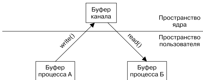
Рис. 43.2. Обмен данными между двумя процессами с помощью канала
