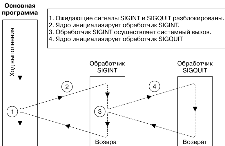
Рис. 22.1. Доставка нескольких разблокированных сигналов
