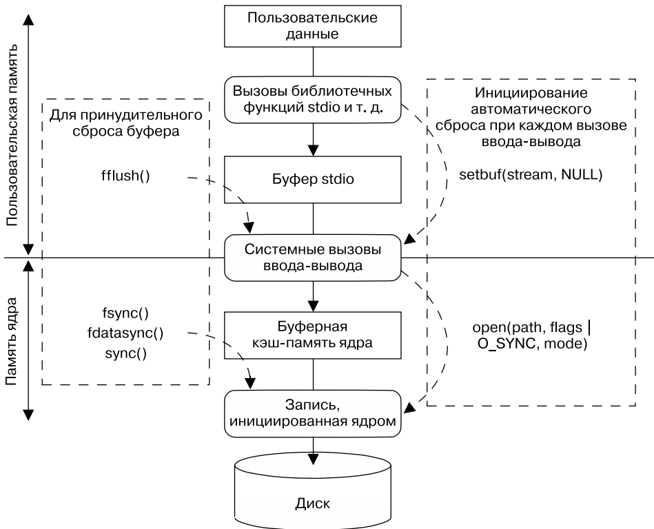
Рис. 13.1. Обзор буферизации ввода-вывода
