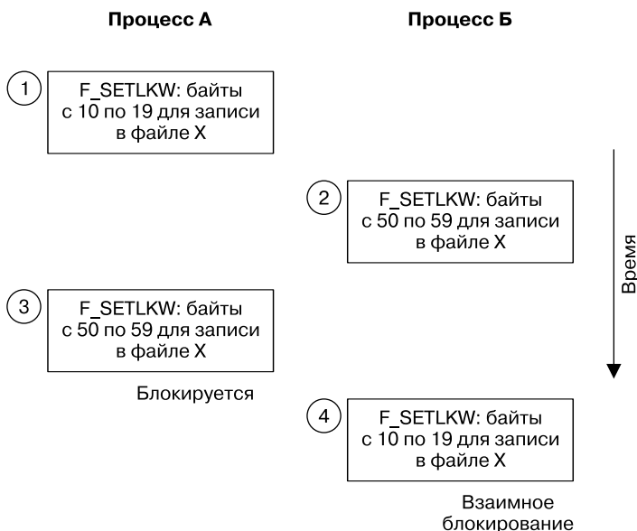
Рис. 51.4. Взаимная блокировка двух процессов, которые не дают друг другу выполнить запрос на получение блокировки
