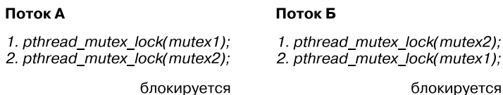
Рис. 30.3. Взаимное блокирование в ситуации, когда два потока закрывают два мьютекса
