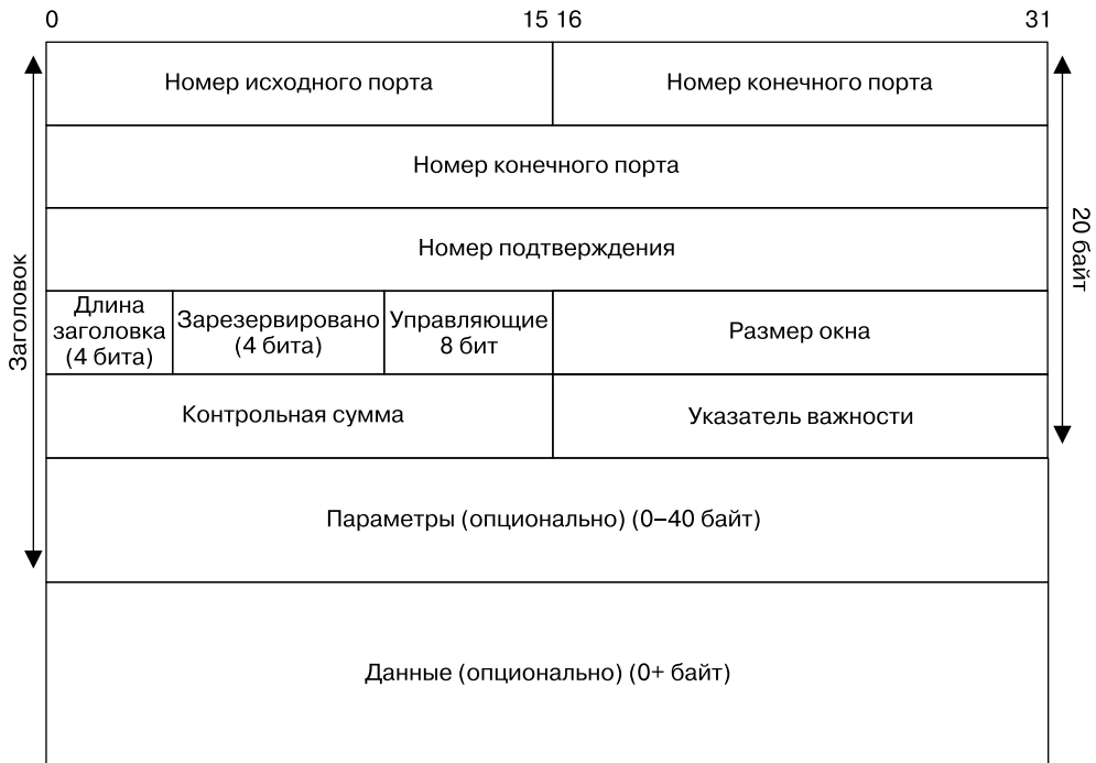
Рис. 57.2. Формат TCP-сегмента
