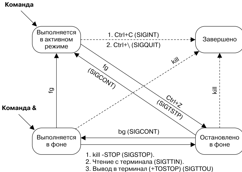
Рис. 34.2. Состояния задания
