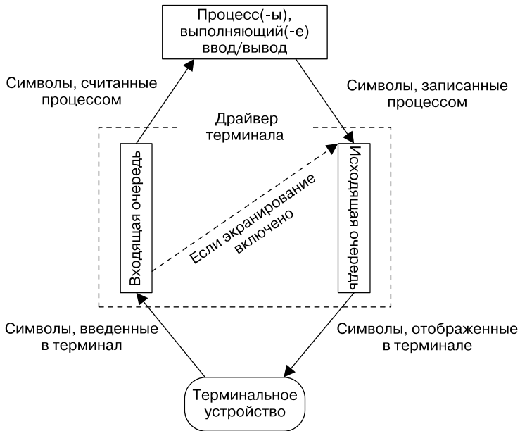
Рис. 58.1. Входящая и исходящая очереди терминального устройства
