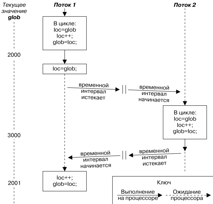
Рис. 30.1. Два потока, инкрементирующих глобальную переменную без синхронизации
