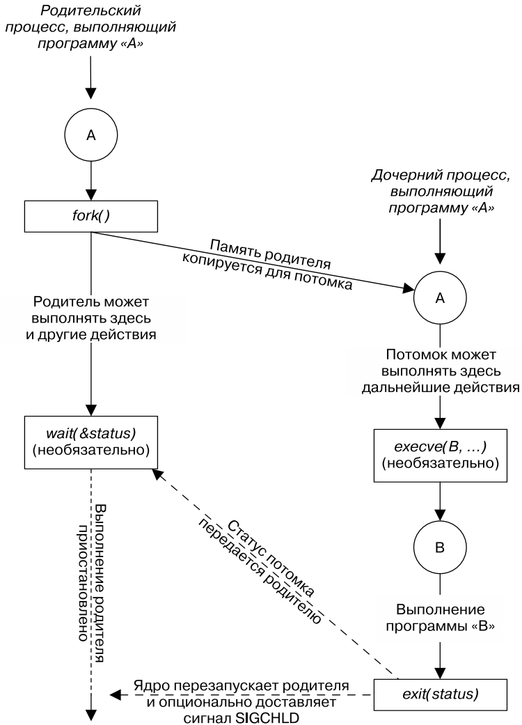
Рис. 24.1. Обор вызовов fork() , exit() , wait() и execve()
