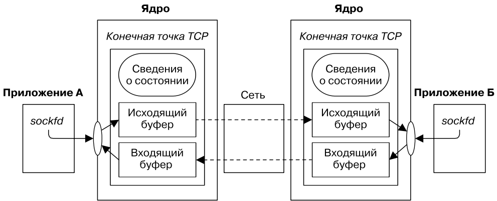
Рис. 54.8. Сокеты, соединенные по TCP
