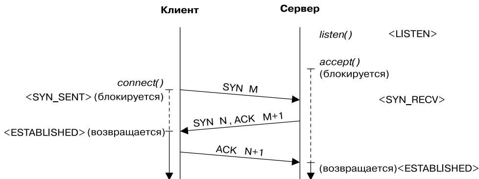
Рис. 57.5. Трехэтапное согласование при установке TCP-соединения
