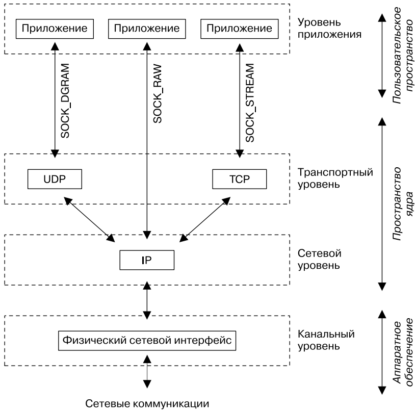
Рис. 54.2. Протоколы семейства TCP/IP
