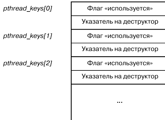
Рис. 31.2. Реализация ключей для данных уровня потока
