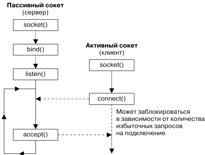
Рис. 52.2. Отложенное соединение с сокетом
