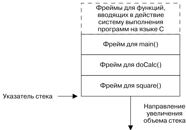
Рис. 6.3. Пример стека процесса
