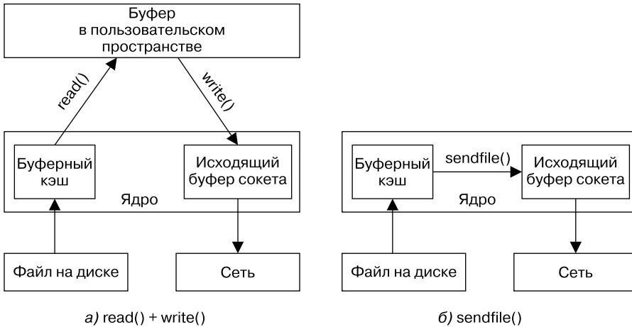
Рис. 57.1. Передача содержимого файла через сокет
