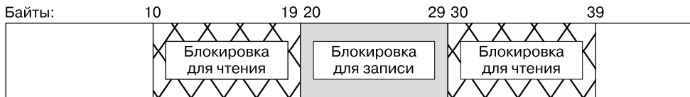
Рис. 51.3. Расщепление существующей блокировки в режиме чтения блокировкой в режиме записи, установленной тем же процессом
