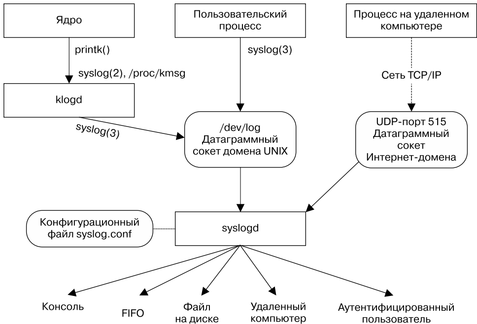
Рис. 37.1. Принцип работы системного журнала
