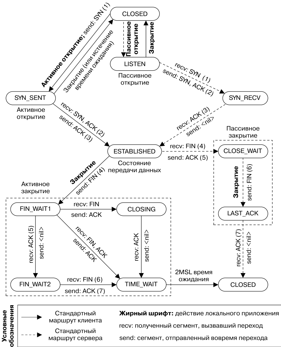
Рис. 57.4. Диаграмма перехода состояний для протокола TCP
