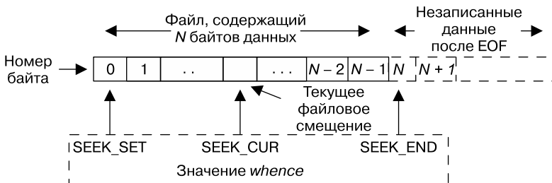
Рис. 4.1. Интерпретация аргумента whence системного вызова lseek()
