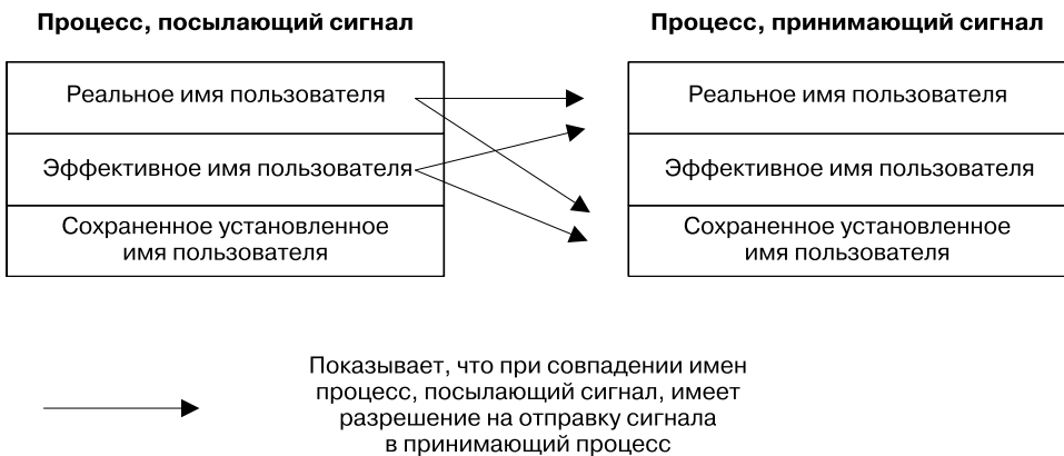
Рис. 20.2. Разрешения, необходимые непривилегированному процессу для отправки сигнала
