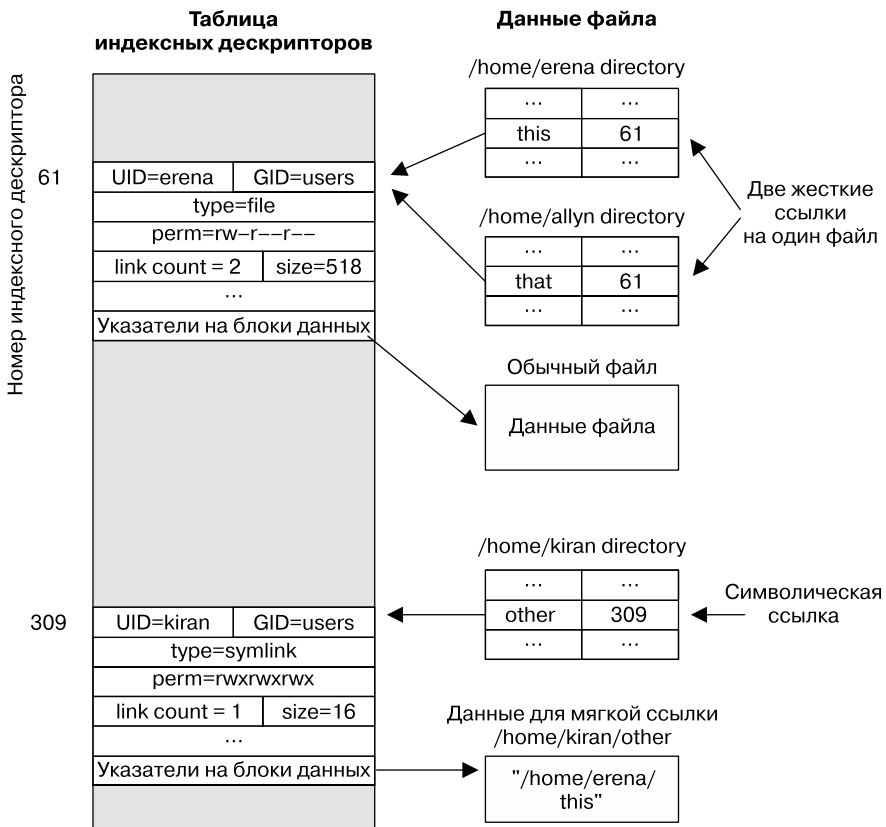
Рис. 18.2. Представление жестких и символических ссылок
