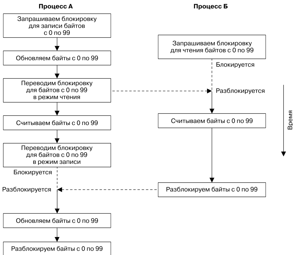
Рис. 51.2. Синхронизация доступа к одному и тому же участку файла с помощью блокировки записей
