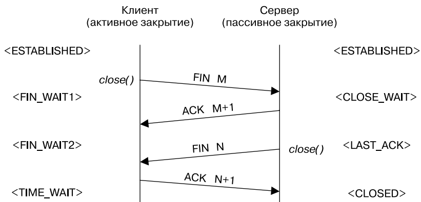
Рис. 57.6. Разрыв TCP-соединения
