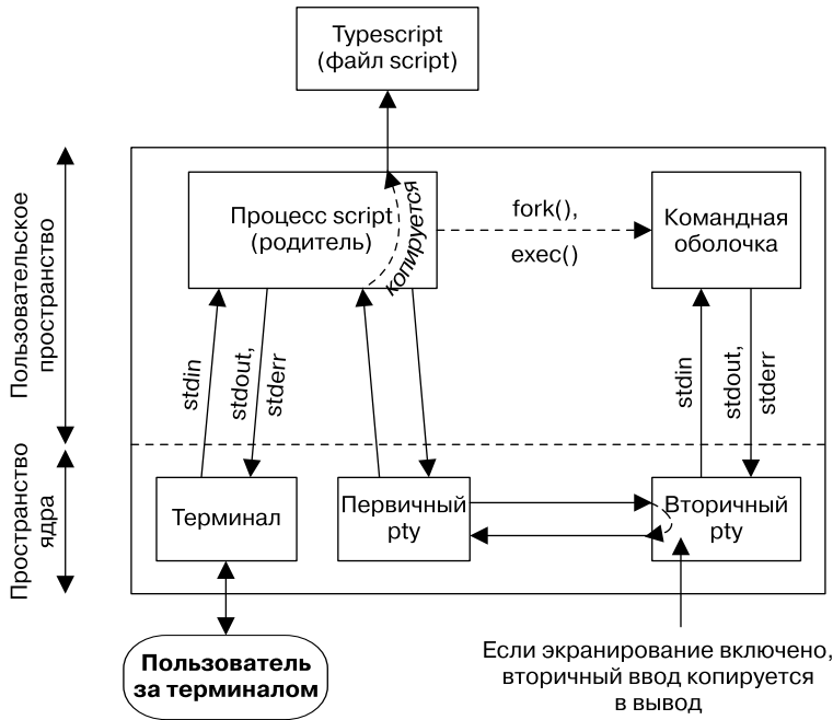
Рис. 60.4. Программа script
