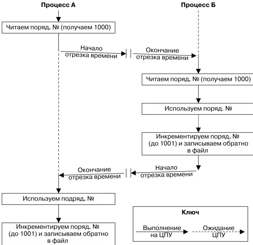
Рис. 51.1. Два процесса одновременно обновляют файл без синхронизации
