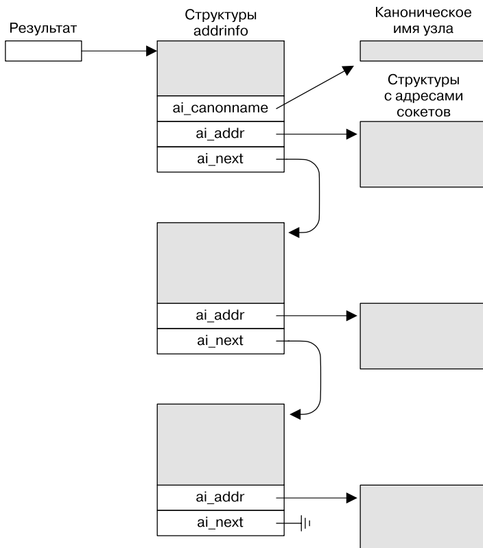
Рис. 55.3. Структуры, выделяемые и возвращаемые функцией getaddrinfo()
