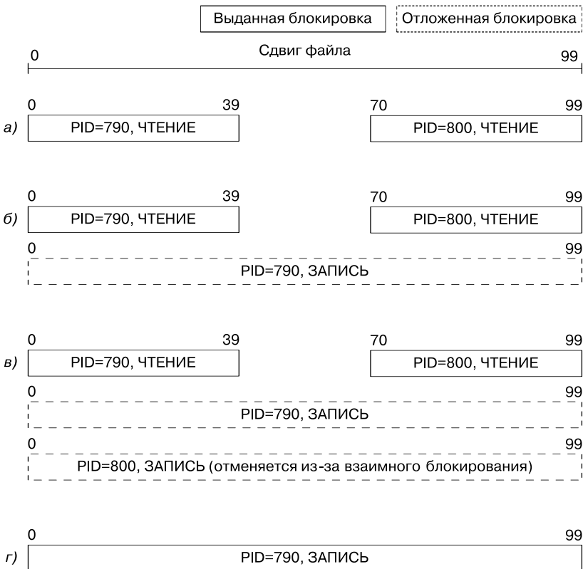
Рис. 51.5. Состояние удовлетворенных и отложенных запросов при выполнении программы i_fcntl_locking.c
