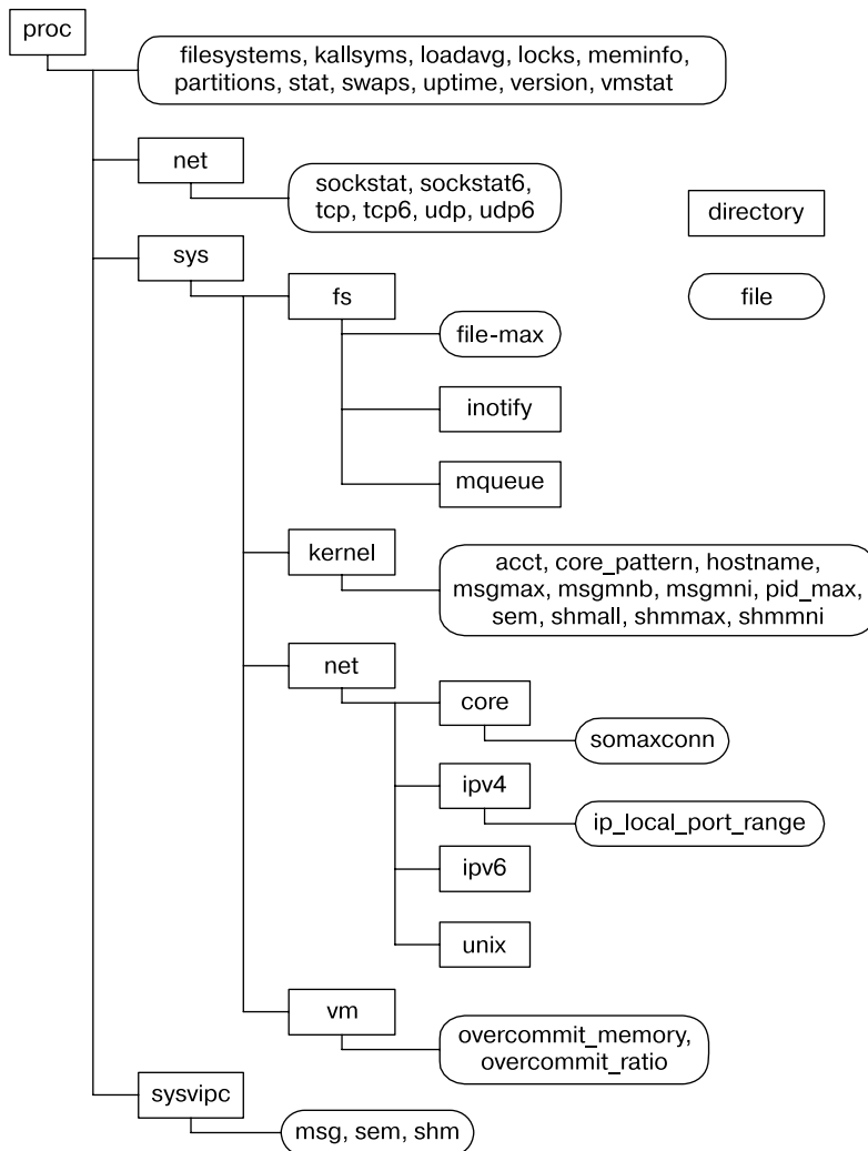
Рис. 12.1. Отдельные файлы и подкаталоги, находящиеся в /proc
