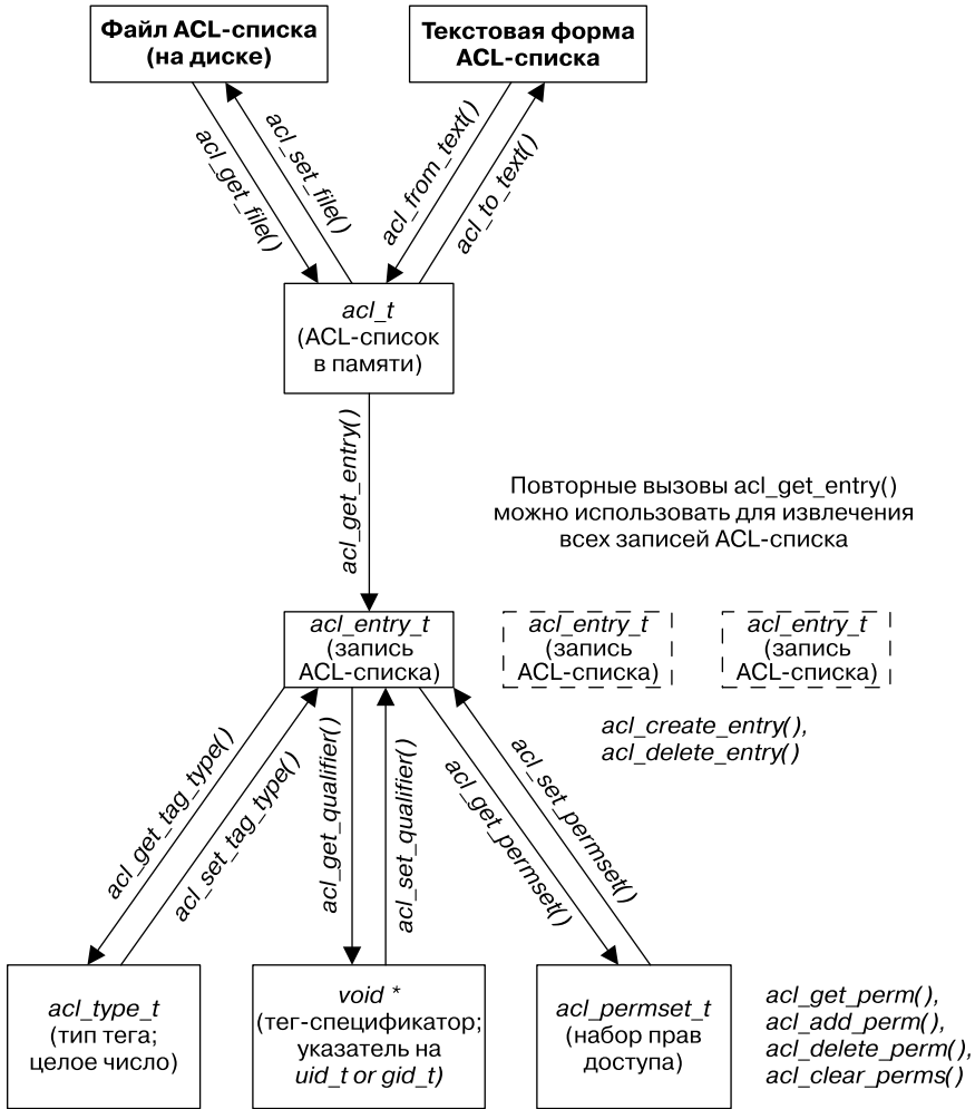
Рис. 17.2. Взаимосвязь между библиотечными ACL-функциями и структурами данных
