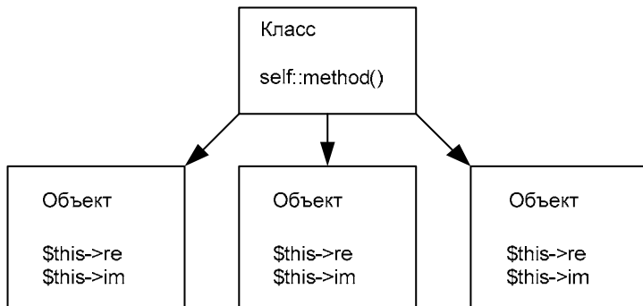
Рис. 14.1. Ключевое слово self используется для обращения к внутренним переменным и методам класса, а ключевое слово $this — к переменным и методам объекта
