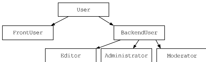
Рис. 31.1. Иерархия наследования пользователей
