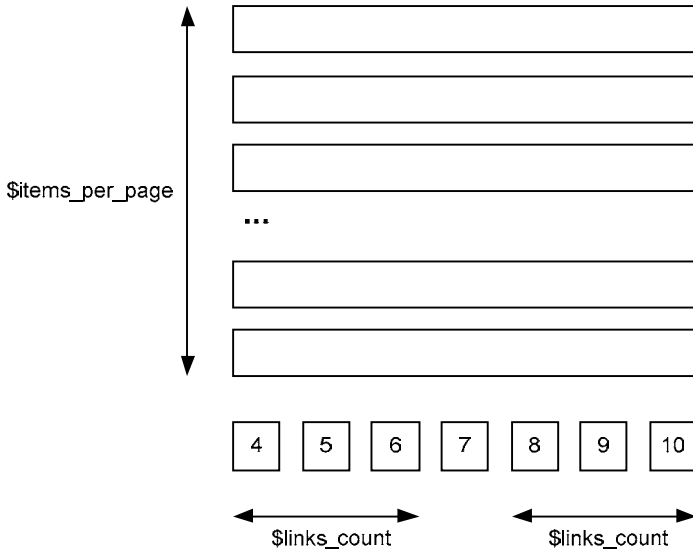
Рис. 50.2. Простейший вариант постраничной навигации
