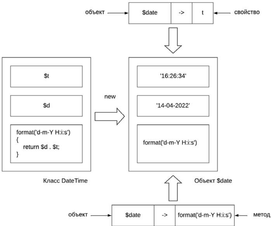
Рис. 6.4. Связь класса, объекта, свойств и методов
