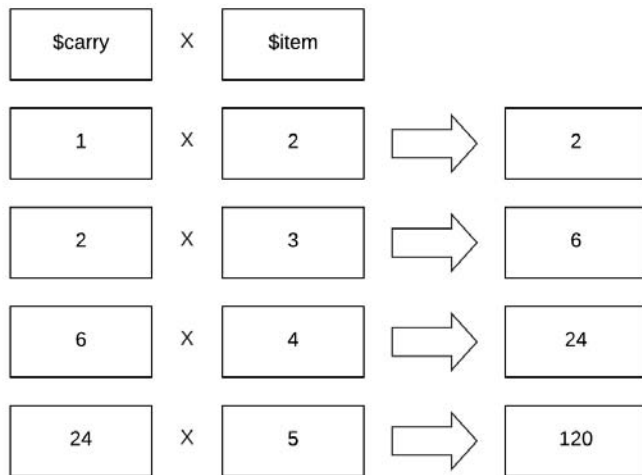
Рис. 13.7. Свертка массива [1, 2, 3, 4, 5] в число 120
