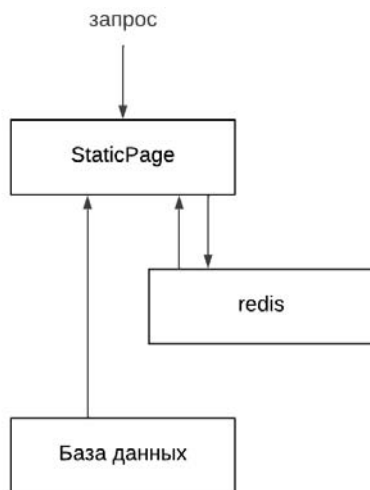
Рис. 30.2. Кеширование данных из базы данных в Redis
