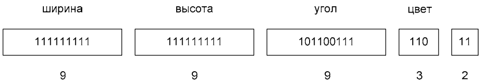
Рис. 8.7. Двоичное представление графического примитива
