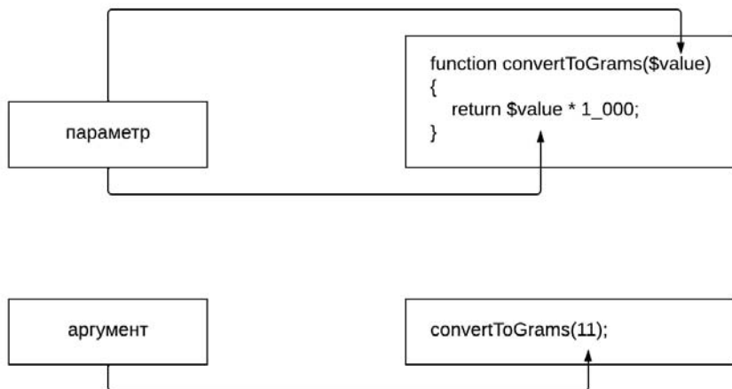
Рис. 12.4. Параметры и аргументы функции
