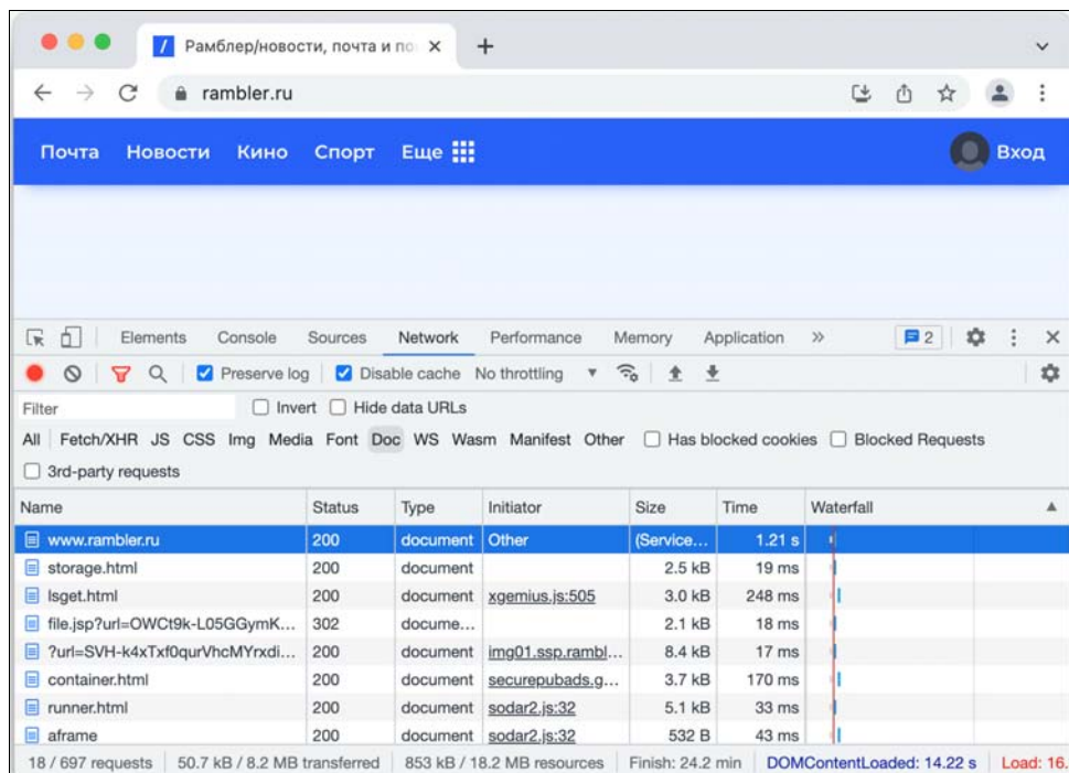
Рис. 2.6. Панель веб-разработчика
