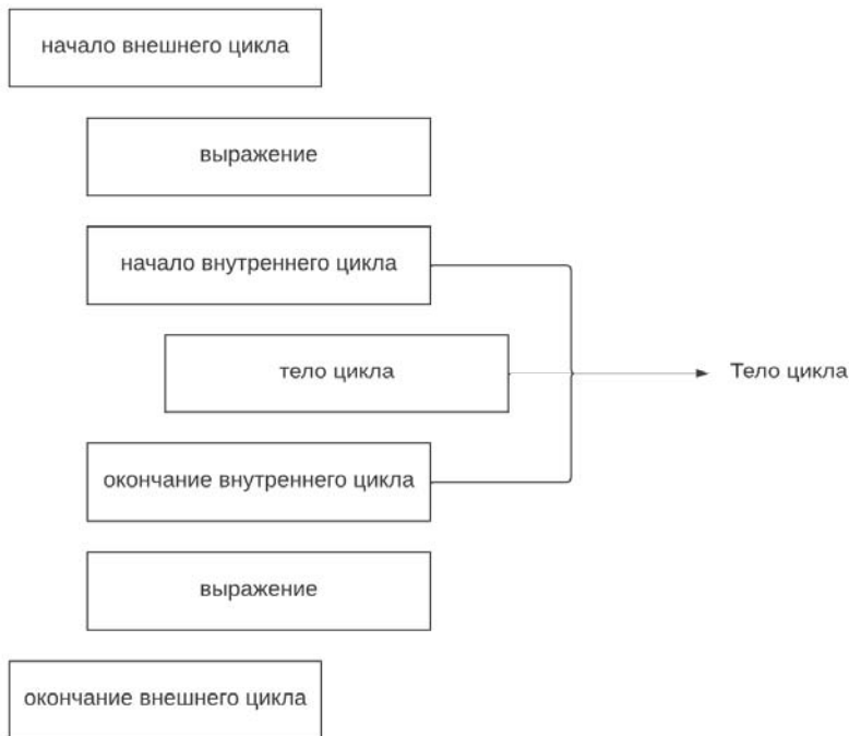
Рис. 10.2. Вложенные циклы
