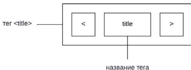
Рис. 17.4. Структура тега
