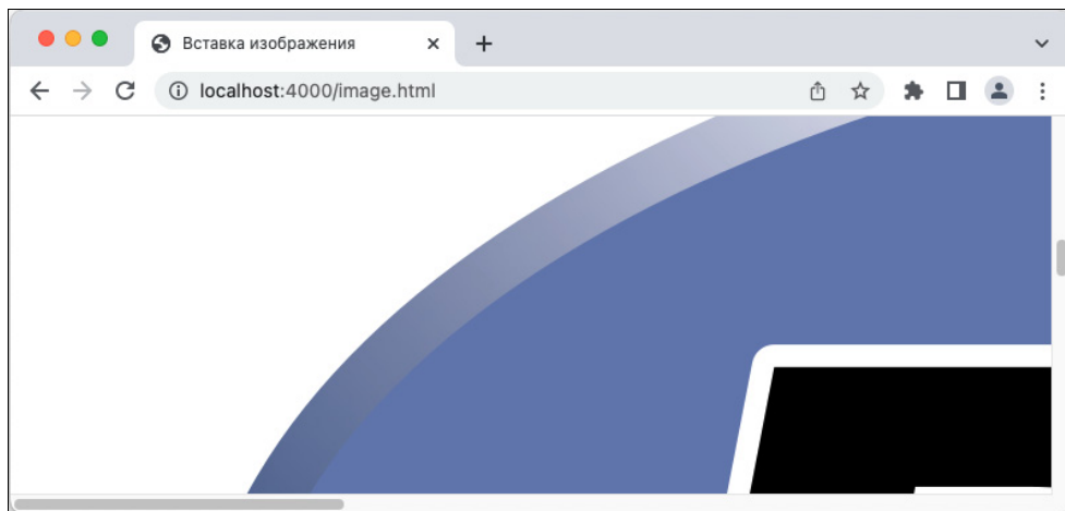
Рис. 17.15. Вывод изображения
