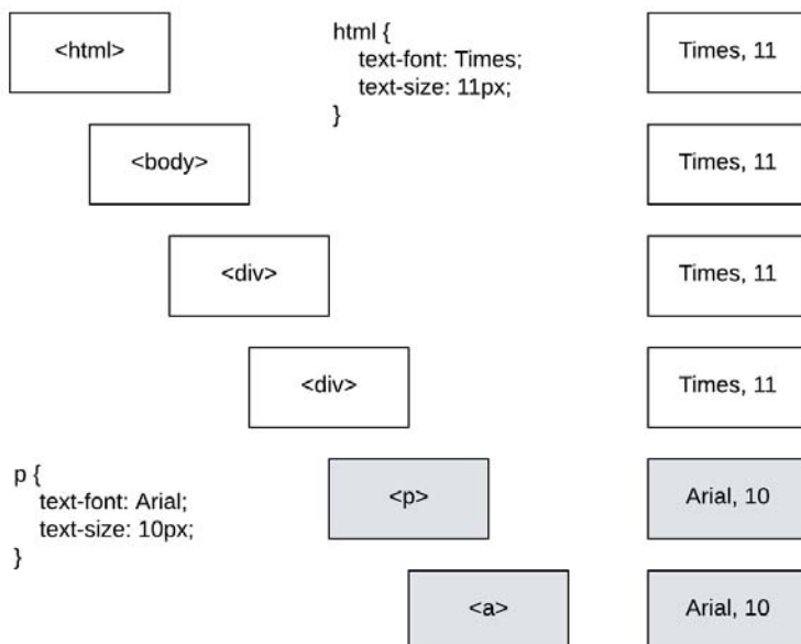
Рис. 17.18. Наследование свойств
