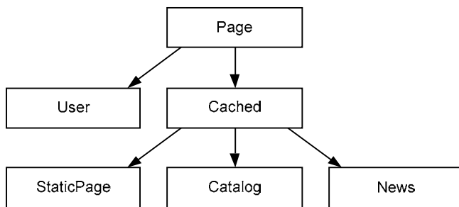
Рис. 30.1. Диаграмма классов
