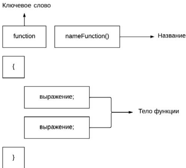
Рис. 12.2. Определение функции
