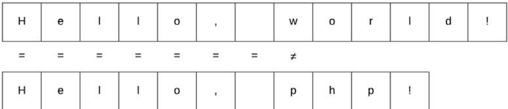
Рис. 8.12. Сравнение строк
