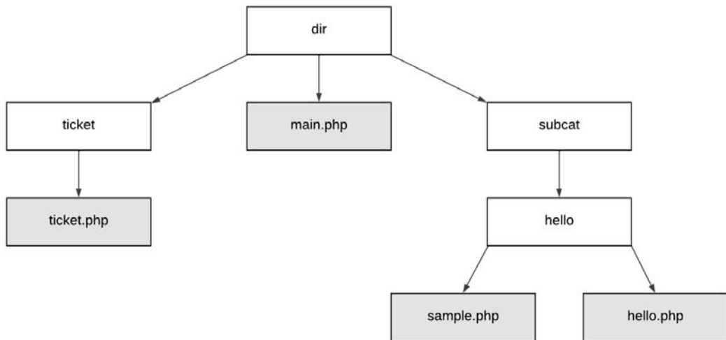
Рис. 13.1. Файловая система
