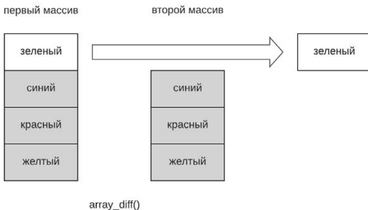
Рис. 11.4. Исключительное пересечение
