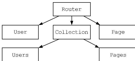
Рис. 37.1. Иерархия классов
