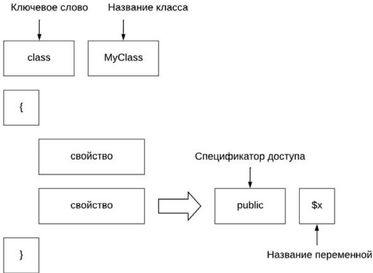
Рис. 6.5. Структура класса
