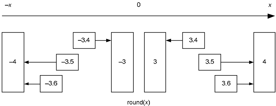
Рис. 22.1. Схема округления числа при помощи функции round()
