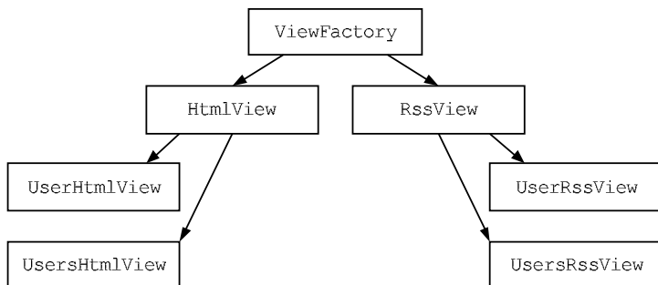
Рис. 37.4. Альтернативная схема наследования классов для представления
