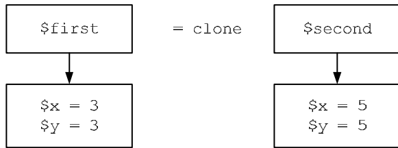
Рис. 6.9. Получение независимой копии объекта $second посредством клонирования
