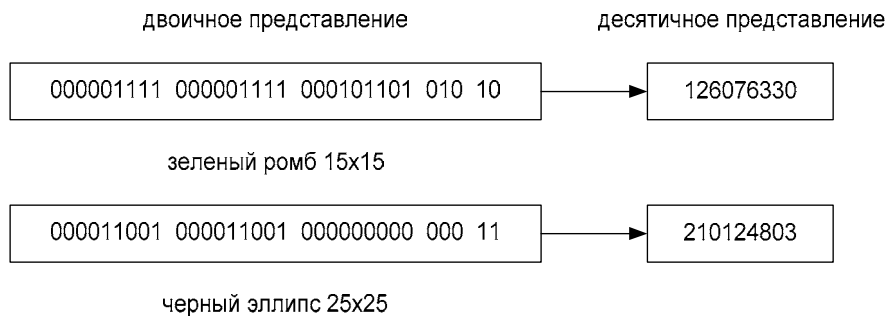
Рис. 8.8. Двоичное и десятичное представления графических примитивов
