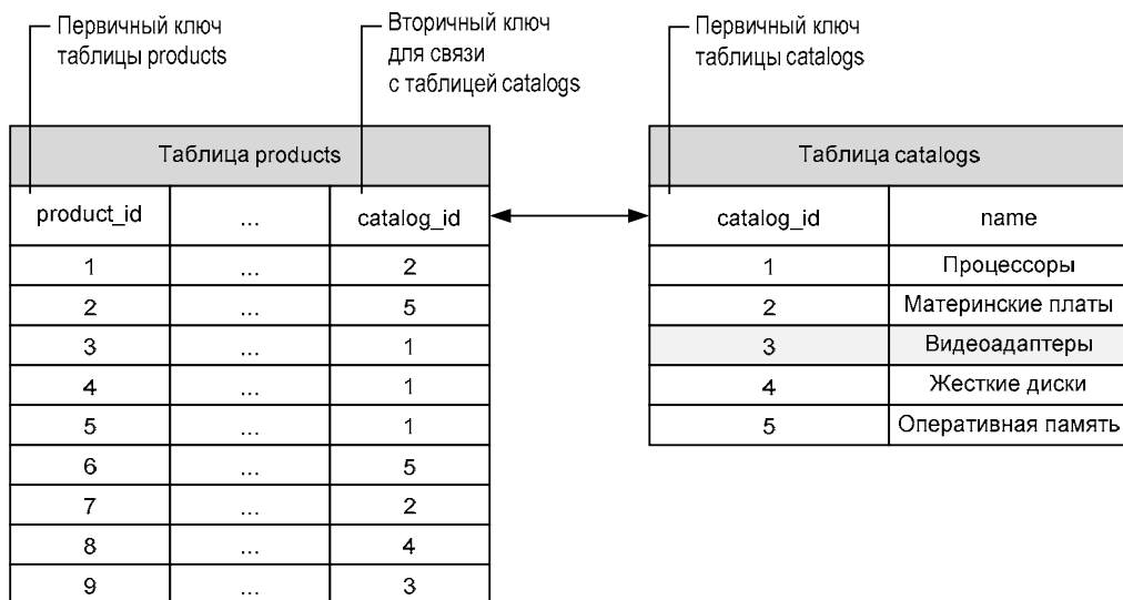
Рис. 41.4. Связь между таблицами products и catalogs
