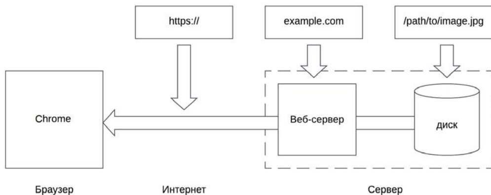
Рис. 2.3. Схема URL
