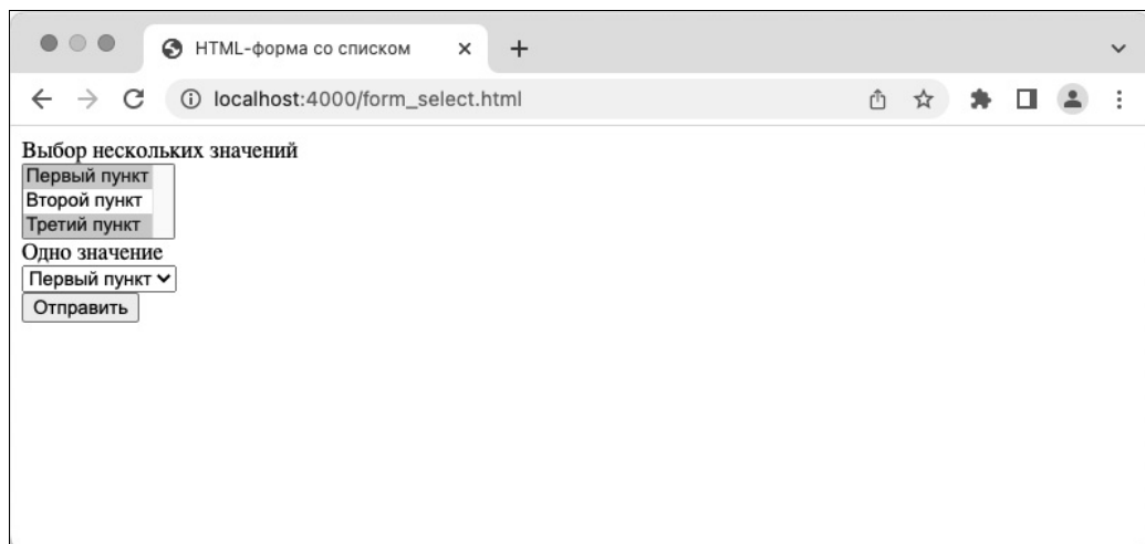
Рис. 18.5. Использование списков
