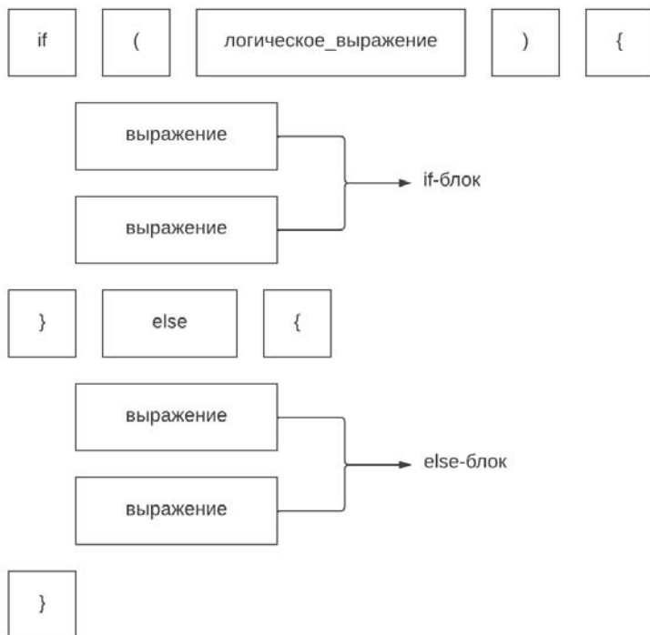
Рис. 9.1. Структура if-конструкции
