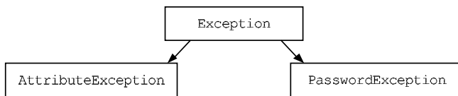
Рис. 34.1. Наследование исключений
