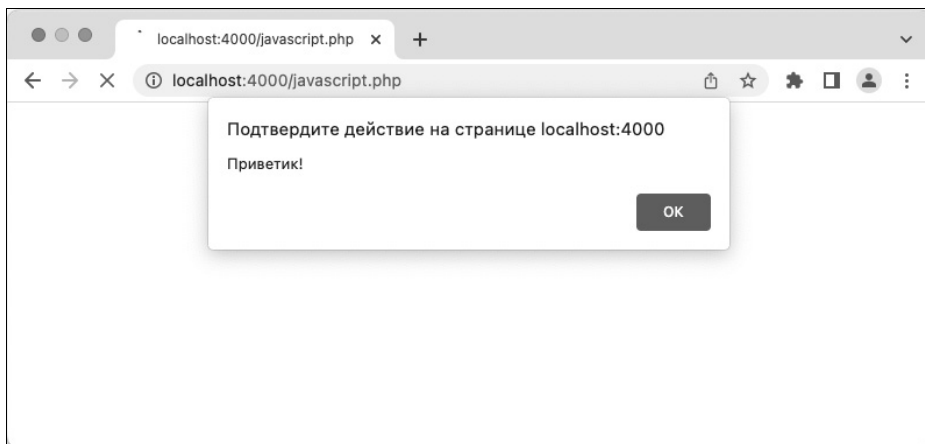
Рис. 16.5. Выполнение JavaScript-кода
