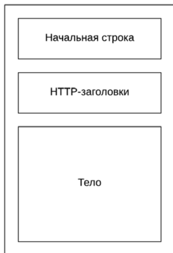
Рис. 2.4. HTTP-сообщение
