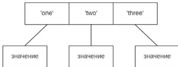
Рис. 11.2. Ассоциативный массив
