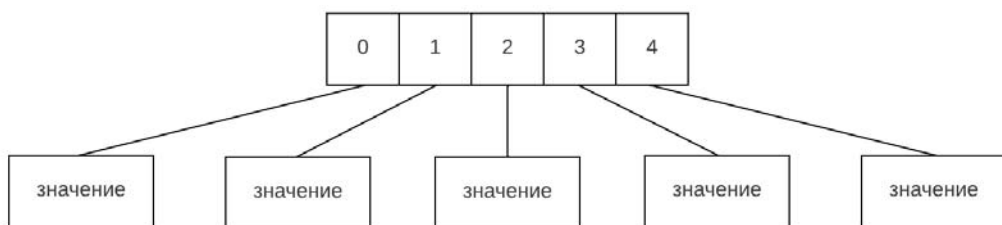
Рис. 11.1. Массив
