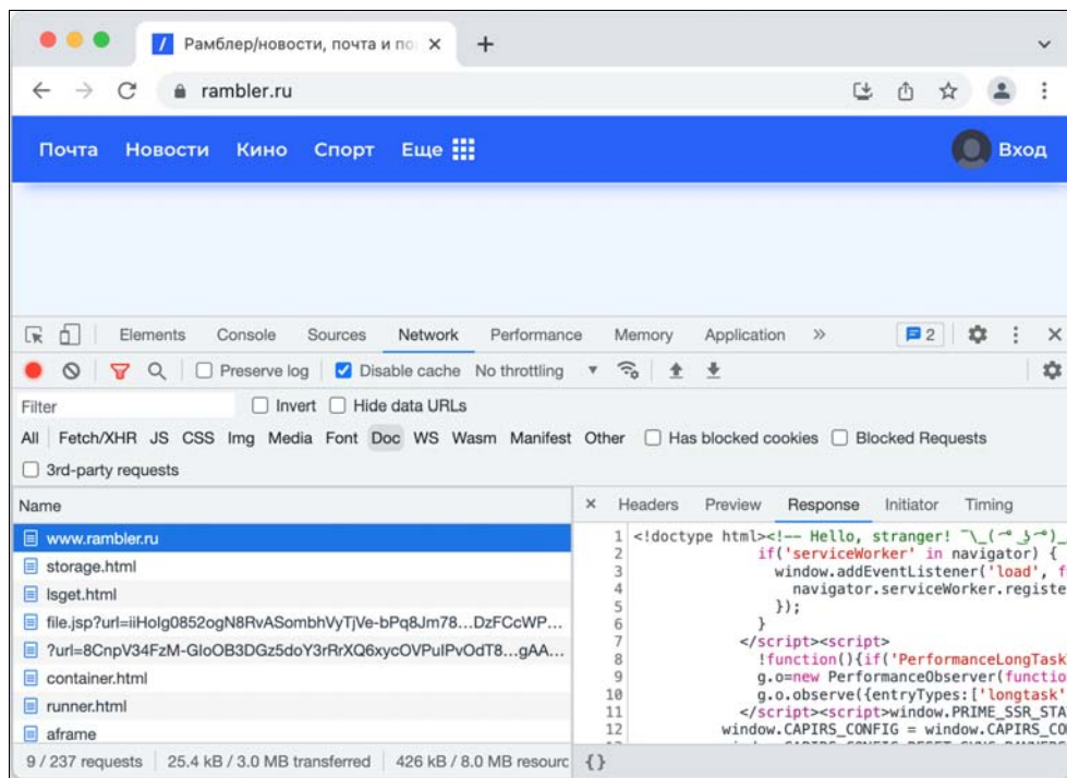
Рис. 2.8. Содержимое HTML-документа
