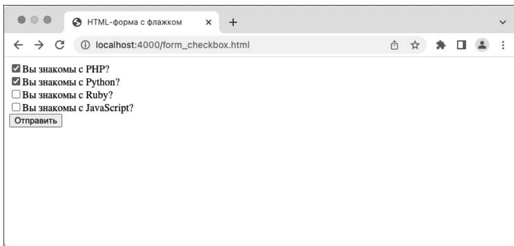
Рис. 18.4. Использование флажков
