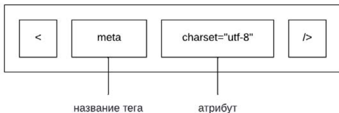
Рис. 17.6. Атрибуты тегов
