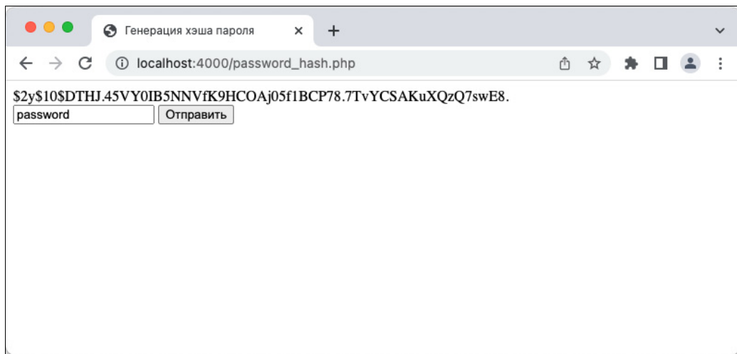
Рис. 29.2. Генерация хэша для произвольной строки
