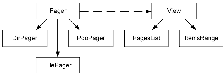
Рис. 50.1. Диаграмма классов компонента постраничной навигации
