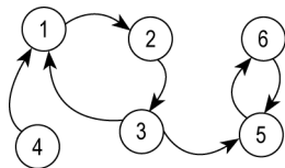
Рис. 27.8. Пример графа
