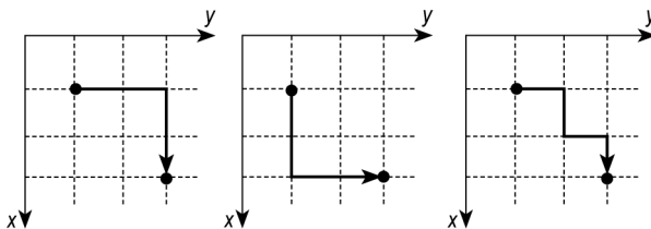
Рис. 5.2. Кратчайшие пути
