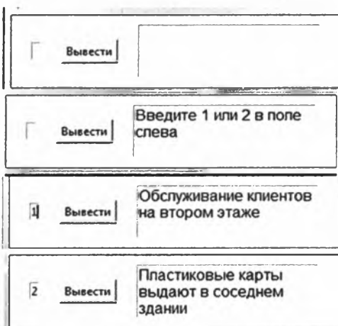
Рис. 5.24. Графический интерфейс
