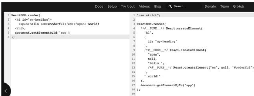
Рис. 5.2. Преобразованный пример Hello World
