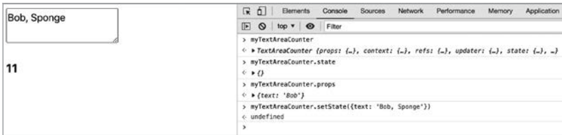
Рис. 2.5. Обращение к выведенному на экран компоненту с помощью ссылки
