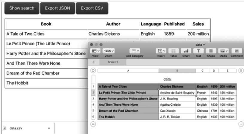
Рис. 3.14. Экспорт данных таблицы в Numbers с использованием CSV-формата
