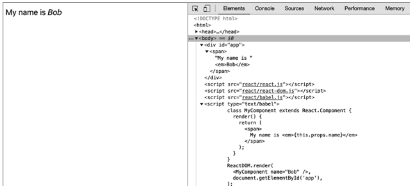
Рис. 2.2. Использование свойств компонентов (файл 02.05.this.props.html)
