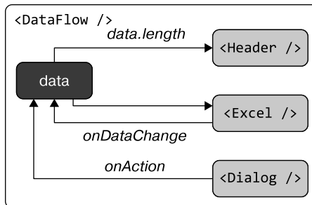
Рис. 8.4. Поток данных (data)
