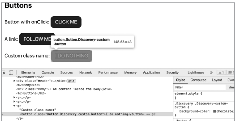
Рис. 7.8. Компонент <Button> с пользовательским именем класса
