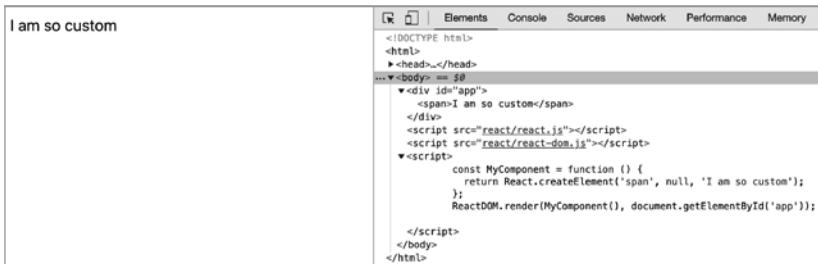
Рис. 2.1. Ваш первый настраиваемый компонент (файл 02.01.custom-functional.html в репозитории книги)
