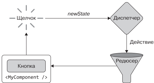
Рис. 4.5. Процесс «компонент — диспетчер — действие — редюсер» (component-dispatch-action-reducer)
