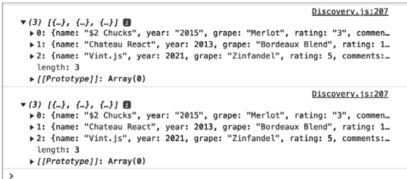
Рис. 7.19. Два консольных сообщения после изменения "$2 Chuck" на "$2 Chucks"
