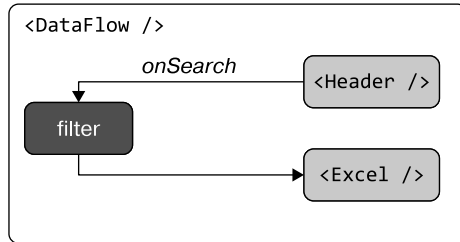
Рис. 8.5. Передача строки поиска ( filter )
