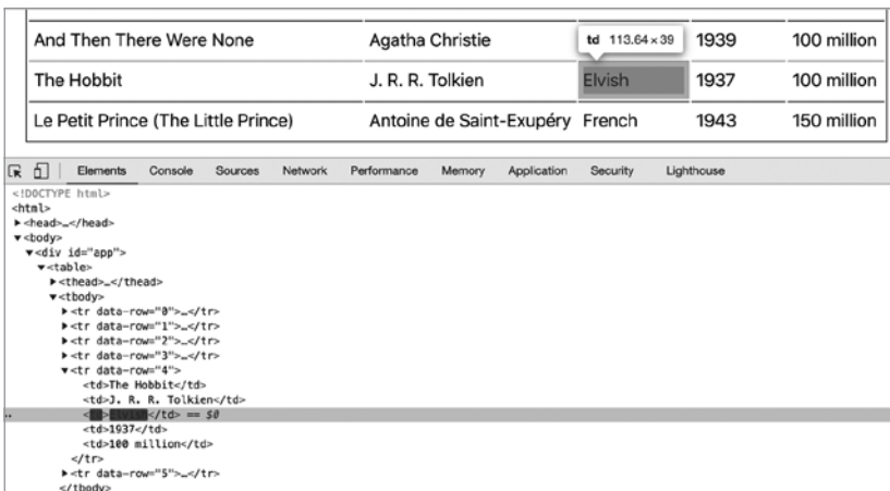
Рис. 3.9. Выделение изменений DOM
