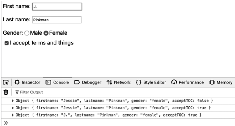
Рис. 5.8. Неуправляемый компонент в действии
