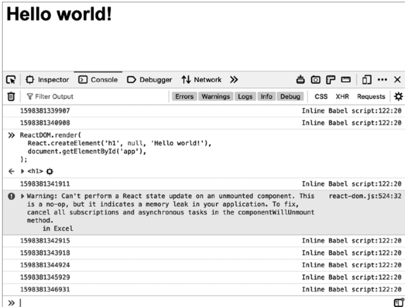
Рис. 3.13. Утечка памяти в действии
