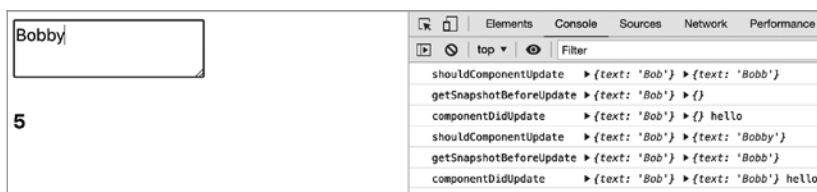
Рис. 2.7. Еще одно обновление компонента
