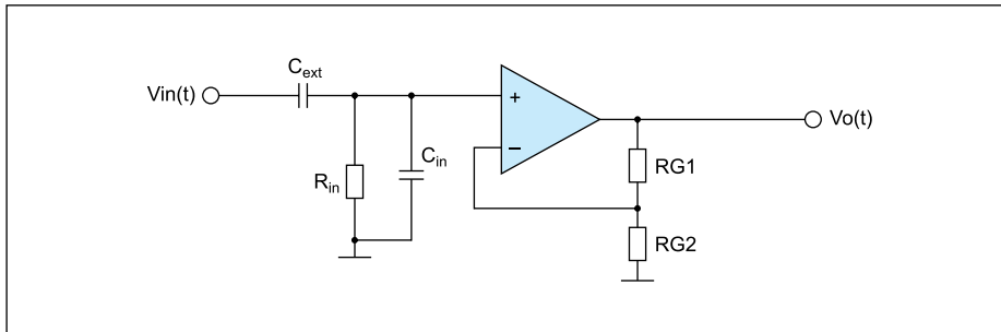
Рис. 2. Входной каскад датчика EPIC
