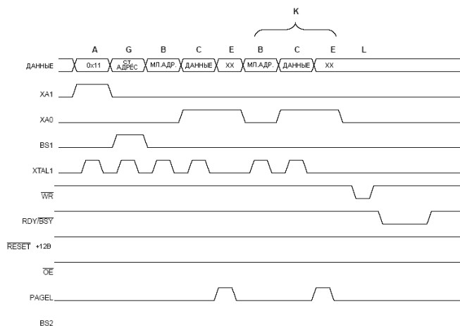
Рисунок 138. Осциллограммы сигналов
