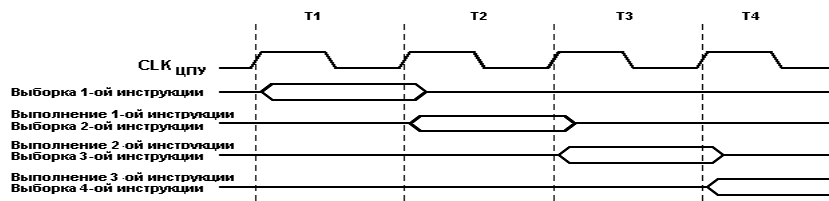
Рисунок 6 \sqrt Параллельные выборы и исполнения инструкций
