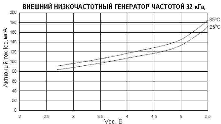
Рисунок 165. Зависимость активного потребляемого тока от напряжения питания (тактирование внешним низкочастотным генератором частотой 32 кГц)
