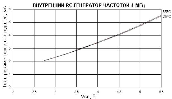
Рисунок 169. Зависимость потребляемого тока в режиме холостого хода (Idle) от напряжения питания (тактирование внутренним RC-генератором частотой 4МГц)
