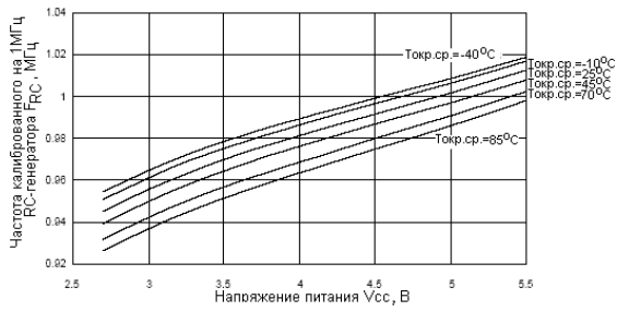
Рисунок 196. Зависимость частоты RC-генератора от напряжения питания (микроконтроллеры откалиброваны на частоту 1 МГц при напряжении питания V_{cc} = 5\text{В} и температуре T=25\text{ }^{\circ}\text{C} )
