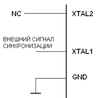
Рисунок 21 √ Схема подключения внешнего источника синхронизации
