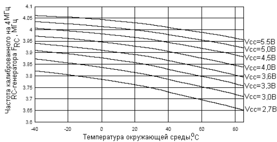
Рисунок 199. Зависимость частоты RC-генератора от температуры (микроконтроллеры откалиброваны на частоту 4 МГц при напряжении питания V_{cc} = 5\text{В} и температуре T=25\text{ }^{\circ}\text{C} )
