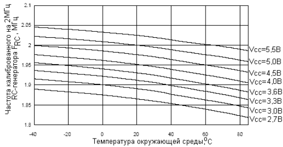
Рисунок 197. Зависимость частоты RC-генератора от температуры (микроконтроллеры откалиброваны на частоту 2 МГц при напряжении питания V_{cc} = 5\text{В} и температуре T=25\text{ }^{\circ}\text{C} )
