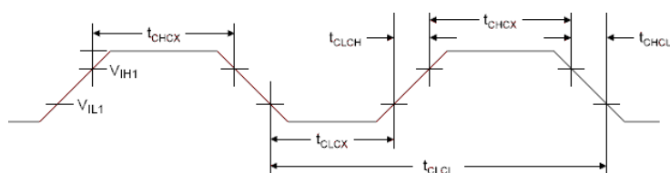
Рисунок 152. Осциллограмма внешнего тактового сигнала
