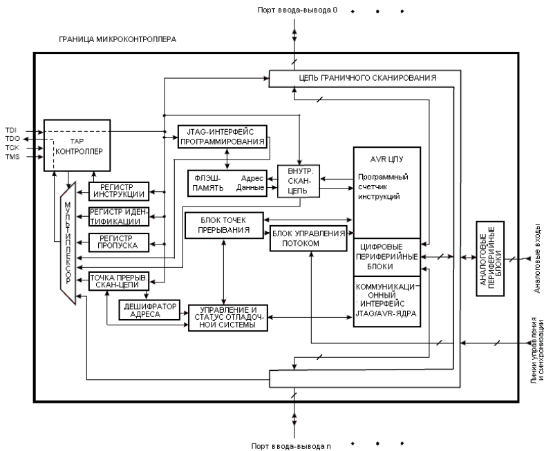
Рисунок 120 √ Функциональная схема интерфейса JTAG и отладочной системы
