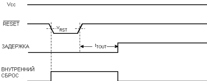
Рисунок 25 √ Внешний сброс микроконтроллера
