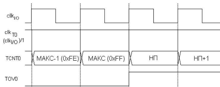
Рисунок 41. Временная диаграмма таймера-счетчика без предделения
