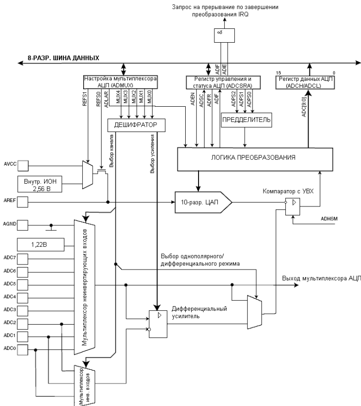
Рисунок 108 - Функциональная схема аналогово-цифрового преобразователя
