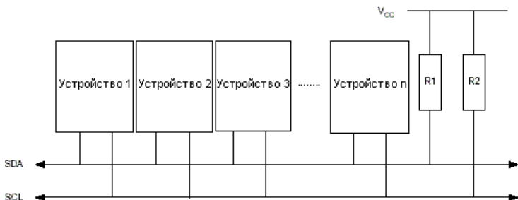
Рисунок 86. Внешние подключения к шине TWI
