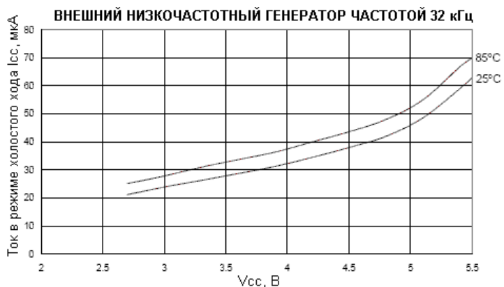
Рисунок 171. Зависимость потребляемого тока в режиме холостого хода (Idle) от напряжения питания (тактирование внешним низкочастотным генератором частотой 32 кГц)
