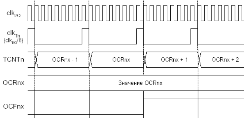
Рисунок 56 √ Временная диаграмма таймера-счетчика с предделением на 8 (fclk_I/O/8) и установкой OCFnx
