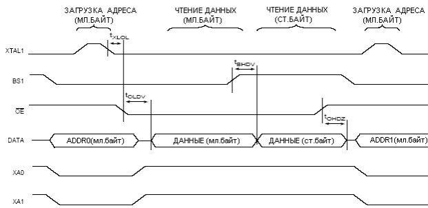
Рисунок 143. Временная диаграмма параллельного программирования: последовательность чтения (в пределах одной страницы)
