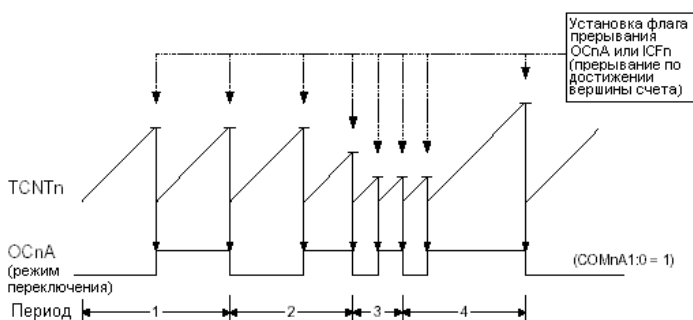
Рисунок 51 √ Временная диаграмма для режима СТС
