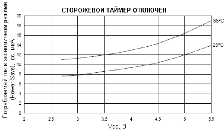
Рисунок 174. Зависимость потребляемого тока в экономичном режиме (Power-save) от напряжения питания (сторожевой таймер отключен)
