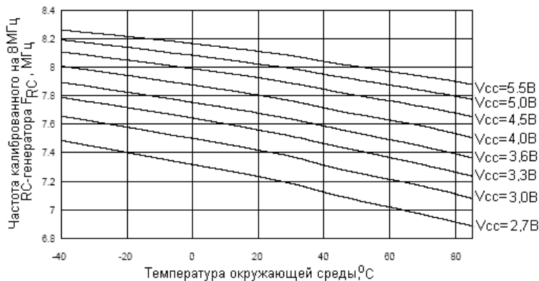
Рисунок 201. Зависимость частоты RC-генератора от температуры (микроконтроллеры откалиброваны на частоту 8МГц при напряжении питания V_{CC} = 5В и температуре T=25\text{ }^{\circ}\text{C} )
