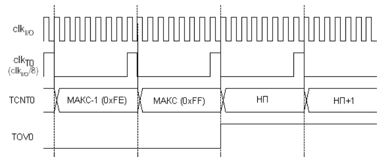
Рисунок 42. Временная диаграмма таймера-счетчика с предделением на 8 (fclk I/O /8)
