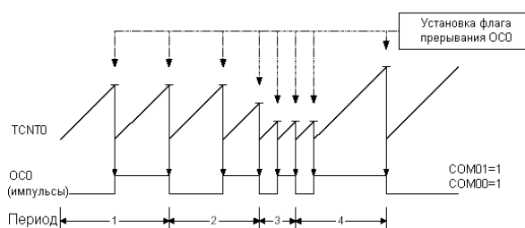
Рисунок 38. Временная диаграмма для режима СТС
