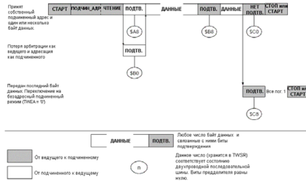
Рисунок 103. Форматы и состояния в режиме подчиненного передатчика
