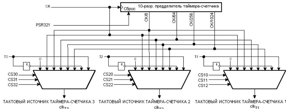
Рисунок 60 √ Предделитель таймеров-счетчиков 1, 2 и 3
