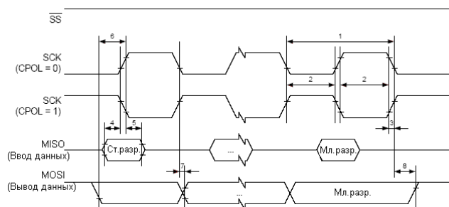
Рисунок 154. Требования к временной диаграмме интерфейса SPI (режим ведущего)
