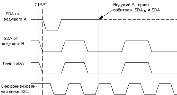
Рисунок 93. Арбитражу двух мастеров
