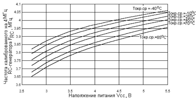
Рисунок 200. Зависимость частоты RC-генератора от напряжения питания (микроконтроллеры откалиброваны на частоту 4 МГц при напряжении питания V_{cc} = 5\text{В} и температуре T=25\text{ }^{\circ}\text{C} )
