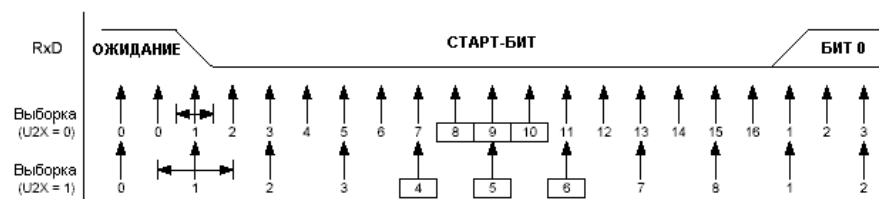
Рисунок 83. Выборка старт-бита
