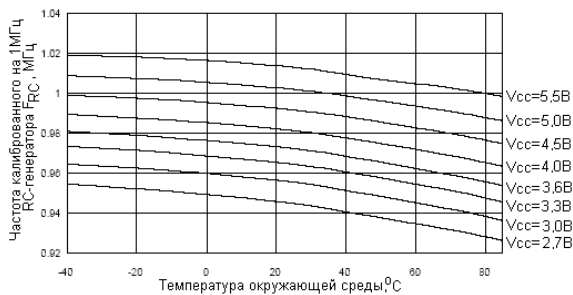
Рисунок 195. Зависимость частоты RC-генератора от температуры (микроконтроллеры откалиброваны на частоту 1МГц при напряжении питания V_{CC} = 5В и температуре T=25\text{ }^{\circ}\text{C} )
