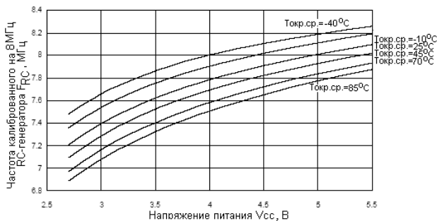
Рисунок 202. Зависимость частоты RC-генератора от напряжения питания (микроконтроллеры откалиброваны на частоту 8МГц при напряжении питания V_{CC} = 5В и температуре T=25\text{ }^{\circ}\text{C} )
