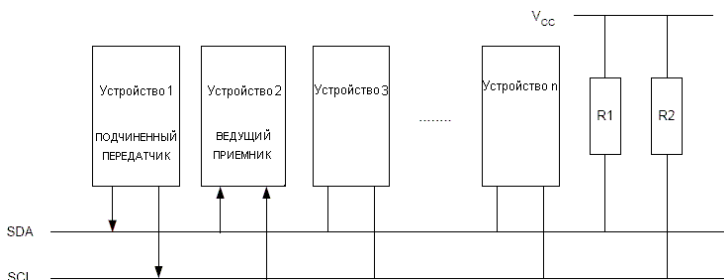
Рисунок 102. Передача данных в режиме подчиненного передатчика
