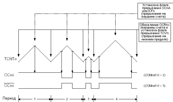
Рисунок 54 \sqrt{\text{Временная диаграмма режима ШИМ с фазовой и частотной коррекцией}}
