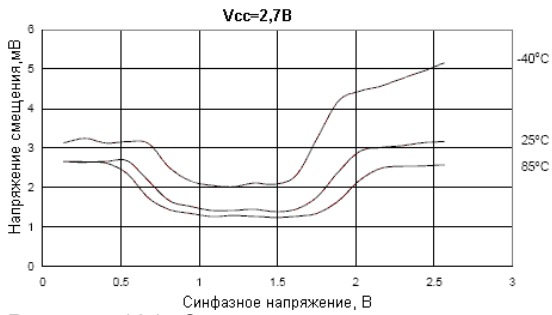
Рисунок 191. Зависимость напряжения смещения аналогового компаратора от синфазного напряжения при напряжении питания V_{CC} = 2,7В
