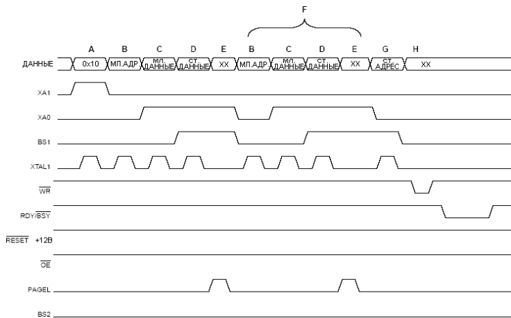
Рисунок 137. Осциллограммы сигналов программирования флэш-памяти
