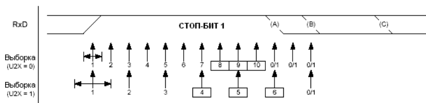
Рисунок 85. Выборка стоп-бита и следующего старт-бита
