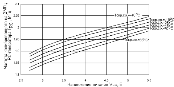
Рисунок 198. Зависимость частоты RC-генератора от напряжения питания (микроконтроллеры откалиброваны на частоту 2 МГц при напряжении питания V_{cc} = 5\text{В} и температуре T=25\text{ }^{\circ}\text{C} )
