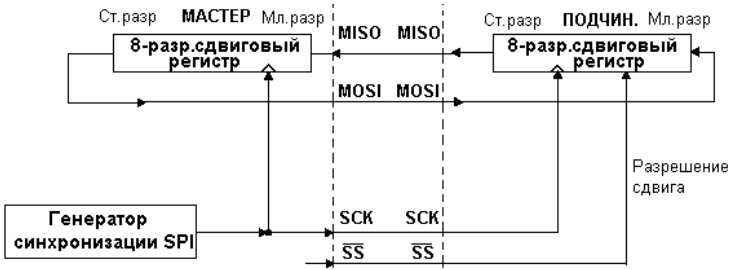
Рисунок 76. Внешнее соединение ведущего (мастера) и подчиненного SPI
