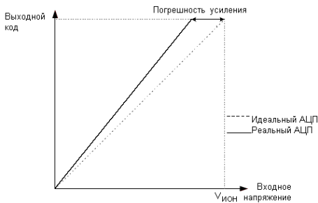
Рисунок 116 √ Погрешность усиления
