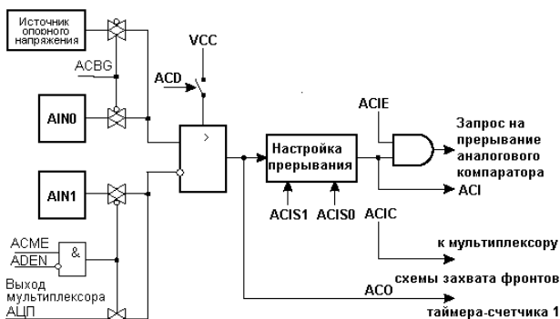
Рисунок 107 √ Функциональная схема аналогового компаратора
