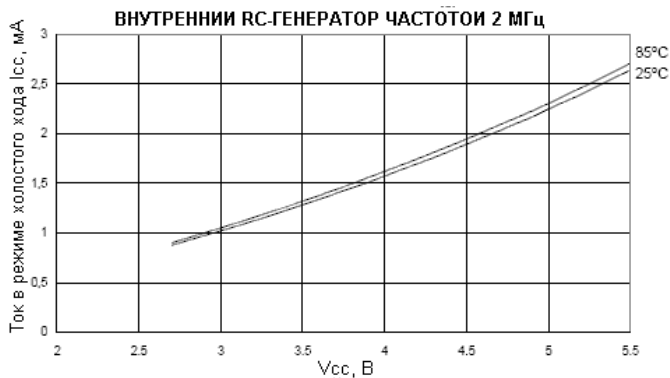
Рисунок 168. Зависимость потребляемого тока в режиме холостого хода (Idle) от напряжения питания (тактирование внутренним RC-генератором частотой 2МГц)
