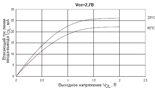
Рисунок 187. Зависимость втекающего тока портов ввода-вывода от выходного напряжения при напряжении питания VCC = 2,7В
