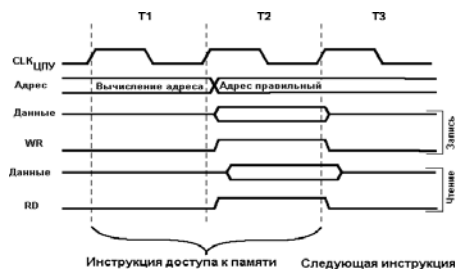
Рисунок 10 Временная диаграмма доступа к встроенному статическому ОЗУ данных
