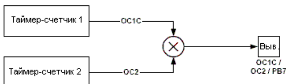
Рисунок 72. Принцип выполнения модуляции
