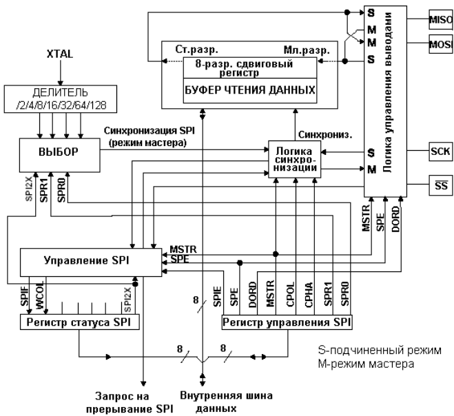
Рисунок 75. Функциональная схема интерфейса SPI
