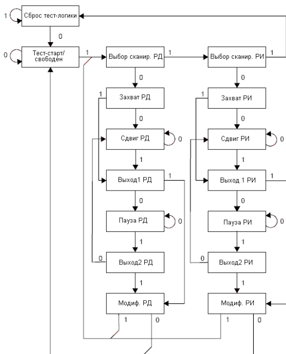
Рисунок 121 √ Граф-автомат TAP-контроллера
