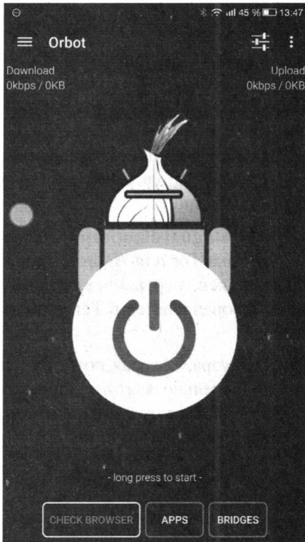
Рис. 5.1. OrBot
