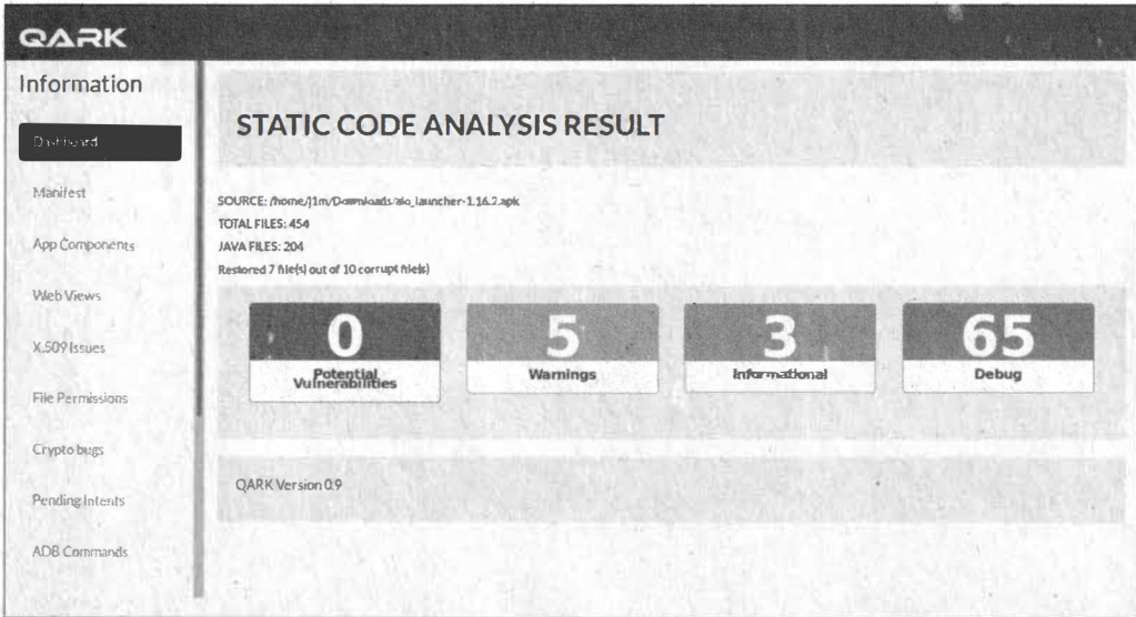
Рис. 11.5. Отчет Qark
