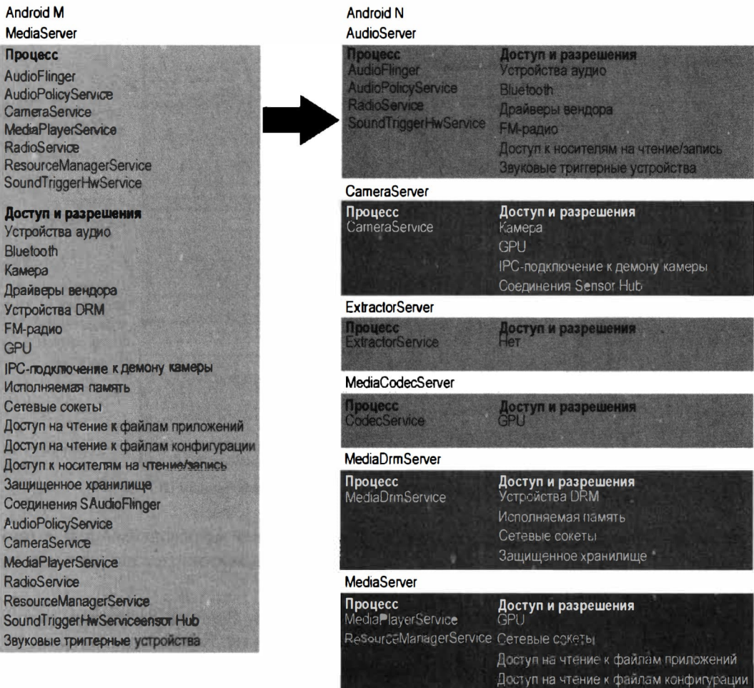
Рис. 4.8. Разделенный MediaServer
