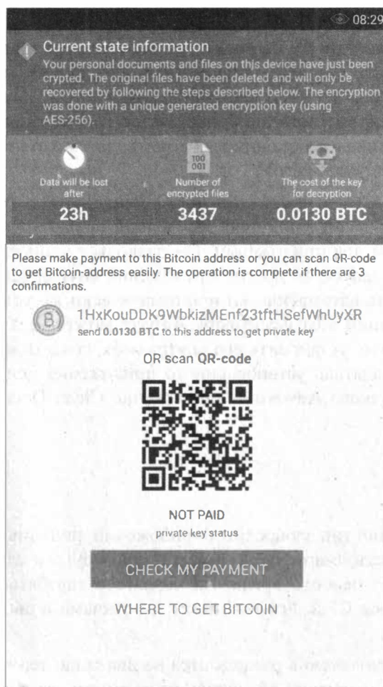
Рис. 12.6. Сообщение DoubleLocker
