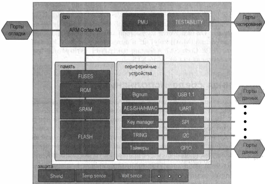
Рис. 4.5. Titan M
