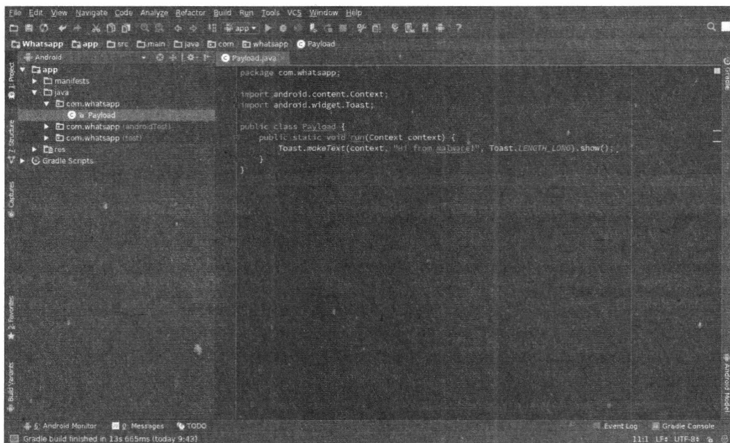
Рис. 7.3. Простейший payload
