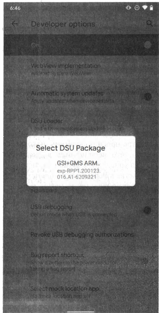
Рис. 3.4. DSU Loader
