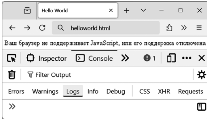
Рис. 13.2. JavaScript отключен
